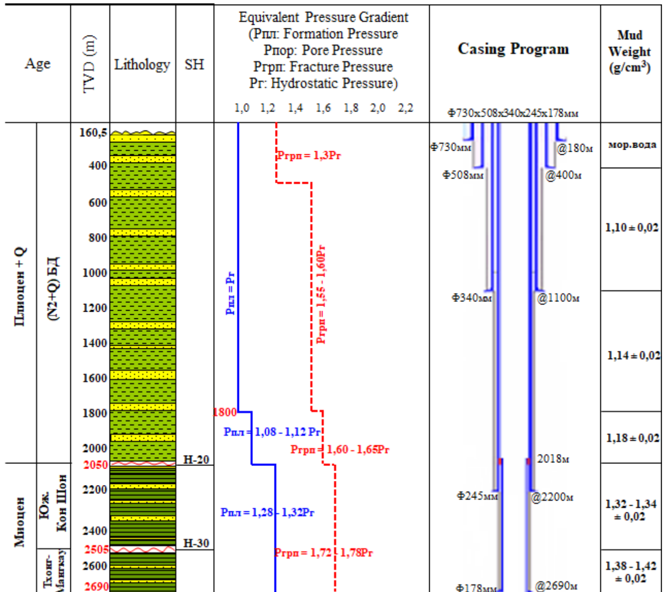
COMBINED PRESSURE GRAPH of THE WELL № TU-16 BLOCK 04-3. (По вертикали от роторного стола)
