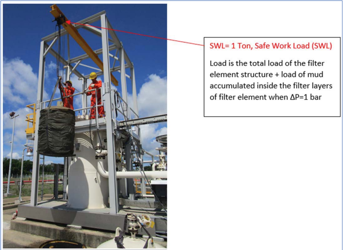
Figure 7: Thiết kế và cấu tạo hiện tại của các thiết bị nâng trên thiết bị lọc F-7907A/B
