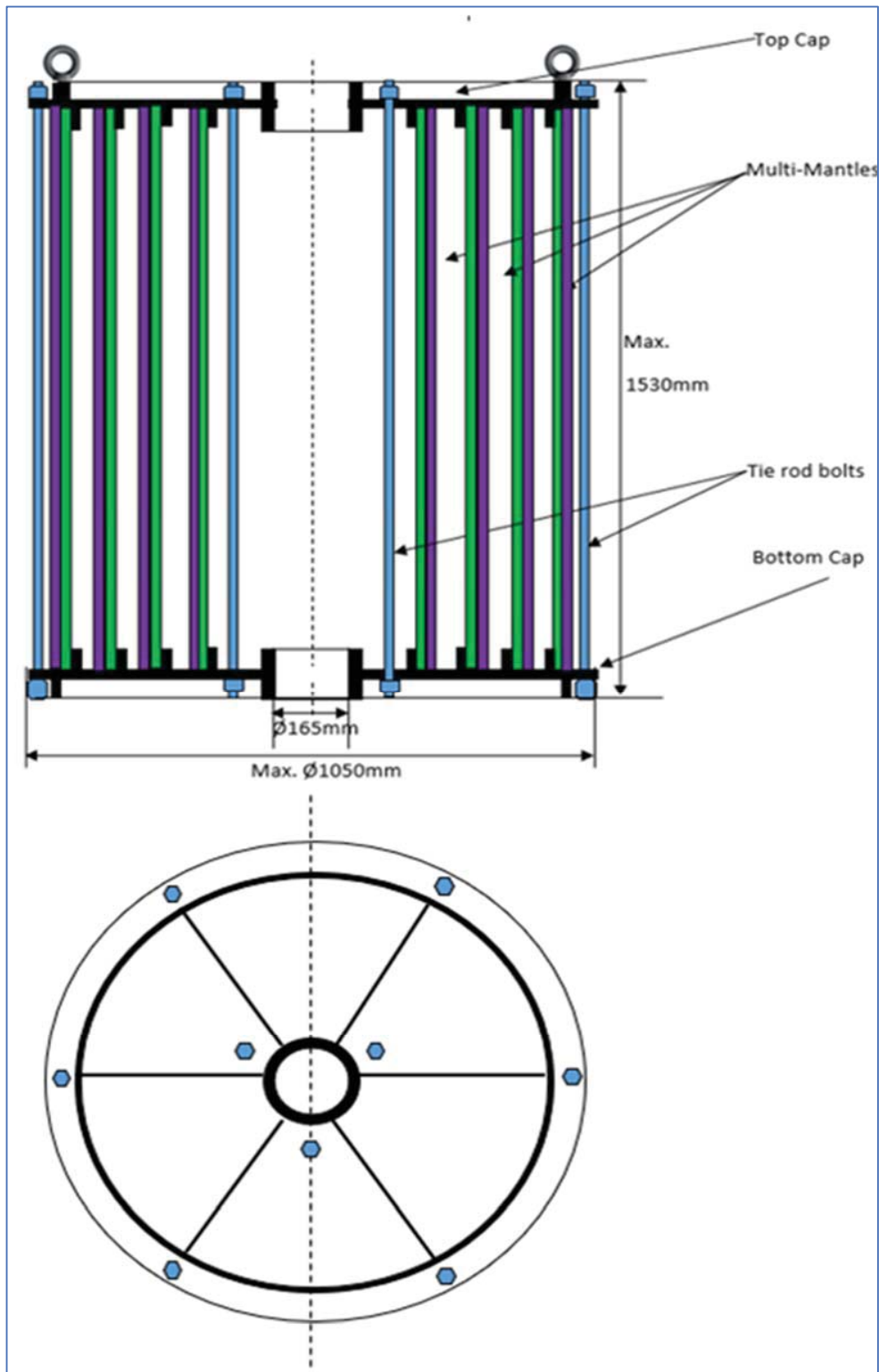
Figure 5: Cấu trúc tổng quan của lõi lọc mới
