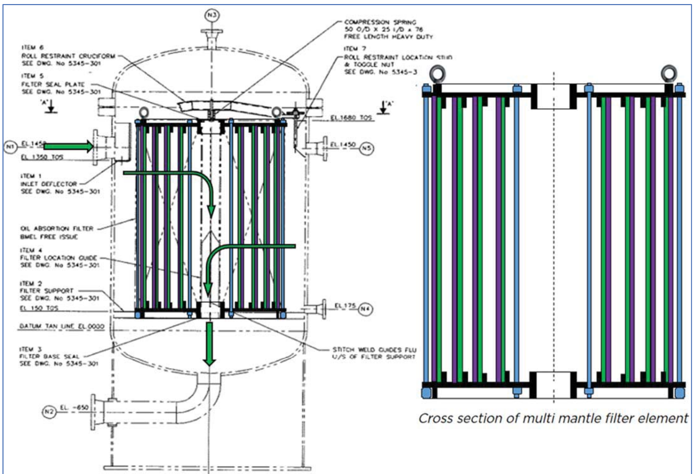
Figure 3: Cấu tạo lỗi lọc mới cho thiết bị lọc hấp thụ dầu F7907A/B
