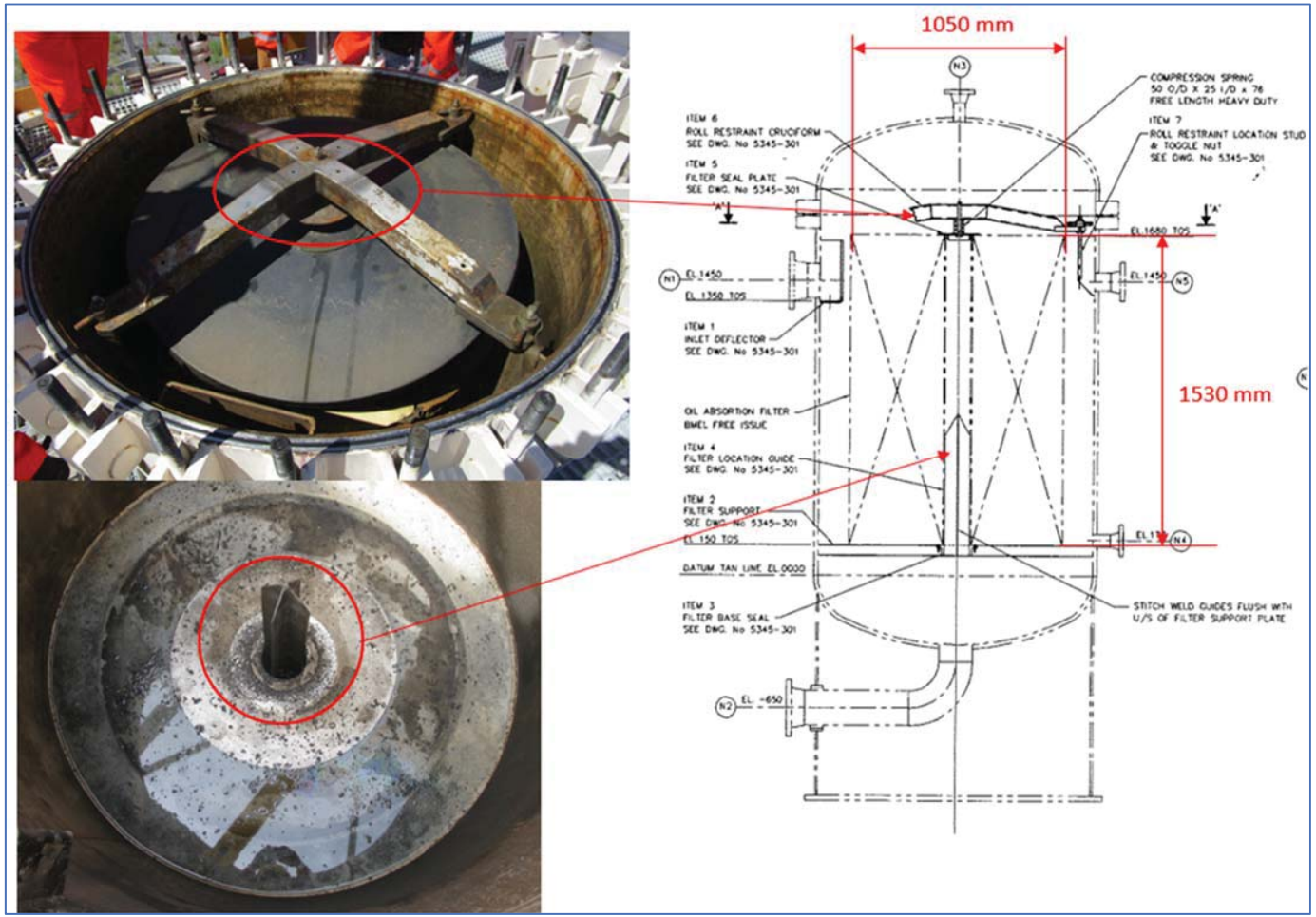
Figure 6: Thiết kế và cấu tạo hiện hữu của thiết bị lọc hấp thụ dầu F7907A/B
