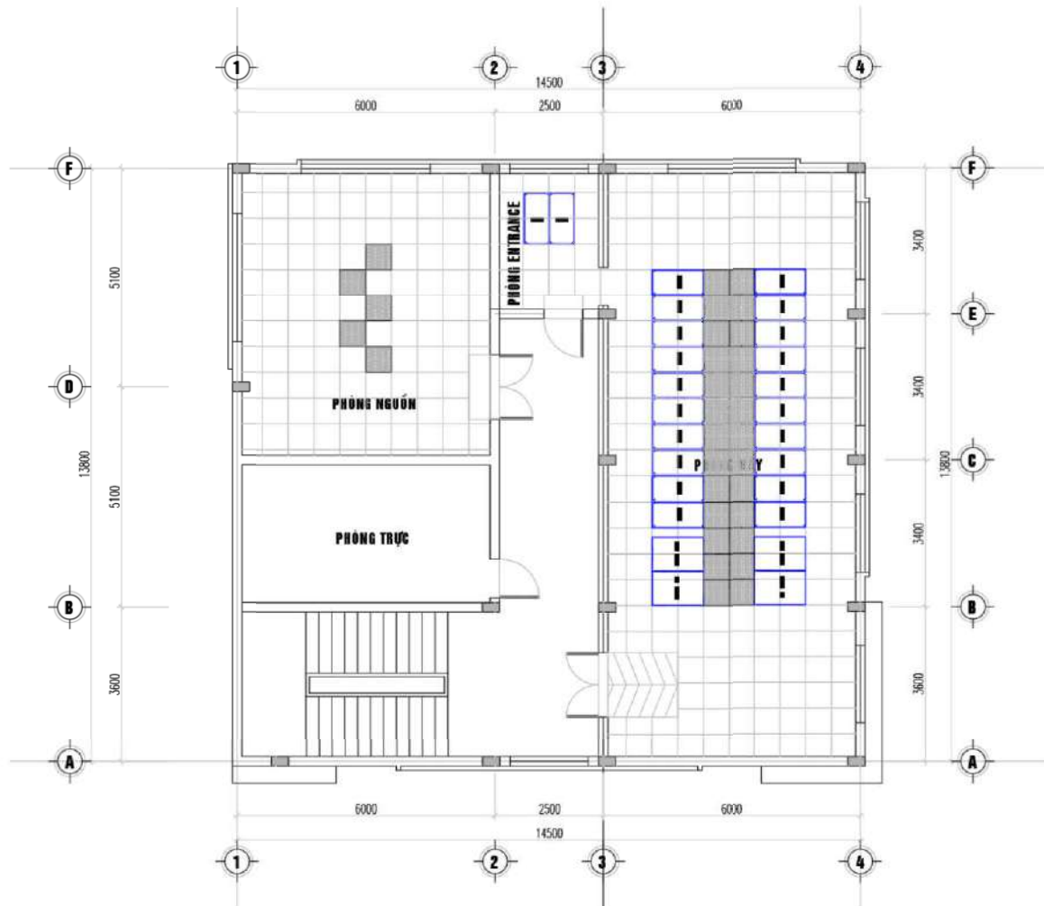
Mặt bằng tủ Rack
