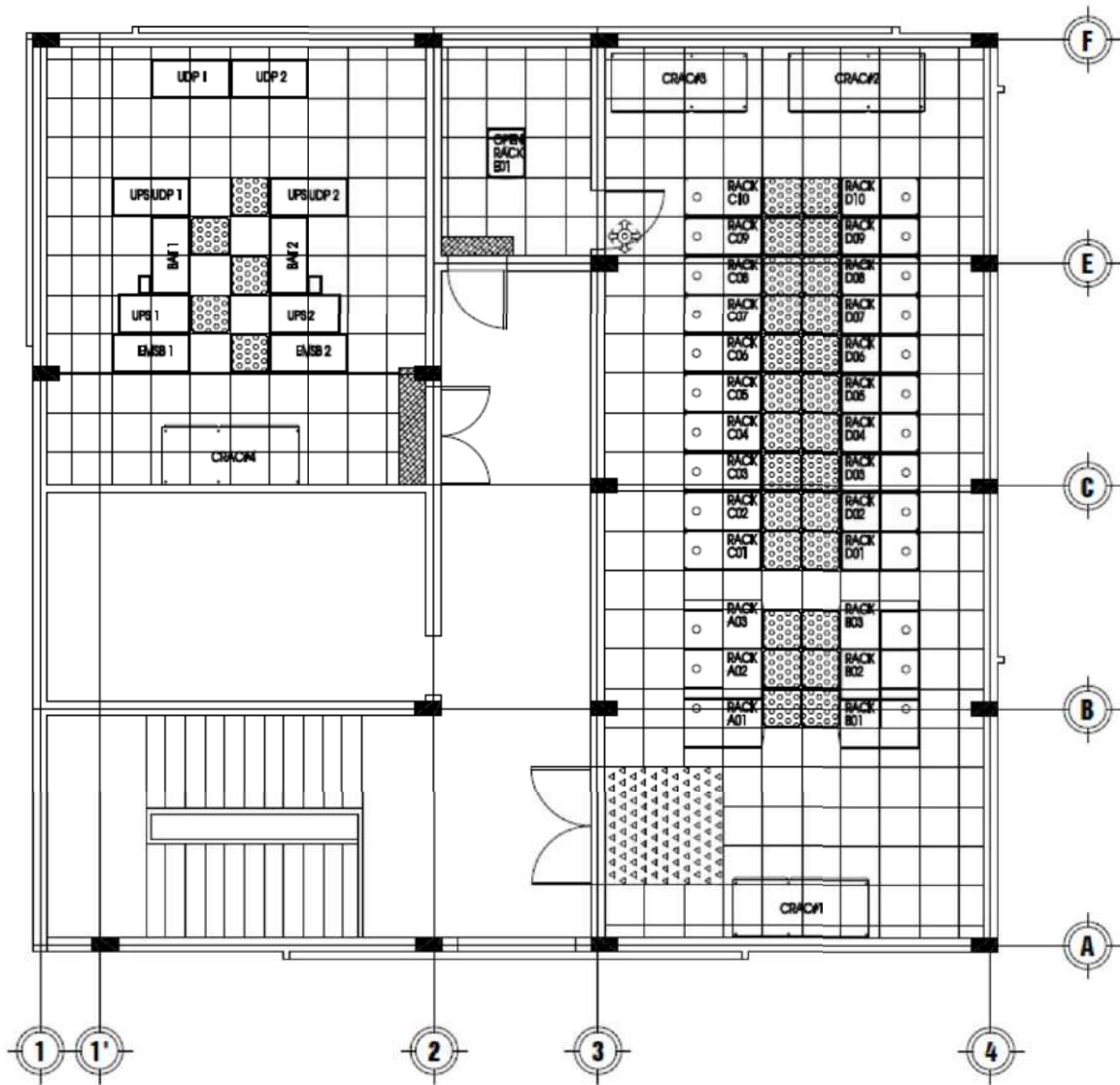
Mặt bằng tổng thể thiết bị TTL
