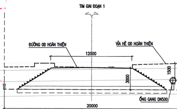
MẶT CẮT NGANG ĐIỂN HÌNH 4-4
