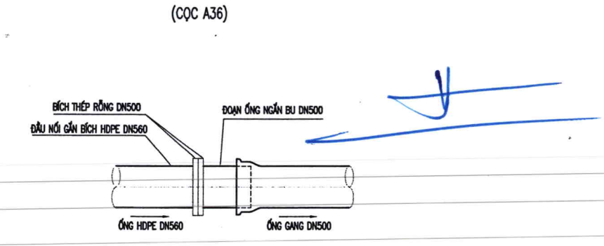
CHI TIẾT ĐẦU NỐI ỐNG HDPE VÀ ỐNG GANG (CỌC A36)
