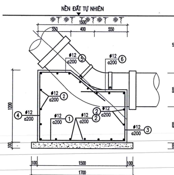
MẶT CẮT 1 CỐT THÉP GỐI ĐỖ
