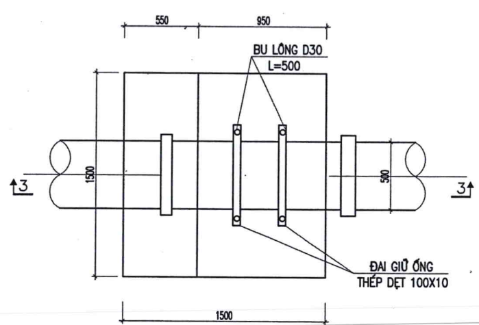
GỐI ĐỖ HƯỚNG XUỐNG 45 ỚNG D500
