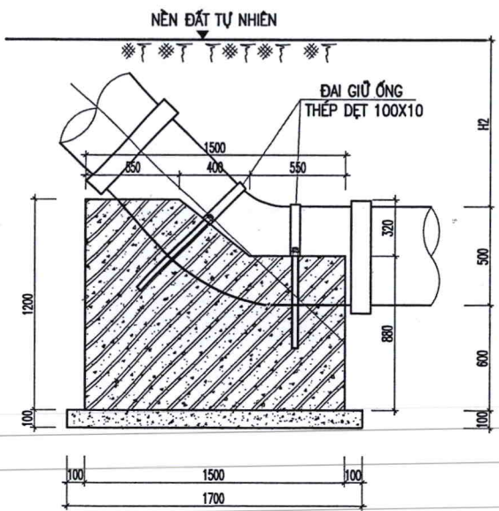
MẶT CẮT 1-1
