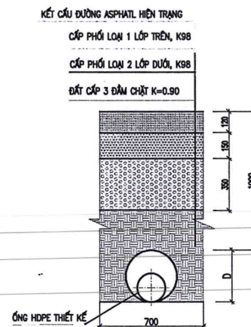
MẶT CẮT MƯƠNG ĐẶT ỚNG
