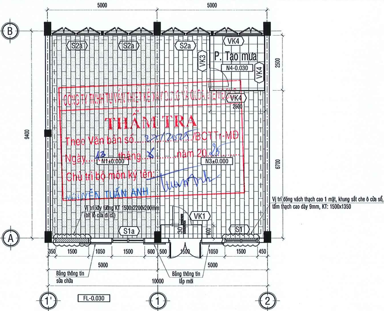
MẶT BẰNG LÁT GẠCH TL: 1/100
