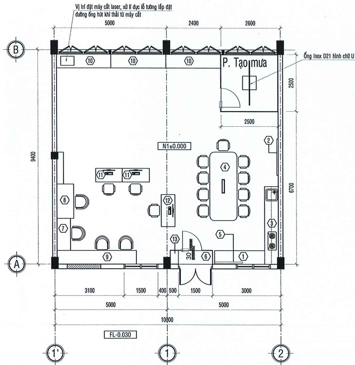
MẶT BẰNG NỘI THẤT TL: 1/100 SỬA CHỮA
