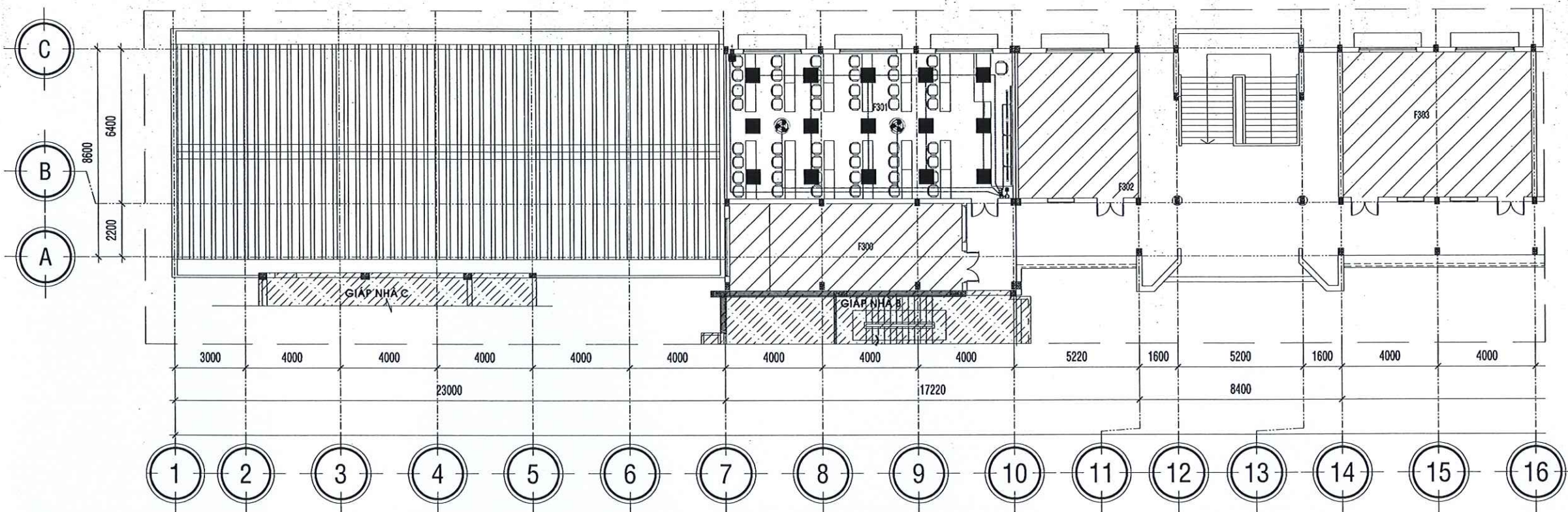
MẶT BẰNG CHIẾU SÁNG LẦU 3 NHÀ F (PHÒNG F-301) TL: 1/200
