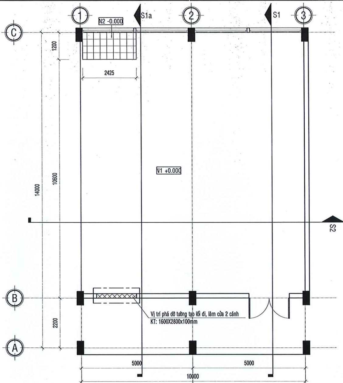
MẶT BẰNG HIỆN TRẠNG TL: 1/100
