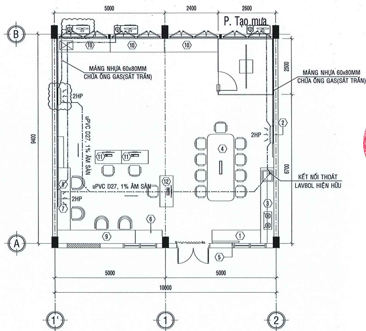
MB BỐ TRÍ ỚNG GAS, NƯỚC NGỪNG MÁY LẠNH TL: 1/100 SỬA CHỮA
