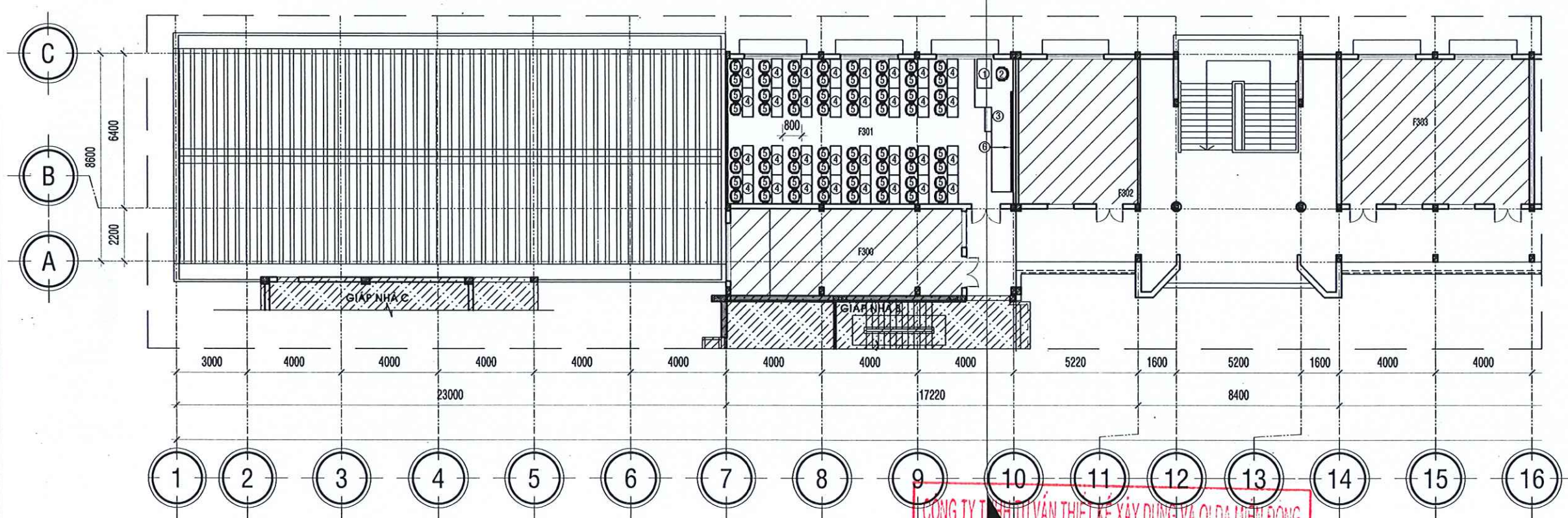
MẶT BẰNG NỘI THẤT LẦU 3 TL: 1/200
