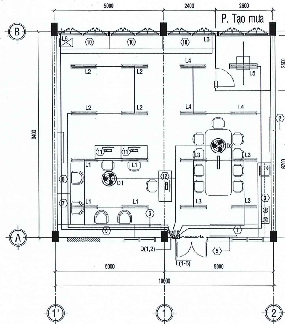
MẶT BẰNG BỐ TRÍ CHIẾU SÁNG TL: 1/100 SỬA CHỮA
