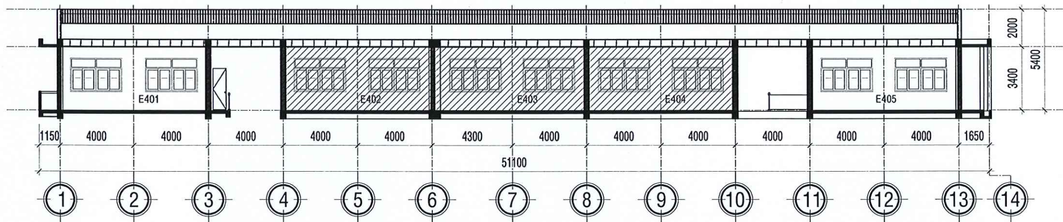
MẶT CẮT S2 TL: 1/200
