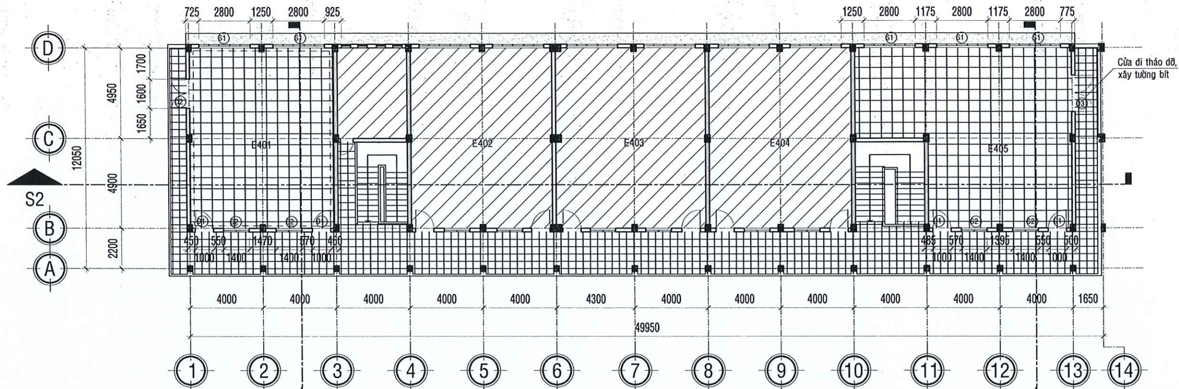
MẶT BẰNG TẦNG 5 HIỆN TRẠNG TL: 1/200
