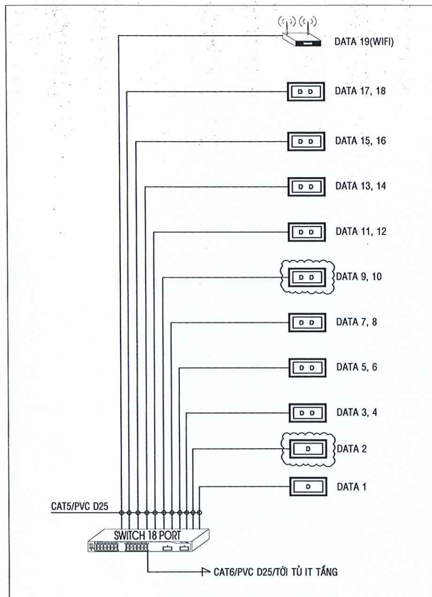
SƠ ĐỒ NGUYÊN LÝ HỆ THỐNG DATA
