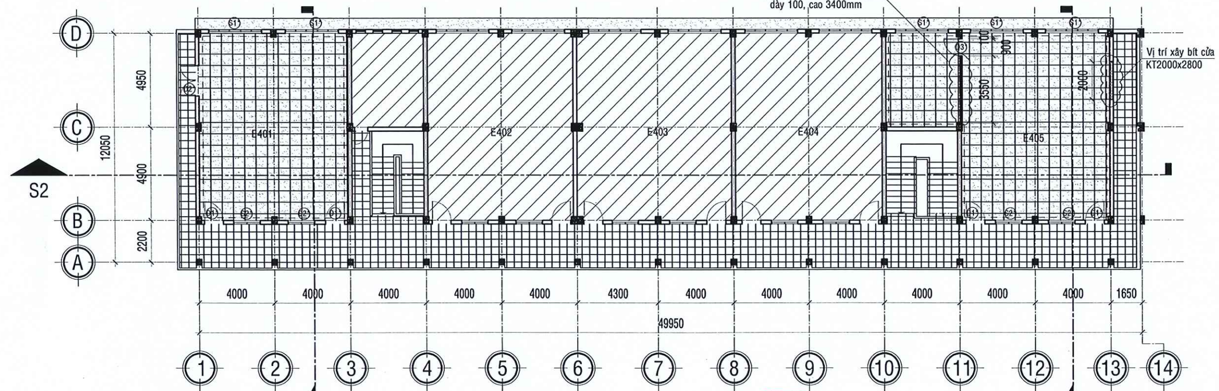
MẶT BẰNG TẦNG 5 SỬA CHỮA TL: 1/200
