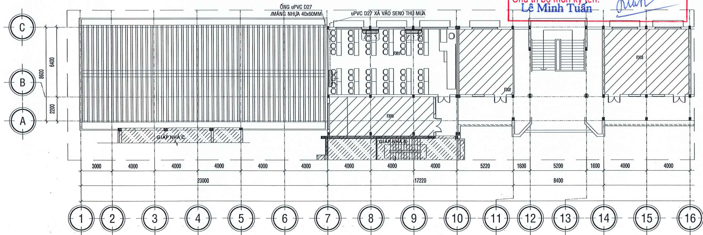
MẶT BẰNG CẤP ỚNG NƯỚC NGỪNG LẦU 3 NHÀ F (PHÒNG F-301) TL: 1/200
