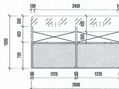
MẶT ĐỨNG TL: 1/50
