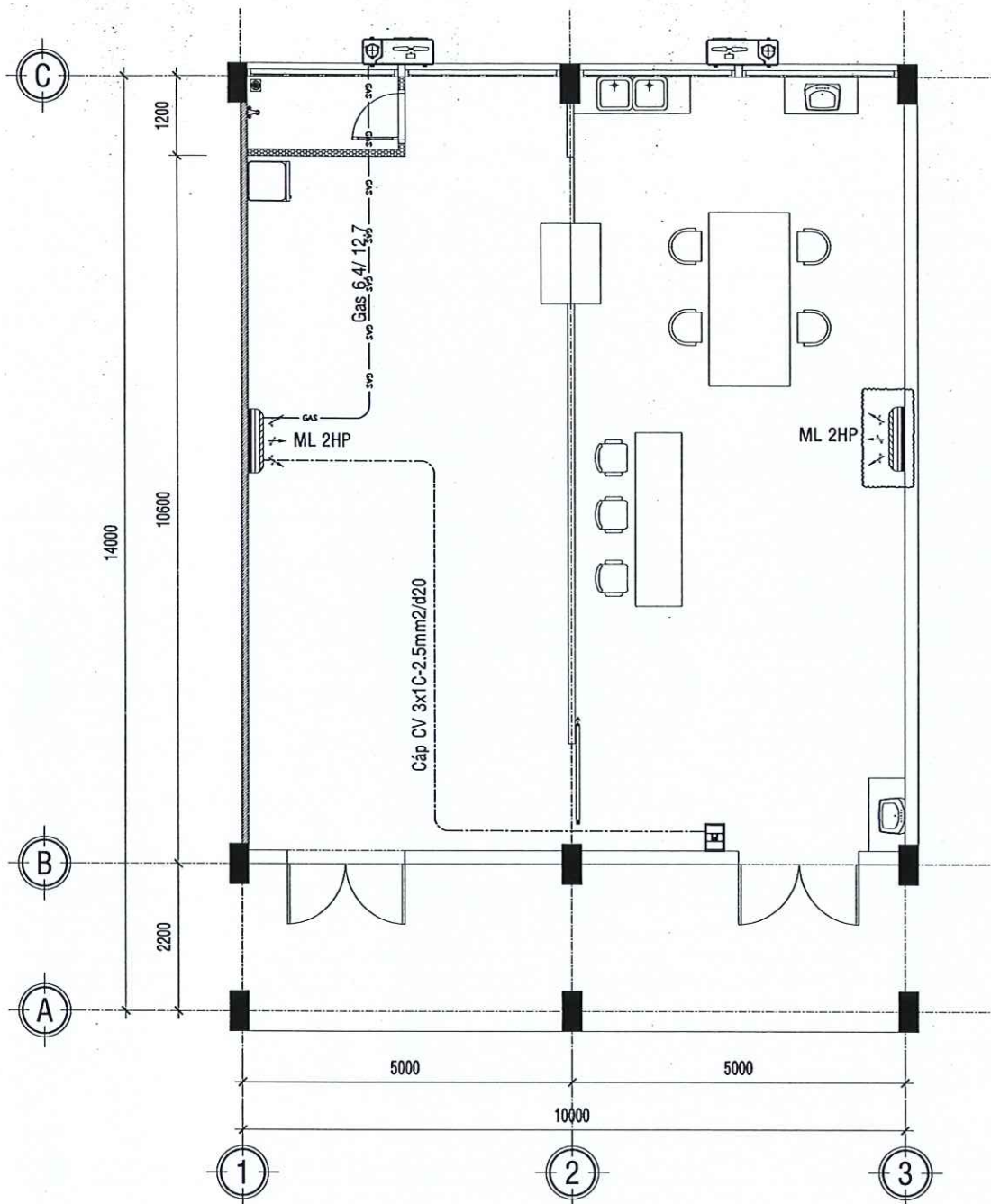
MẶT BẰNG CẤP NGUỒN MÁY LẠNH, ỐNG GAS P.Y TẾ TL: 1/100 SỬA CHỮA
