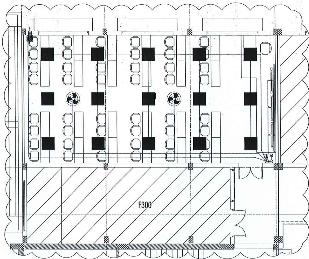
MB CHI TIẾT CHIẾU SÁNG PHÒNG F 301
