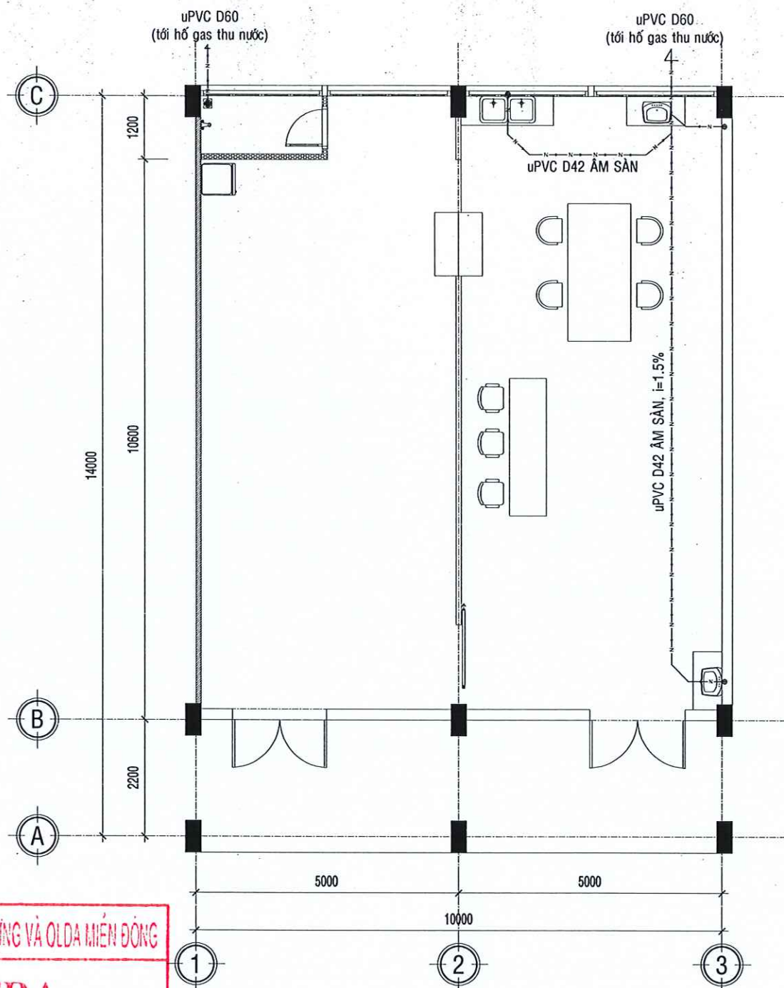
MẶT BẰNG THOÁT NƯỚC P. Y TẾ SỬA CHỮA
