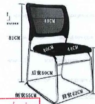
MẪU GHẾ SINH VIÊN
