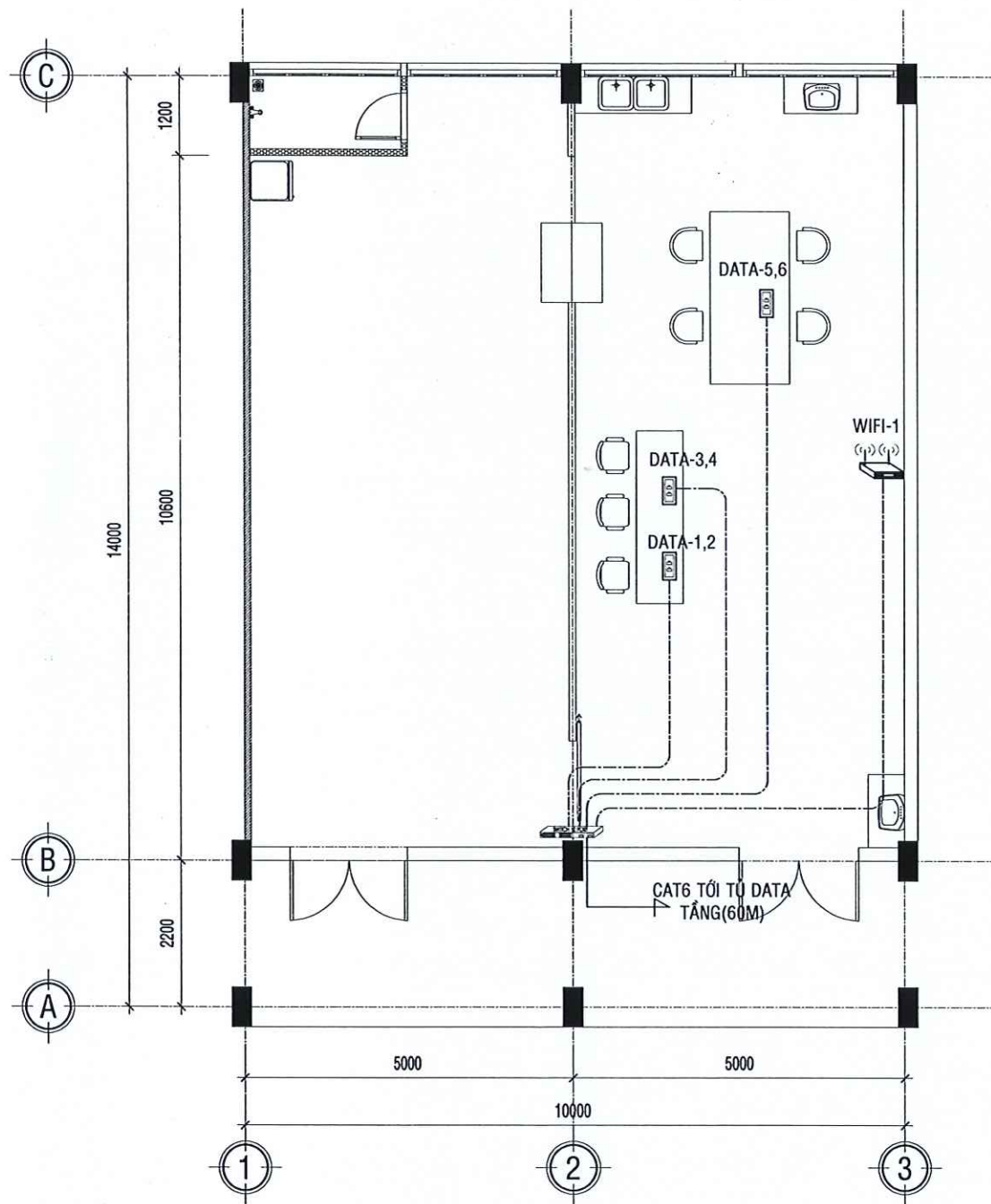
MẶT BẰNG DATA P. Y TẾ TL: 1/100 SỬA CHỮA
