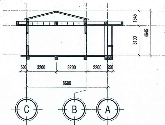
MẶT CẮT S1 TL: 1/200
