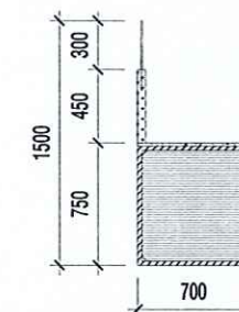
MẶT BÊN TL: 1/50
