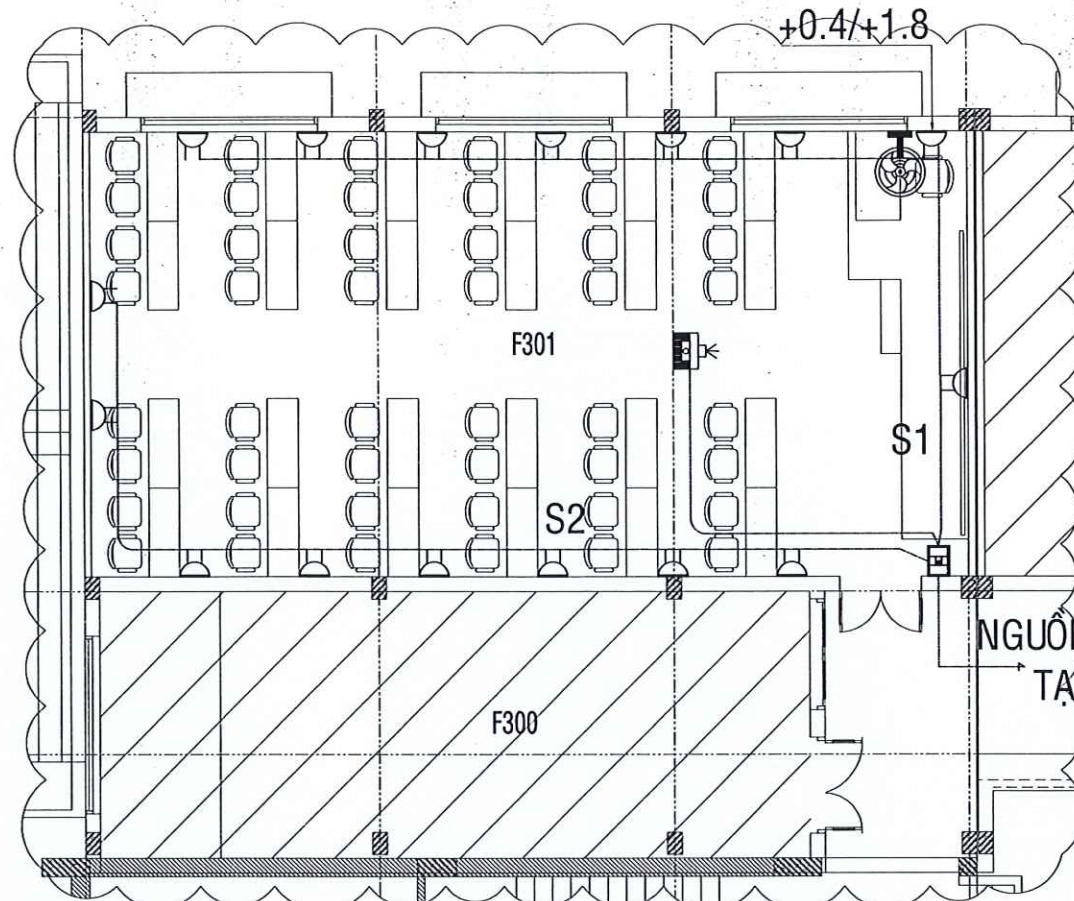
MB CHI TIẾT CẤP NGUỒN PHÒNG F 301
