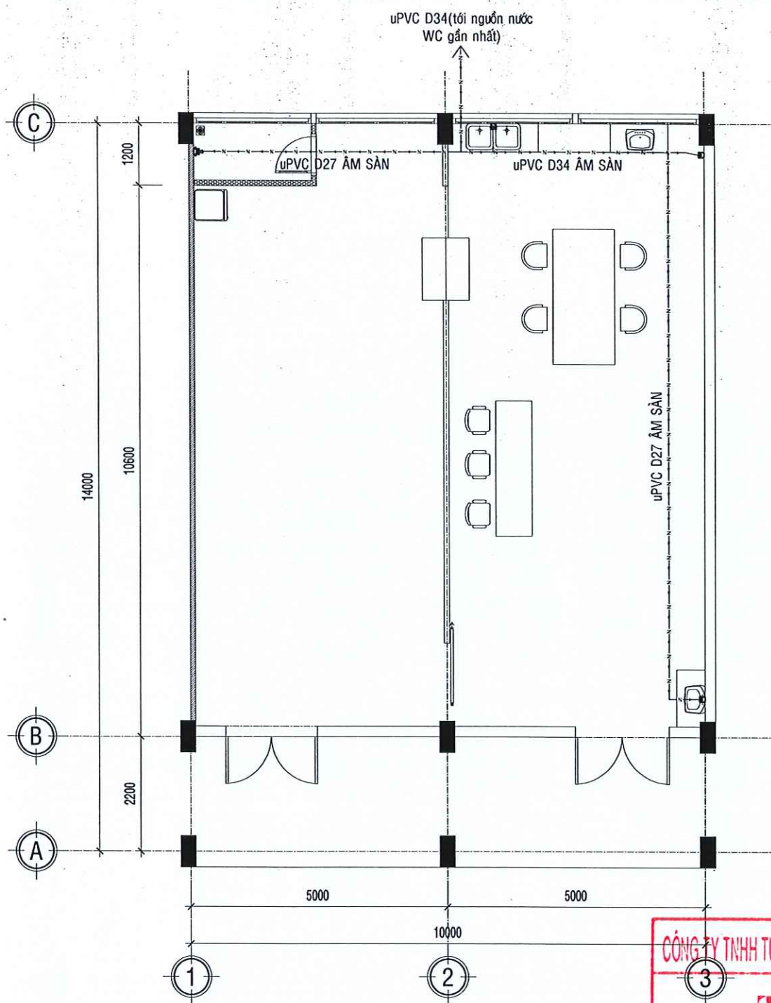
MẶT BẰNG CẤP NƯỚC P. Y TẾ SỬA CHỮA
