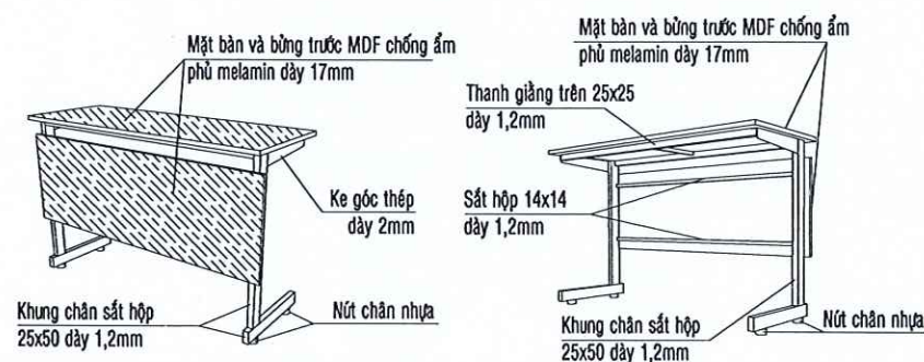
CHI TIẾT BÀN SINH VIÊN TL: 1/50
