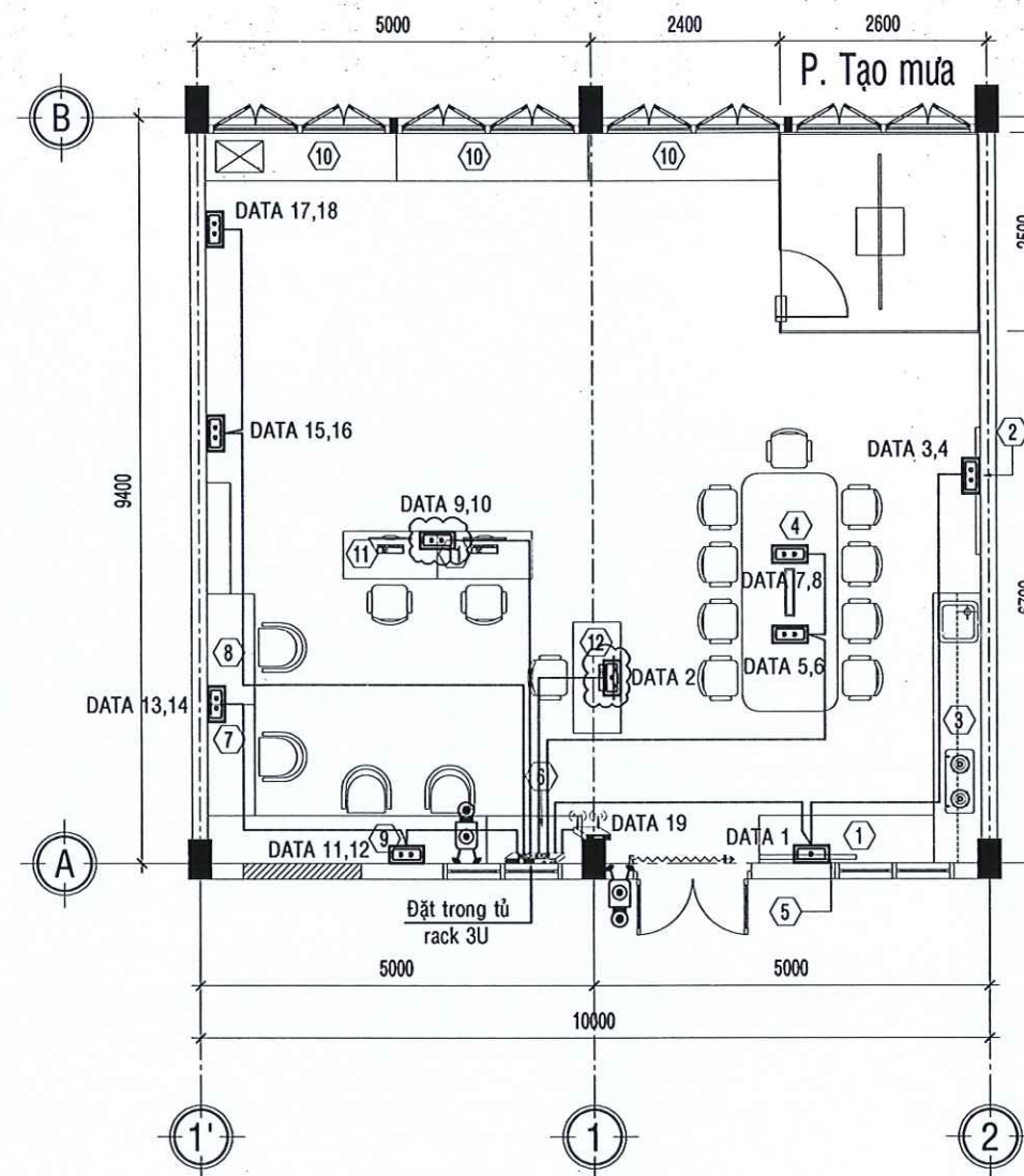
MẶT BẰNG BỐ TRÍ HỆ DATA-CAMERA TL: 1/100 SỬA CHỮA
