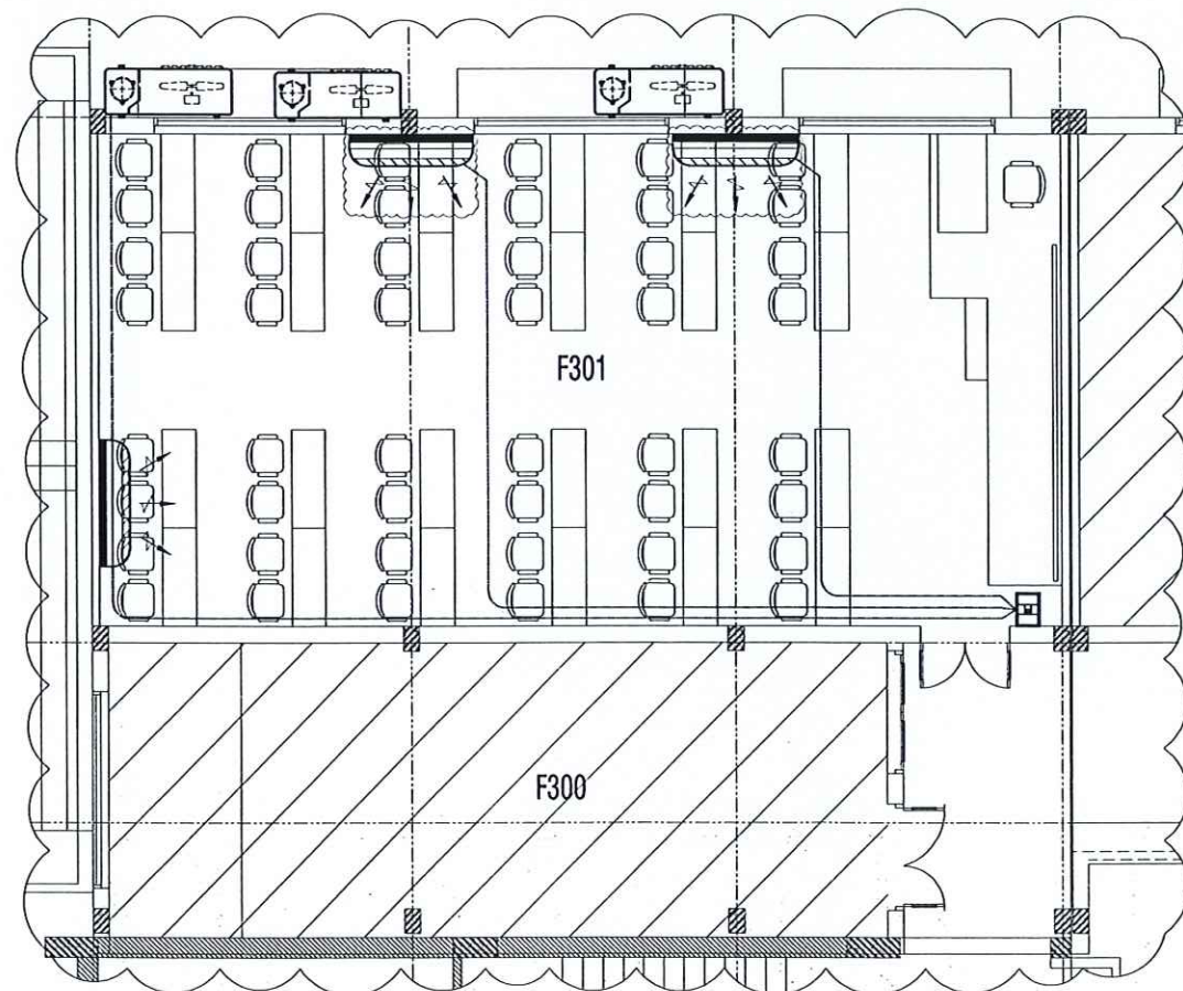
MB CHI TIẾT CẤP NGUỒN ĐHKK PHÒNG F 301
