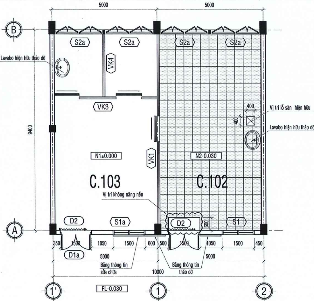
MẶT BẰNG PHÒNG C.102, C.103 TL: 1/100
