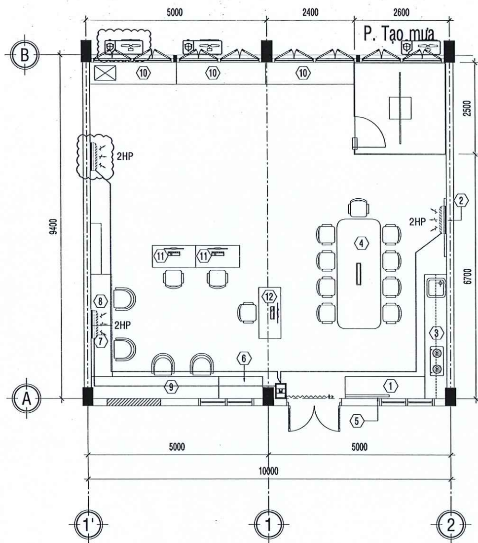
MẶT BẰNG BỐ TRÍ CẤP NGUỒN MÁY LẠNH TL: 1/100 SỬA CHỮA
