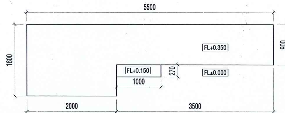
CHI TIẾT BỤC GIẢNG TL: 1/50
