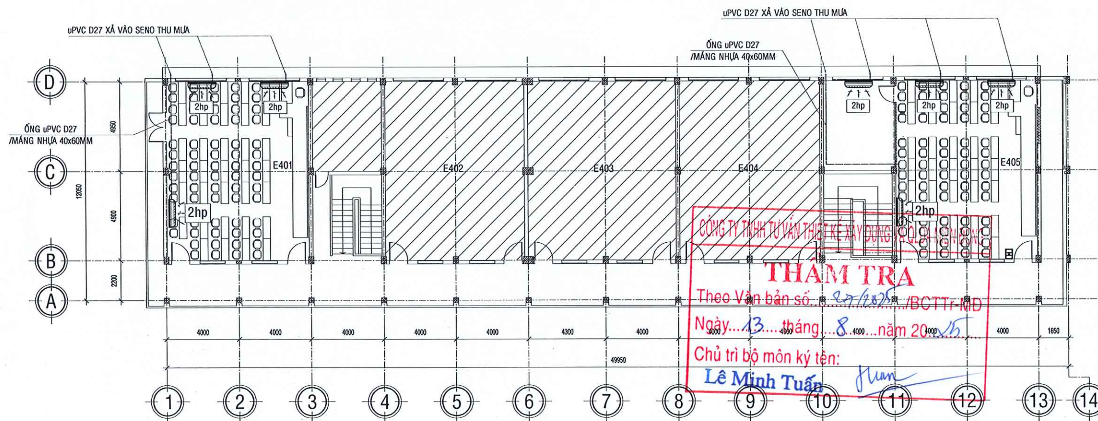
MẶT BẰNG CẤP NGUỒN VÀ ỐNG GAS ĐIỀU HÒA KHÔNG KHÍ TẦNG 5 TL: 1/200
