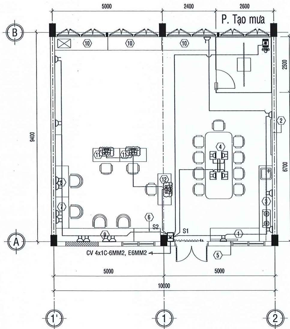
MẶT BẰNG BỐ TRÍ CẤP NGUỒN TL: 1/100 SỬA CHỮA
