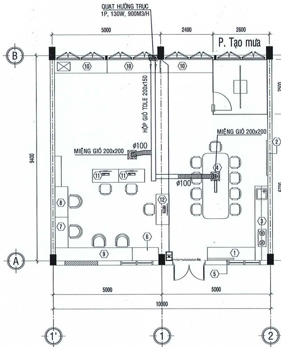
MẶT BẰNG BỐ TRÍ LỘC KHÔNG KHÍ ĐHKK TL: 1/100 SỬA CHỮA
