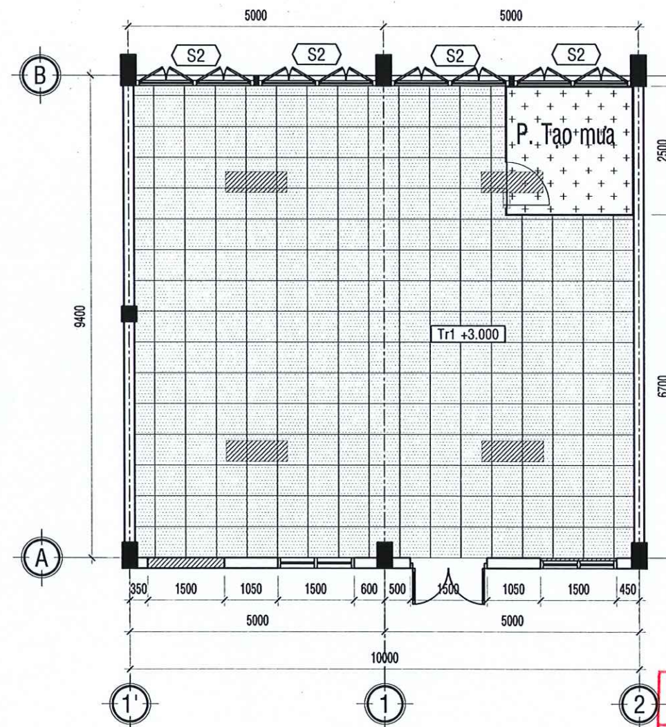
MẶT BẰNG TRẦN TL: 1/100 SỬA CHỮA
