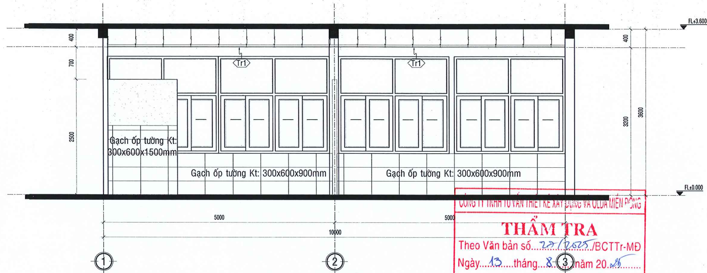
MẶT CẮT S2 TL: 1/50 SỬA CHỮA
