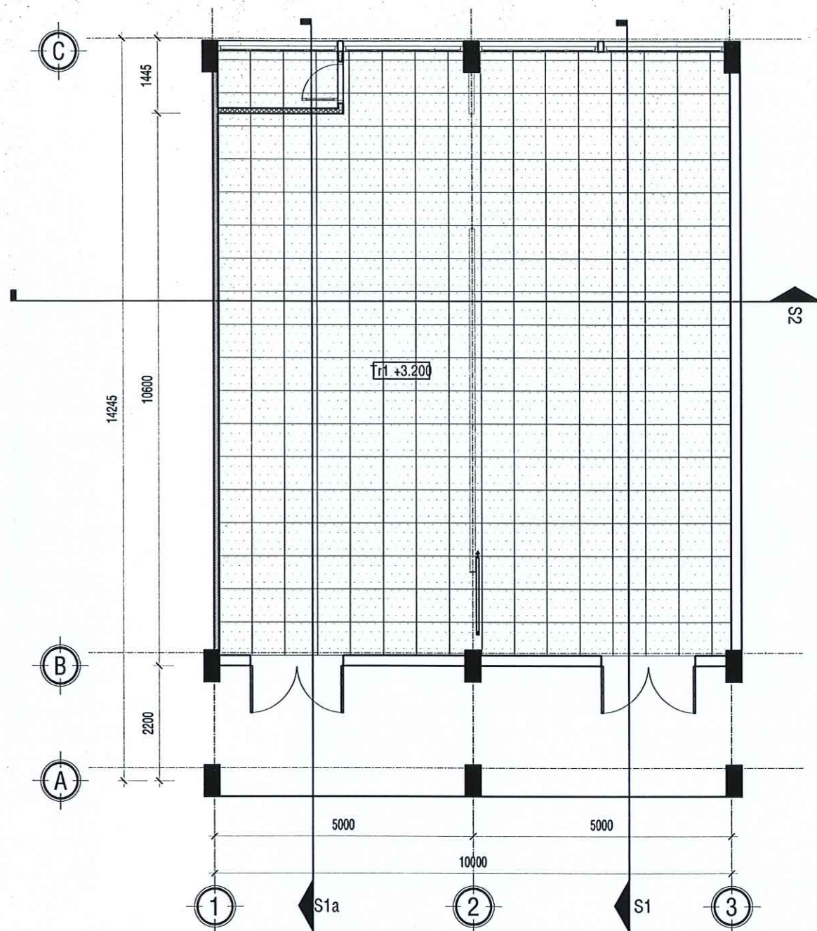
MẶT BẰNG TRẦN Y TẾ SỬA CHỮA TL: 1/100
