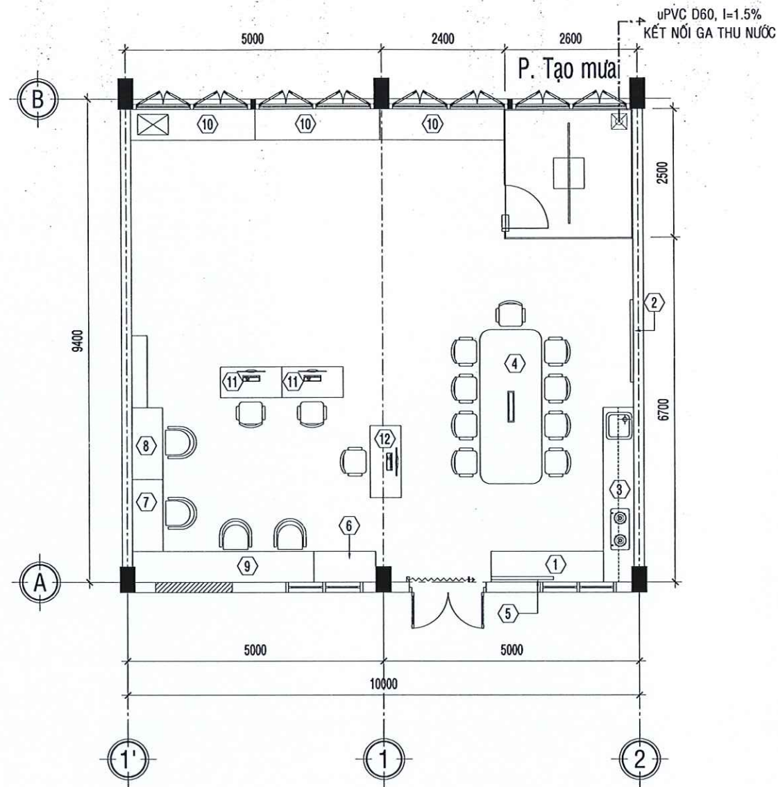
MB BỐ TRÍ CẤP NƯỚC PHÒNG TẠO MƯA TL: 1/100 SỬA CHỮA
