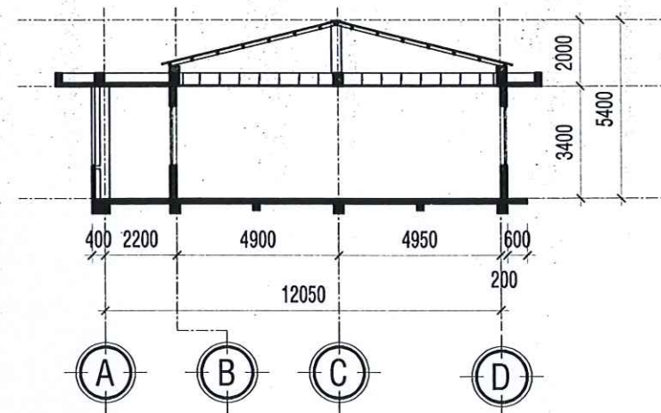
MẶT CẮT S1 TL: 1/200
