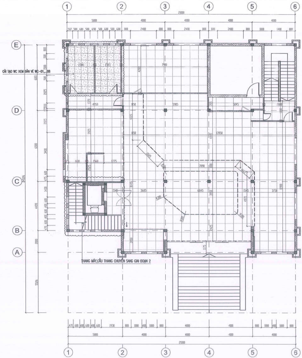
MB SÀN CẢI TẠO TẦNG 1
