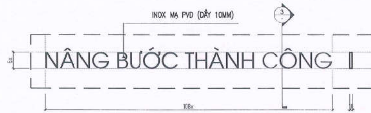
CHI TIẾT CHỮ NHẬN ĐIỆN THƯƠNG HIỆU MẶT CẮT 3-3
