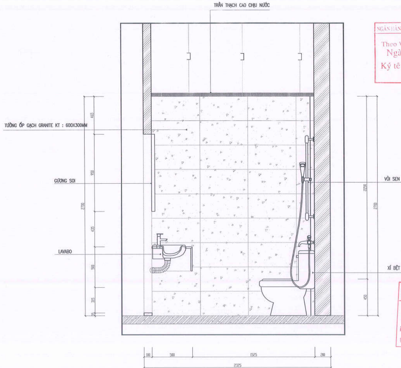
MẶT ĐỪNG HƯỚNG NHÌN A
