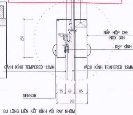
CHI TIẾT 1
