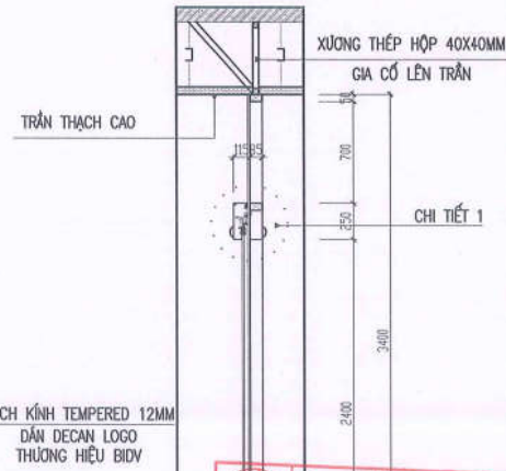
CHI TIẾT 1
