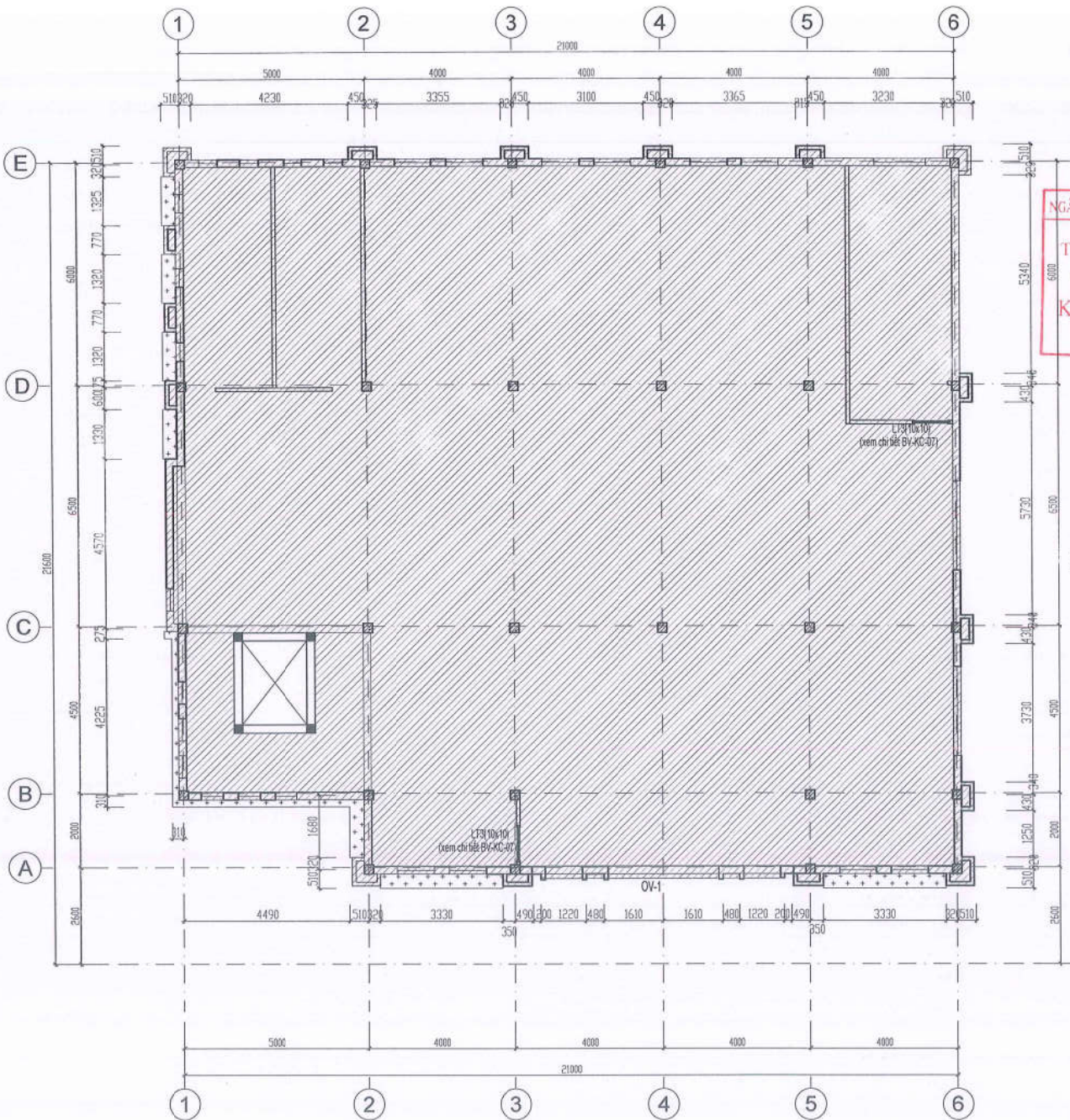
MẶT BẰNG KẾT CẤU TẦNG 3
