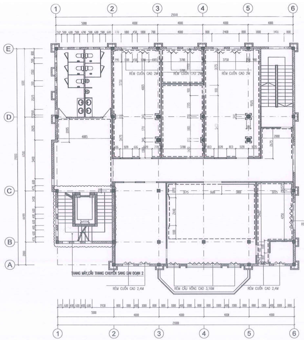
MB PHÀO CỎ TRẦN + RÈM TẦNG 3
