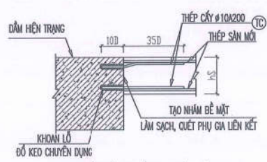
CHI TIẾT CÂY SÀN MỚI VÀO DẪM HIỆN TRẠNG
