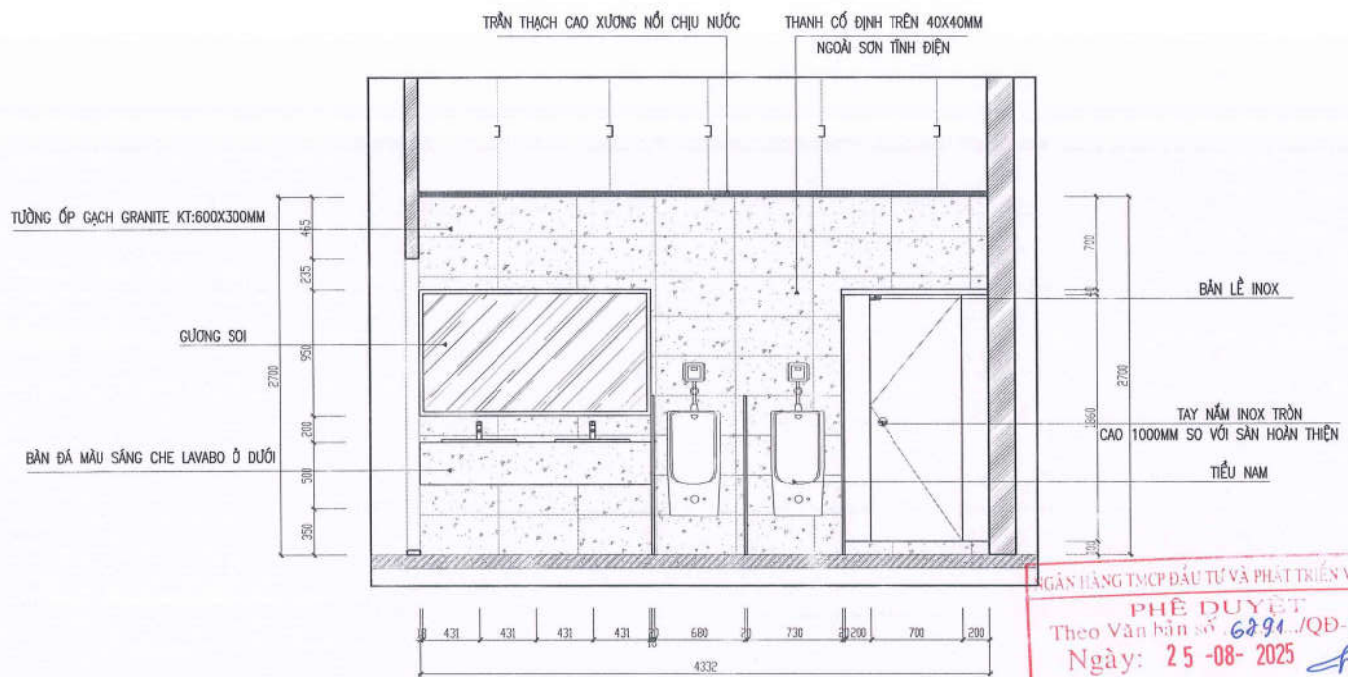
MẶT ĐỨNG HƯỚNG NHÌN D
