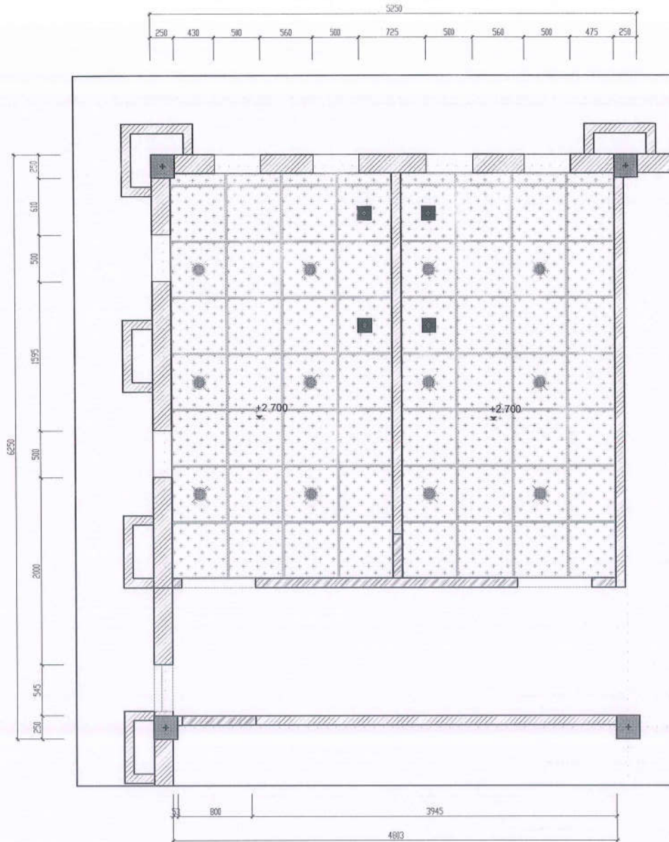
MẶT BẰNG TRẦN CẢI TẠO WC T1
