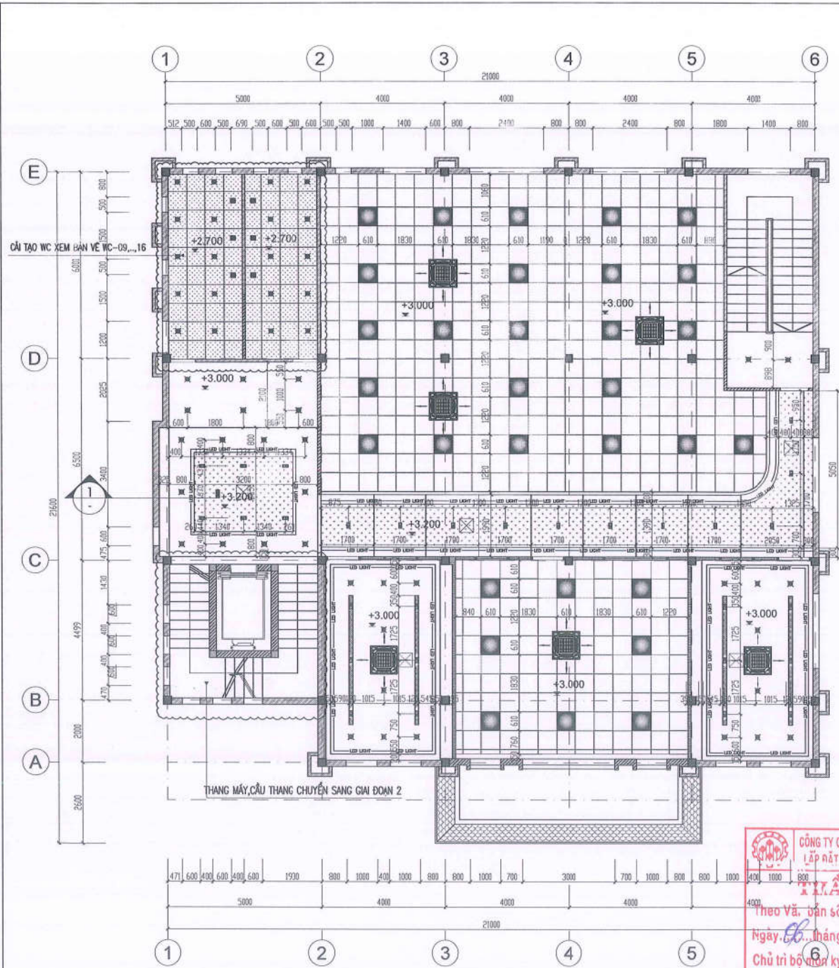
MB TRẦN CẢI TẠO TẦNG 2
