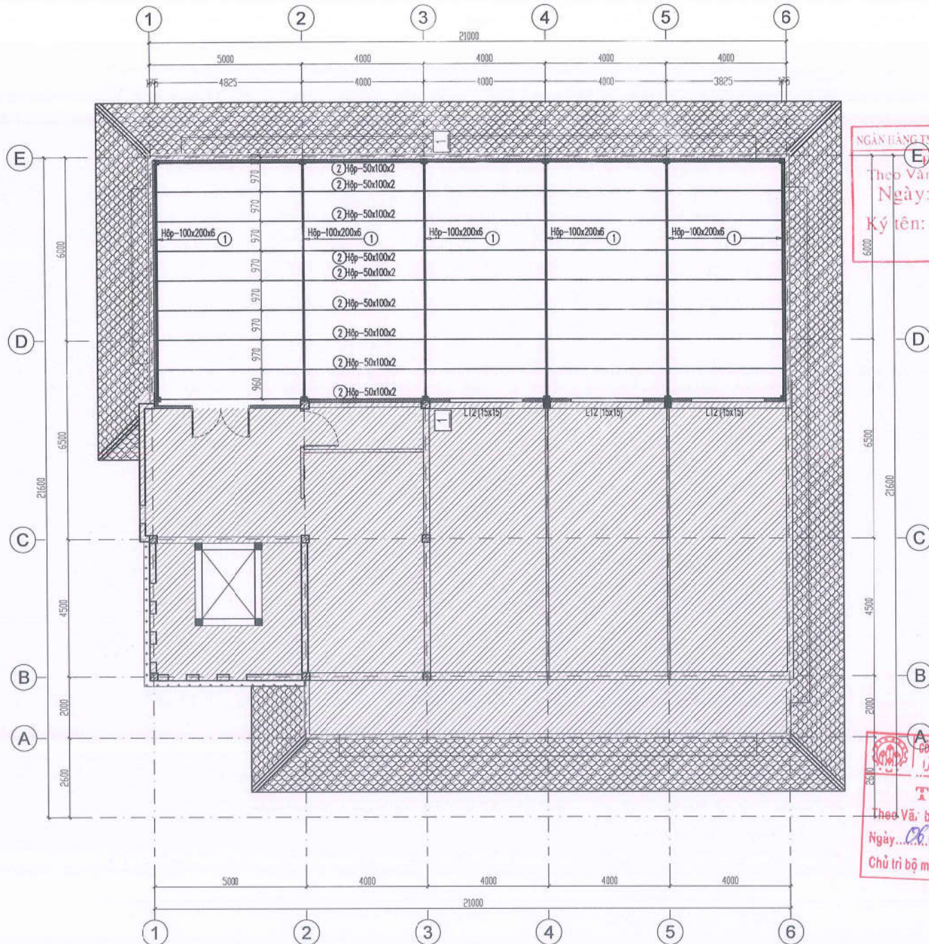
MẶT BẰNG KHUNG KÈO MÁI
