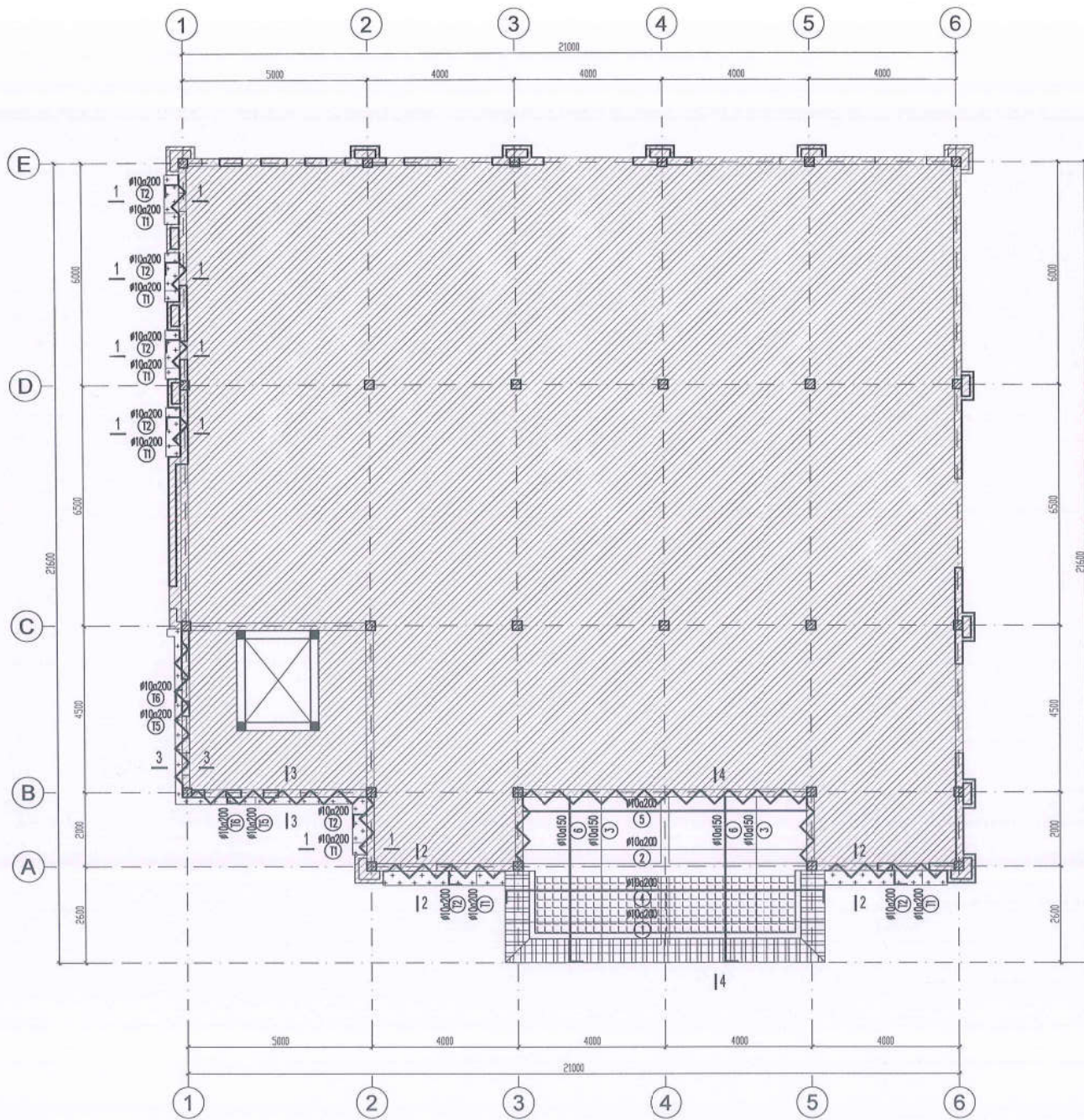
MẶT BẰNG THÉP SÀN TẦNG 2
