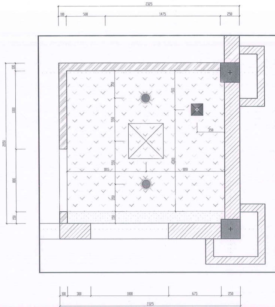
MẶT BẰNG TRẦN CẢI TẠO WC PHÒNG GIÁM ĐỐC
