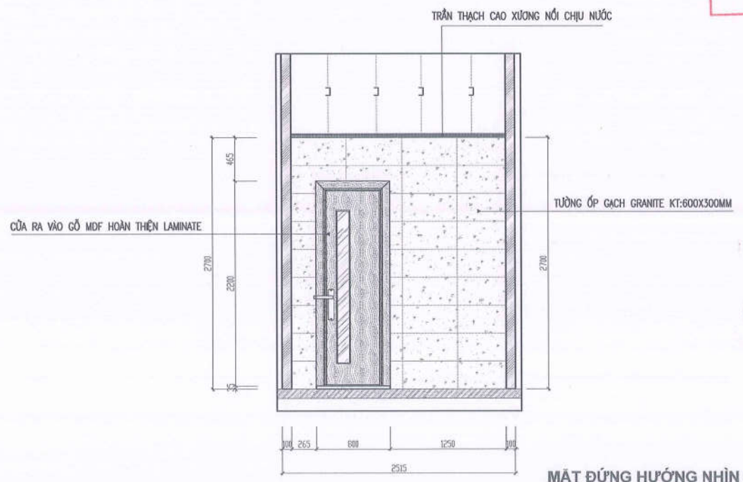
MẶT ĐỨNG HƯỚNG NHÌN D
