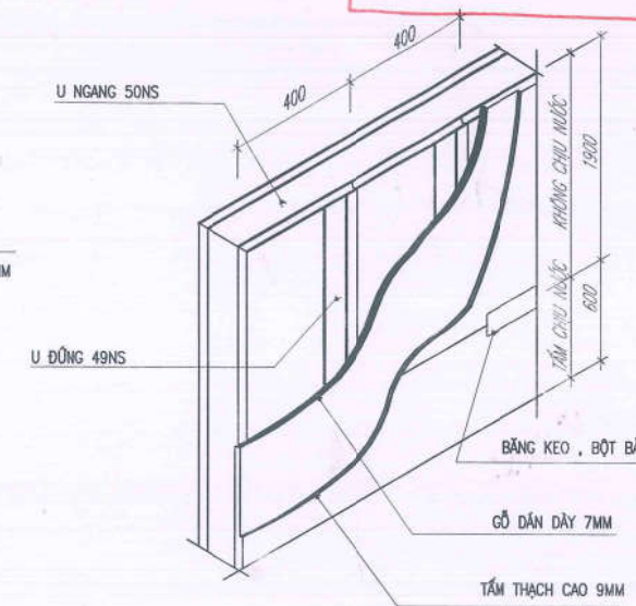
CHI TIẾT VÁCH NGĂN 2 MẶT
