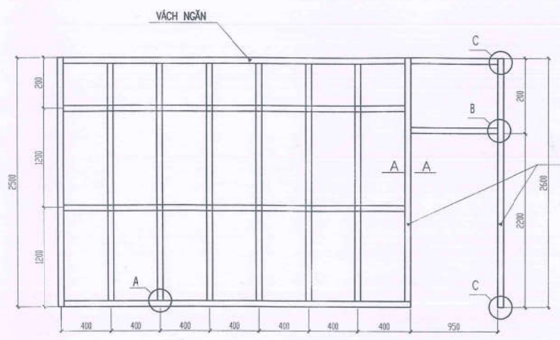
MẶT ĐỨNG KHUNG VÁCH
