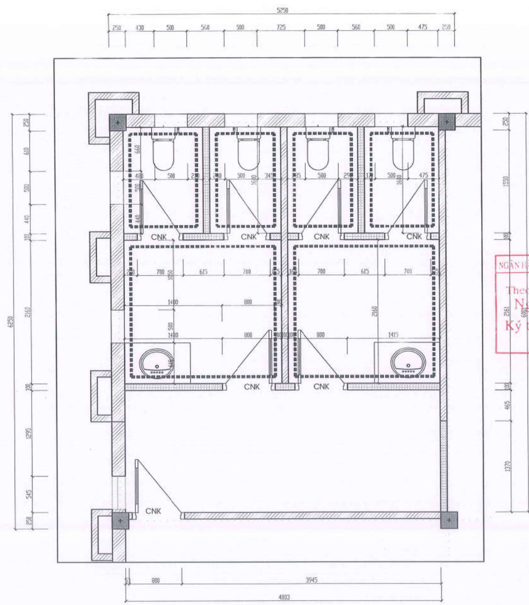
MẶT BẰNG HIỆN TRẠNG WC T1
