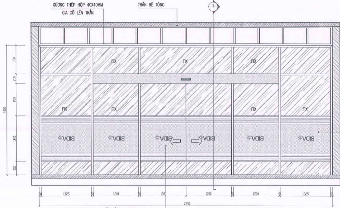
MẶT ĐƯƠNG VÁCH CỬA TỰ ĐỘNG CTĐ1
