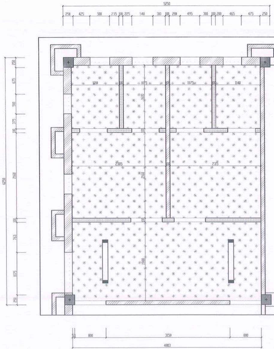
MẶT BẰNG TRẦN HIỆN TRẠNG WC T2+T3
