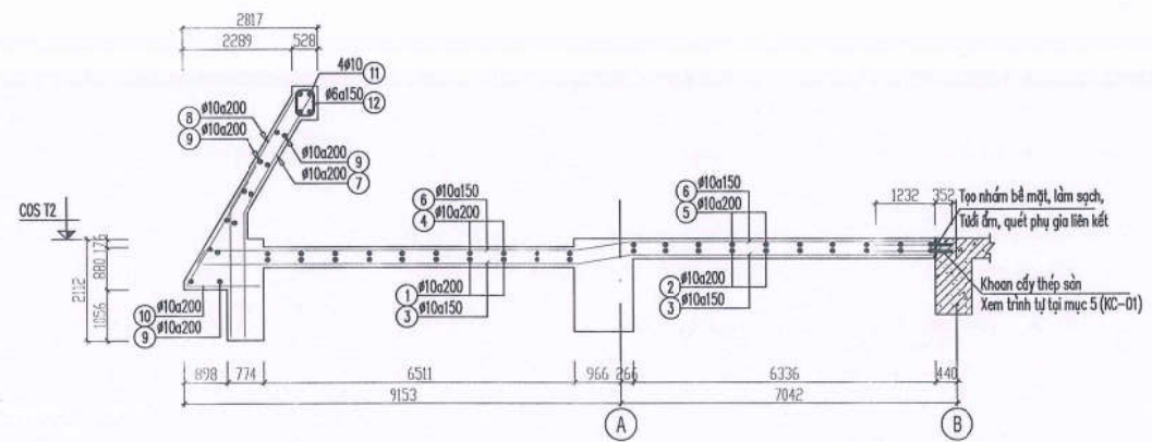
MẶT CẮT 4-4
