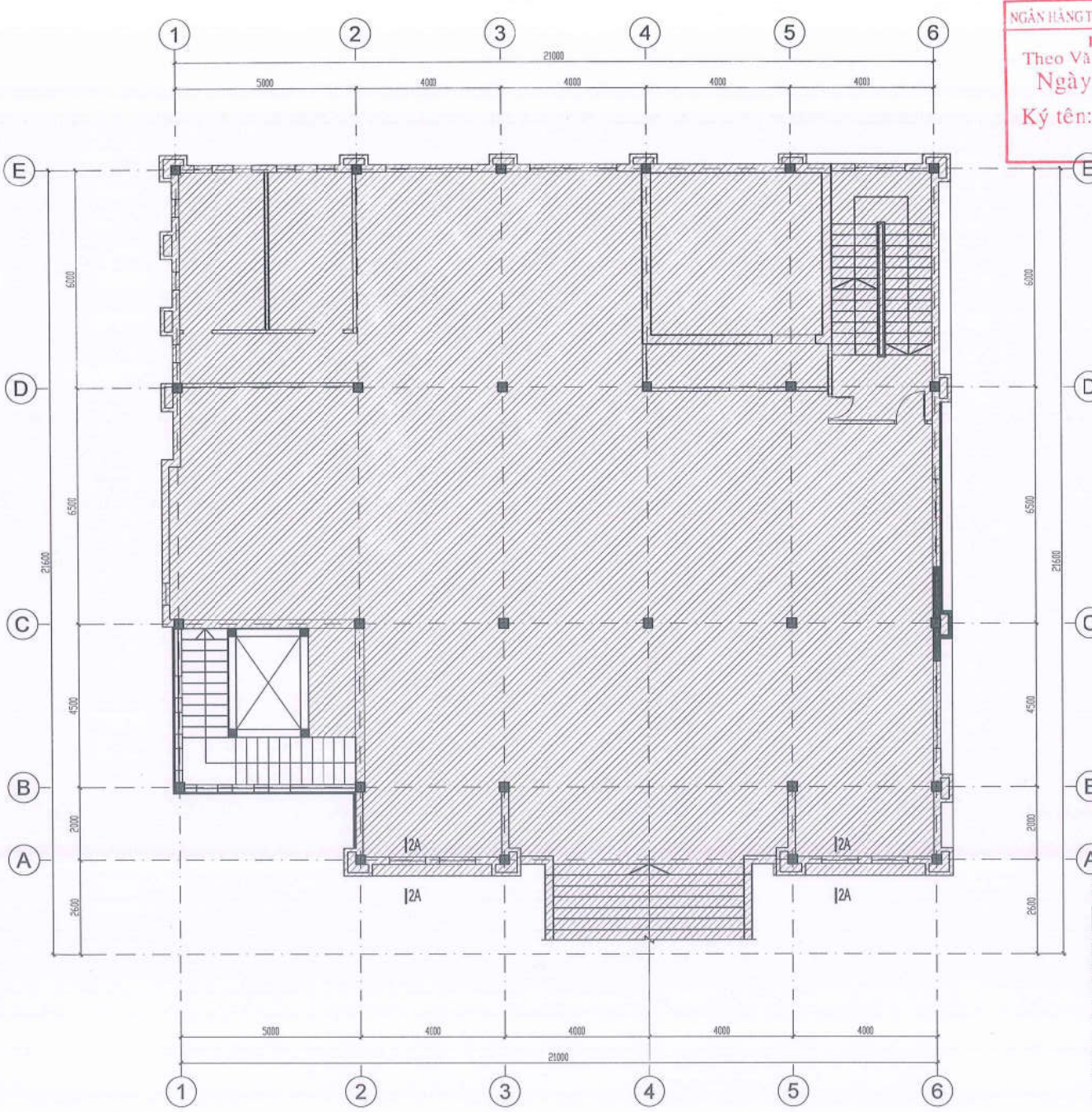
MẶT BẰNG THÉP SÀN TẦNG 1
