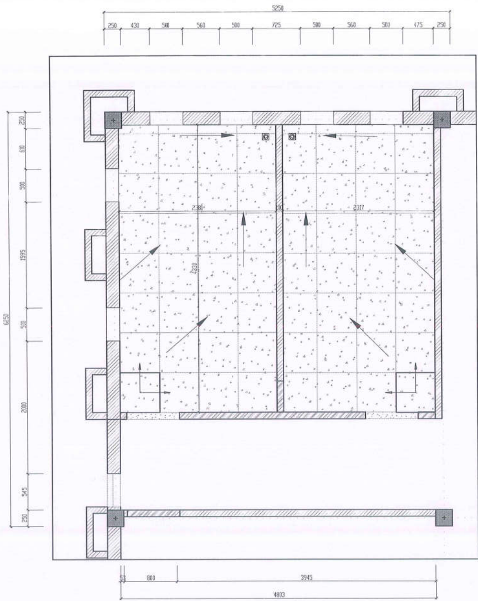
MẶT BẰNG SÀN CẢI TẠO WC T1
