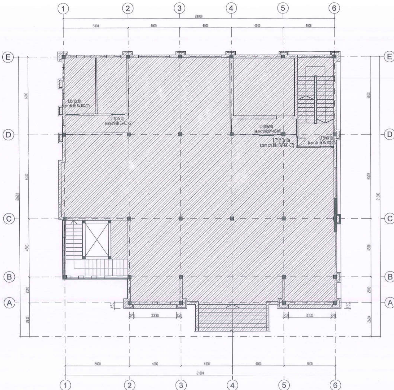
MẶT BẰNG KẾT CẤU TẦNG 1
