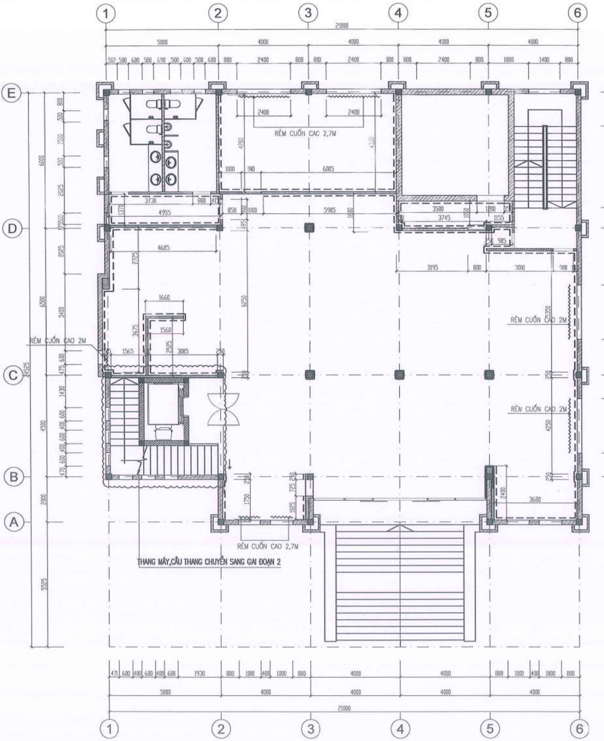
MB PHẠO CỔ TRẦN + RÈM TẦNG 1
