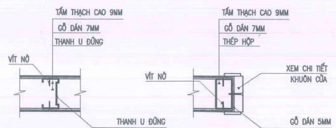
CHI TIẾT VÁCH
