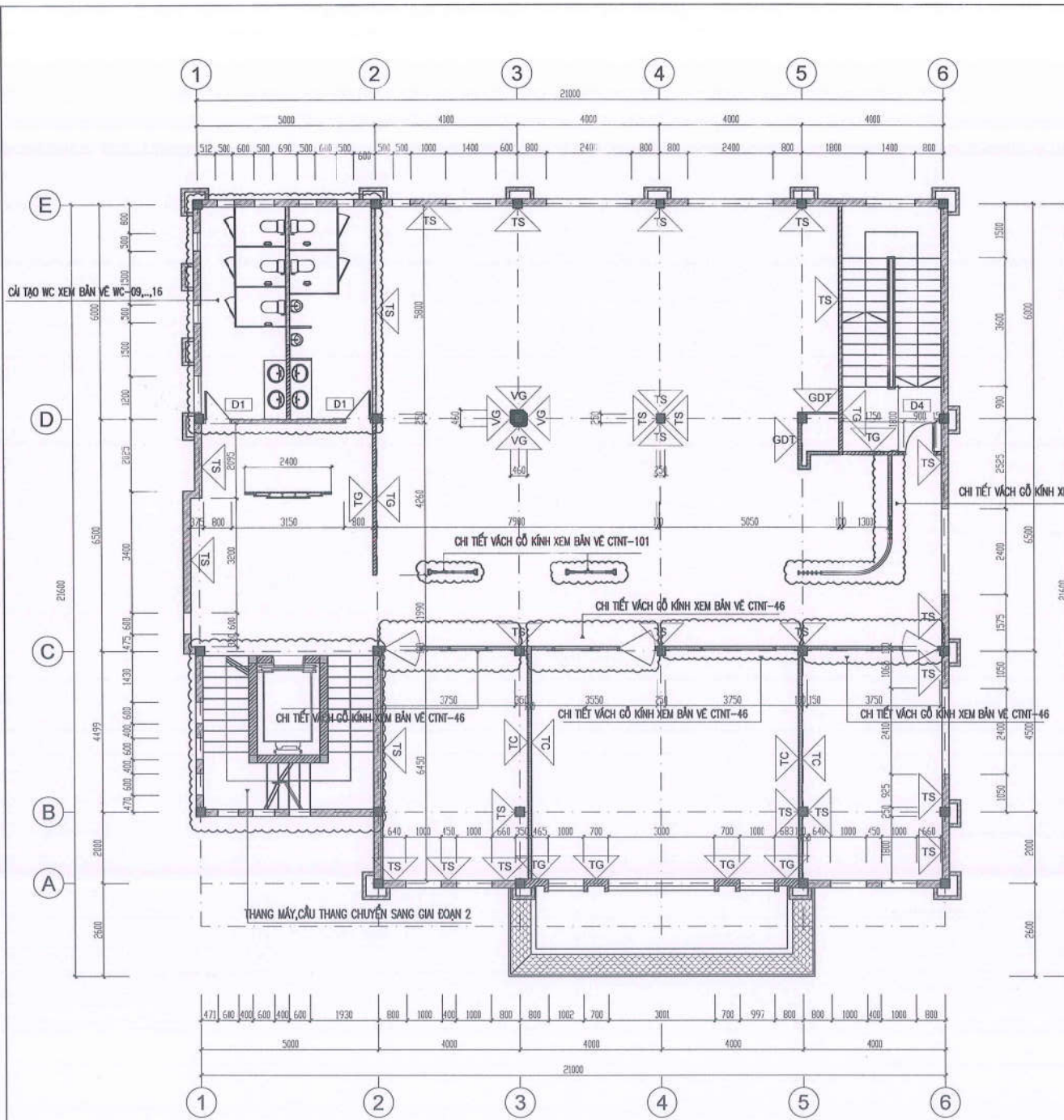
MB CẢI TẠO VÁCH TẦNG 2
