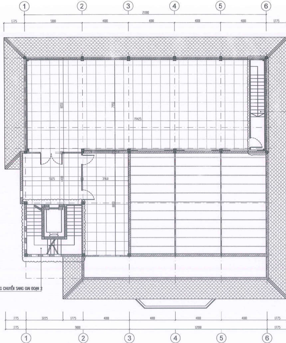
MB SÀN CẢI TẠO TẦNG 4
