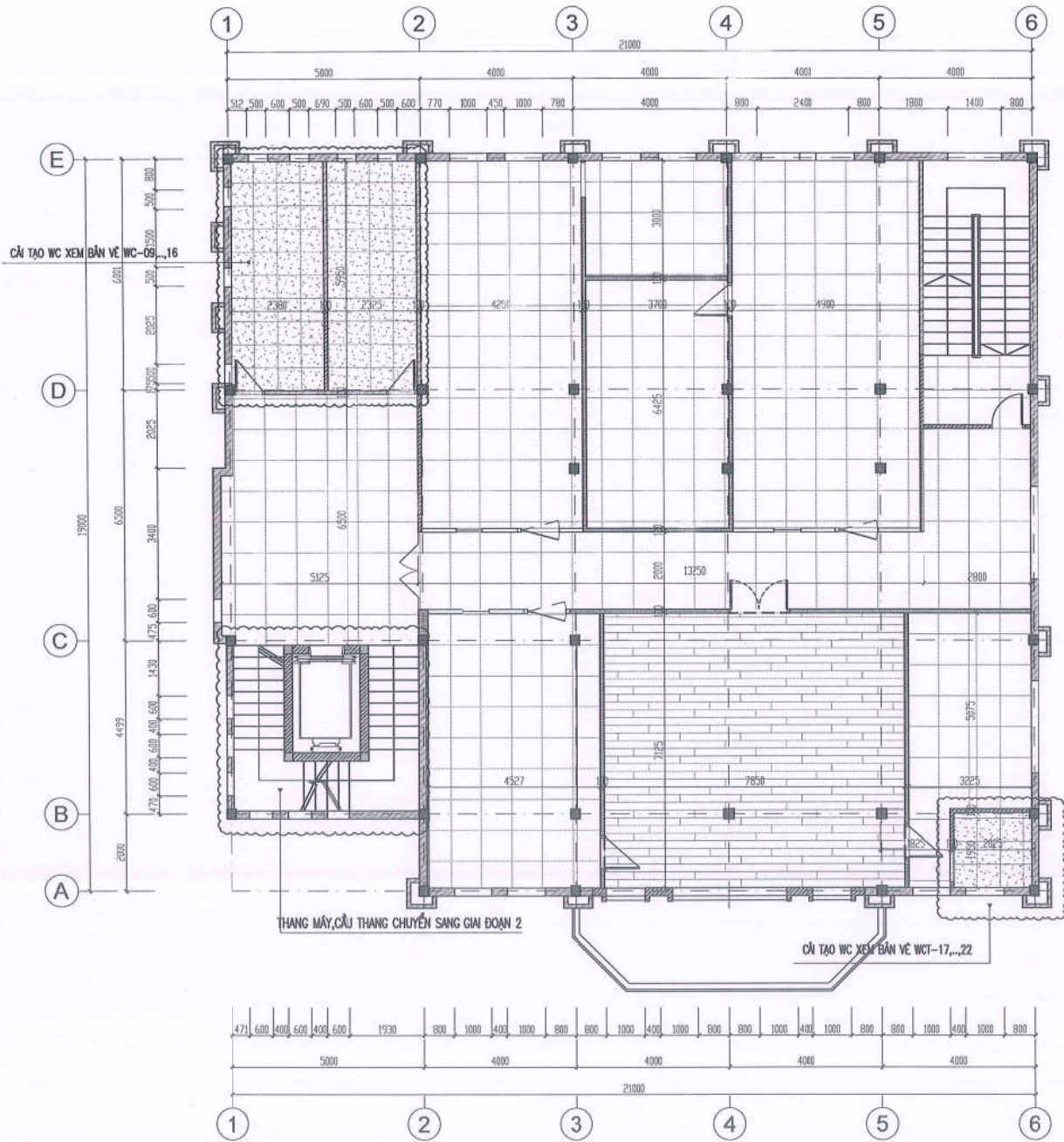
MB SÀN CÁI TẠO TẦNG 3
