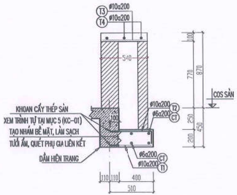
MẶT CẮT 2-2
