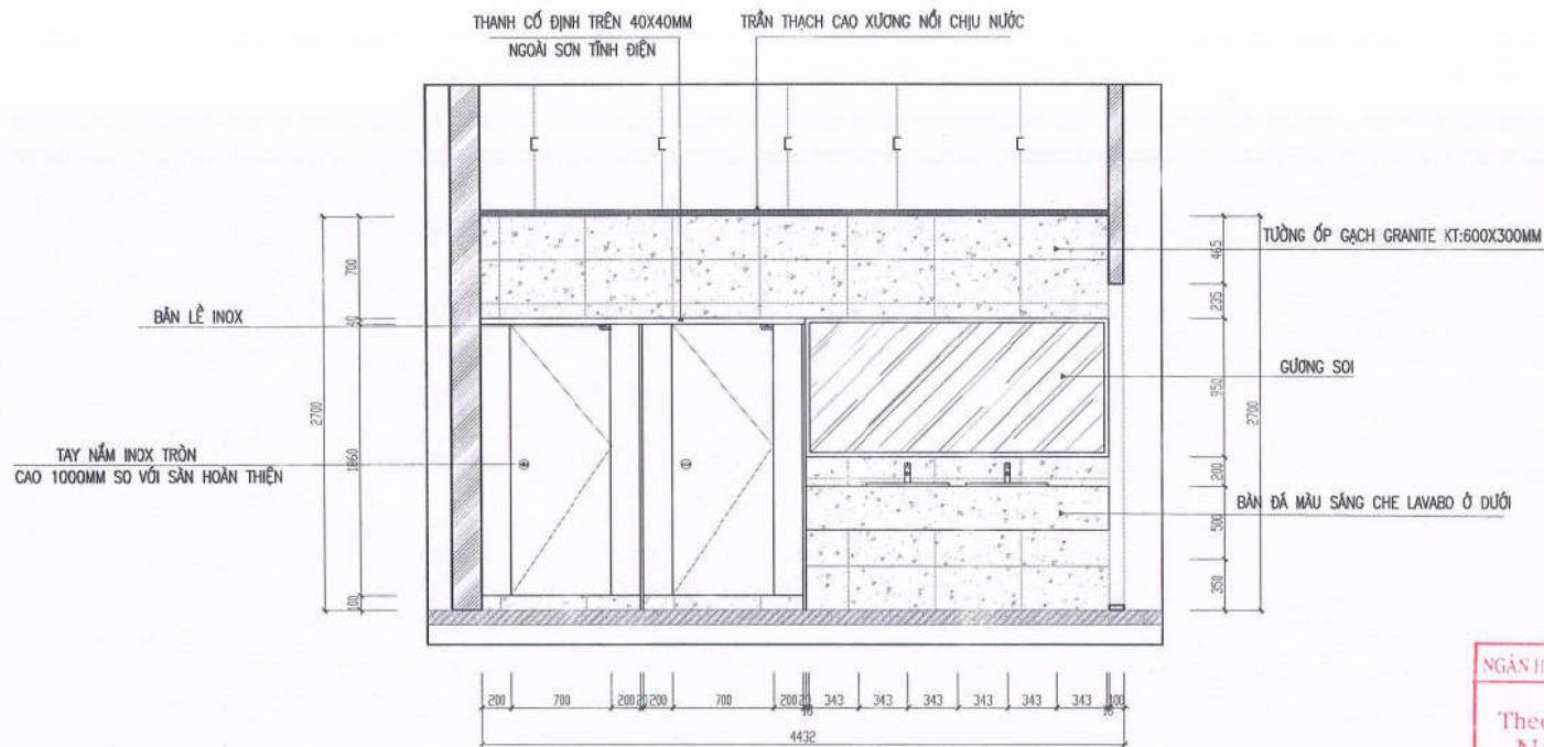
MẶT ĐỨNG HƯỚNG NHÌN B
