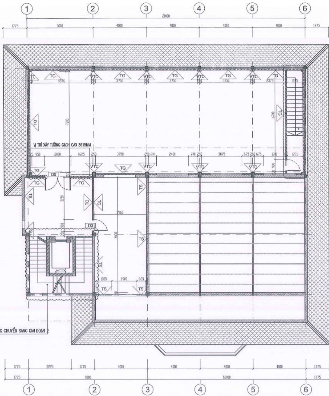
MB CẢI TẠO VÁCH TẦNG 4
