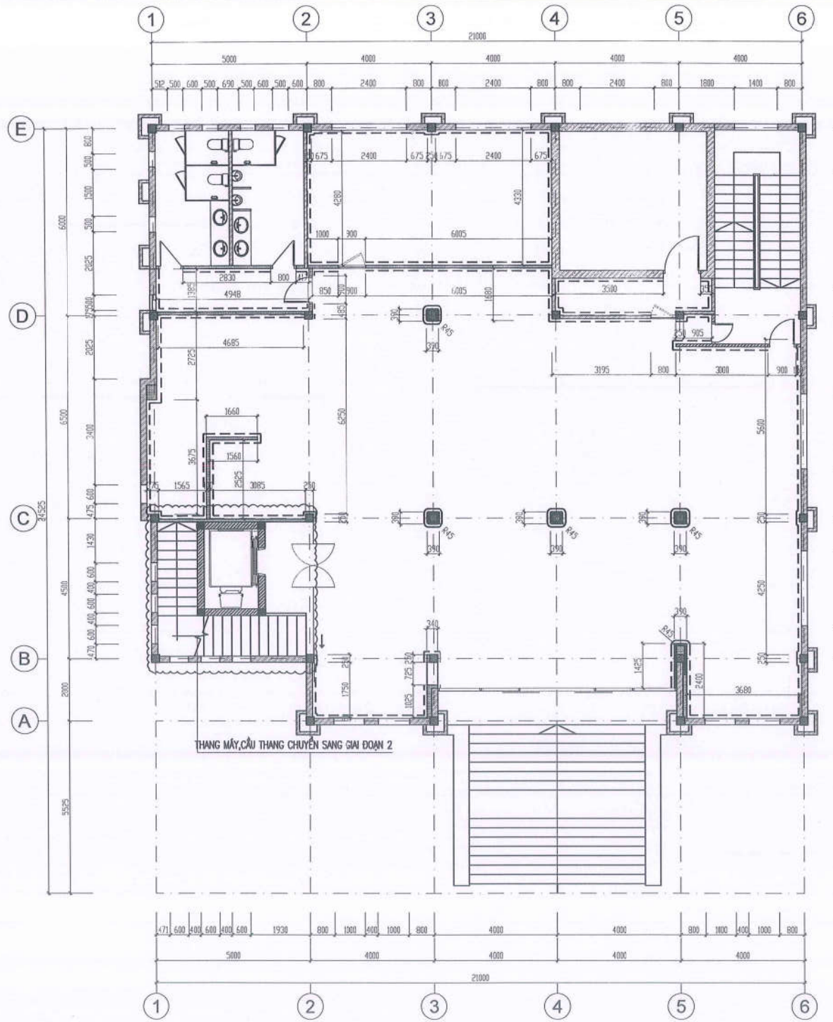
MB PHẠO CHÂN TƯỜNG TẦNG 1
