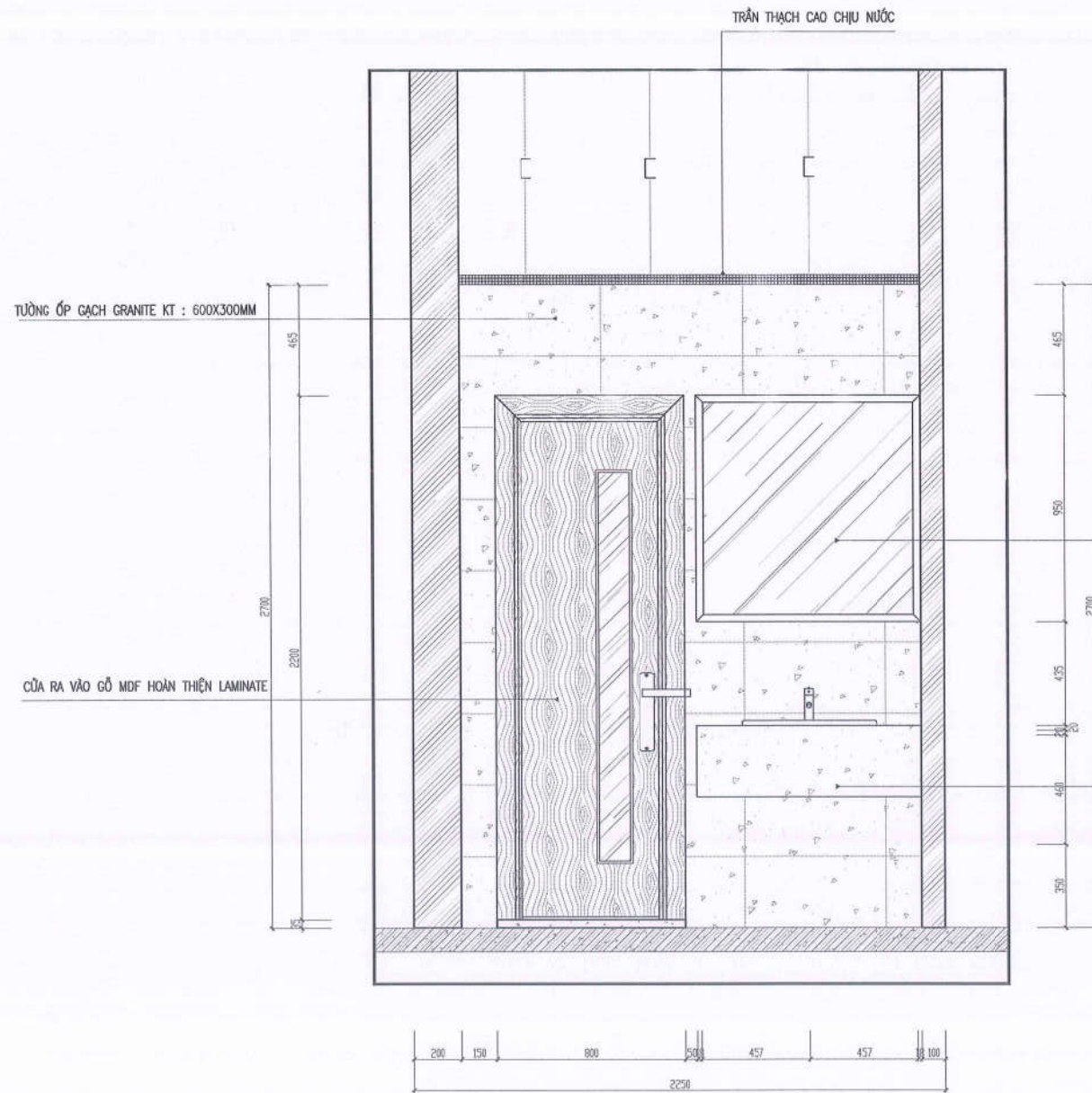
MẶT ĐỪNG HƯỚNG NHÌN D
