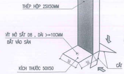
CHI TIẾT LIÊN KẾT C
