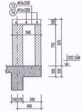
MẶT CẮT 2A-2A
