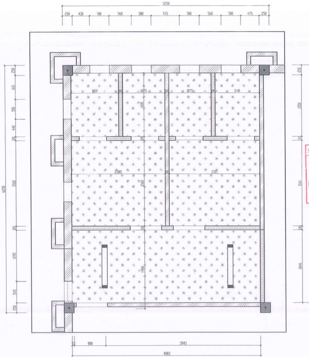
MẶT BẰNG TRẦN HIỆN TRẠNG WC T1
