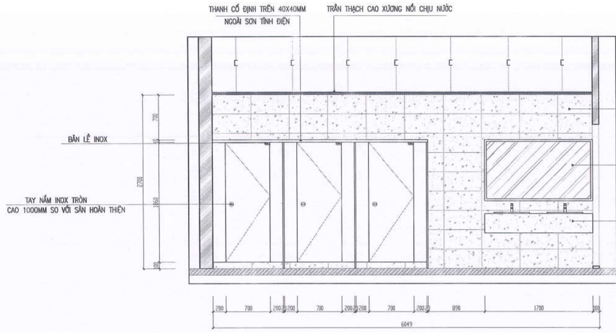
MẶT ĐỨNG HƯỚNG NHÌN B
