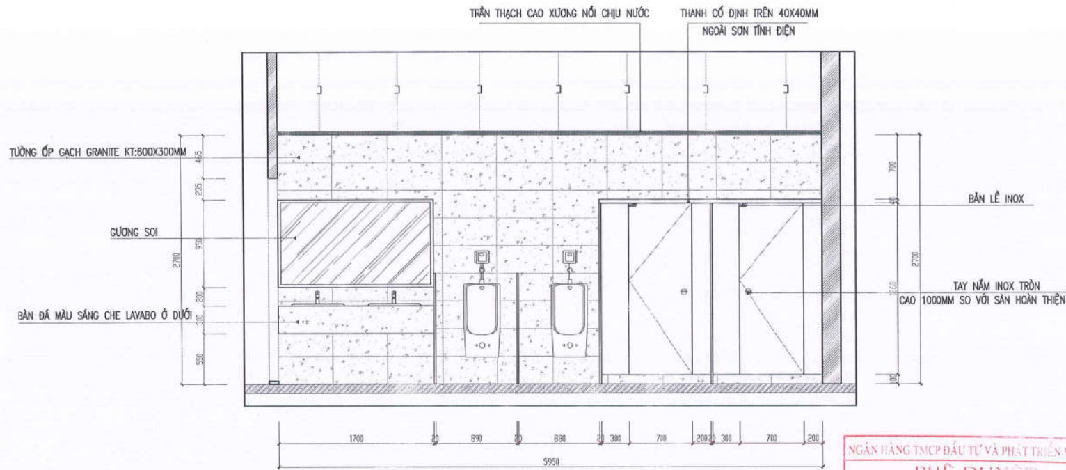
MẶT ĐỨNG HƯỚNG NHÌN D
