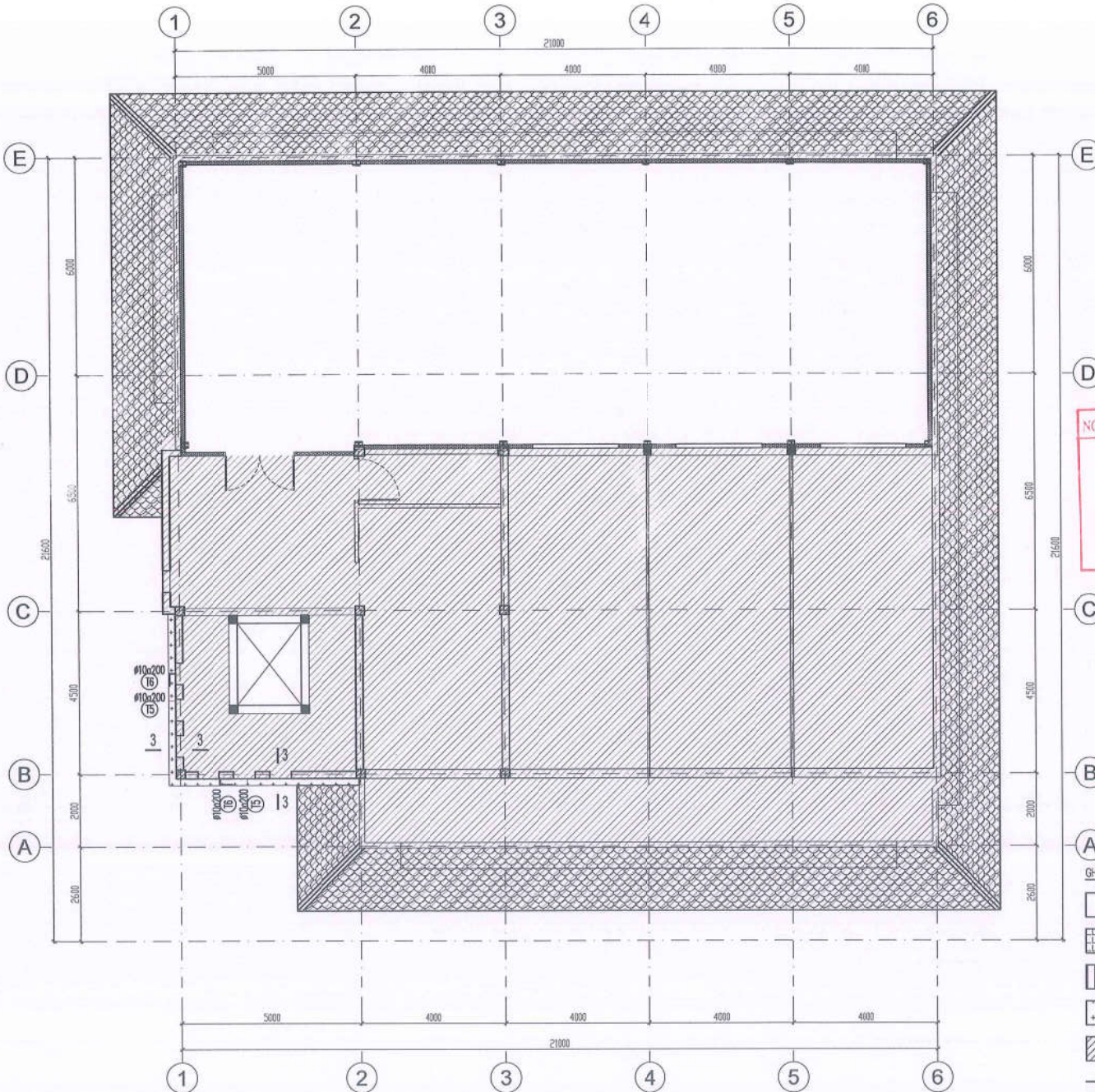
MẶT BẰNG THÉP SÀN TẦNG 4
