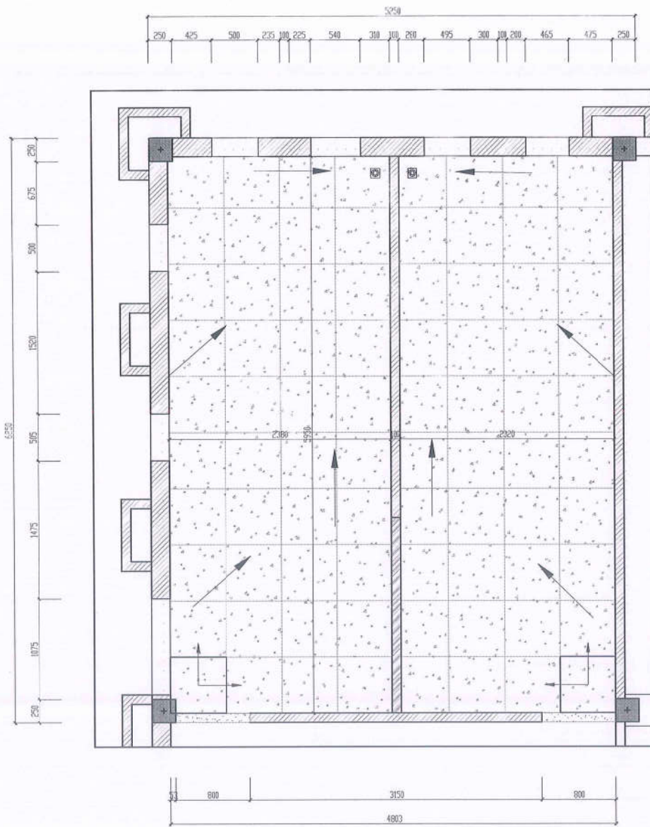
MẶT BẰNG CẢI TẠO WC T2+T3
