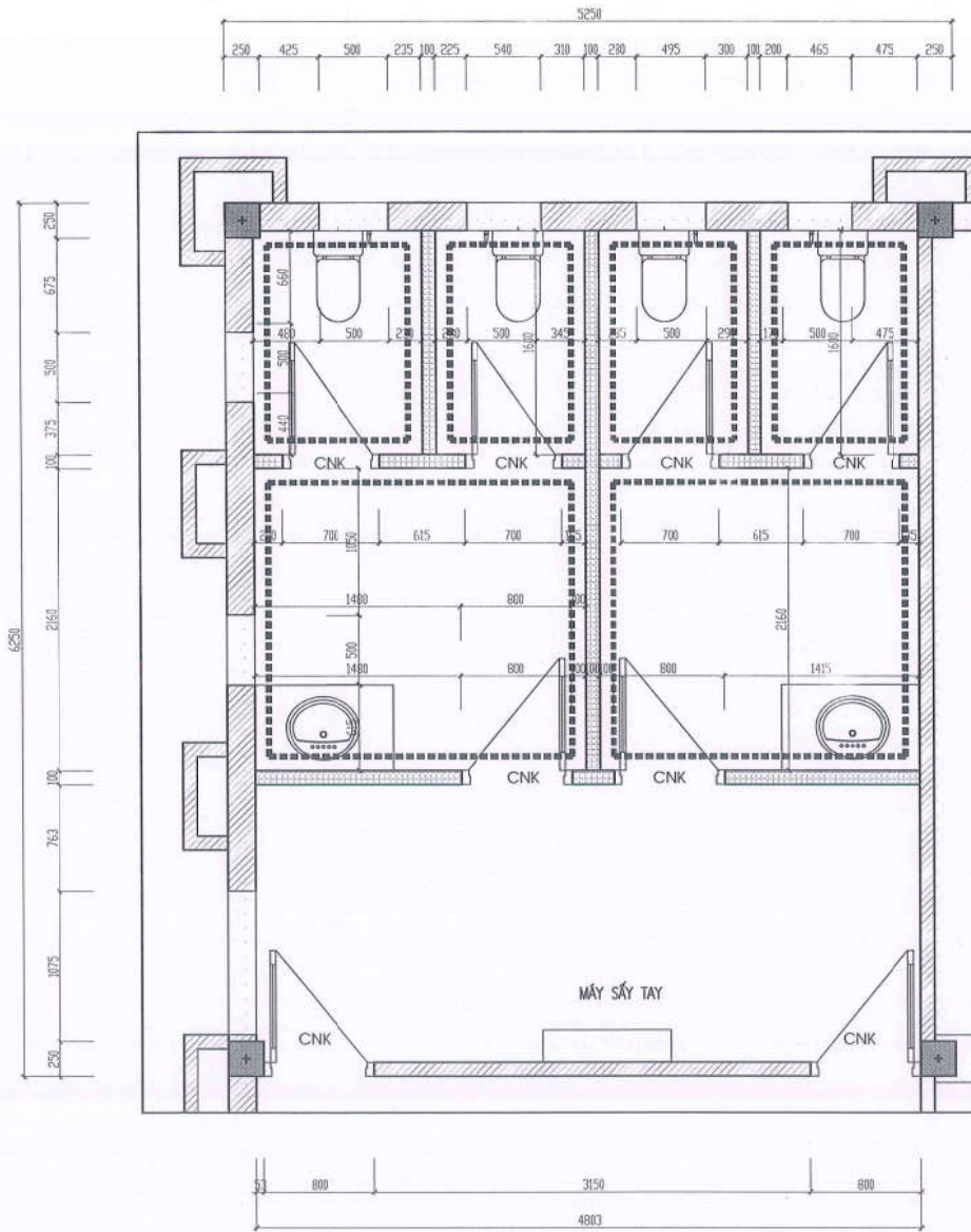
MẶT BẰNG HIỆN TRẠNG WC T2+T3
