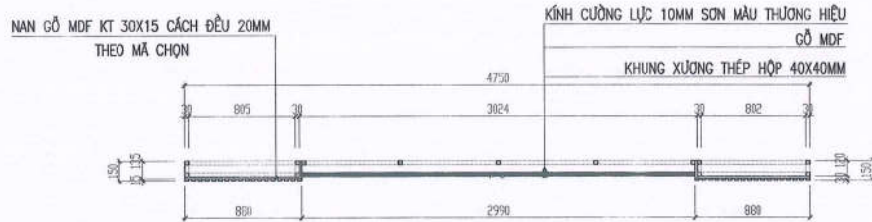
MẶT CẮT 1-1
