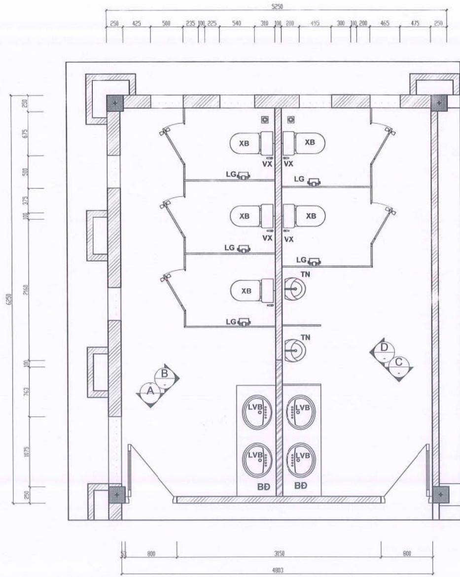
MẶT BẰNG CẢI TẠO NỘI THẤT WC T2+T3
