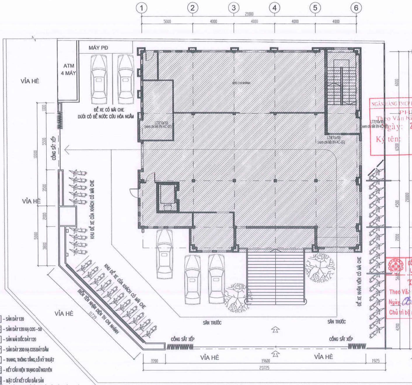
MẶT BẰNG KẾT CẤU TẦNG TRỆT
