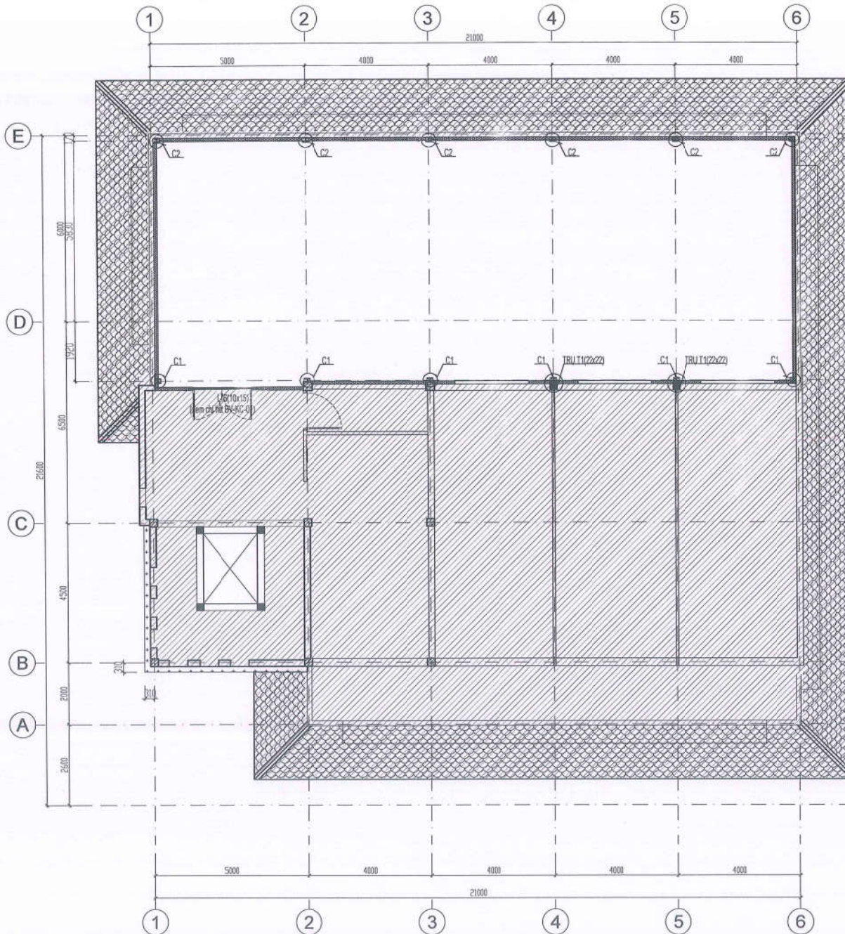
MẶT BẰNG KẾT CẤU TẦNG 4
