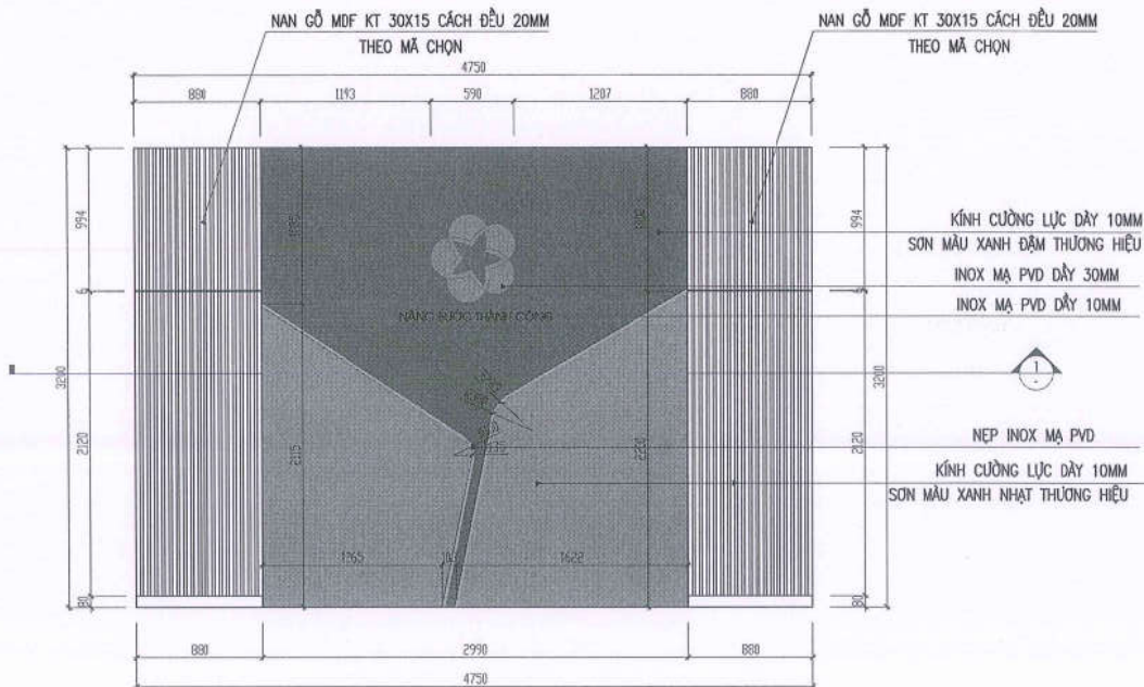
MẶT ĐỨNG VÁCH PREMIER
