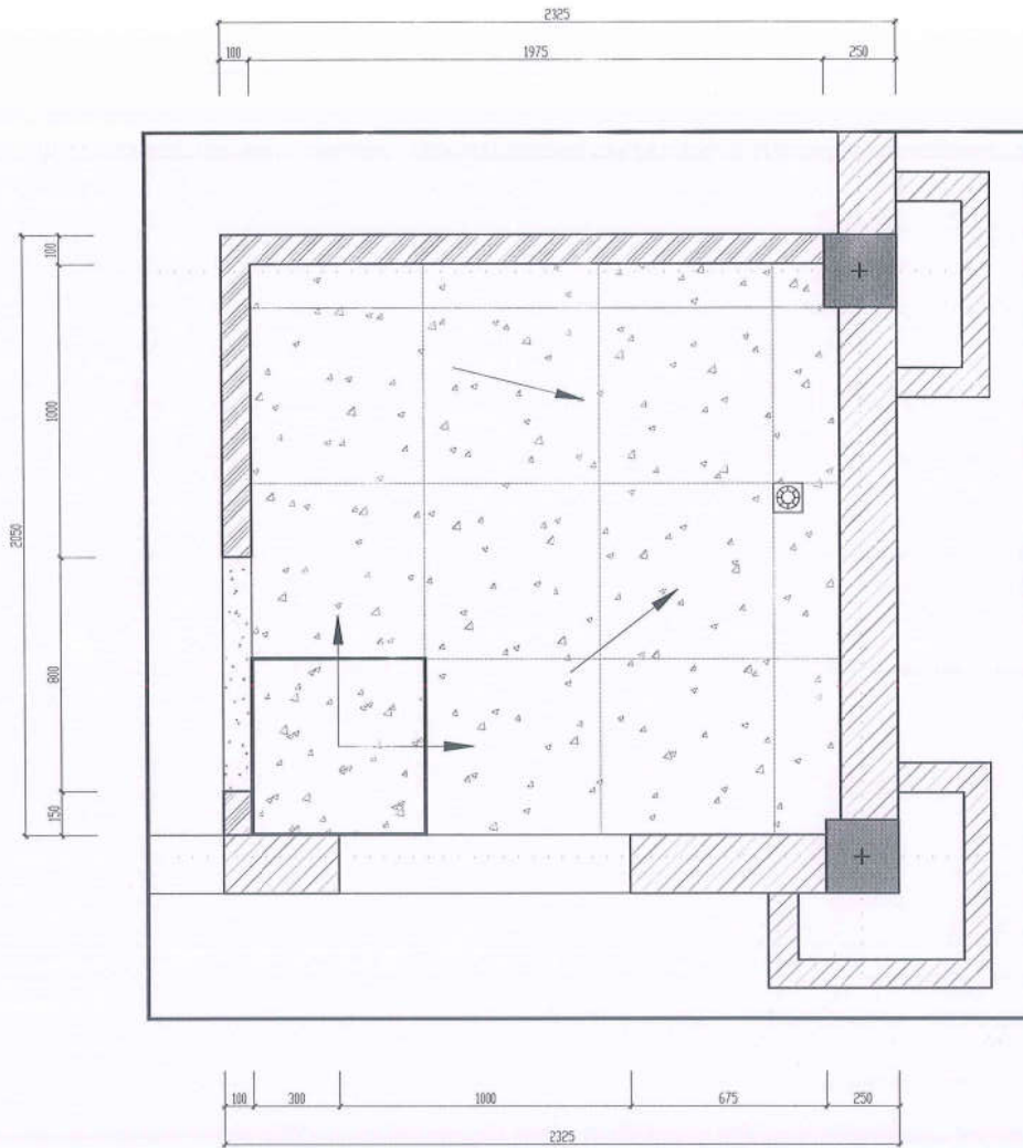
MẶT BẰNG SÀN CẢI TẠO WC PHÒNG GIÁM ĐỐC
