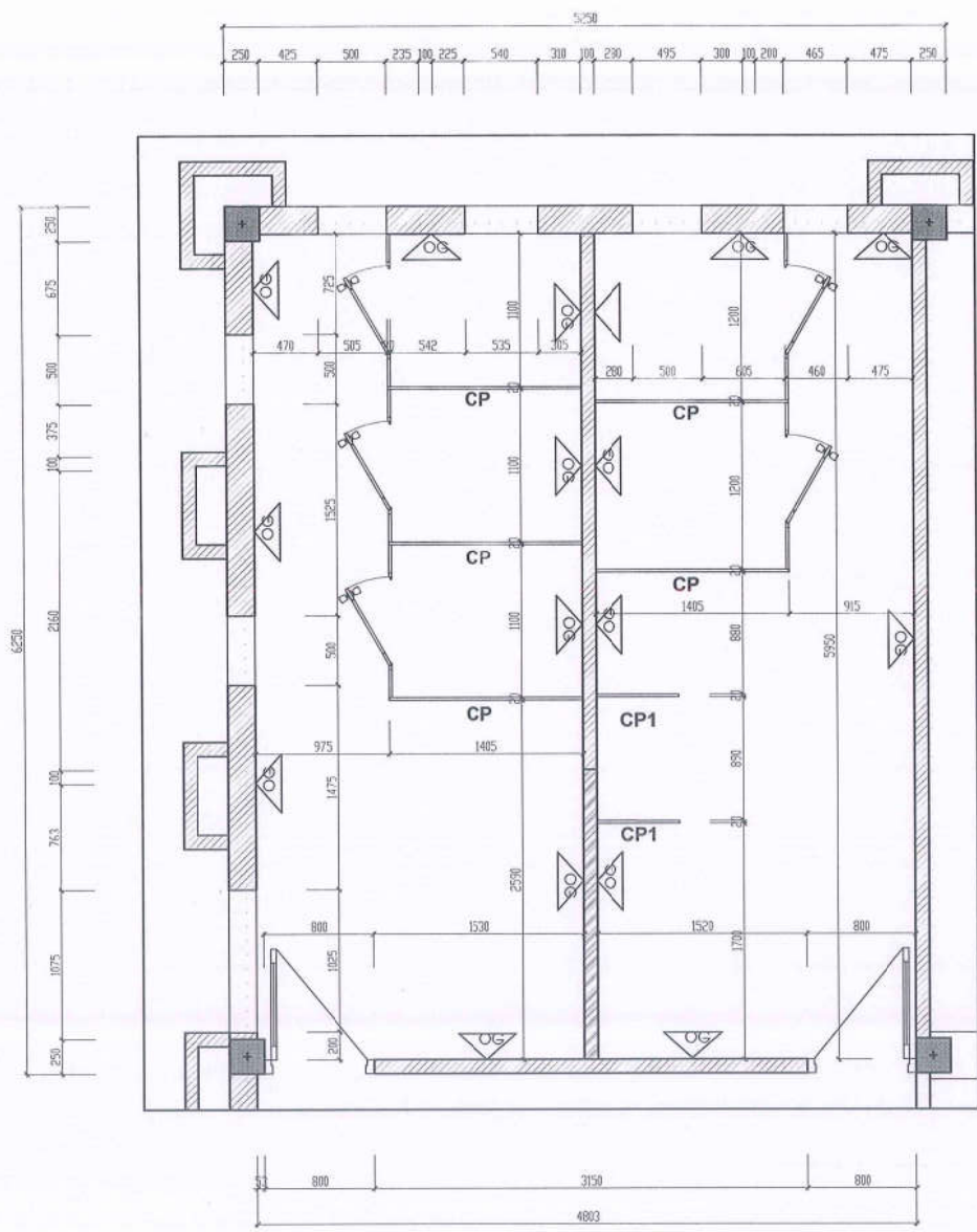
MẶT BẰNG CẢI TẠO VÁCH WC T2+T3
