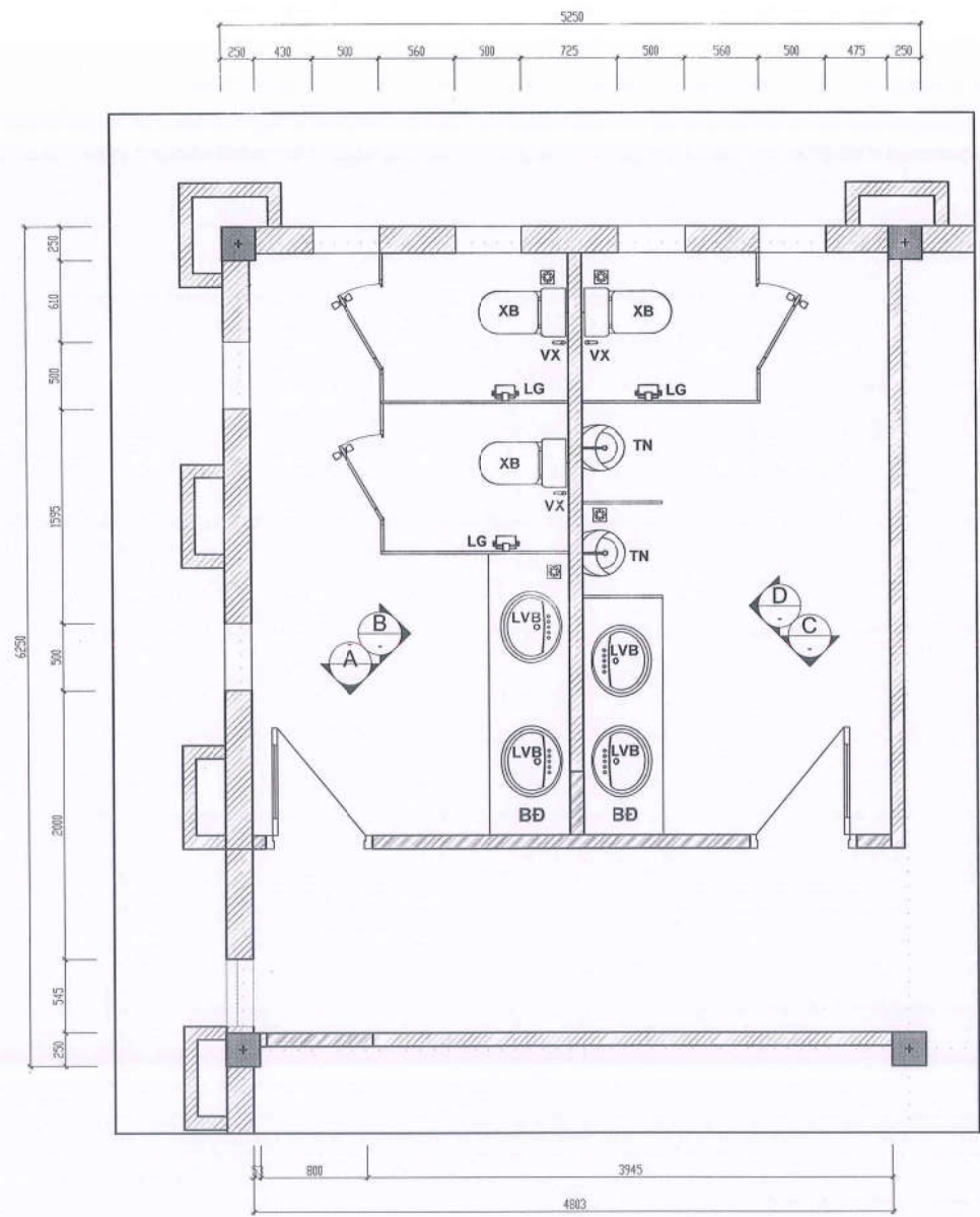
MẶT BẰNG CẢI TẠO NỘI THẤT WC T1
