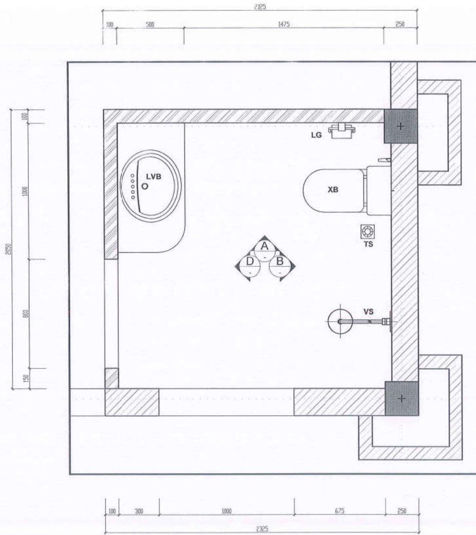
MẶT BẰNG CẢI TẠO NỘI THẤT WC PHÒNG GIÁM ĐỐC
