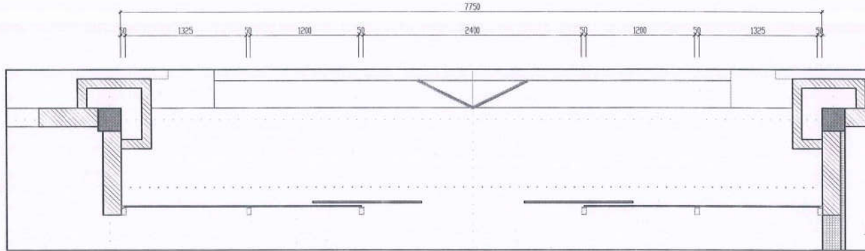
MẶT BẰNG VÁCH CỬA TỰ ĐỘNG CTĐ1
