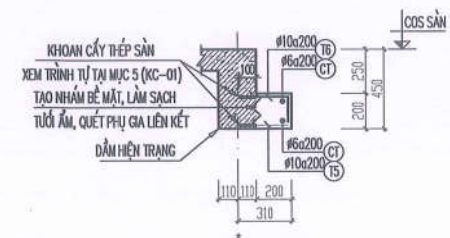
MẶT CẮT 3-3
