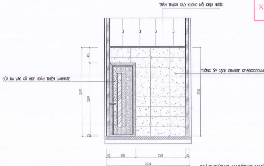
MẶT ĐỨNG HƯỚNG NHÌN C
