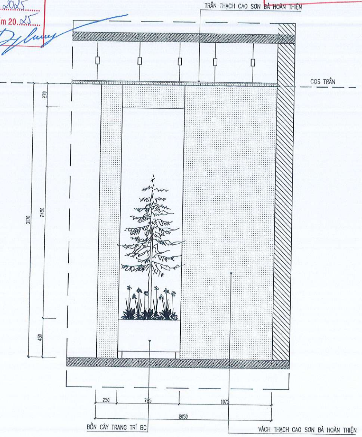
MẶT ĐỨNG VÁCH TẦNG 1
