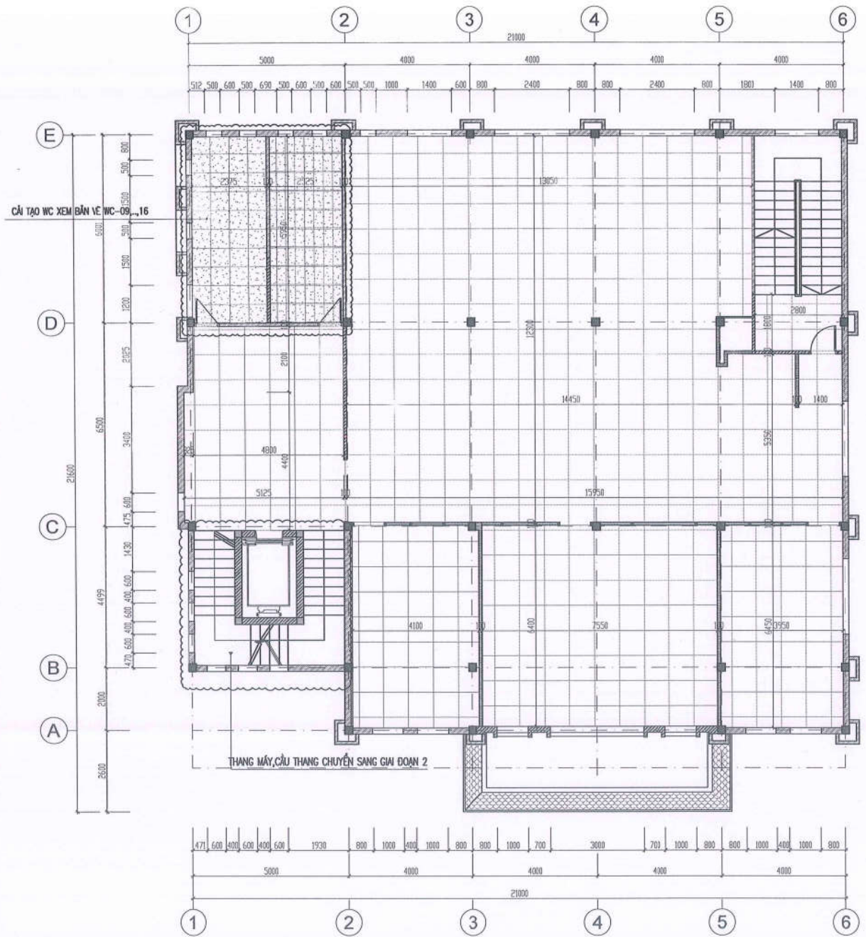
MB SÀN CẢI TẠO TẦNG 2
