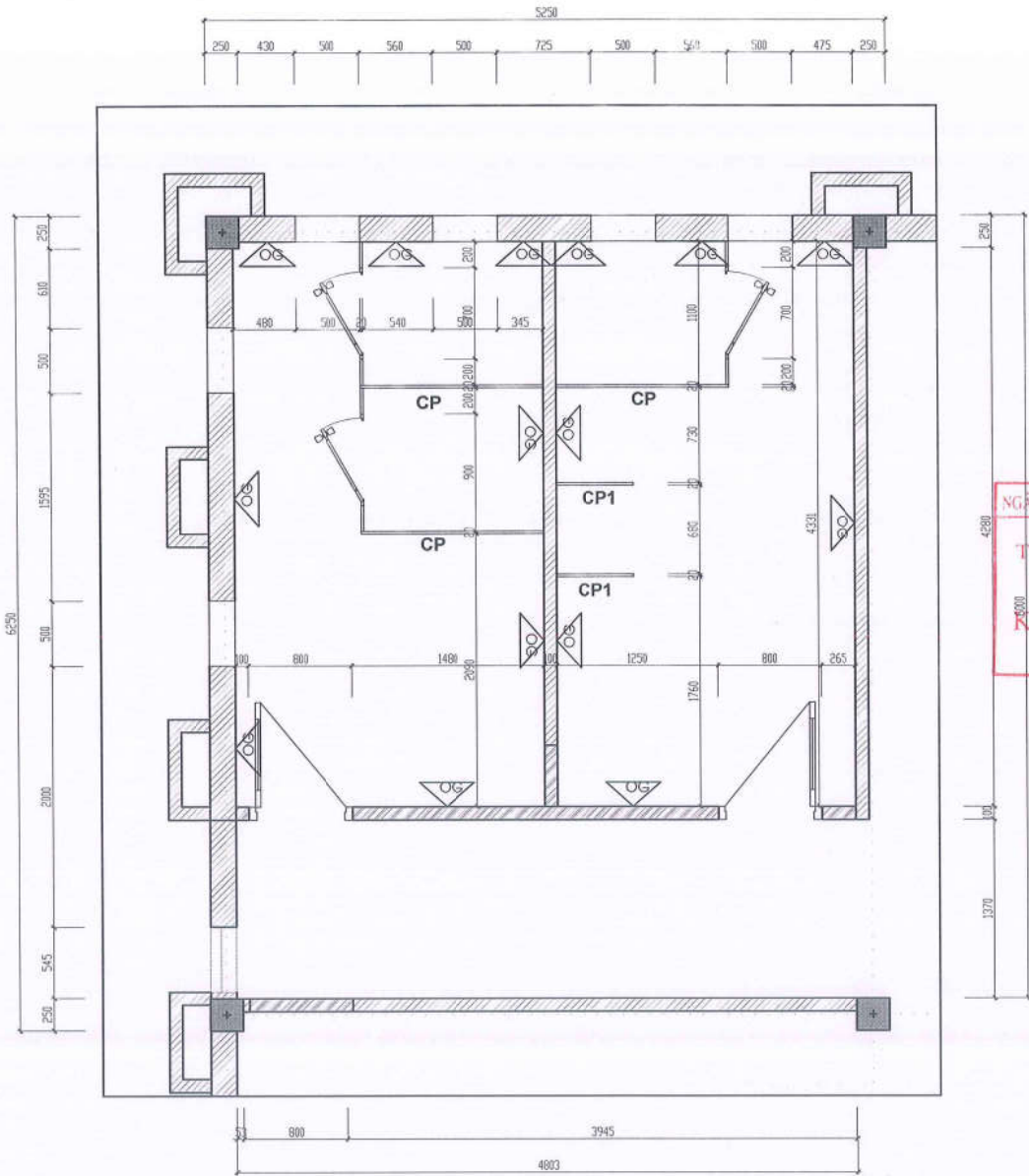
MẶT BẰNG CẢI TẠO VÁCH WC T1
