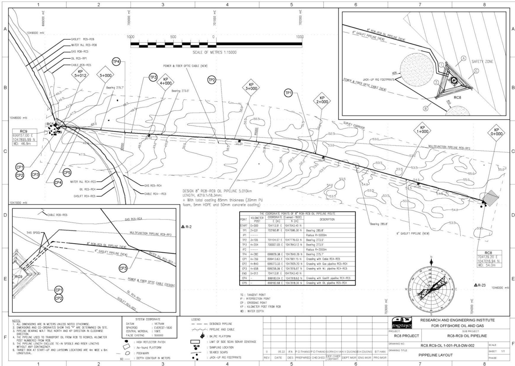
Hình 3-1: Sơ đồ tuyến ống dầu RC8-RC9
