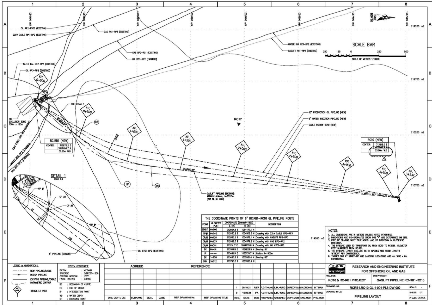
Hình 3-4: Sơ đồ tuyến ống gaslift RC.RC1-RC10
