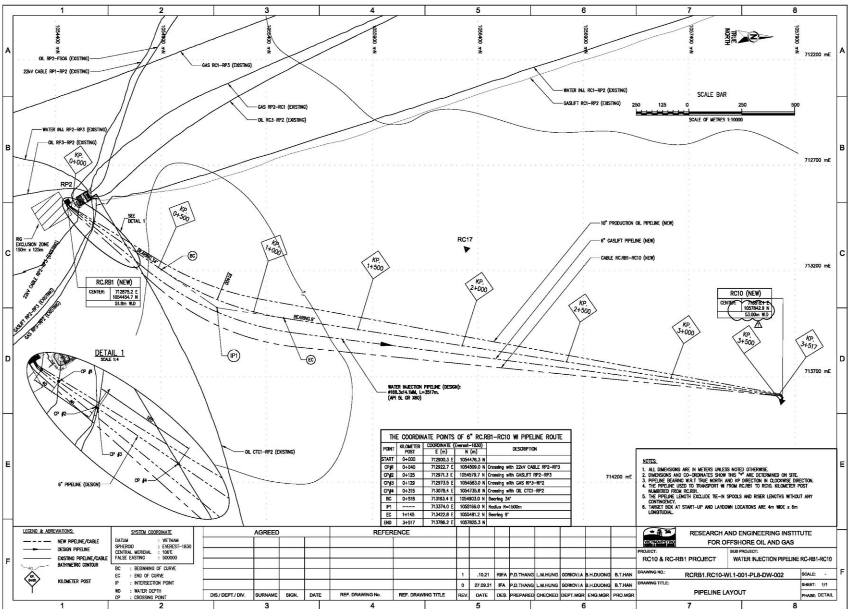
Hình 3-3: Sơ đồ tuyến ống nước ép via RC.RC1-RC10
