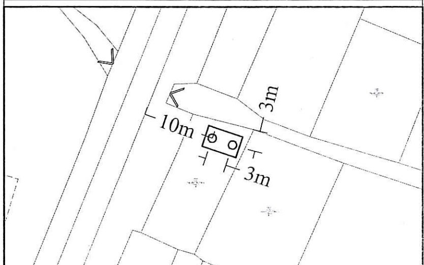
TRÍCH LỤC VỊ TRÍ ĐẶT TRẠM BIẾN ÁP TBA Vĩnh Sơn 7 180kVA-35/0,4kV
