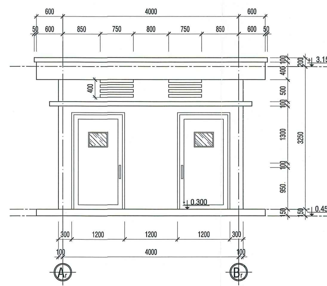
MẶT ĐỨNG TRỰC Br-Ar TL 1/50
