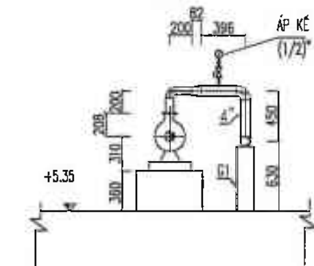
MẶT CẮT 3-3 TỶ LỆ 1/50
