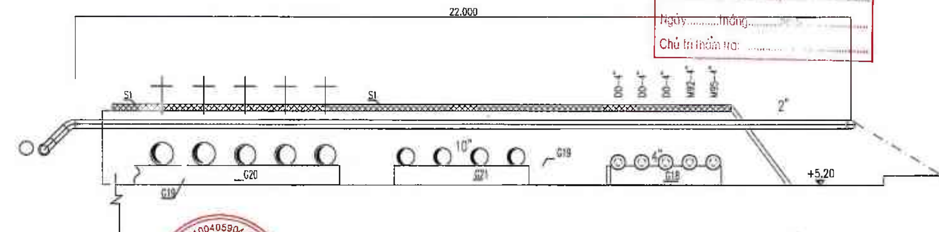
MẶT CẮT 6-6 TỶ LỆ 1/50
