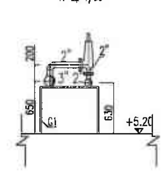
MẶT CẮT 4-4 TỶ LỆ 1/50
