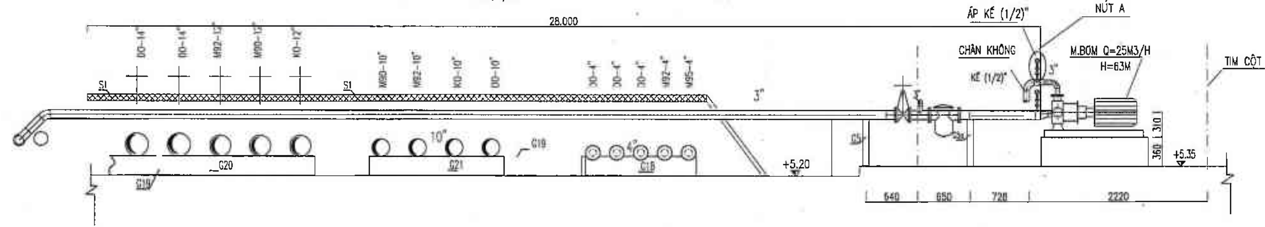
MẶT CẮT 1-1 TỶ LỆ 1/50
