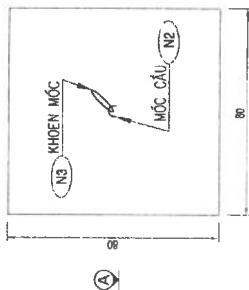
MẶT BẰNG NẮP ĐÀN
