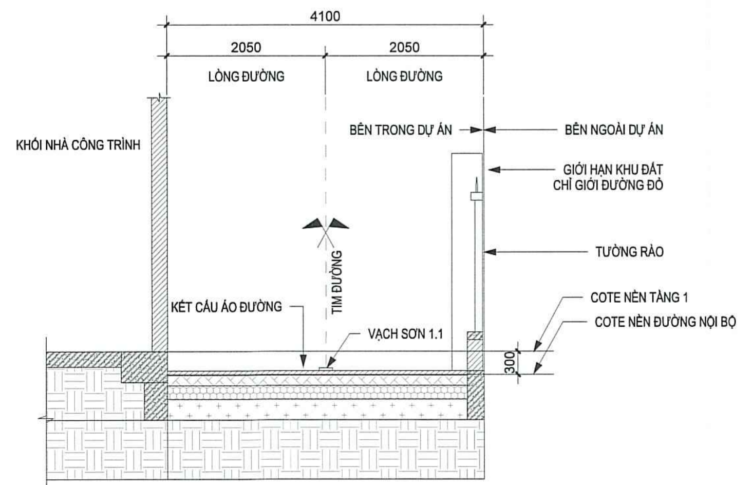
MẶT CẮT 2-2
