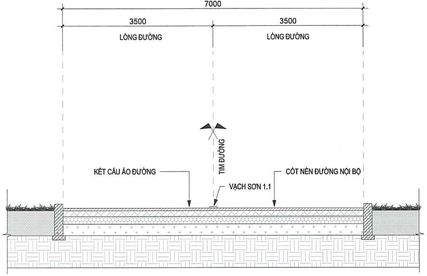
MẶT CẮT 1-1
