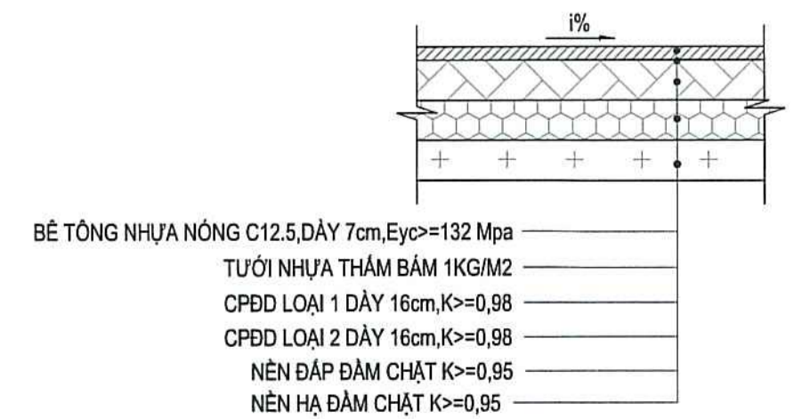
KẾT CẤU ĐƯỜNG BÊ TÔNG NHỰA
