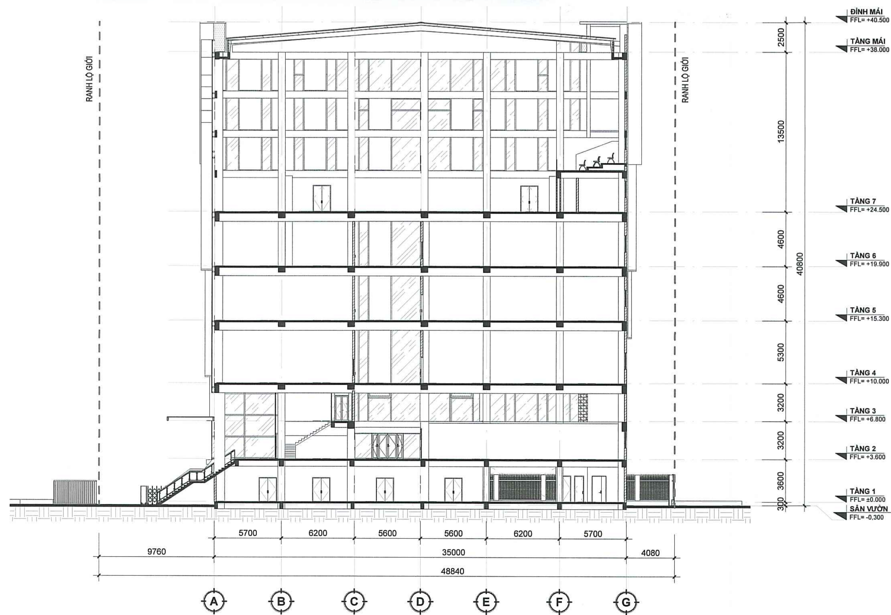
MẶT CẮT TOÀN KHU B-B TL/ 1 : 200
