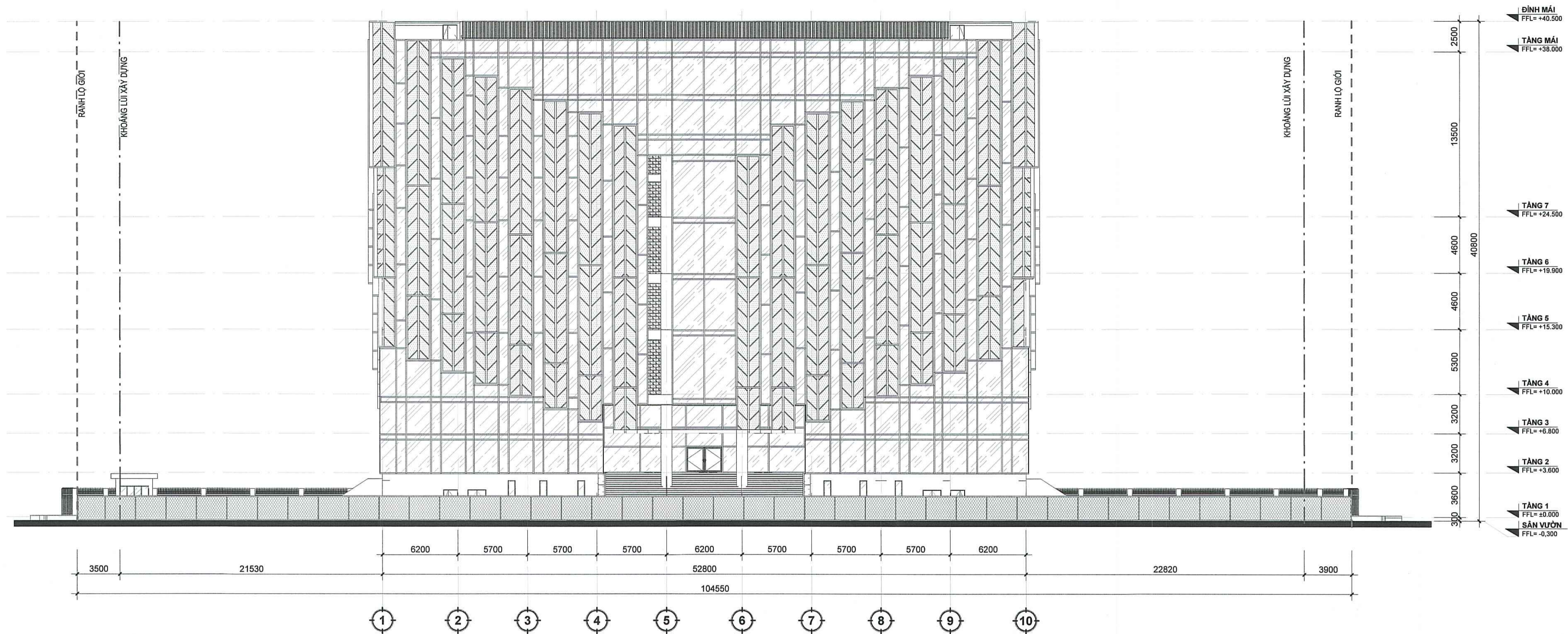
MẶT ĐỨNG TOÀN KHU TRỤC 1-10 TL/ 1 : 200
