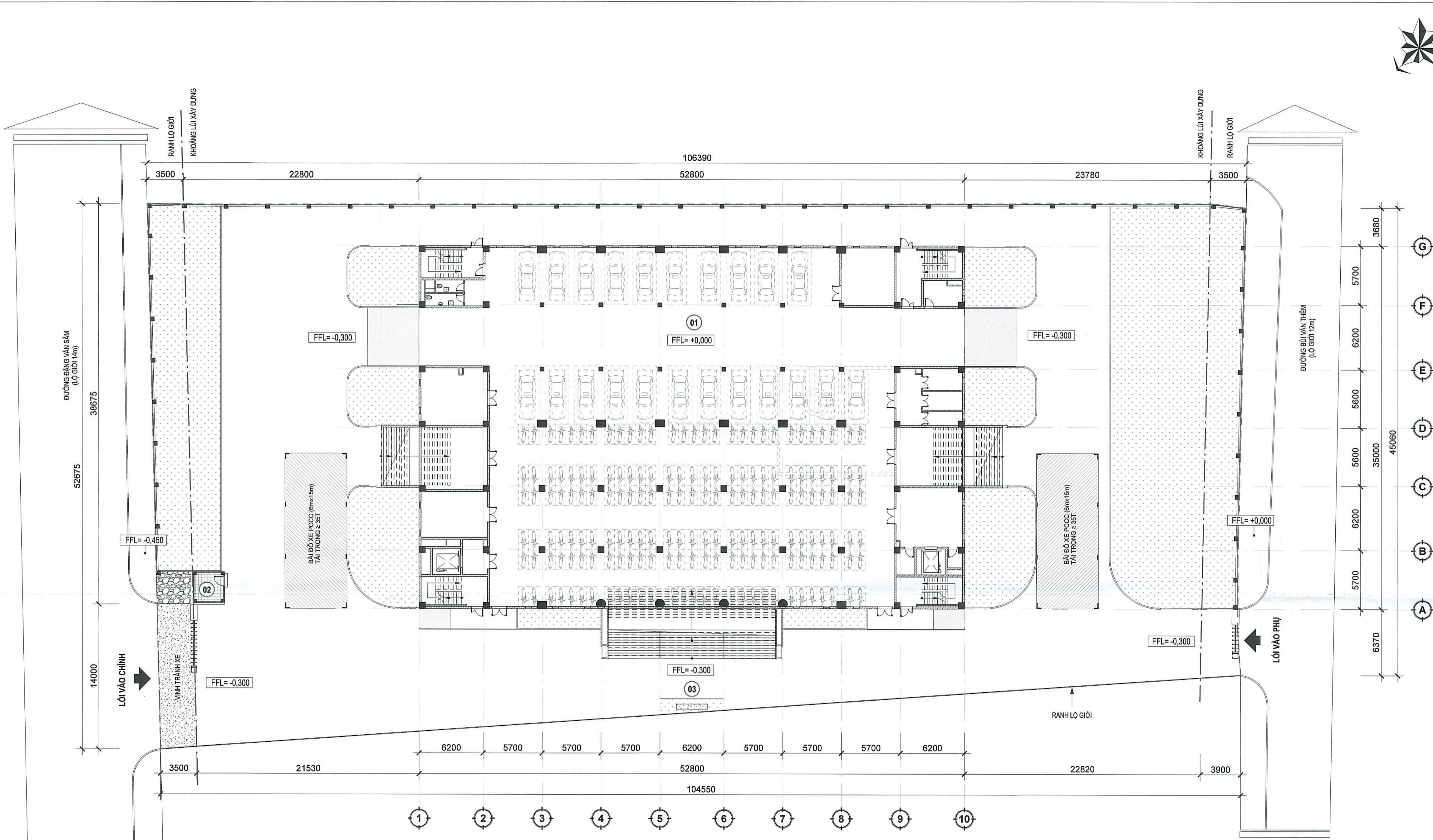
MẶT BẰNG TỔNG THỂ TẦNG 1 TL/ 1 : 200
