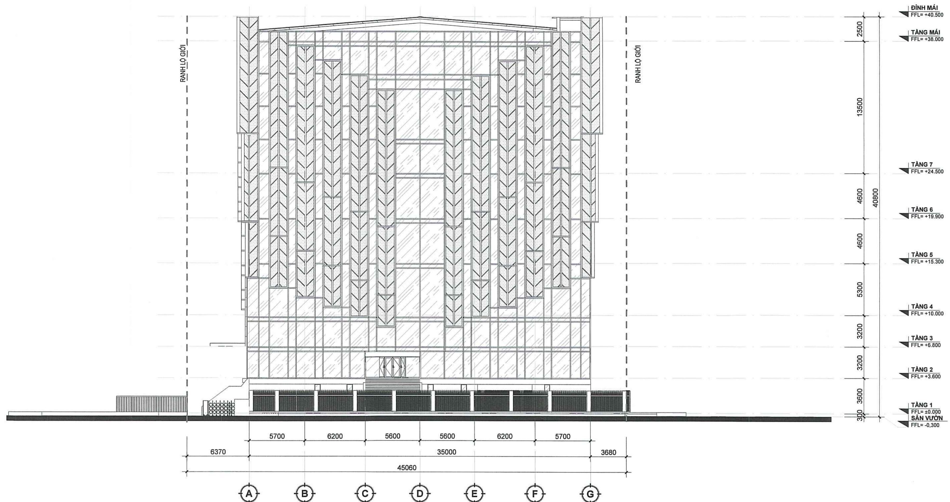
MẶT ĐỨNG TOÀN KHU TRỤC A-G TL/ 1 : 200
