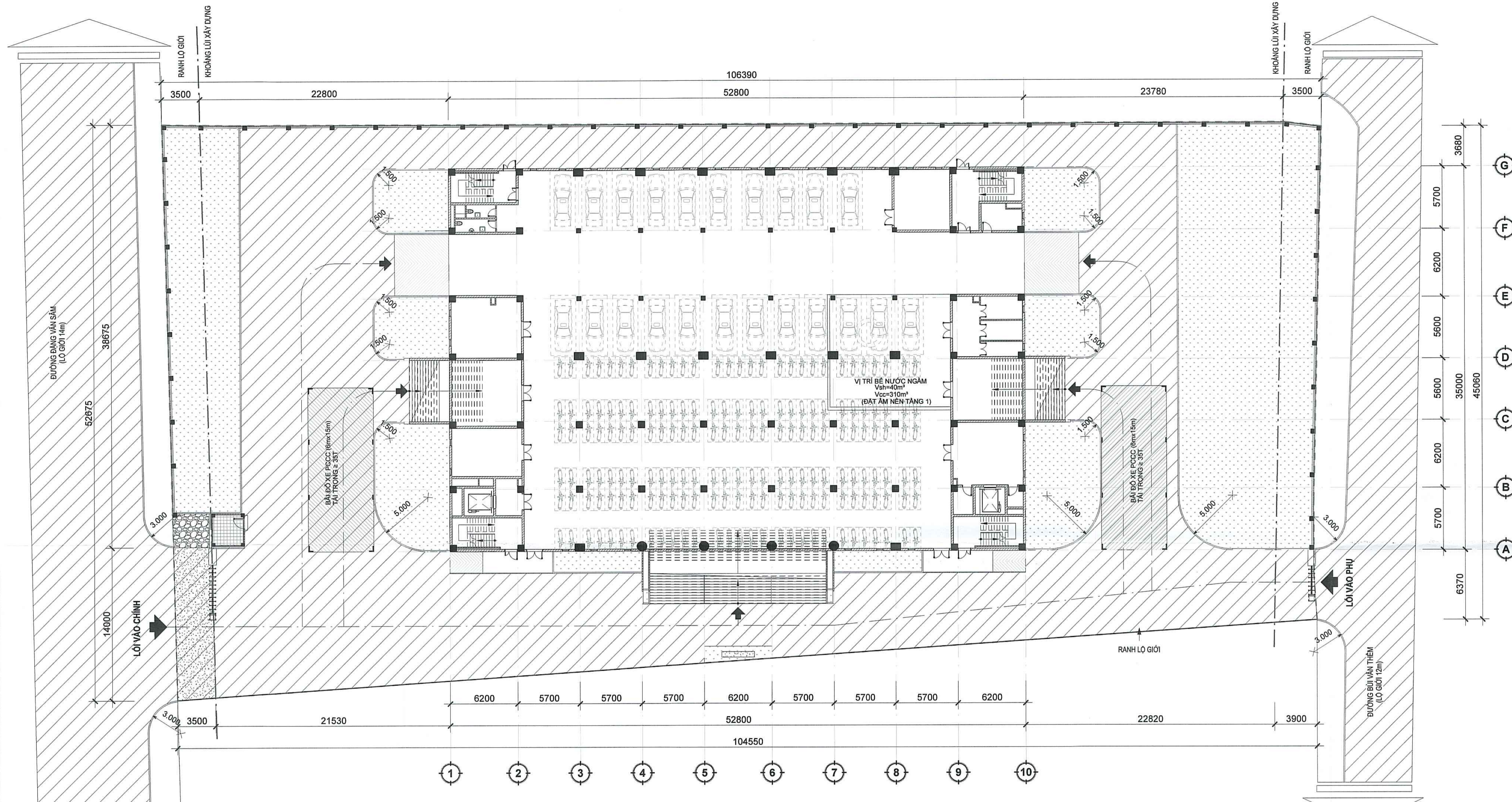
MẶT BẰNG TỔNG THỂ SÂN ĐƯỜNG TL/ 1 : 200
