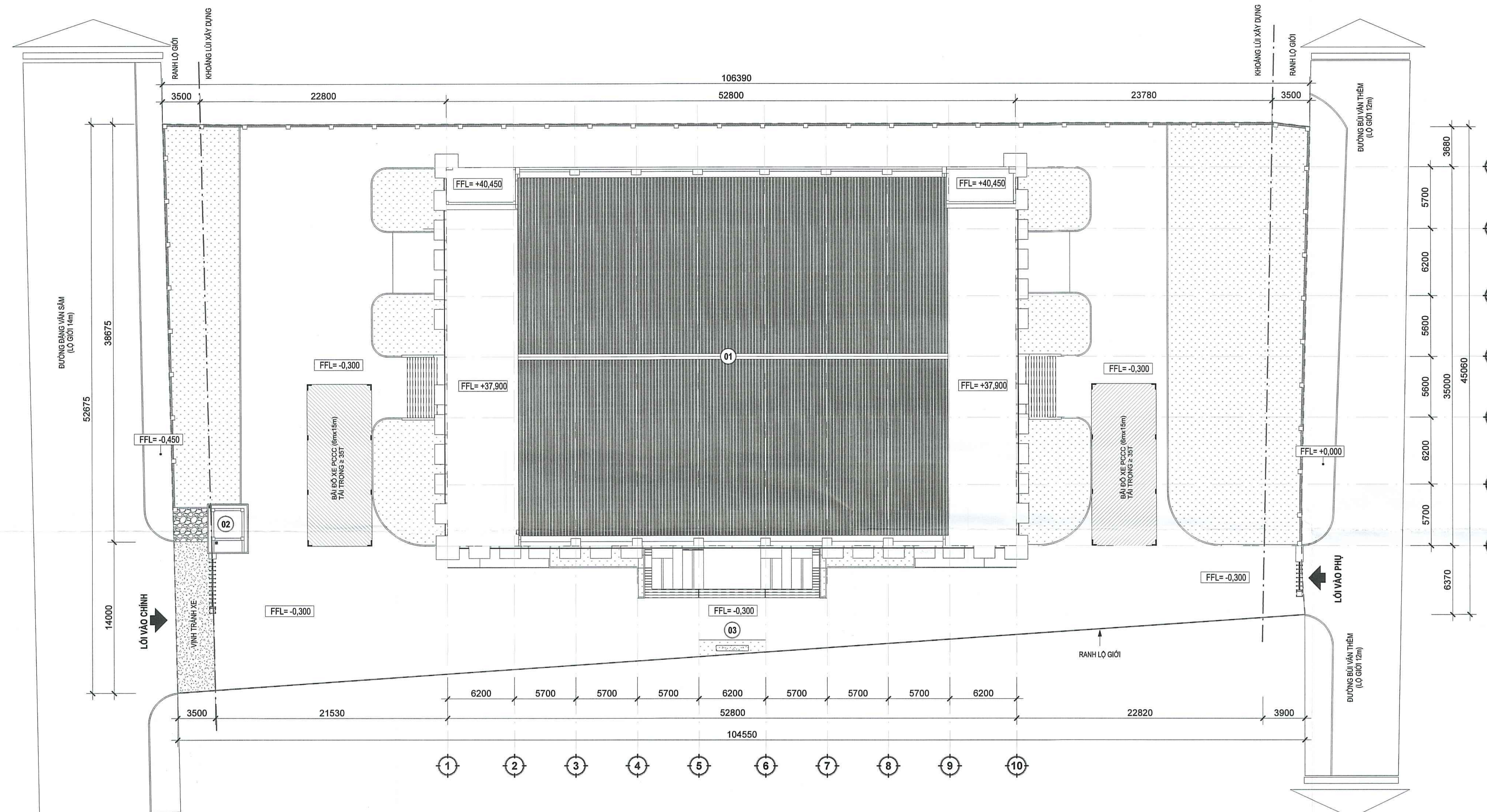
MẶT BẰNG TỔNG THỂ TẦNG MÁI TL/ 1 : 200
