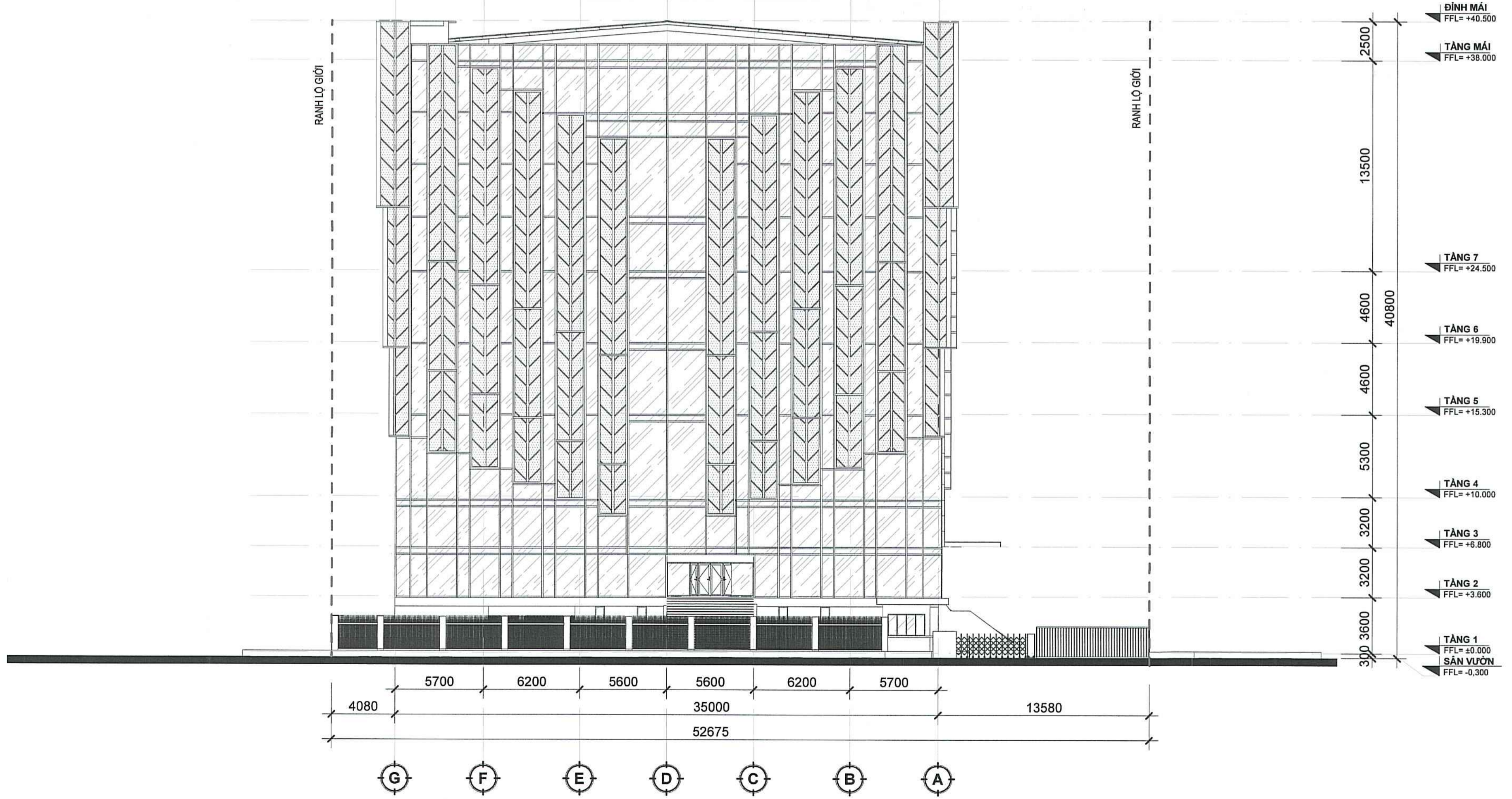
MẶT ĐỨNG TOÀN KHU TRỤC G-A TL/ 1 : 200
