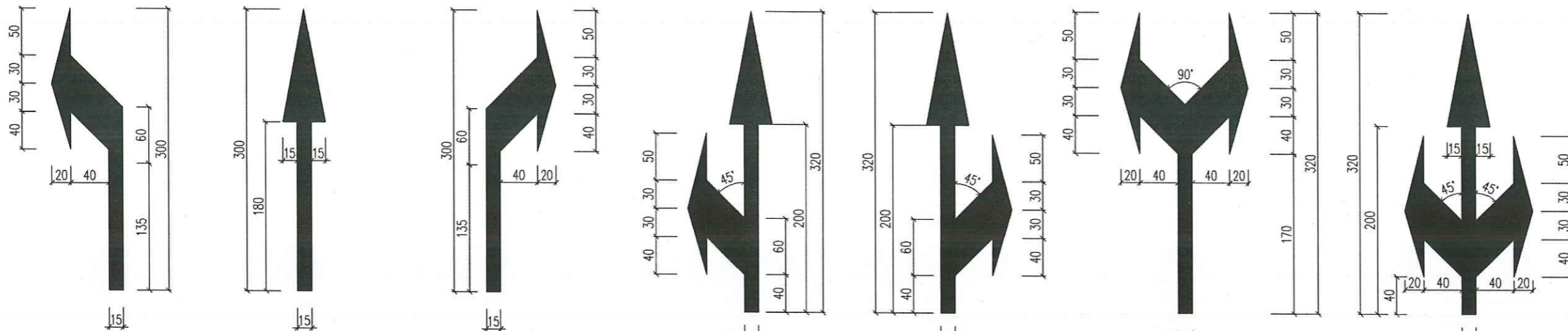
Vạch 9.3 a (Vạch mũi tên chỉ hướng rẽ trái) Vạch 9.3 b (Vạch mũi tên chỉ hướng đi thẳng) Vạch 9.3 c (Vạch mũi tên chỉ hướng rẽ phải) Vạch 9.3 e (Vạch mũi tên chỉ hướng đi thẳng và rẽ trái) Vạch 9.3 f (Vạch mũi tên chỉ hướng đi thẳng và rẽ phải) Vạch 9.3 g (Vạch mũi tên chỉ hướng rẽ trái và rẽ phải) Vạch 9.3 h (Vạch mũi tên chỉ hướng đi thẳng, rẽ trái và rẽ phải)
