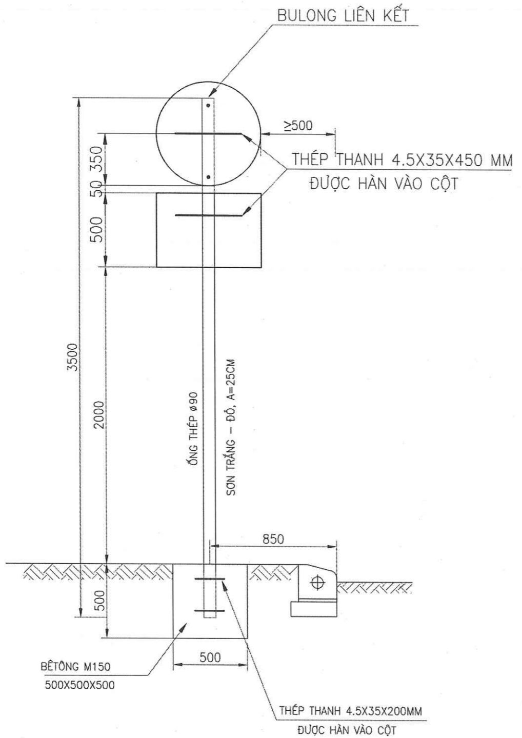
CHI TIẾT CỘT BIỂN BÁO LOẠI 1A
