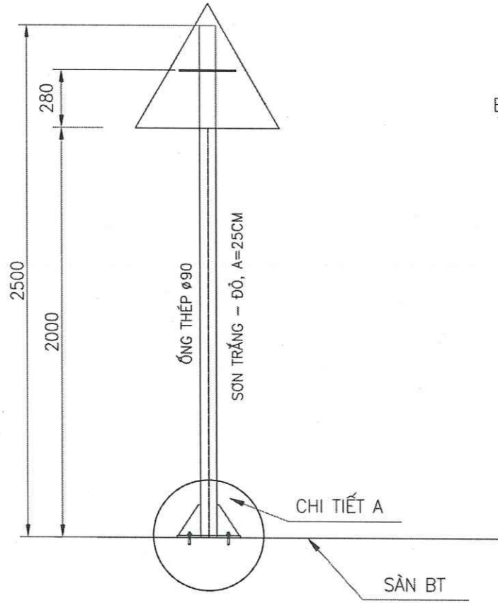
CHI TIẾT CỘT BIỂN BÁO LOẠI 1C
