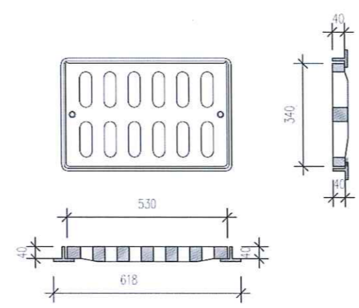
CHI TIẾT SONG CHẨN RÁC 530x340x40, TẢI TRỌNG 25T
