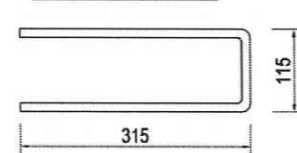
CHI TIẾT 4: D12, L=745
