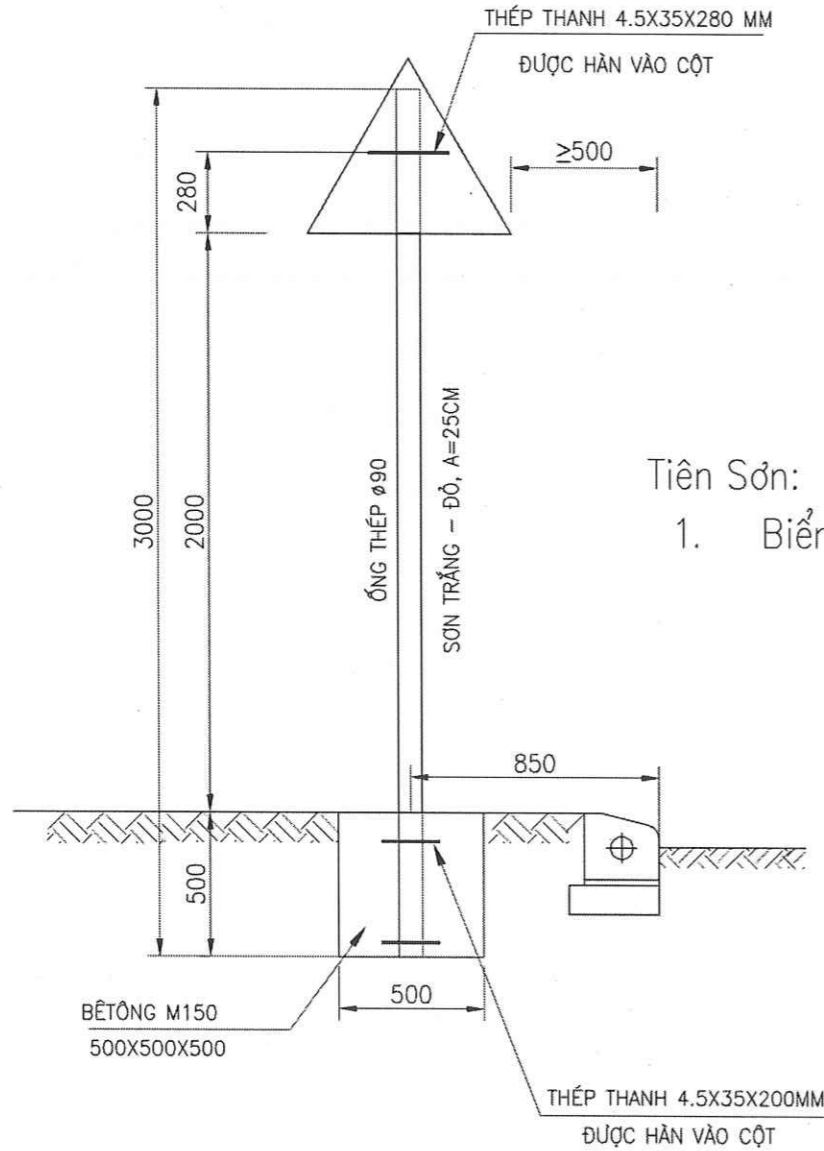
CHI TIẾT CỘT BIỂN BÁO LOẠI 1B
