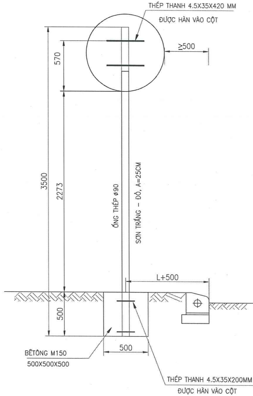
CHI TIẾT CỘT BIỂN BÁO LOẠI 1A
