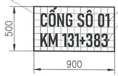
CHI TIẾT BIỂN TÊN CỐNG
