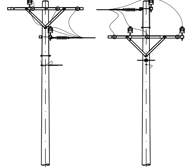
TRỤ V.NGBI.T158P .18T TRƯỚC VÀ SAU SỬA CHỮA
