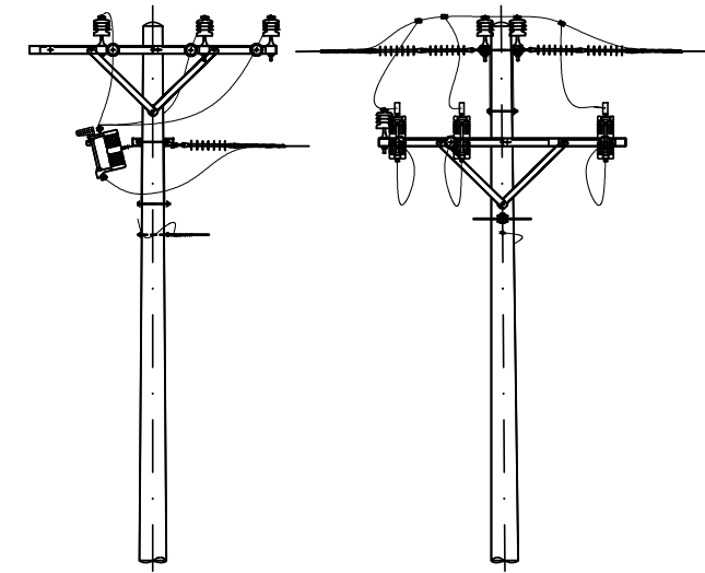
TRỤ V.NGBI.T148P SAU SỬA CHỮA
