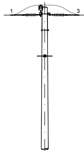
TRỤ V.LA2-3.T07T.33P SAU SỬA CHỮA
