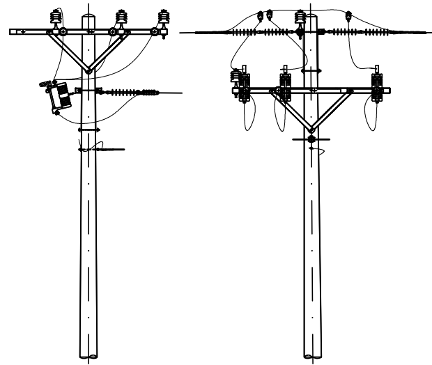
TRỤ V.NGBI.T148P TRƯỚC SỬA CHỮA
