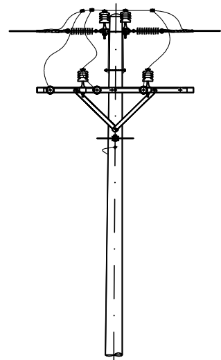
TRỤ V.NGBI.T162P SAU SỬA CHỮA
