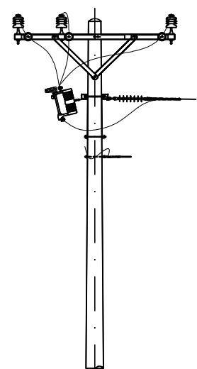
TRỤ V.ĐS6.T15T TRƯỚC SỬA CHỮA
