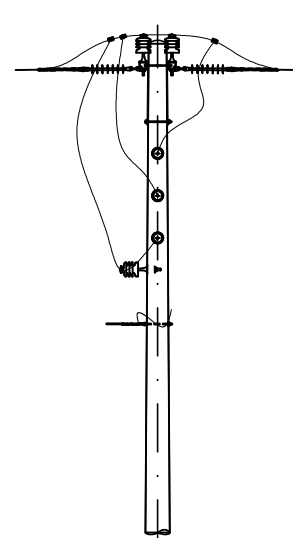
TRỤ V.NGBI.T158P-158AP SAU SỬA CHỮA
