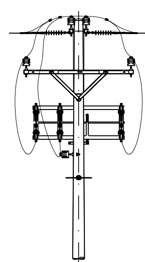
TRỤ V.HUTP.T41P TRƯỚC VÀ SAU SỬA CHỮA
