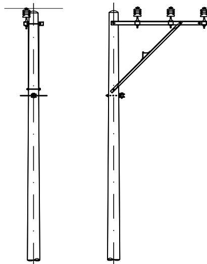
TRỤ V.LEVL.T81P, V.HUTP.T61P, V.NGBI.T95P TRƯỚC VÀ SAU SỬA CHỮA
