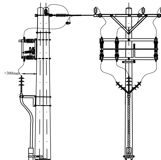
TRỤ V.NGBI.T99P TRƯỚC VÀ SAU SỬA CHỮA
