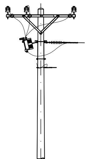
TRỤ V.ĐS6.T15T SAU SỬA CHỮA
