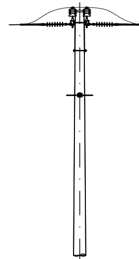
TRỤ V.NGBI.T166P.6T SAU SỬA CHỮA
