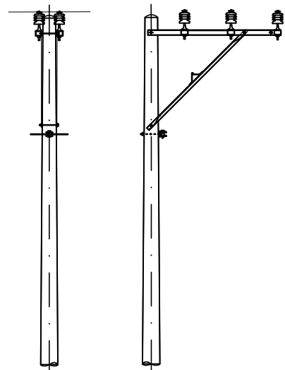
TRỤ V.NGBI.T40P.3T TRƯỚC VÀ SAU SỬA CHỮA
