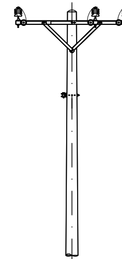
TRỤ V.NGBI.T166P.6T SAU SỬA CHỮA
