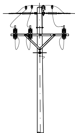
TRỤ V.ĐS6.T15T TRƯỚC SỬA CHỮA
