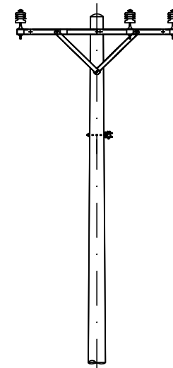
TRỤ V.NGBI.T166P.5T SAU SỬA CHỮA
