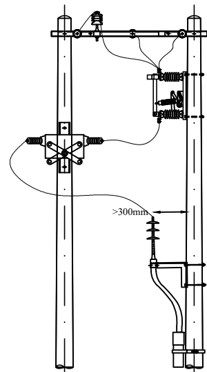
TRỤ V.NGBI.T154P TRƯỚC SỬA CHỮA
