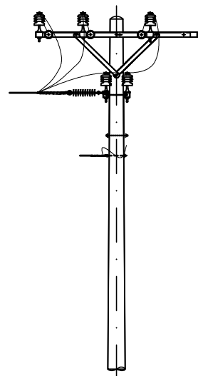
TRỤ V.AP4.T16T TRƯỚC VÀ SAU SỬA CHỮA
