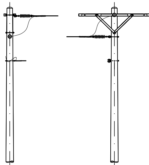
TRỤ V.AP4.T16P.33.10P TRƯỚC SỬA CHỮA
