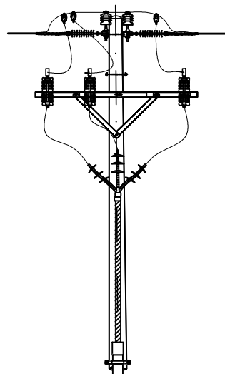
TRỤ V.LEVL.T70AP TRƯỚC VÀ SAU SỬA CHỮA
