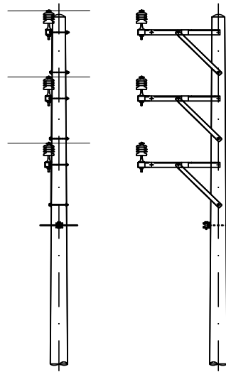
TRỤ V.NGBI.T135.1 TRƯỚC VÀ SAU SỬA CHỮA
