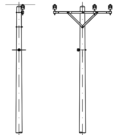
TRỤ V.LA2-3.T103T, V.LA2-3.T107T, V.T148P.1T TRƯỚC VÀ SAU SỬA CHỮA
