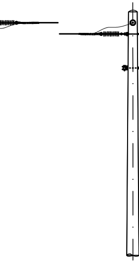
TRỤ V.LA2-3.T49T.28T SAU SỬA CHỮA
