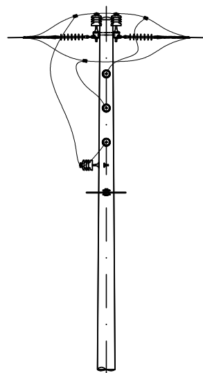
TRỤ V.NGBI.T158P-158AP TRƯỚC SỬA CHỮA
