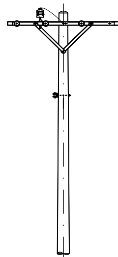
TRỤ V.LA2-3.T07T.33P TRƯỚC SỬA CHỮA
