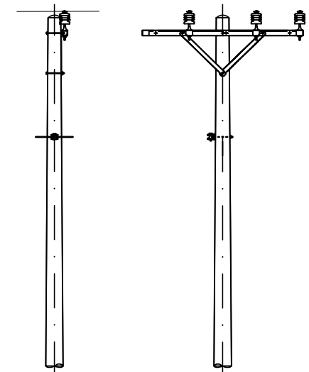
TRỤ V.AP4.T13T, V.AP4.T16P.63P, V.LA2-3.T07T.28P, V.LA2-3.T07T.30P, V.LEVL.T16P.1, V.NGBI.T147P TRƯỚC VÀ SAU SỬA CHỮA
