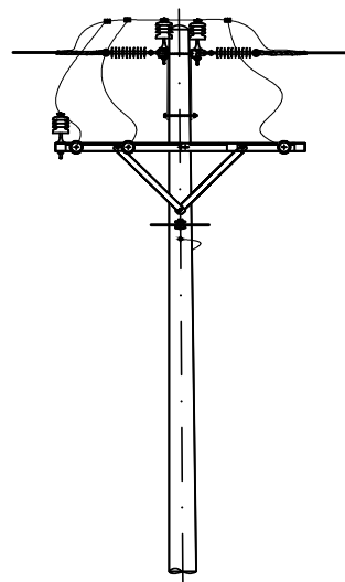
TRỤ V.AP4.T16T TRƯỚC VÀ SAU SỬA CHỮA
