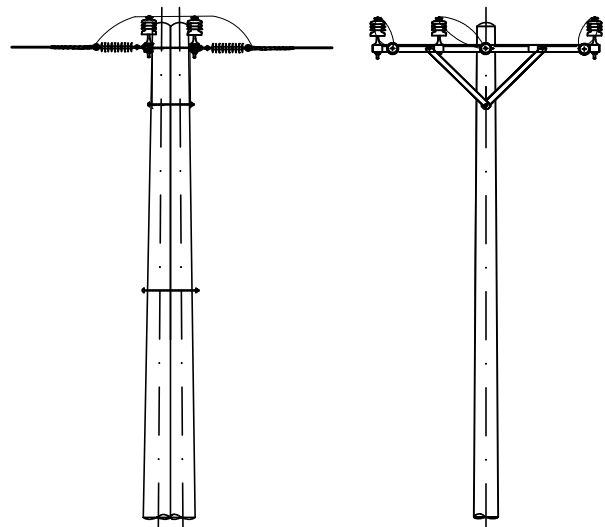
TRỤ V.AP4.T20T TRƯỚC VÀ SAU SỬA CHỮA
