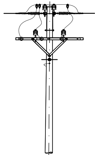
TRỤ V.NGBI.T162P TRƯỚC SỬA CHỮA
