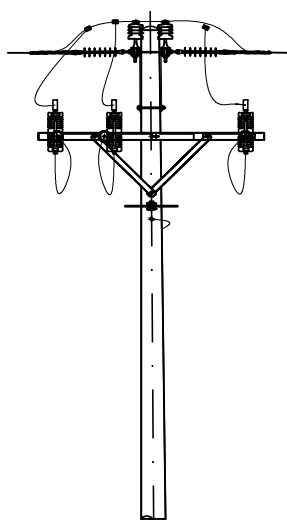
TRỤ V.ĐS6.T15T SAU SỬA CHỮA
