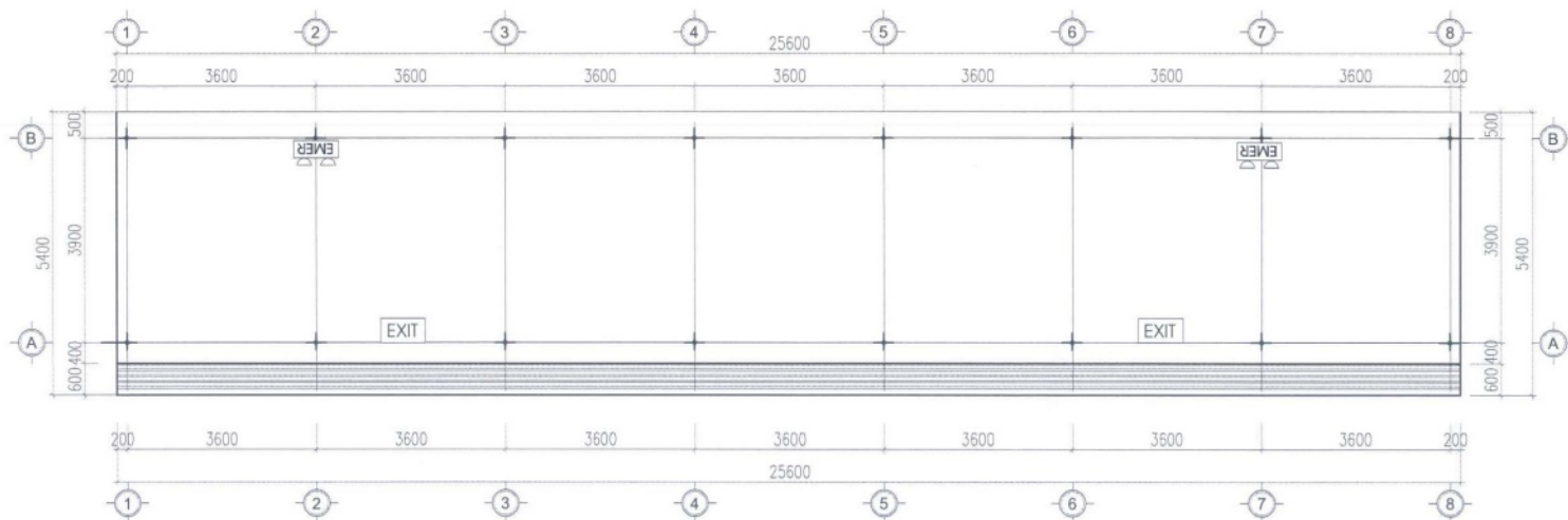
MẶT BẰNG HỆ THỐNG ĐÈN EXIT-SỰ CỐ TẦNG 1 NHÀ ĐÉ XE GIÁO VIÊN
