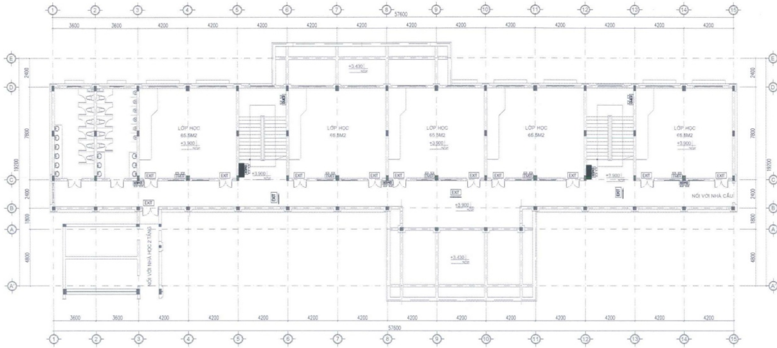
MẶT BẰNG HỆ THỐNG ĐÈN EXIT- SỰ CỐ TẦNG 2 NHÀ LỚP HỌC 20 PHÒNG
