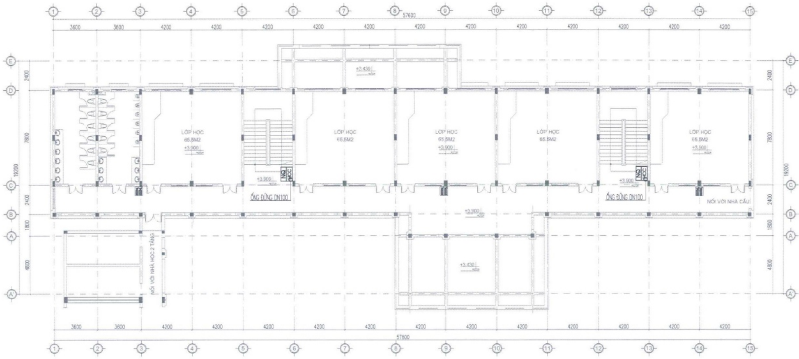
MẶT BẰNG HỆ THỐNG CHỮA CHÁY TẦNG 2 NHÀ LỚP HỌC 20 PHÒNG
