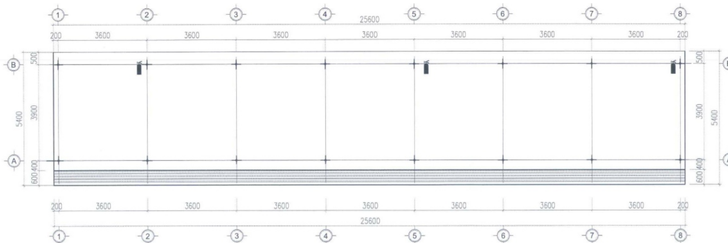
MẶT BẰNG CHỮA CHÁY TẦNG 1 NHÀ ĐỂ XE GIÁO VIÊN
