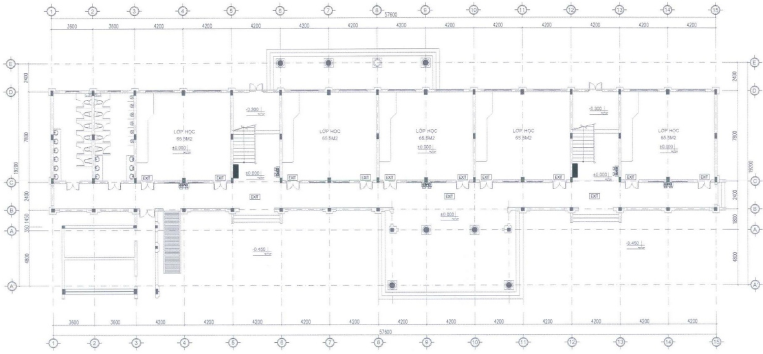
MẶT BẰNG HỆ THỐNG ĐÈN EXIT- SỰ CỐ TẦNG 1 NHÀ LỚP HỌC 20 PHÒNG
