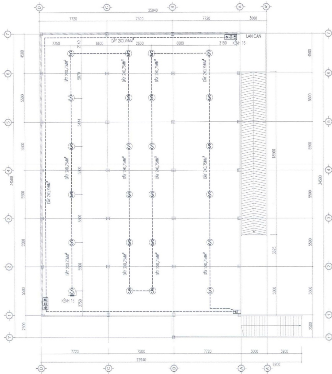
MẶT BẰNG HỆ THỐNG BÁO CHÁY TẦNG 2 NHÀ ĐỂ XE HỌC SINH
