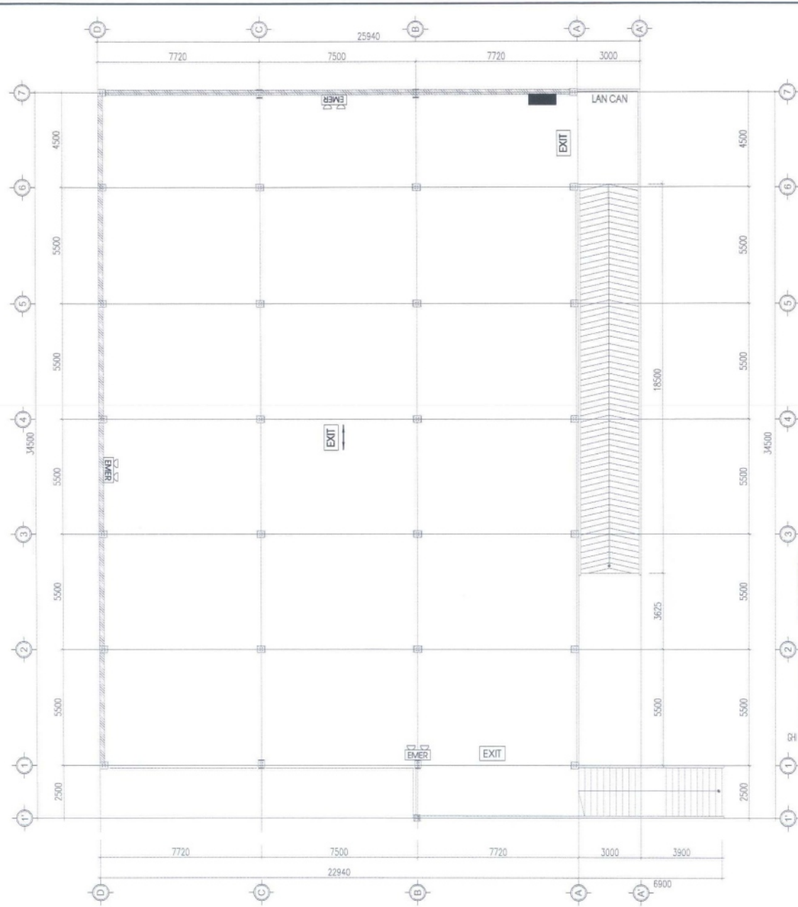
MẶT BẰNG HỆ THỐNG ĐÈN EXIT- SỰ CỐ TẦNG 2 NHÀ ĐỂ XE HỌC SINH
