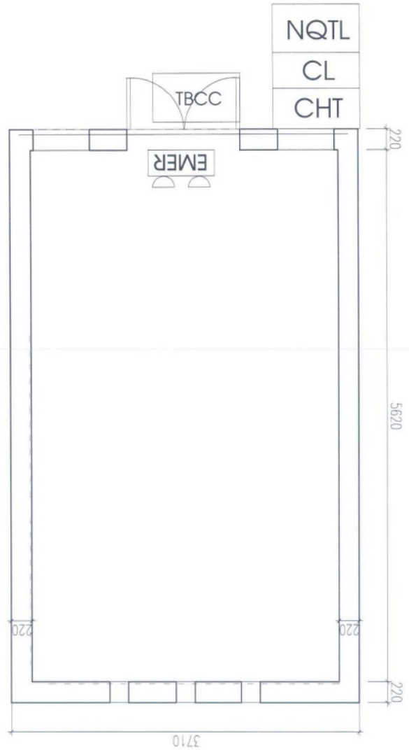
MẶT BẰNG HỆ THỐNG ĐÈN EXIT-SỰ CỐ TRẠM BƠM CHỮA CHÁY
