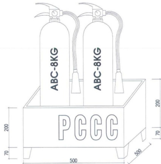
CHI TIẾT LẮP ĐẶT BÌNH CHỮA CHÁY XÁCH TAY
