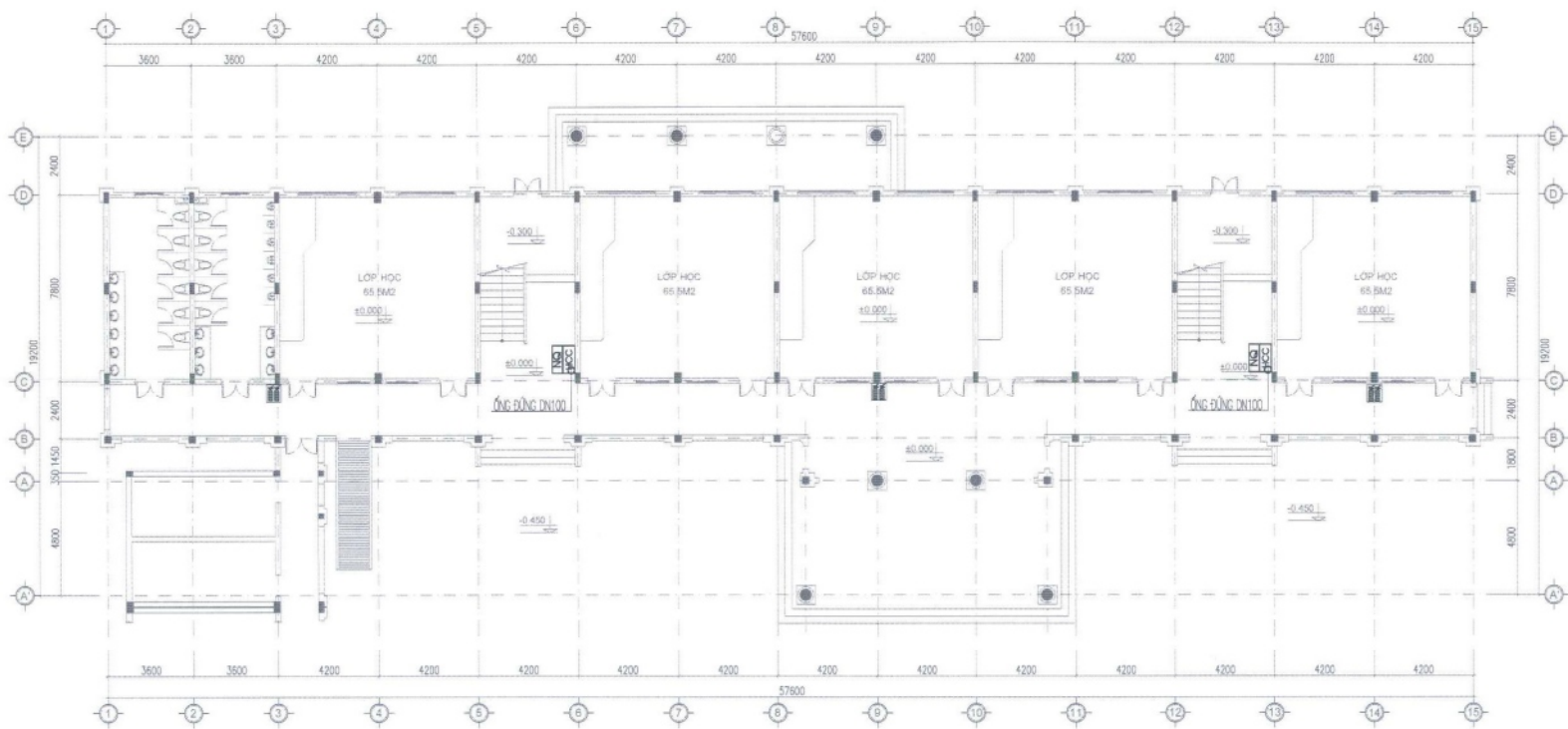
MẶT BẰNG HỆ THỐNG CHỮA CHÁY TẦNG 1 NHÀ LỚP HỌC 20 PHÒNG
