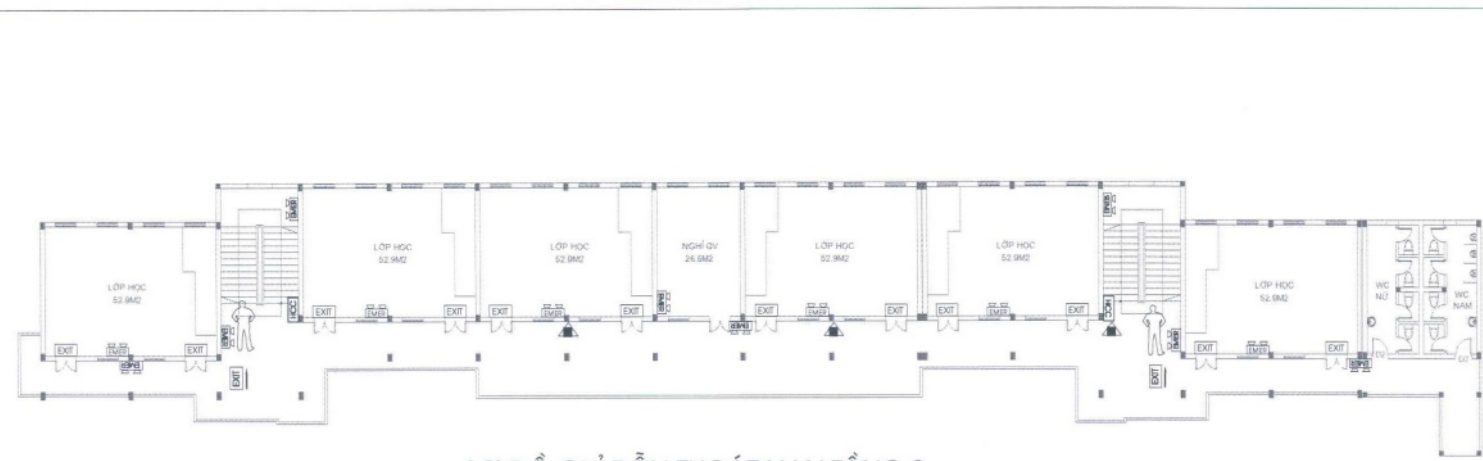
SƠ ĐỒ CHỈ DẪN THOÁT NAN TẦNG 2 NHÀ LỚP HỌC 12 PHÒNG
