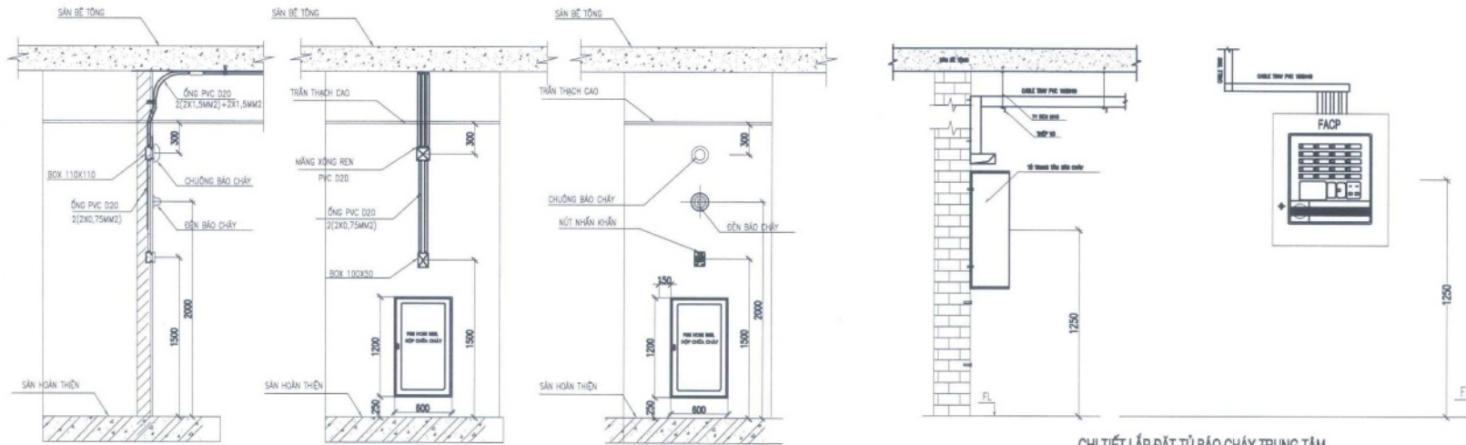
CHI TIẾT LẮP ĐẶT CHUÔNG ĐÈN NÚT NHẤN KHẨN
