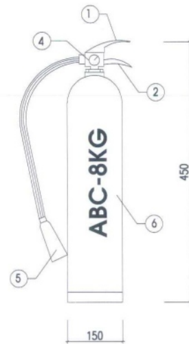
BÌNH CHỮA CHÁY MFZL8 - 8KG
