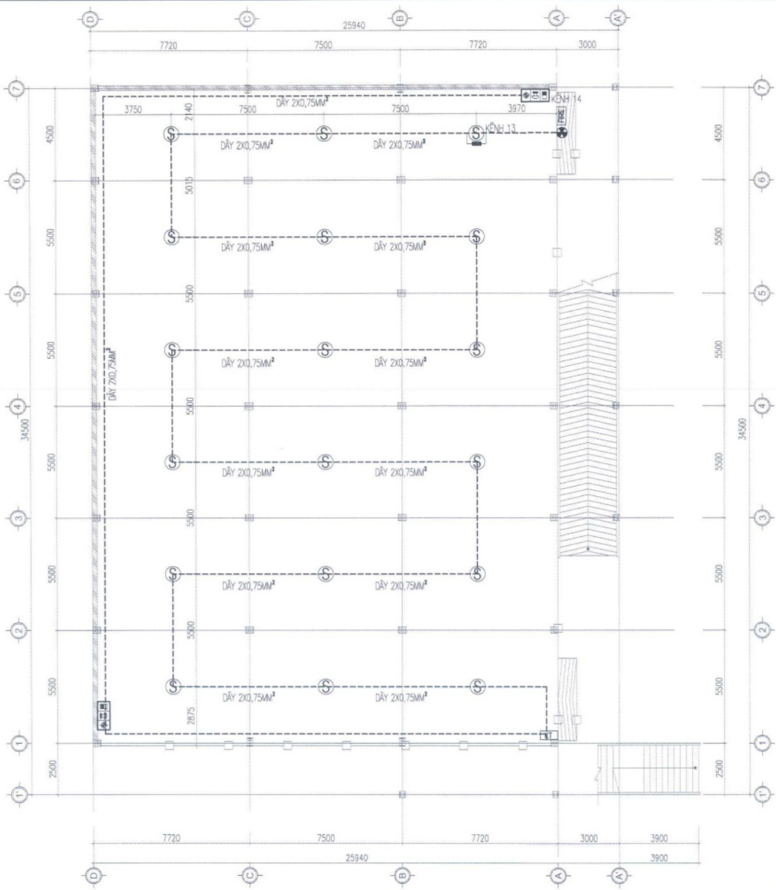
MẶT BẰNG HỆ THỐNG BÁO CHÁY TẦNG 1 NHÀ ĐỂ XE HỌC SINH
