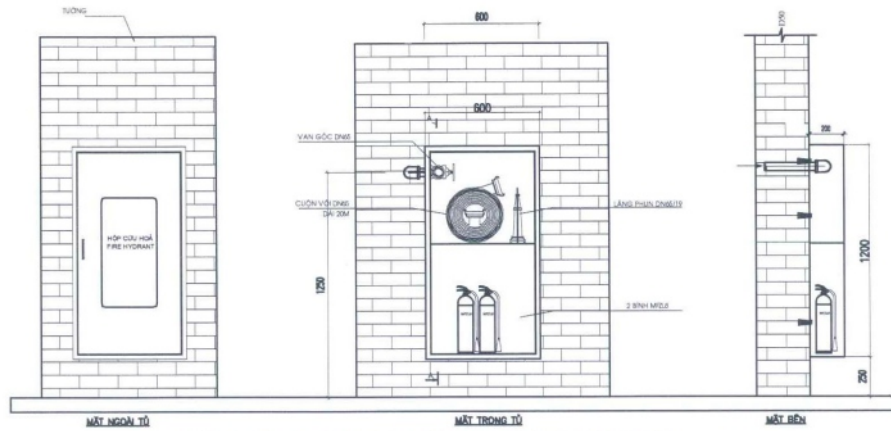
CHI TIẾT HỘP PHƯƠNG TIỆN PCCC TRONG NHÀ
