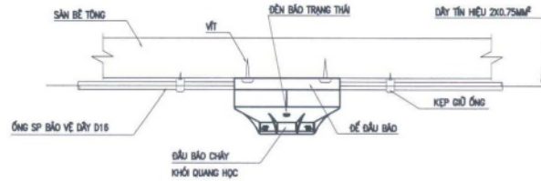
CHI TIẾT LẮP ĐẶT ĐẦU BÁO KHÓI
