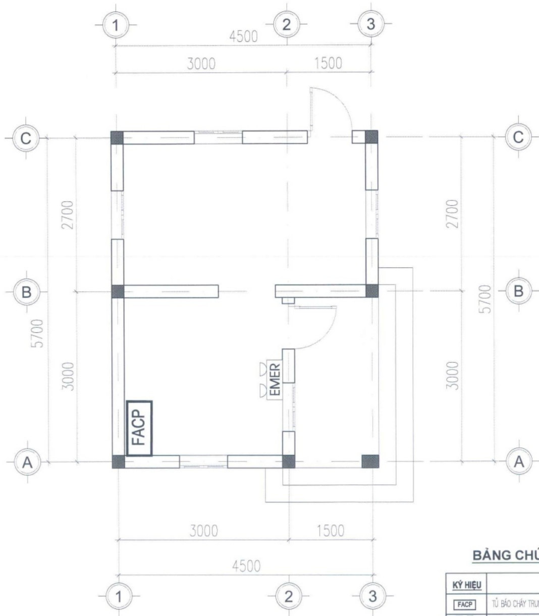
MẶT BẰNG HỆ THỐNG ĐÈN EXIT-SỰ CỐ NHÀ BẢO VỆ
