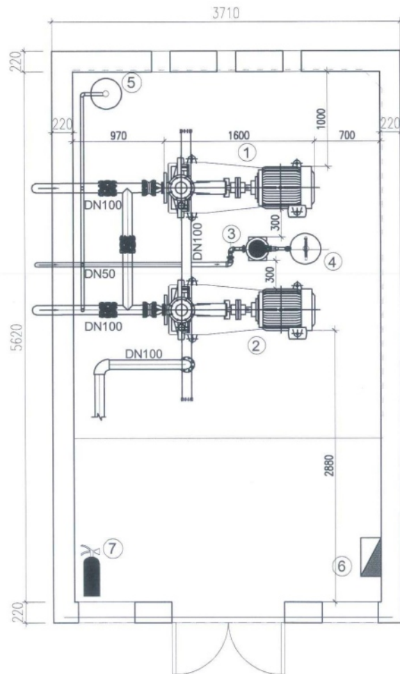
MẶT BẰNG LẮP ĐẶT TRẠM BƠM CHỮA CHÁY
