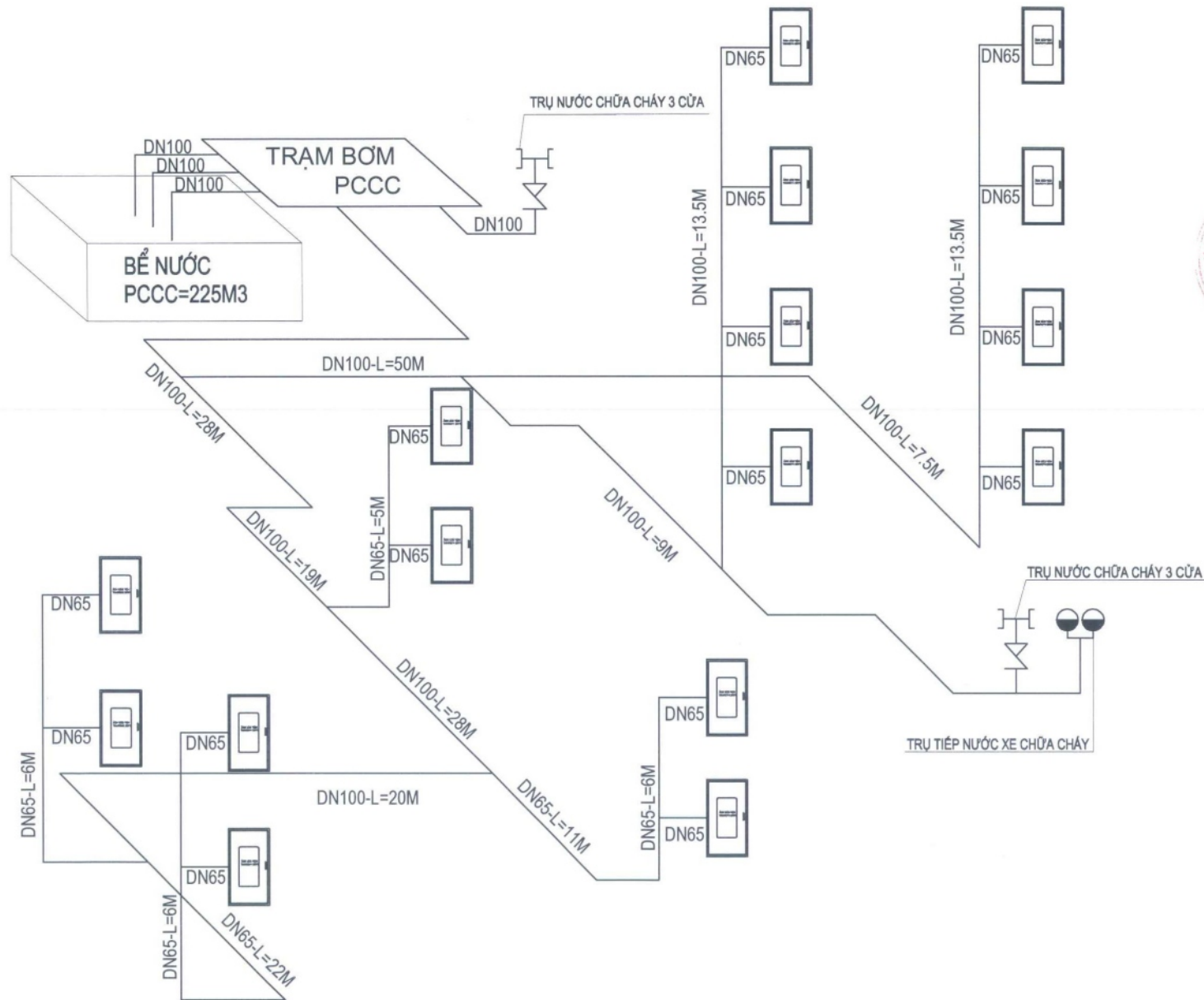
SƠ ĐỒ KHÔNG GIAN HỆ THỐNG CẤP NƯỚC CHỮA CHÁY
