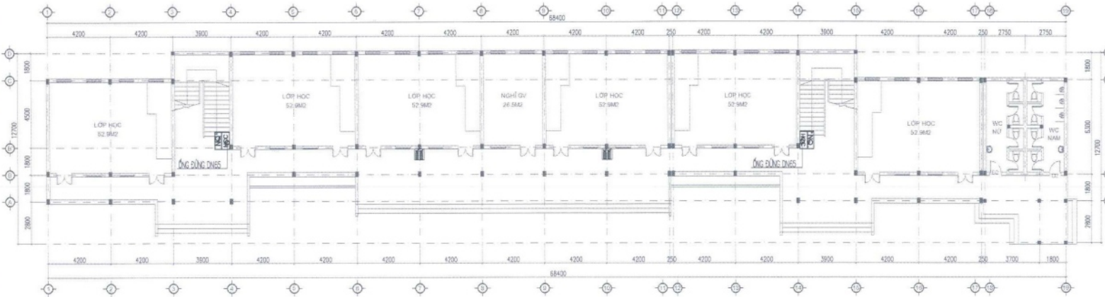
MẶT BẰNG HỆ THỐNG CHỮA CHÁY TẦNG 1 NHÀ LỚP HỌC 12 PHÒNG
