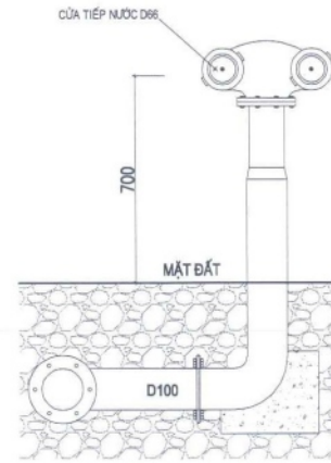
TRỤ TIẾP NƯỚC CHỮA CHÁY
