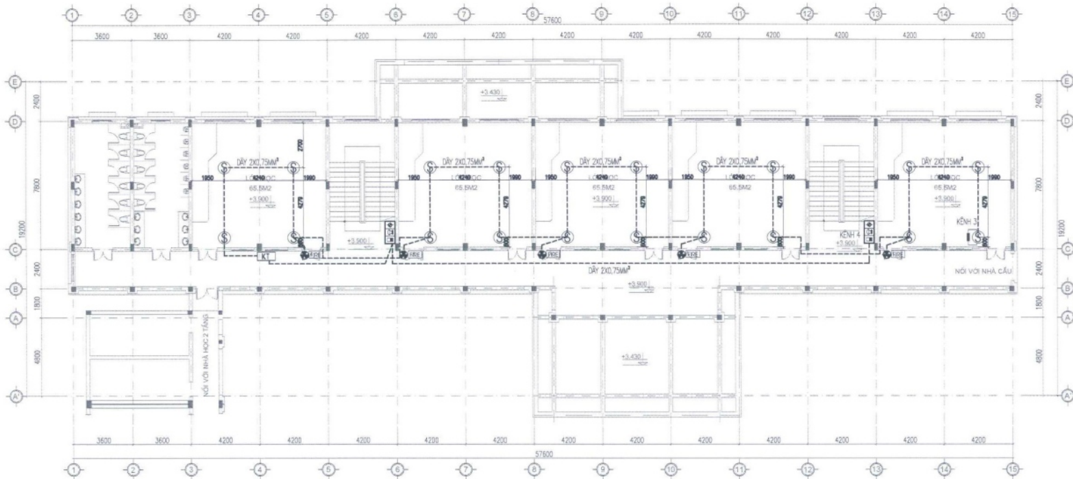
MẶT BẰNG HỆ THỐNG BÁO CHÁY TẦNG 2 NHÀ LỚP HỌC 20 PHÒNG
