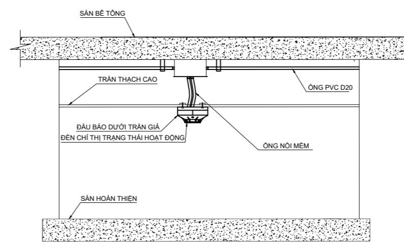
CHI TIẾT LẮP ĐẶT ĐẦU BÁO KHU VỰC CÓ TRẦN GIẢ
