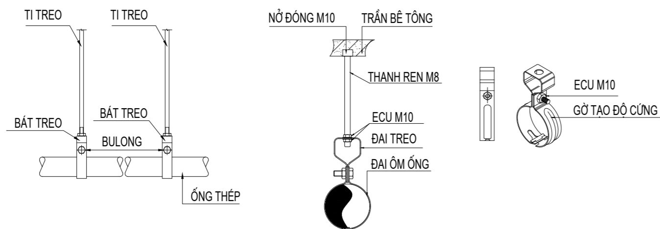
CHI TIẾT TREO ỚNG CHO 1 ỚNG D80 TRỞ XUỐNG
