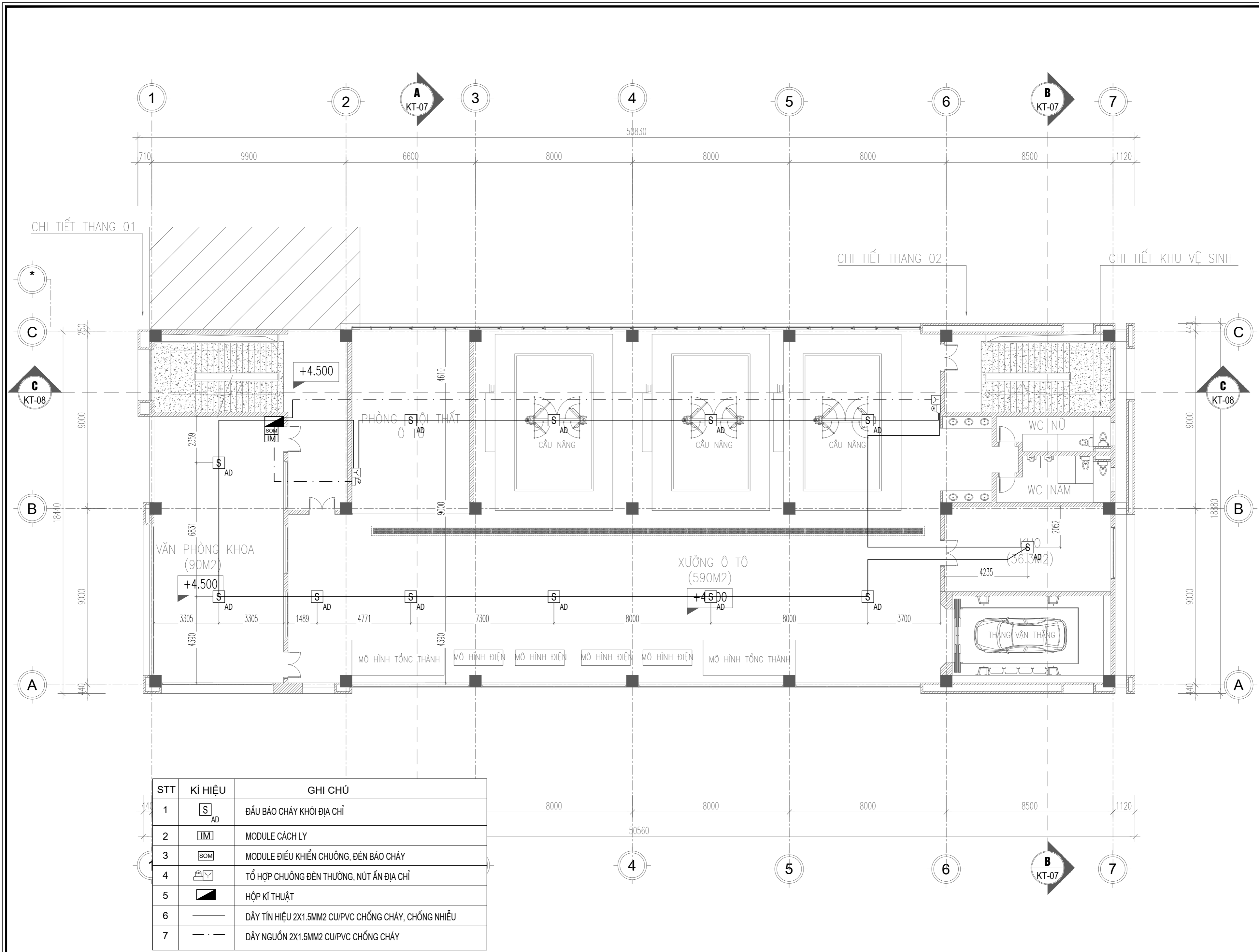
MẶT BẰNG BÁO CHÁY NHÀ XƯỞNG TẦNG 2
