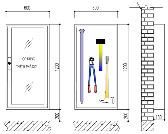
HỘ DỤNG DỤNG CỤ PHÁ ĐỠ:
