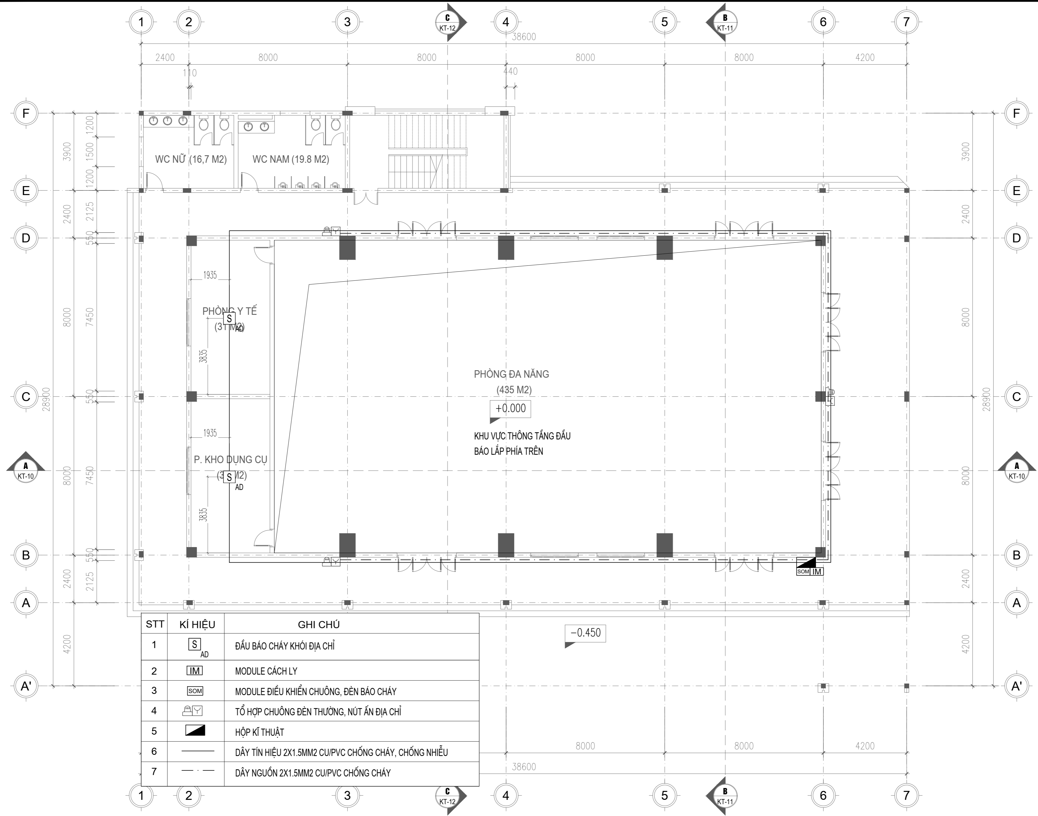
MẶT BẰNG BÁO CHÁY NHÀ GIÁO DỤC THỂ CHẤT TẦNG 1
