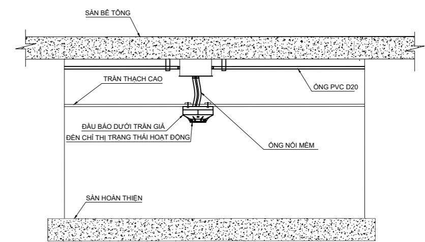
CHI TIẾT LẮP ĐẶT ĐẦU BÁO KHU VỰC CÓ TRẦN GIẢ
