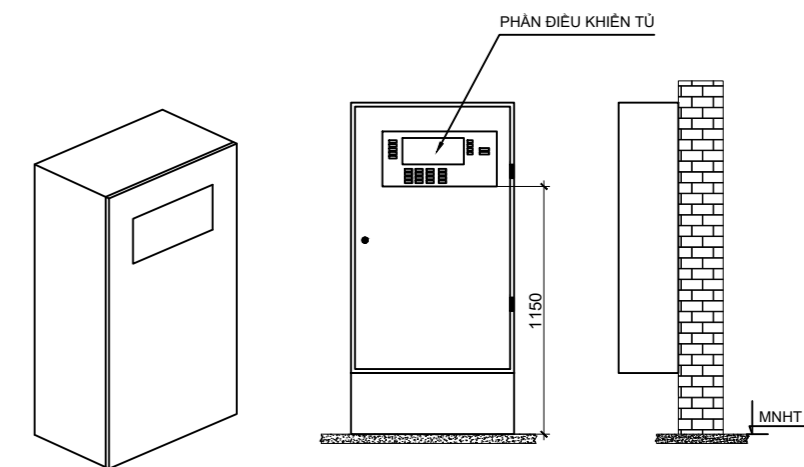
CHI TIẾT LẮP ĐẶT TRUNG TÂM BÁO CHÁY TẠI PHÒNG THƯỜNG TRỰC
