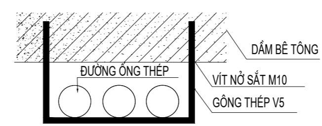
CHI TIẾT TREO ỚNG THÉP D>=80 TẬP TRUNG
