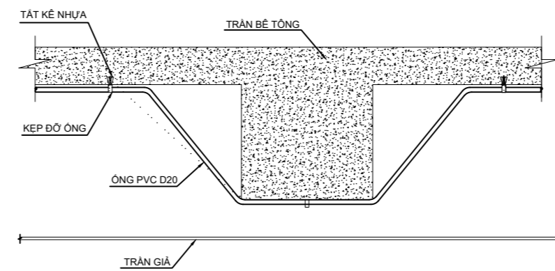
CHI TIẾT LẮP ĐẶT ỚNG QUA DÀM
