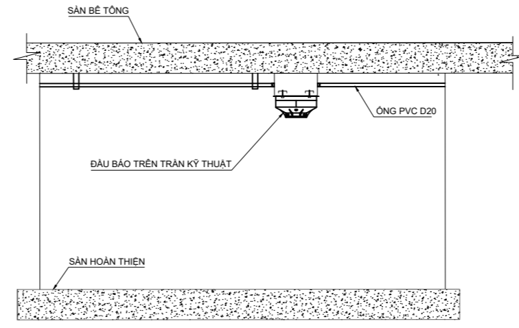
CHI TIẾT LẮP ĐẶT ĐẦU BÁO TRÊN TRẦN KỸ THUẬT
