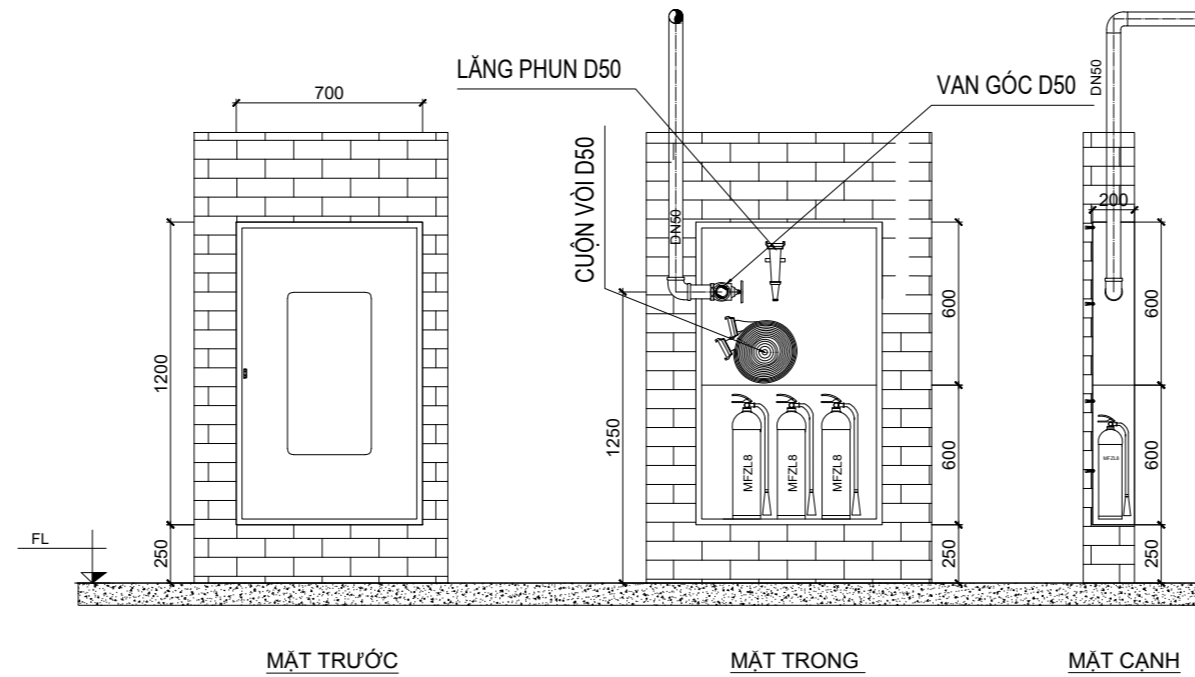
MẶT TRƯỚC
