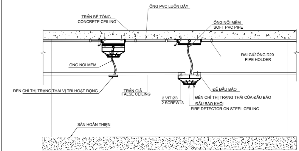
CHI TIẾT LẮP ĐẶT ĐẦU BÁO Ở PHÍA TRÊN TRẦN GIẢ
