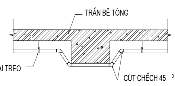
CHI TIẾT LẮP ĐẶT ỚNG QUA DẦM, ỚNG GIÓ
