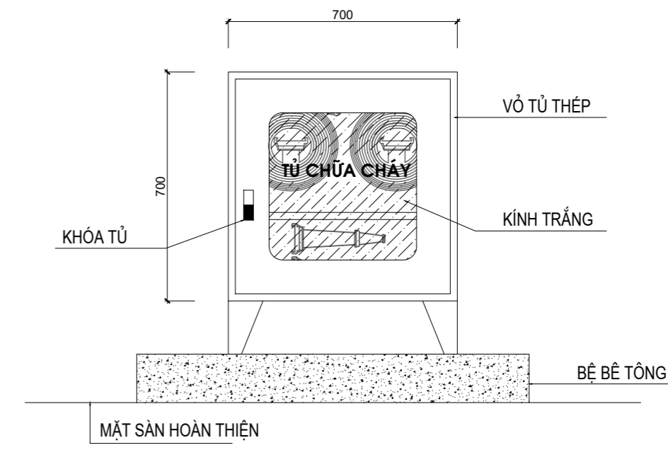
BÊN NGOÀI TỦ HỘ DỤNG PHƯƠNG TIỆN CHỮA CHÁY NGOÀI NHÀ
