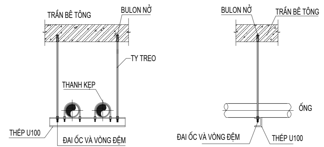
CHI TIẾT TREO ỚNG CHO 1 ỚNG D80 TRỞ LÊN
