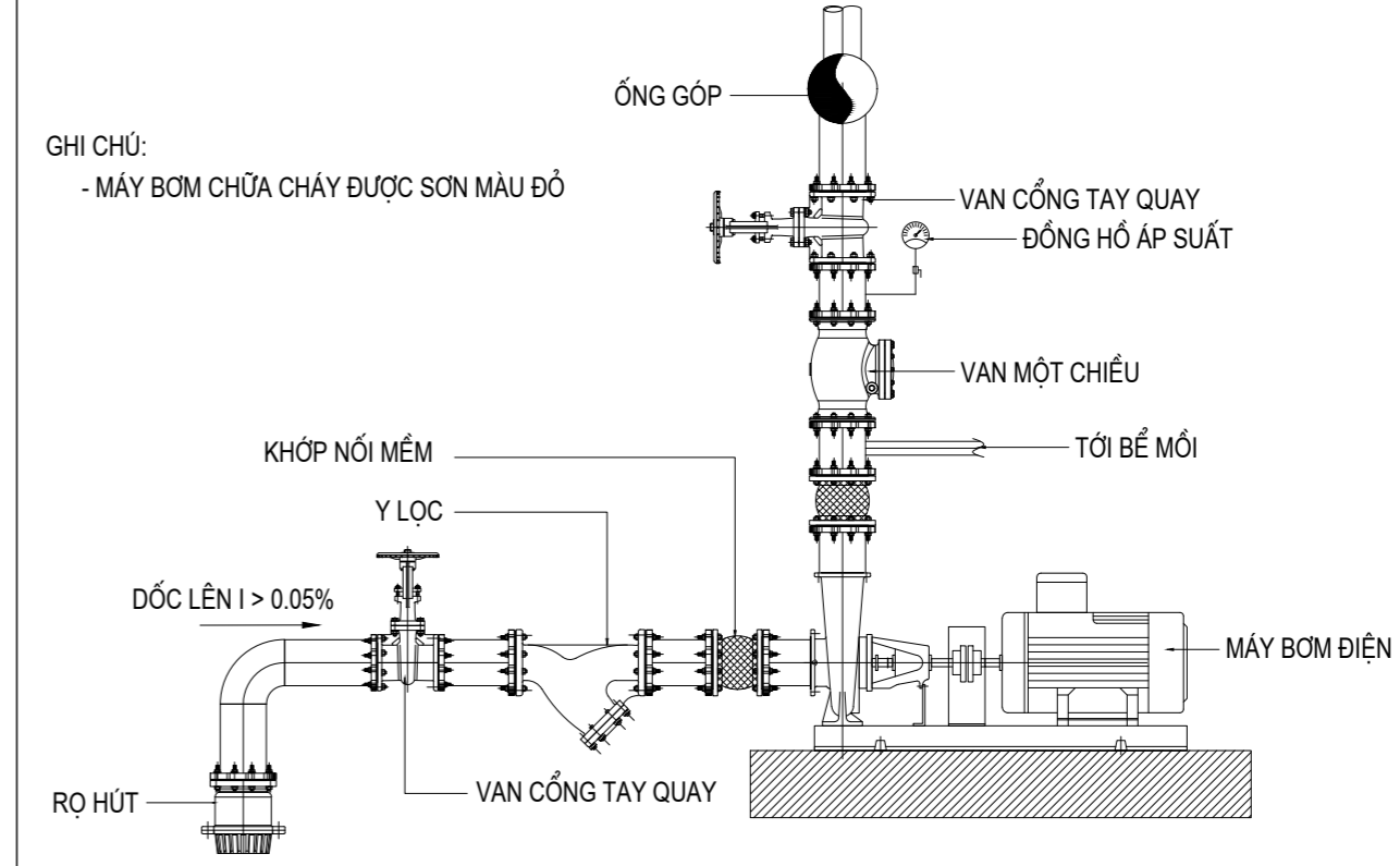
MÁY BƠM CHỮA CHÁY ĐỘNG CƠ ĐIỆN
