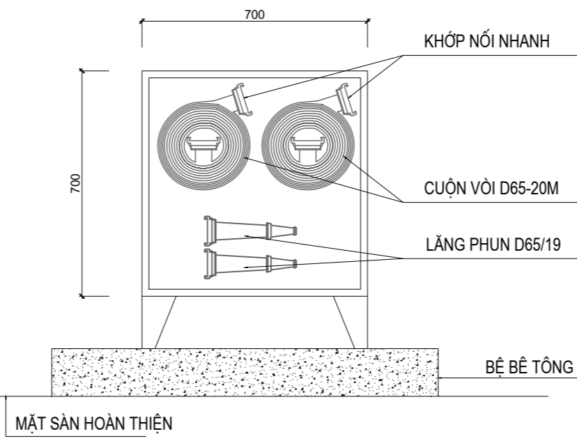
BÊN TRONG TỦ HỘ DỤNG PHƯƠNG TIỆN CHỮA CHÁY NGOÀI NHÀ
