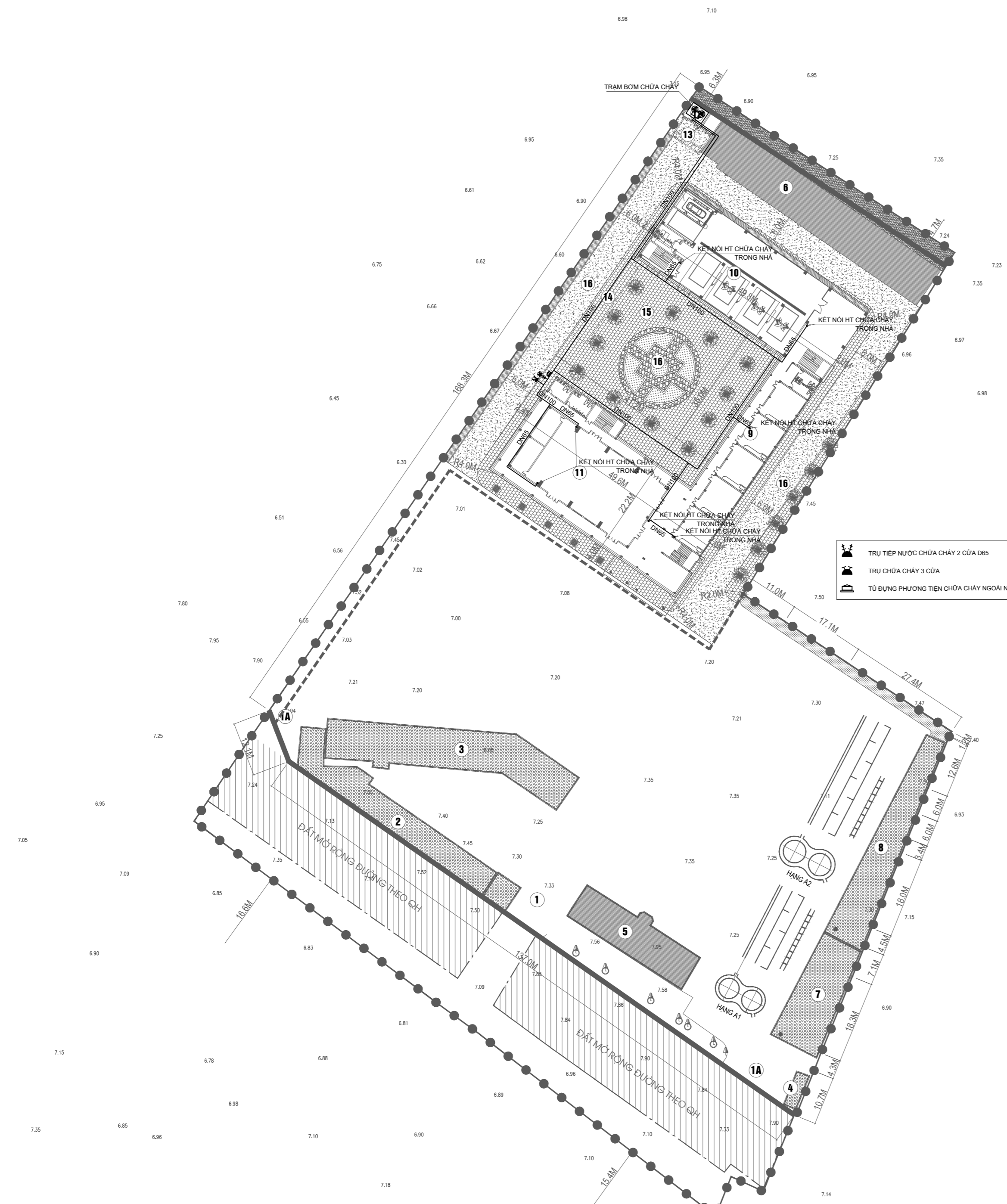
TỔNG MẶT BẰNG CHỮA CHÁY
