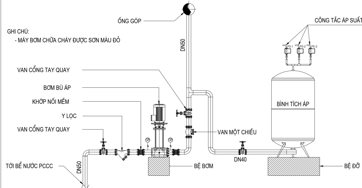
MÁY BƠM BÙ ÁP + BÌNH TÍCH ÁP
