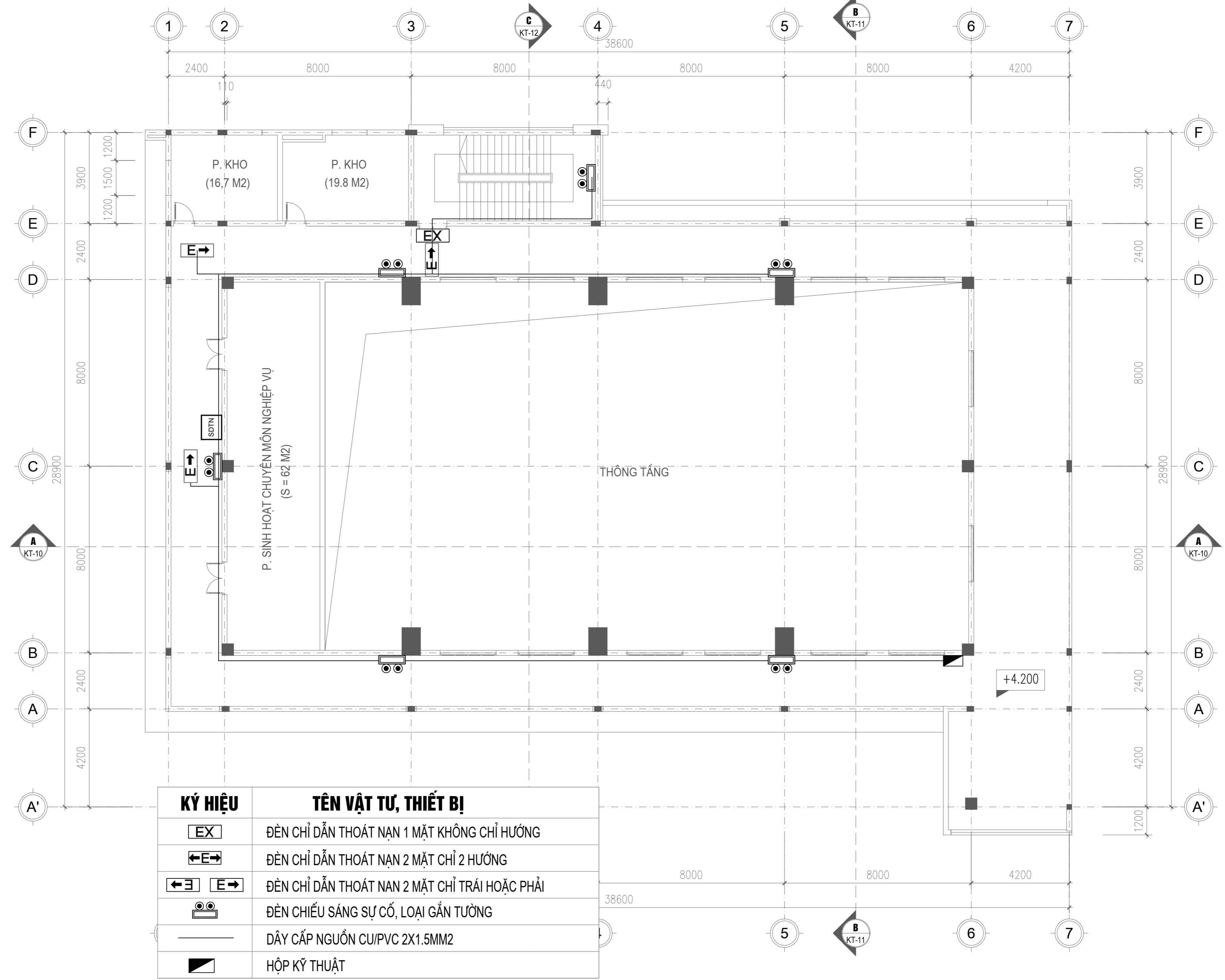
MẶT BẰNG EXIT, SỰ CỐ NHÀ GIÁO DỤC THỂ CHẤT TẦNG 2
