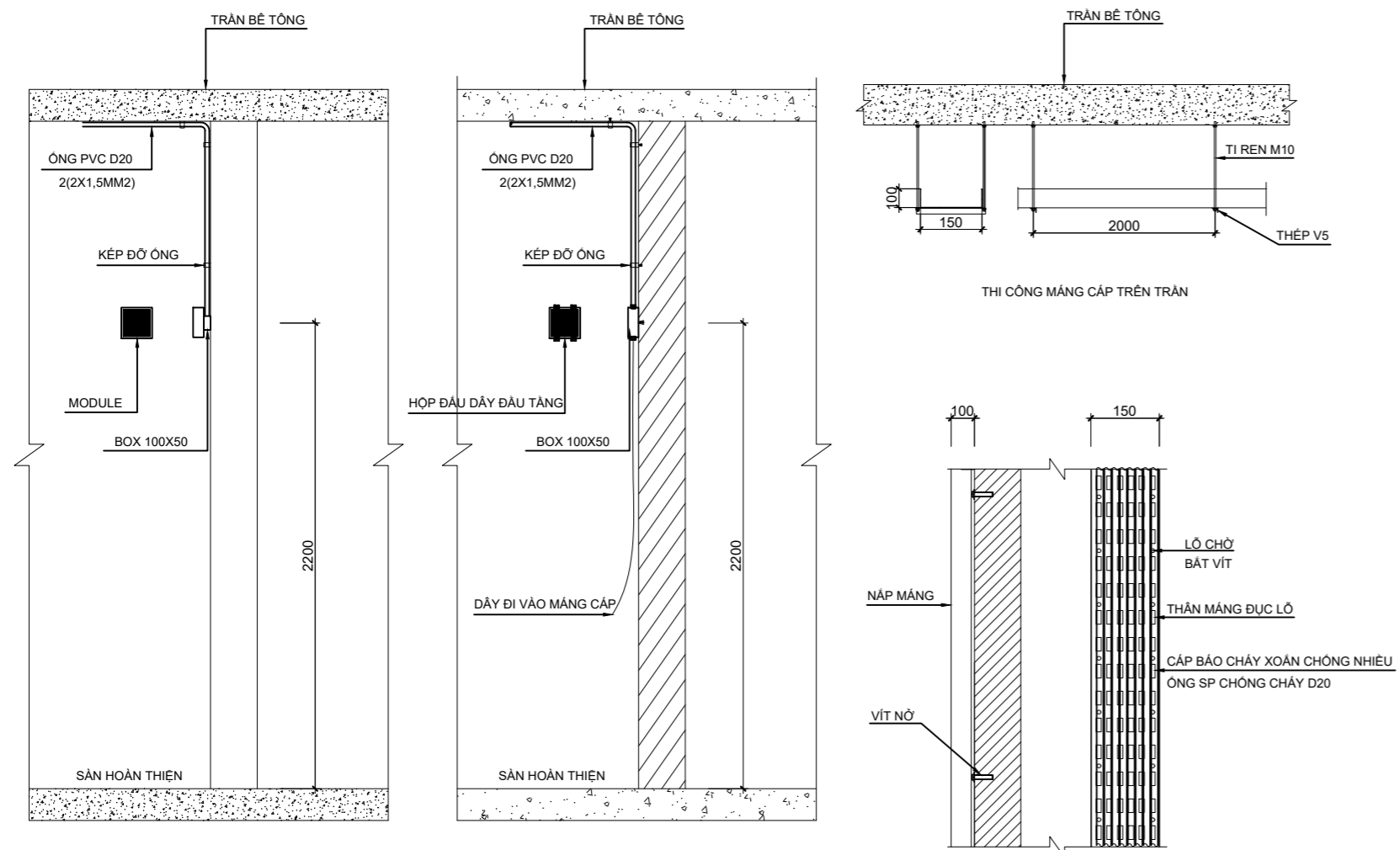
CHI TIẾT LẮP ĐẶT MODULE
