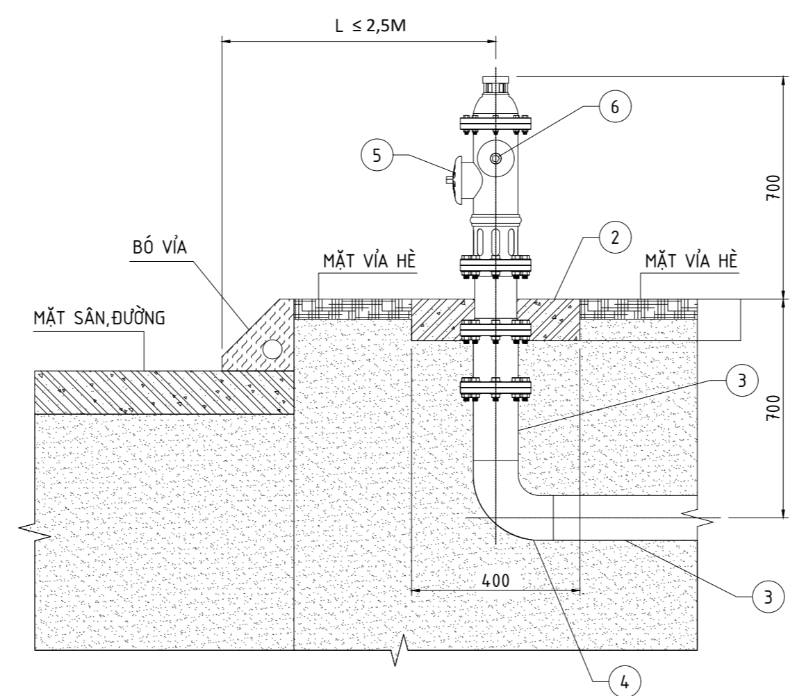
CHI TIẾT LẮP ĐẶT TRỤ NƯỚC CHỮA CHÁY 3 CỬA
