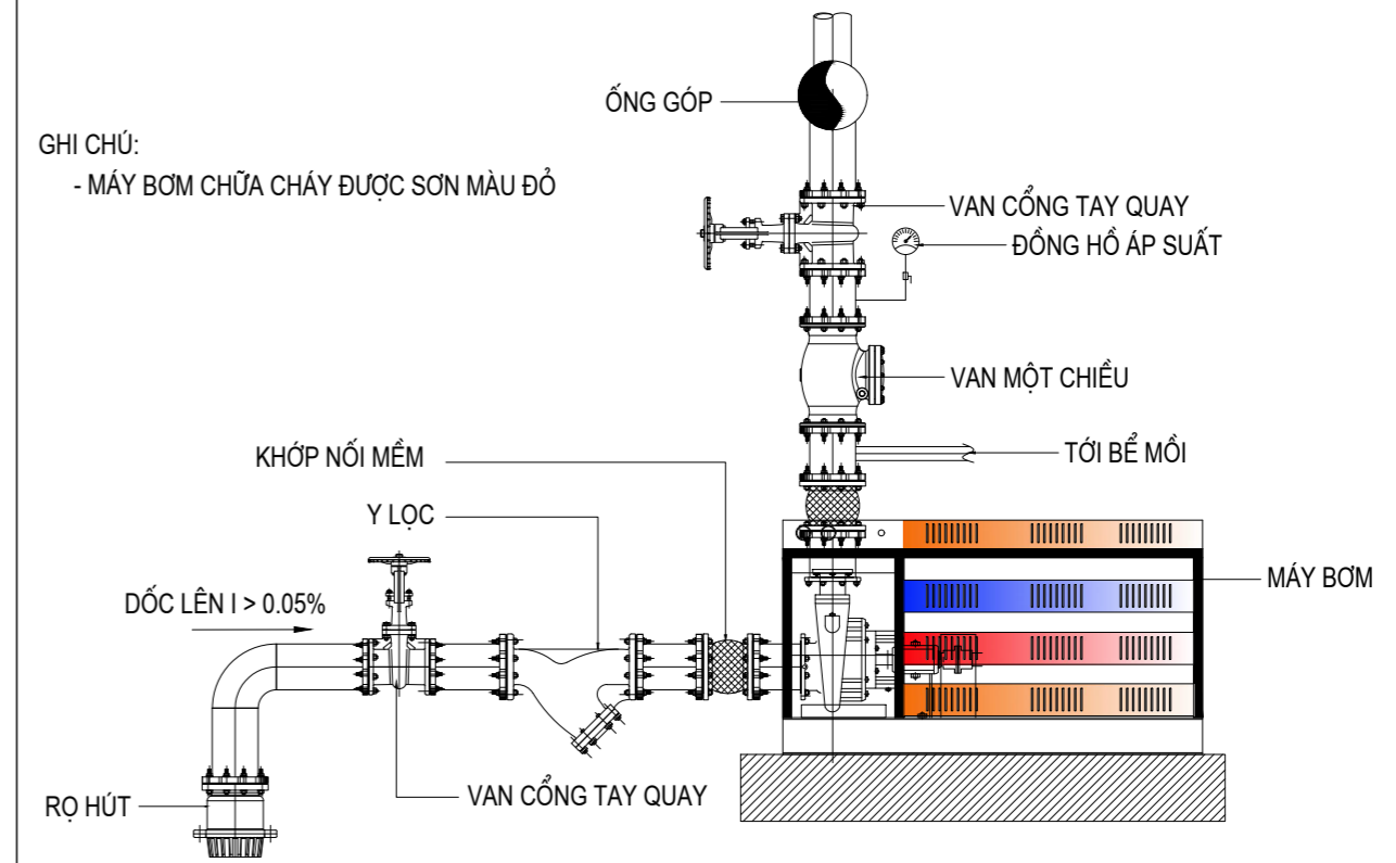
MÁY BƠM CHỮA CHÁY ĐỘNG CƠ DIESEL
