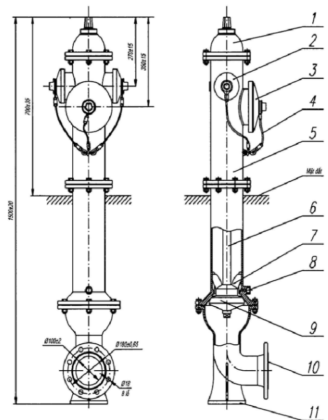
CHI TIẾT TRỤ NƯỚC CHỮA CHÁY 3 CỬA
