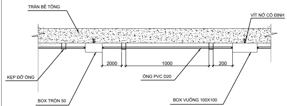
CHI TIẾT LẮP ĐẶT BOX VÀ PHỤ KIỆN
