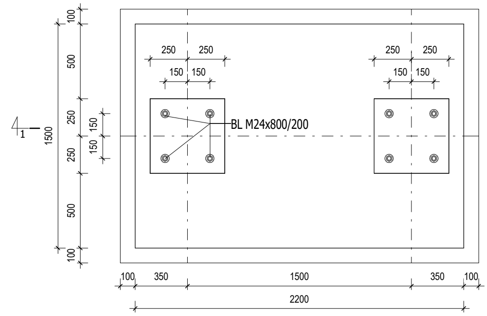
MẶT BẰNG MÓNG TỶ LỆ: 1 : 25
