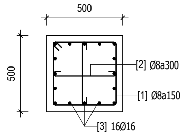
MẶT CẮT 2-2 TỶ LỆ: 1 : 25
