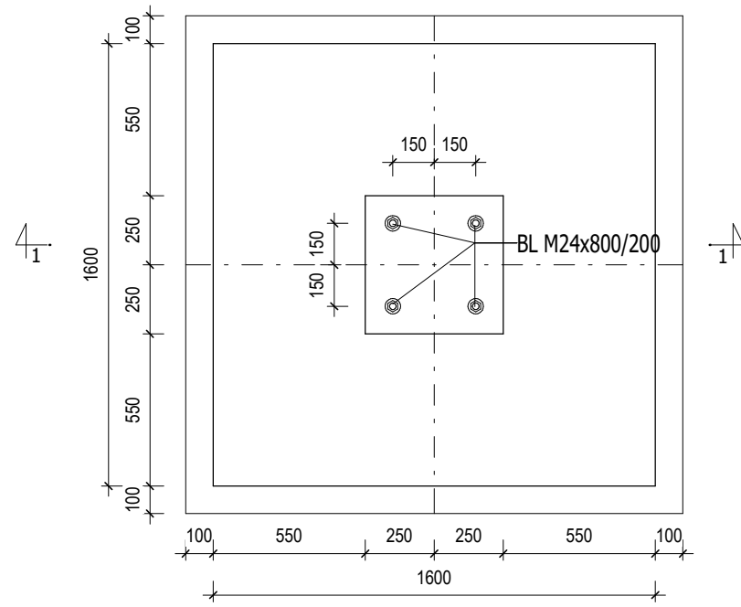
MẶT BẰNG MÓNG TỶ LỆ: 1:25
