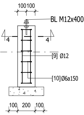
MẶT CẮT 5-5
