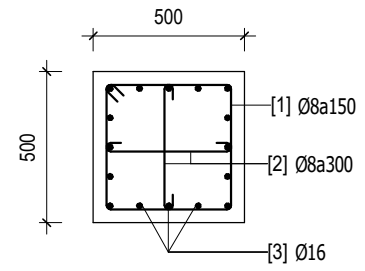
MẶT CẮT 2-2 TỶ LỆ: 1:25
