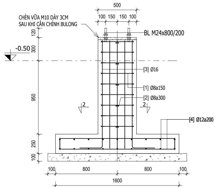
MẶT CẮT 1-1 TỶ LỆ: 1:25
