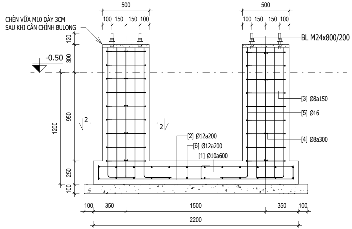
MẶT CẮT 1-1 TỶ LỆ: 1 : 25
