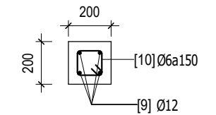
MẶT CẮT 4-4
