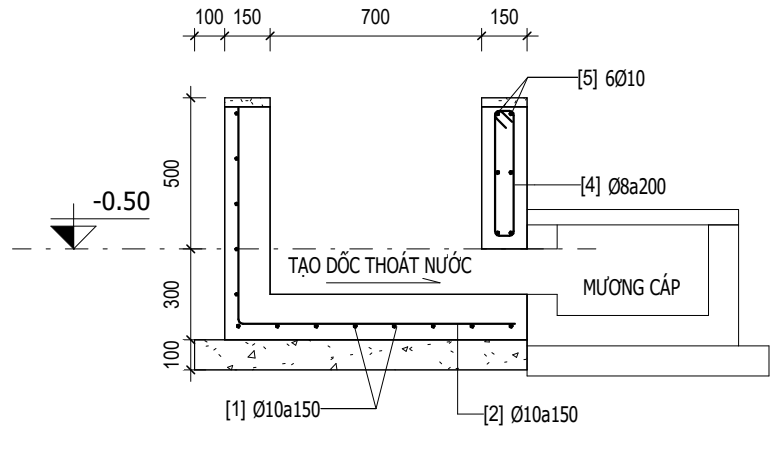
MẶT CẮT 2-2 TỶ LỆ: 1 : 25
