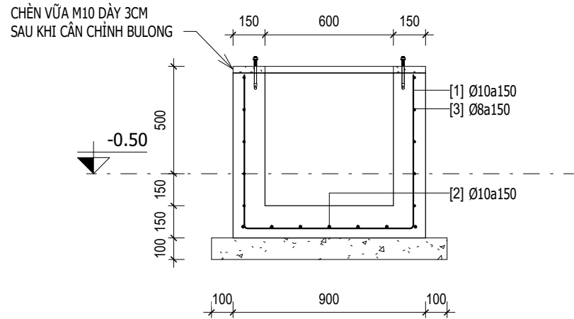
MẶT CẮT 1-1 TỶ LỆ: 1 : 25
