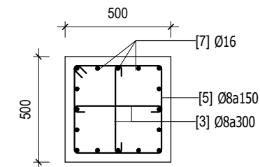
MẶT CẮT 2-2
