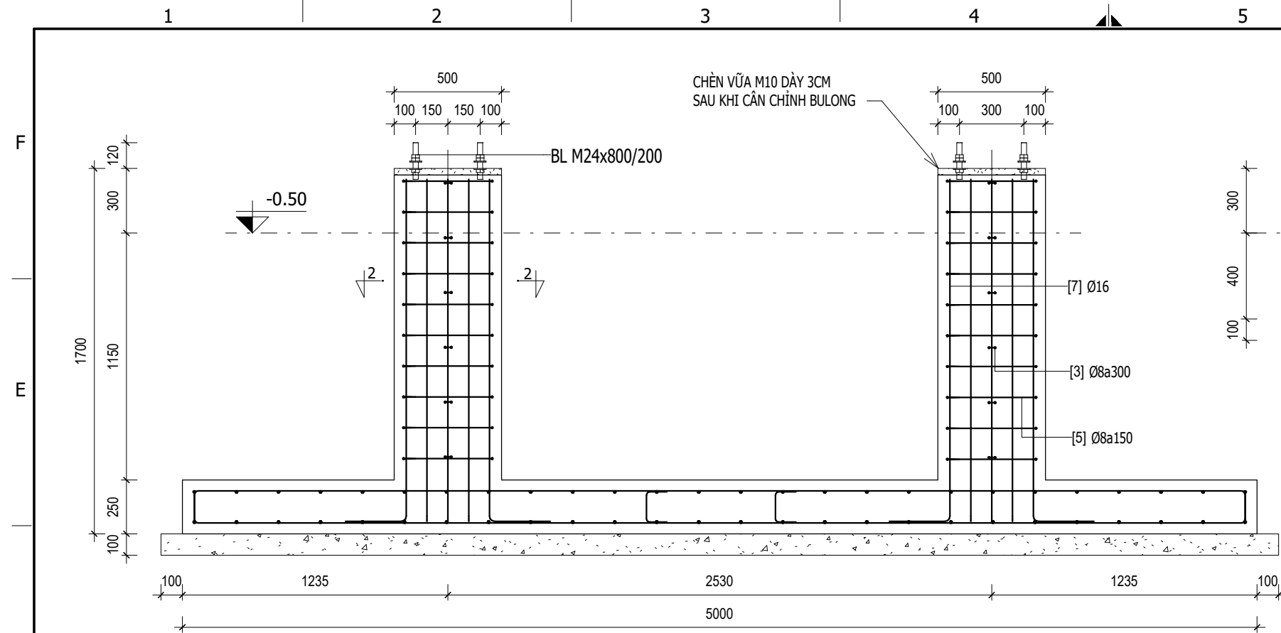
MẶT CẮT 1-1
