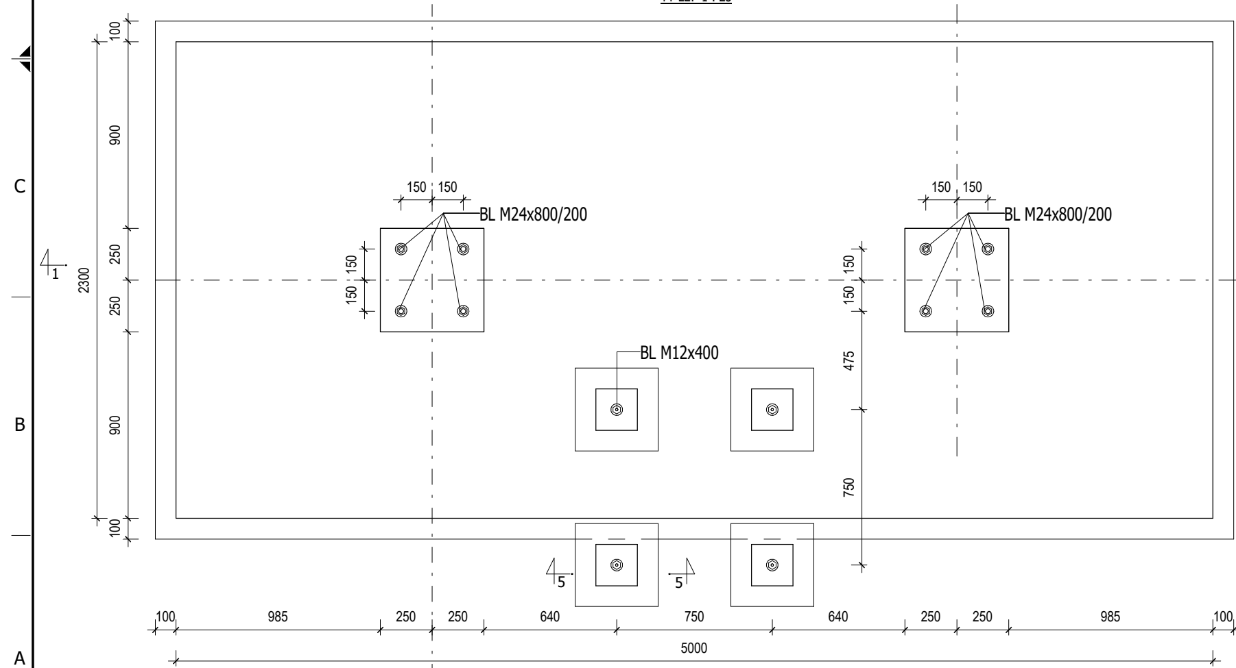
MẶT BẰNG MÓNG
