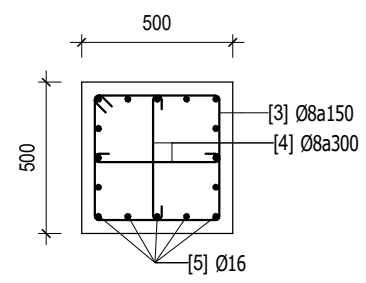
MẶT CẮT 2-2 TỶ LỆ: 1 : 25
