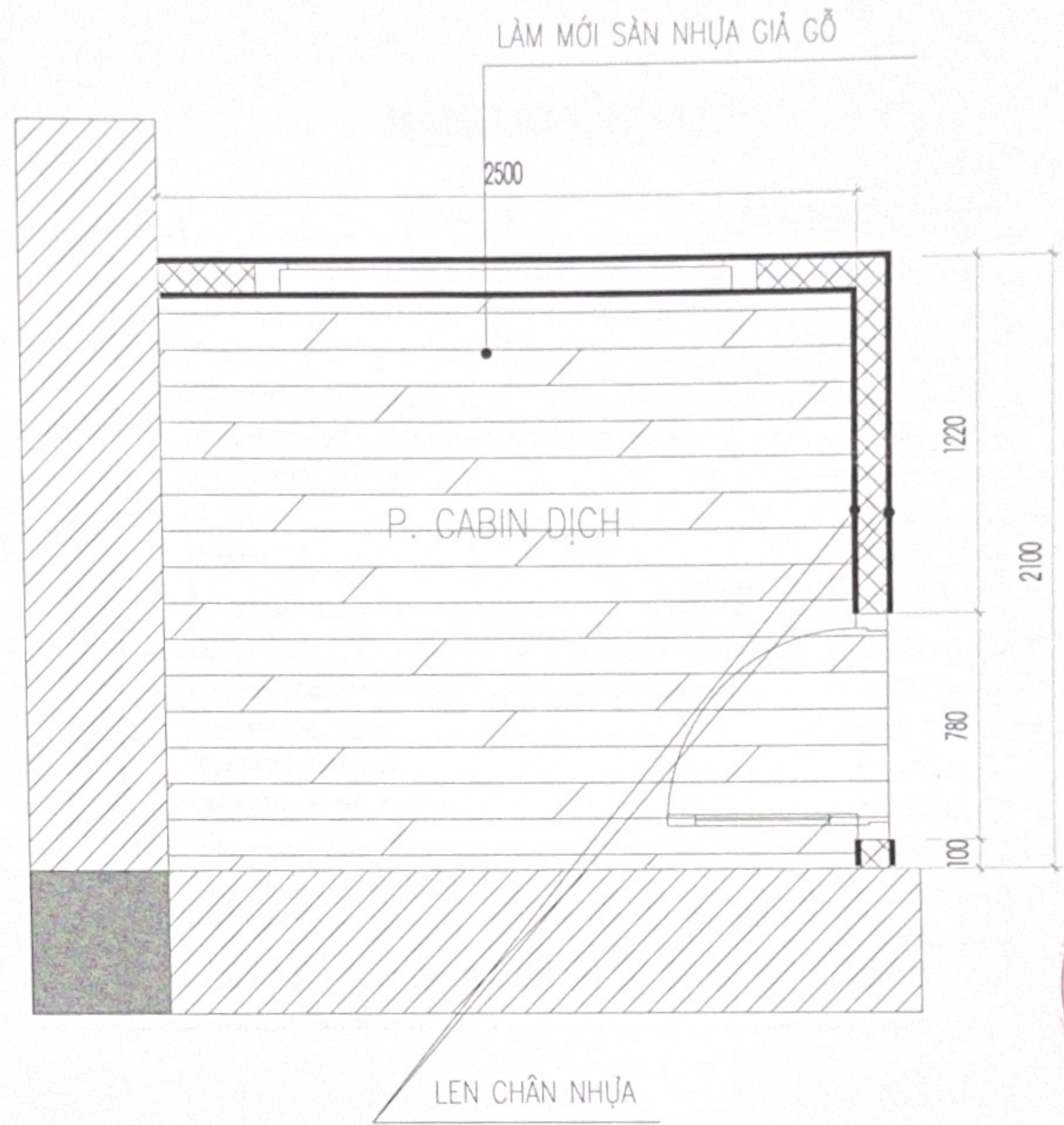
MẶT BẰNG LÁT SÀN
