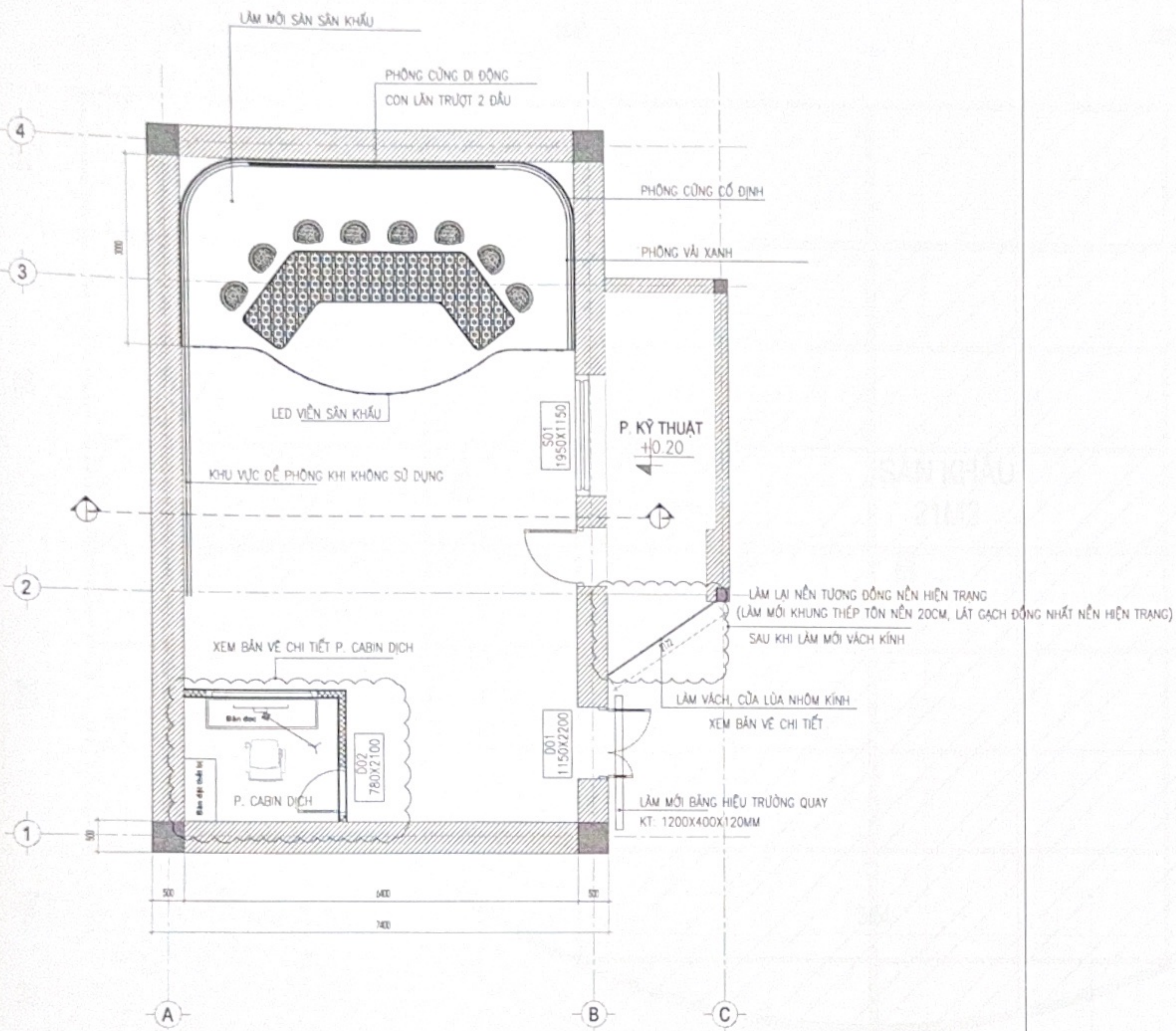
MẶT BẰNG CẢI TẠO
