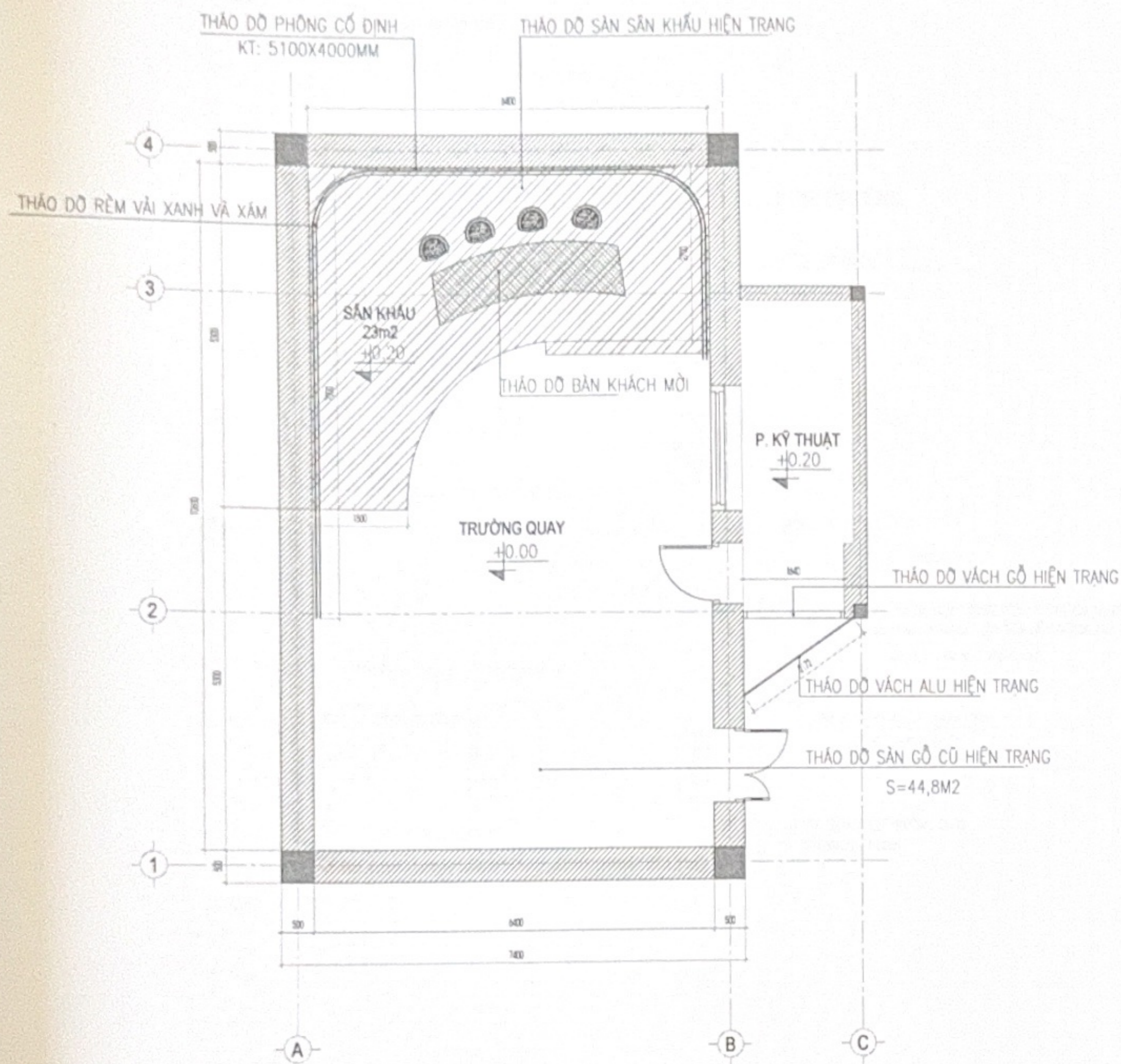
MẶT BẰNG THẢO ĐỒ
