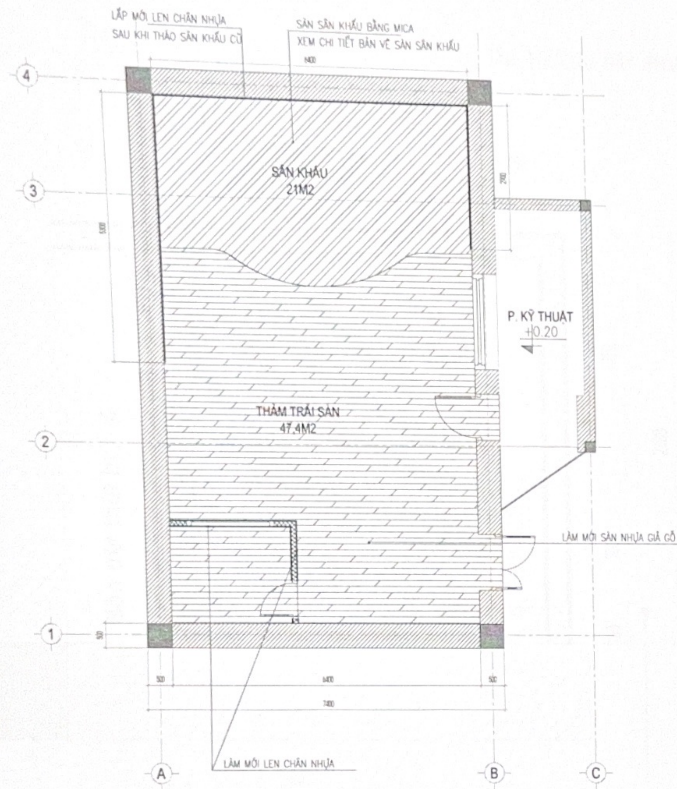
MẶT BẰNG CẢI TẠO SÀN
