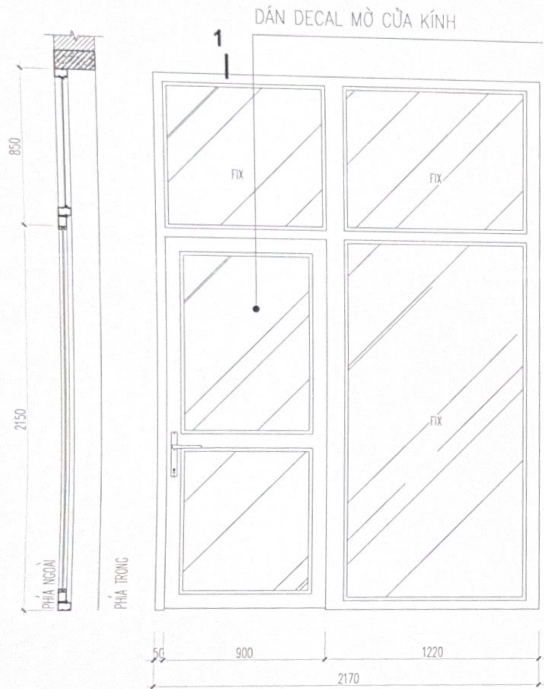
CHI TIẾT VÁCH KÍNH P KỸ THUẬT
