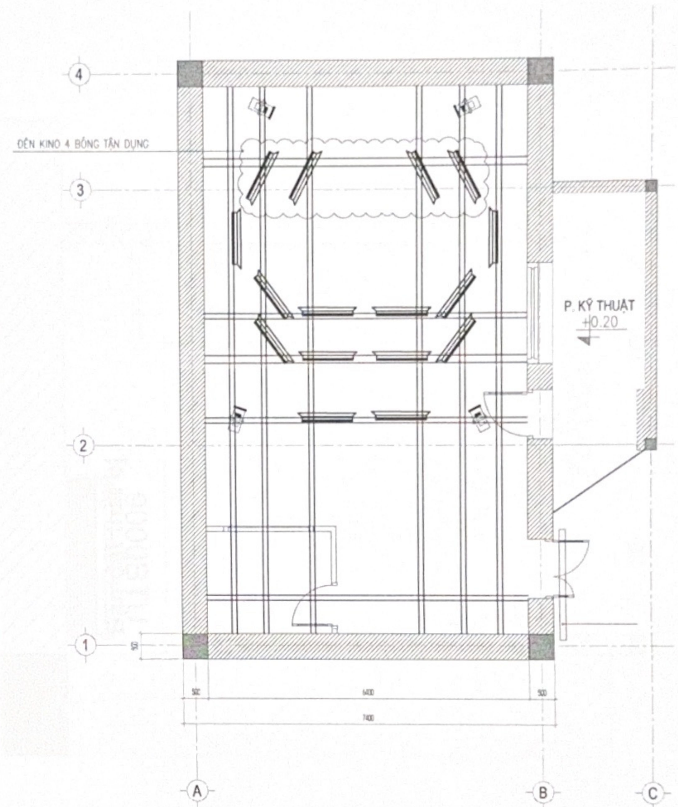
MẶT BẰNG CẢI TẠO CHIẾU SÁNG
