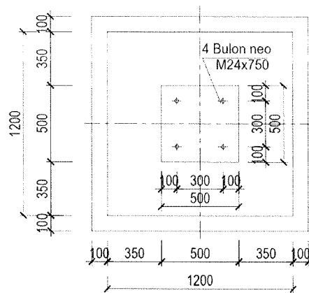
MẶT BẰNG
