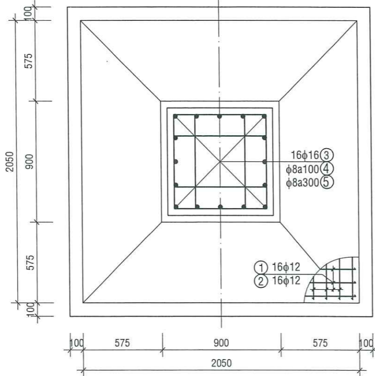
MÓNG TRỤ LÁ NHỎ TL:1/ 25; SL=06
