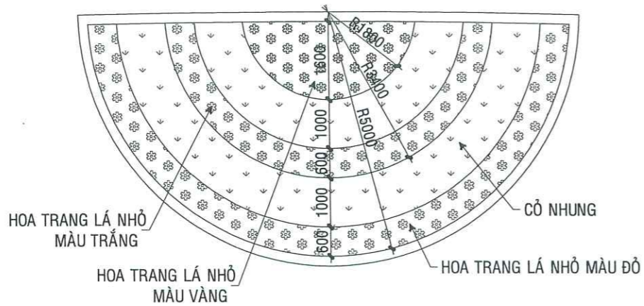
MẶT BẰNG TRỒNG HOA (BỒN 3)
