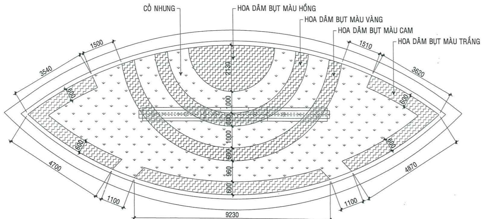
MẶT BẰNG TRỒNG HOA (BỒN 2)
