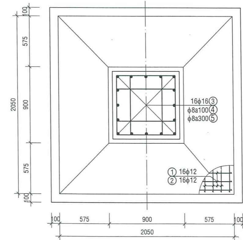
MÓNG TRỤ LÁ SEN NHỎ TL:1/ 25; SL=04
