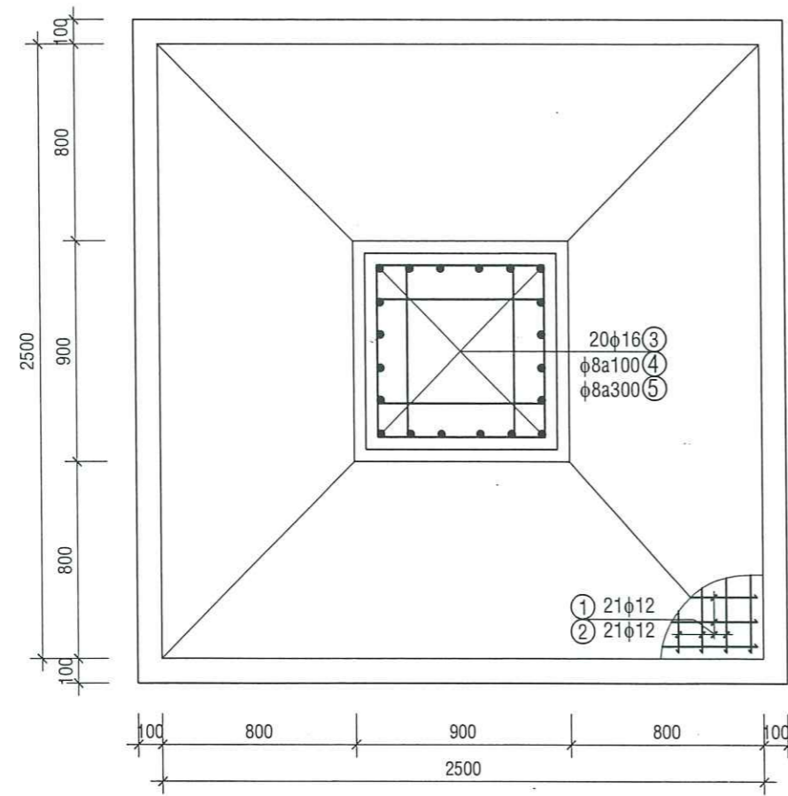
MÓNG TRỤ LÁ SEN LỚN TL:1/ 25; SL=03
