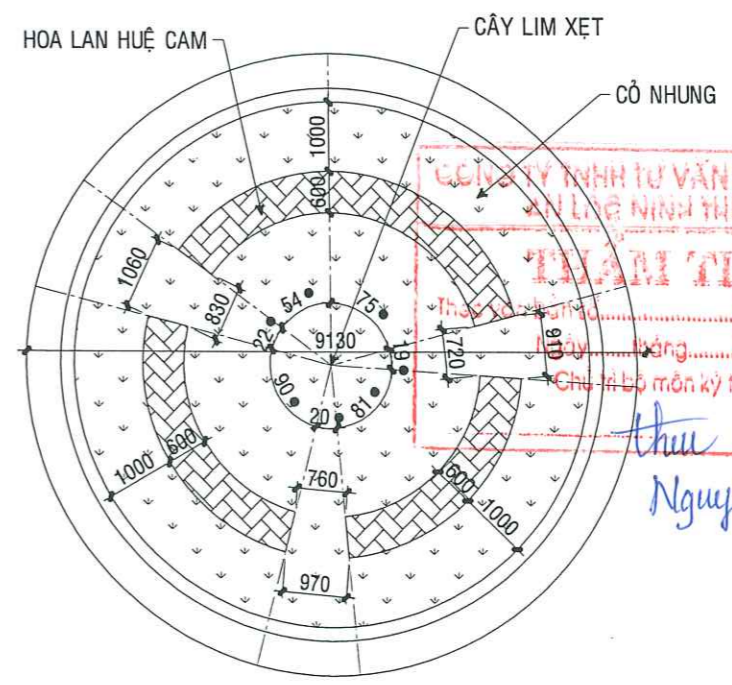
MẶT BẰNG TRỒNG HOA (BỒN 6) TL 1/100
