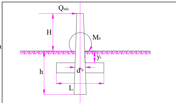
Móng chôn sâu đặt 1 thanh ngang
