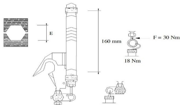
Hình 2.5 Kẹp đầu rãnh
