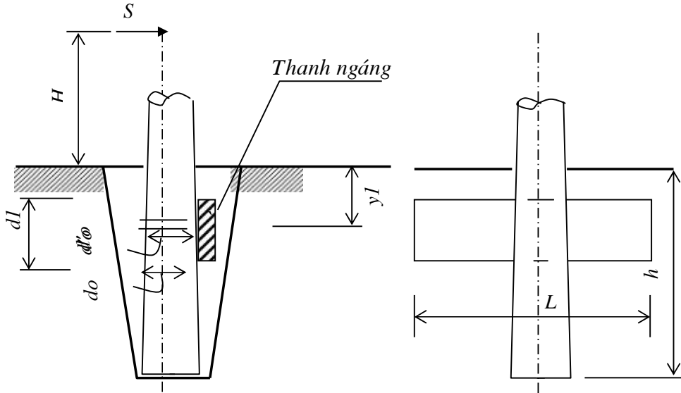
Móng chôn sâu đặt 1 thanh ngang
