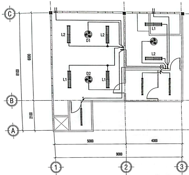
MẶT BẰNG CHIẾU SÁNG BẾP LẦU 2 TL: 1/100
