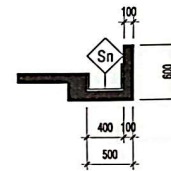
CHI TIẾT SÊ NÔ TL: 1/50
