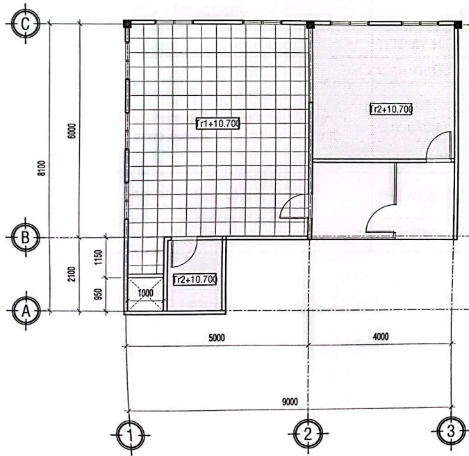
MẶT BẰNG TRẦN BẾP LẦU 2 TL: 1/100
