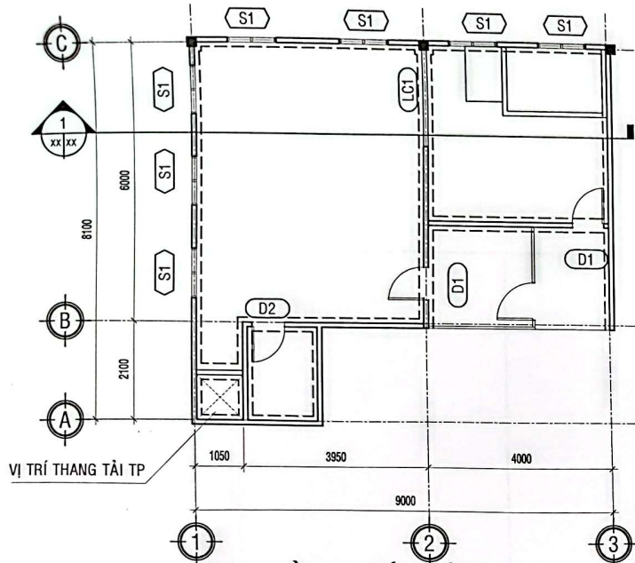
MẶT BẰNG BẾP LẦU 2 TL: 1/100
