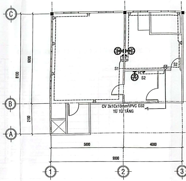
MẶT BẰNG CẤP NGUỒN BẾP LẦU 2 TL: 1/100
