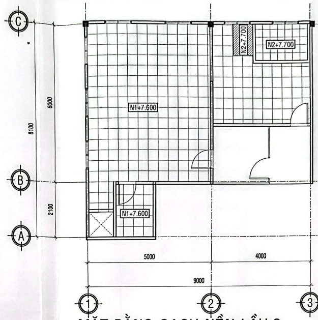
MẶT BẰNG GẠCH NỀN LẦU 2 TL: 1/100
