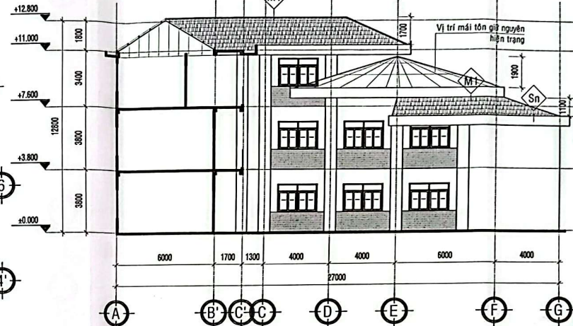
MẶT ĐỨNG TL: 1/200
