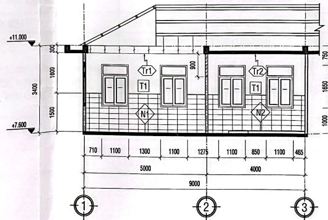
MẶT CẮT 1-1 TL: 1/100
