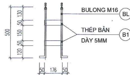
CHI TIẾT BU LÔNG NEO M16
