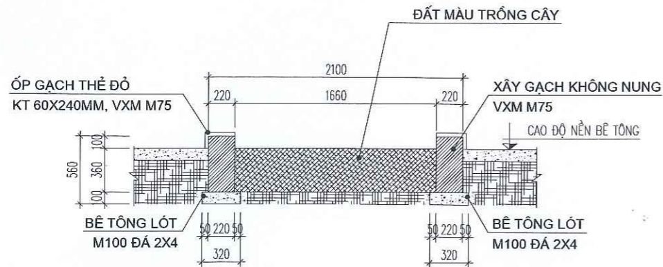
MẶT CẮT 1-1
