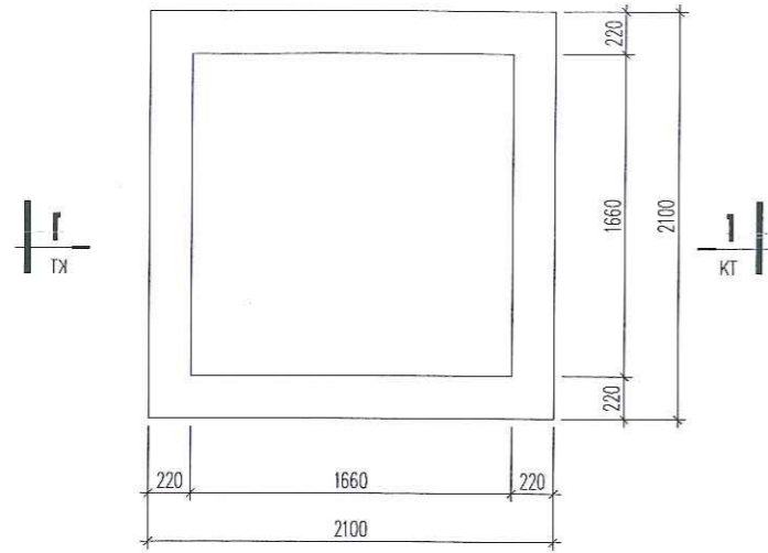
MẶT BẰNG BỒN CÂY 02
