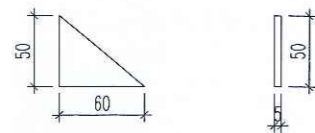
CHI TIẾT THÉP GIA CƯỜNG
