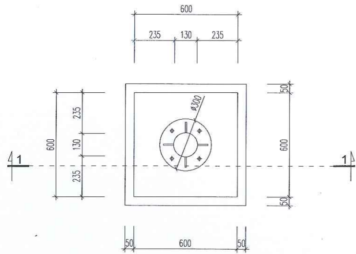
MẶT BẰNG MÓNG M1
