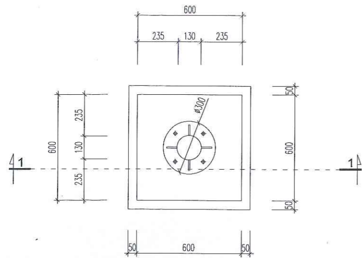
MẶT BẰNG MÓNG M1; M2
