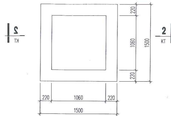
MẶT BẰNG BỒN CÂY 01
