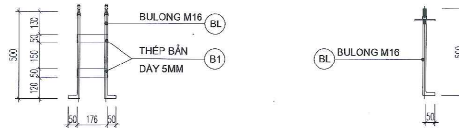
CHI TIẾT BU LÔNG NEO M16
