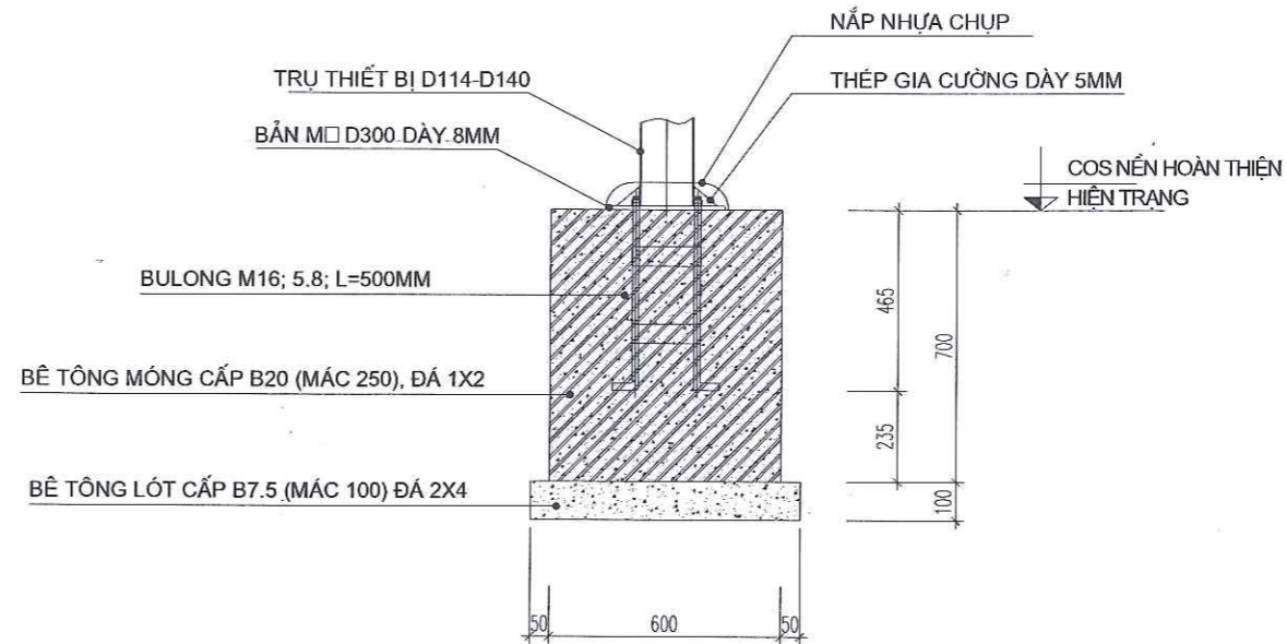
MẶT CẮT 1-1
