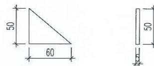
CHI TIẾT THÉP GIA CƯỜNG
