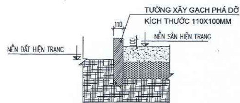
CHI TIẾT TƯỜNG BỐ PHÁ DỠ
