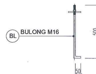
CHI TIẾT BU LÔNG NEO M16
