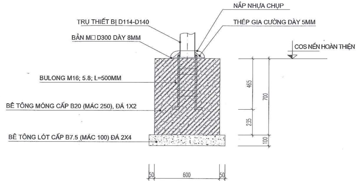
MẶT CẮT 1-1
