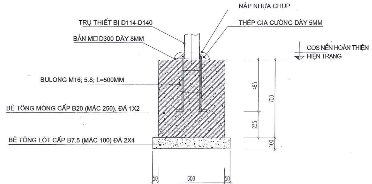
MẶT CẮT 1-1
