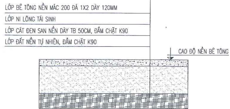
KẾT CẤU NỀN BÊ TÔNG
