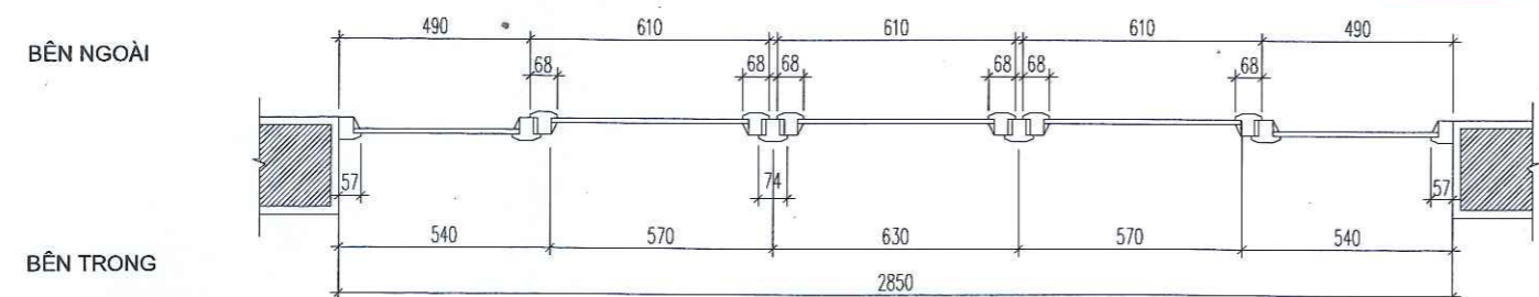
MẶT CẮT 1-1
