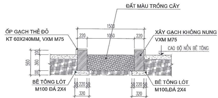
MẶT CẮT 2-2
