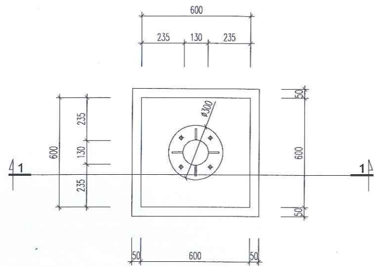
MẶT BẰNG MÓNG M1 (SỐ LƯỢNG: 16 CẤU KIỆN)
