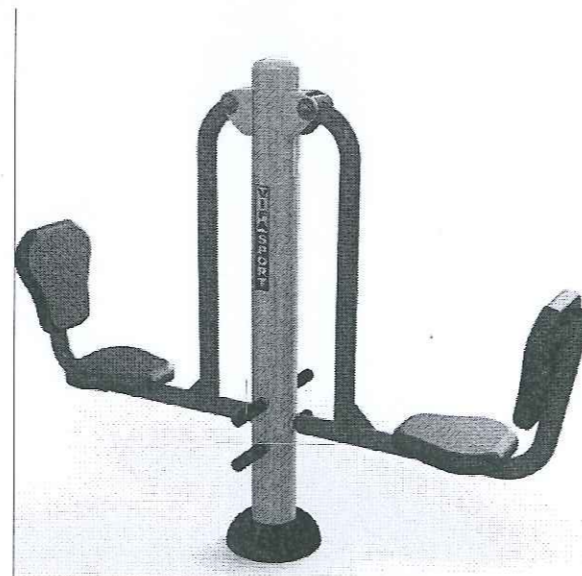
TB5: THIẾT BỊ 05 (MÁY TẬP ĐẠP CHÂN) (SỐ LƯỢNG: 01 CẤU KIỆN)
