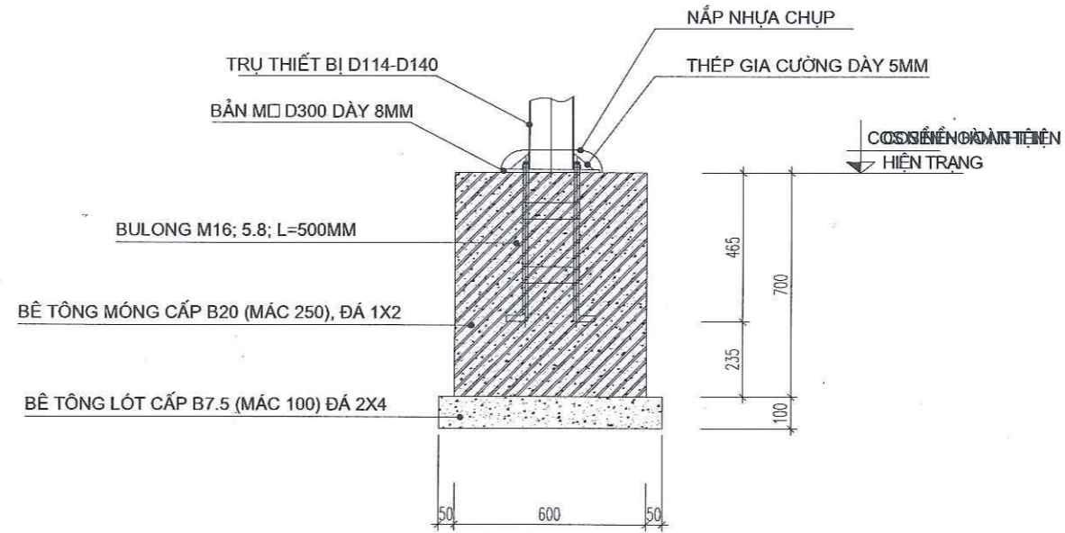
MẶT CẮT 1-1
