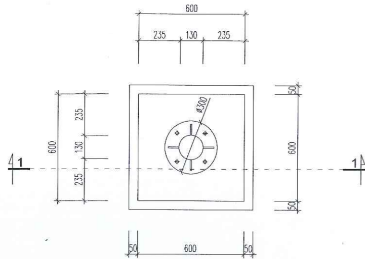
MẶT BẰNG MÓNG M1 (SỐ LƯỢNG: 10 CẤU KIỆN)
