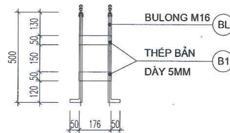
CHI TIẾT BU LÔNG NEO M16
