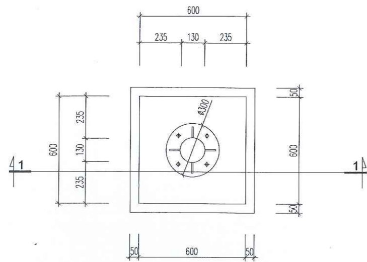
MẶT BẰNG MÓNG M1 (SỐ LƯỢNG: 11 CẤU KIỆN)
