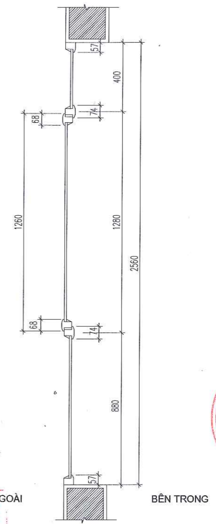
MẶT CẮT 2-2
