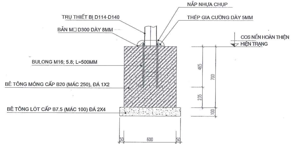
MẶT CẮT 1-1
