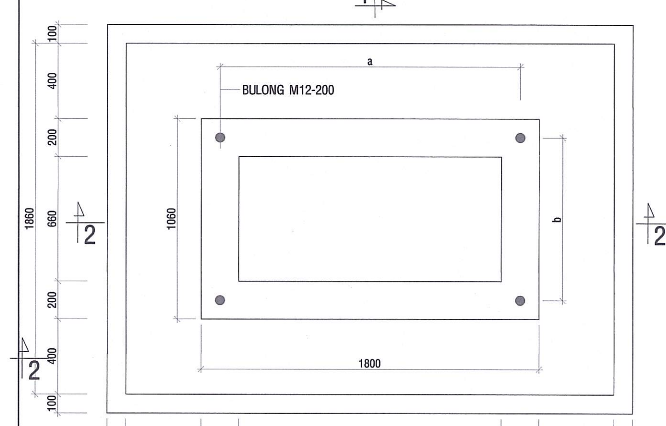
MẶT BẰNG BỐ TRÍ THÉP; TL : 1/20
