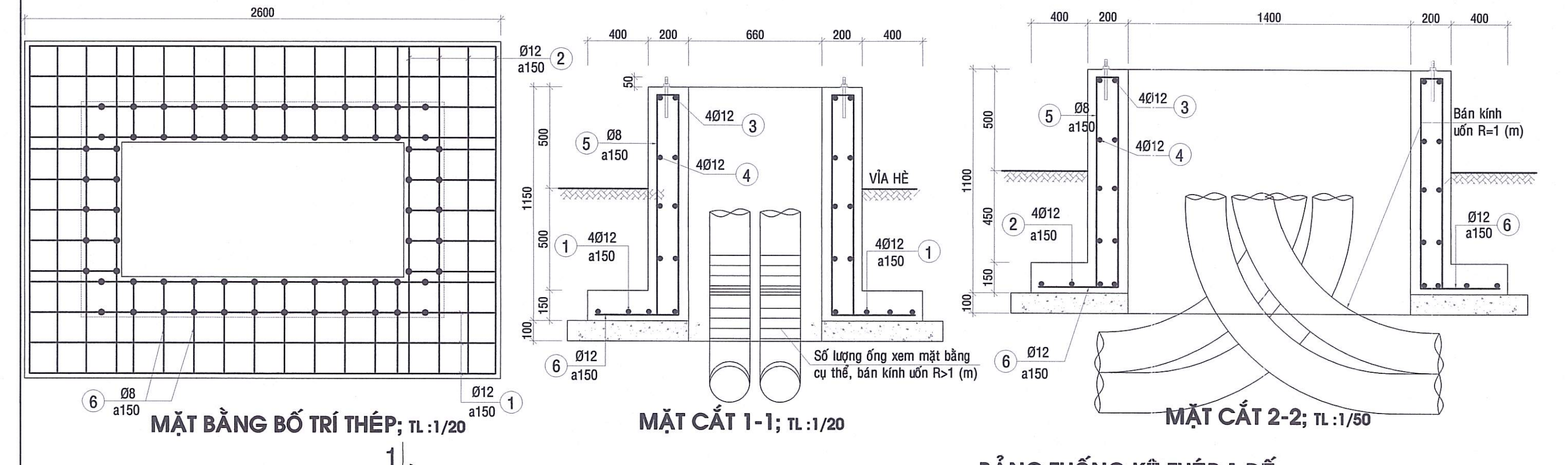
MẶT BẰNG BỐ TRÍ THÉP; TL : 1/20
