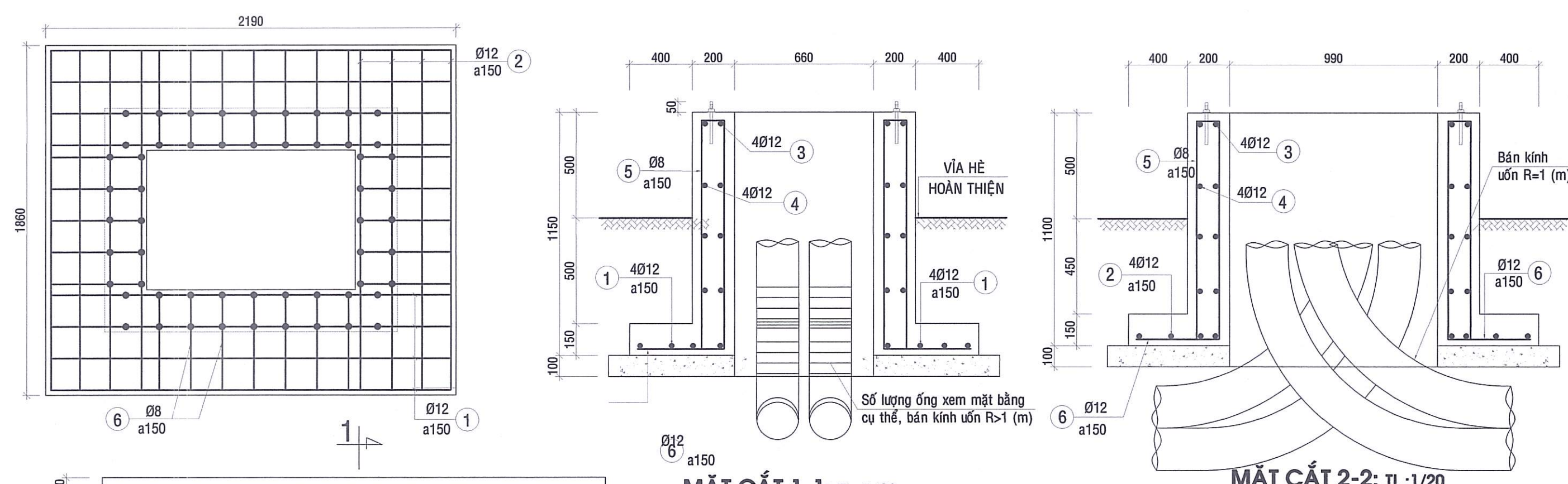
MẶT CẮT 1-1; TL : 1/20
