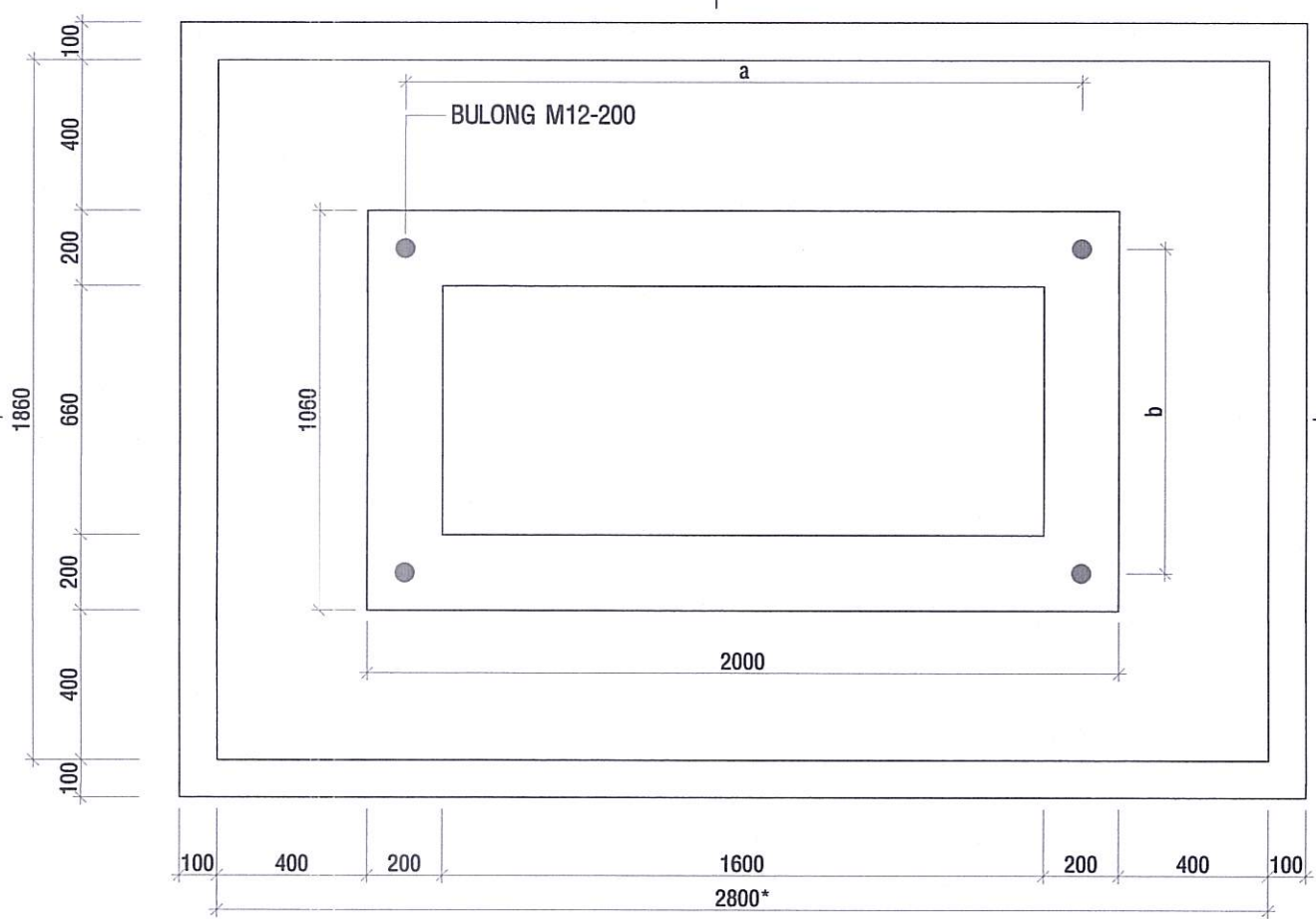
MẶT BẰNG ĐỂ; TL : 1/20
