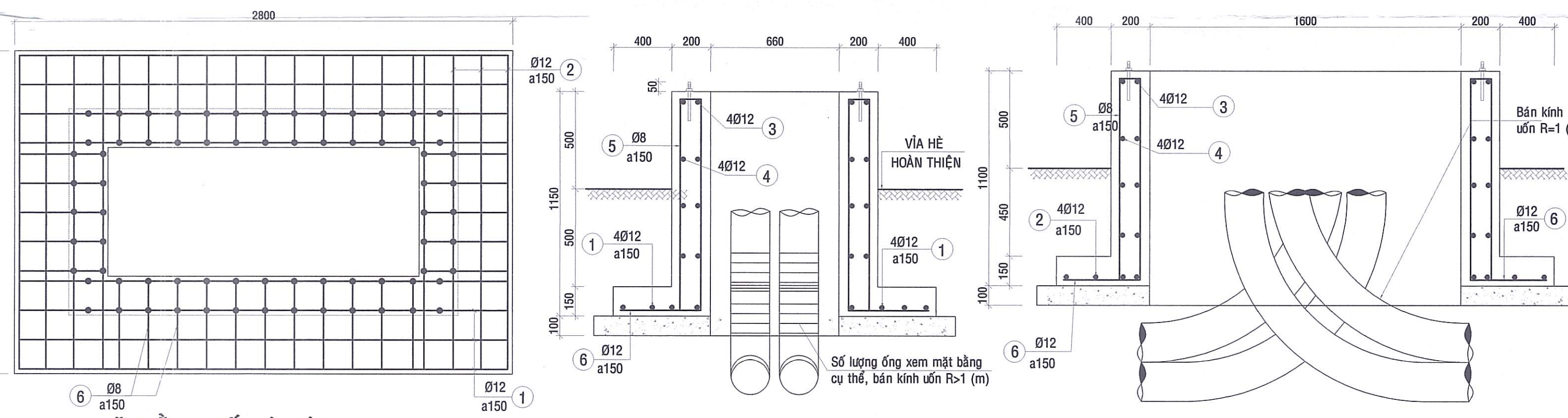
MẶT BẰNG BỐ TRÍ THÉP; TL : 1/20
