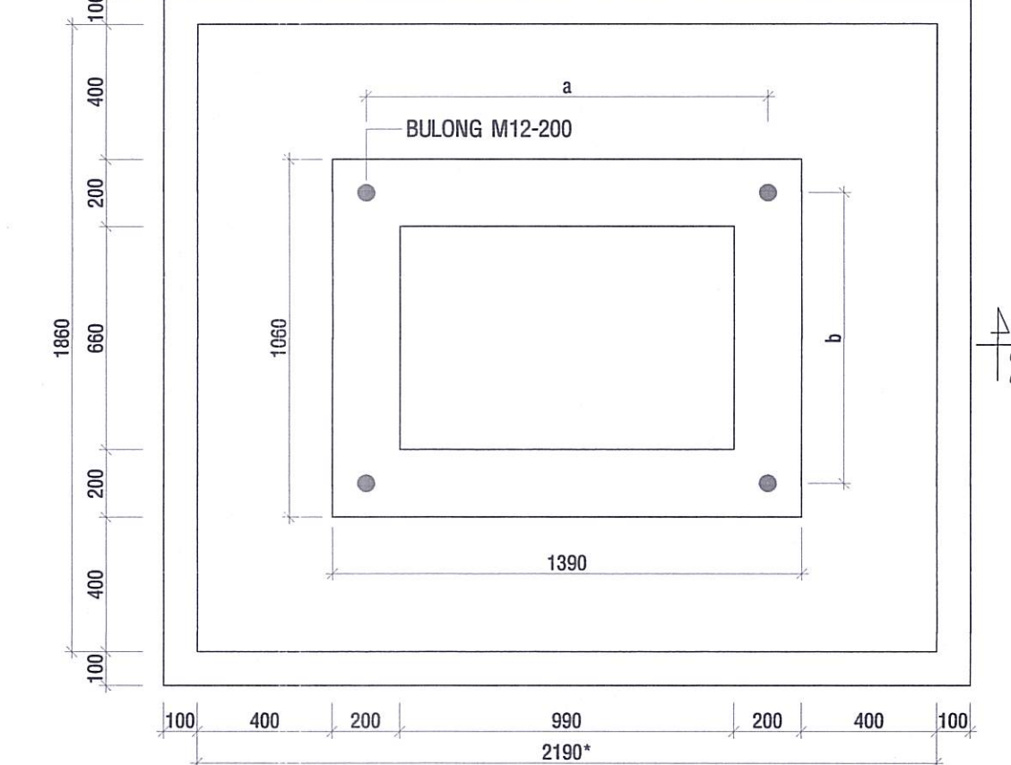
MẶT BẰNG ĐỂ; TL : 1/20
