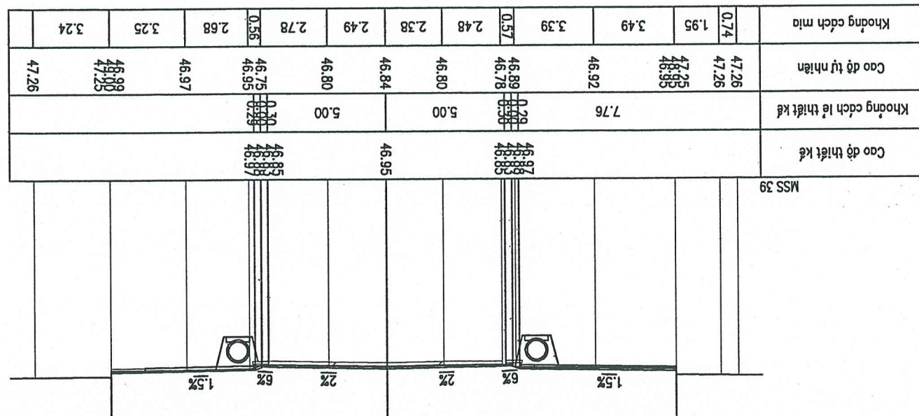
Cọc C28 Km 0 + 414.96
