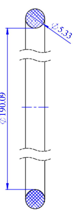
O-ring CS5.33xID190.09
