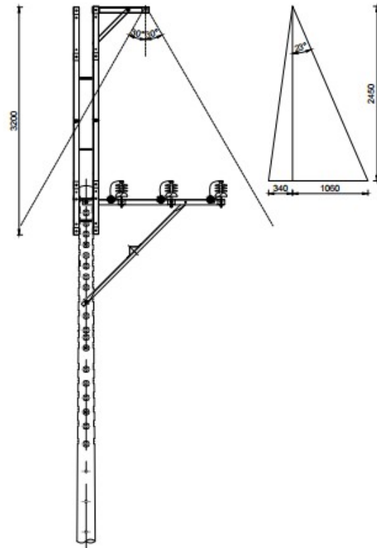
Mẫu đầu trụ CS-02A
