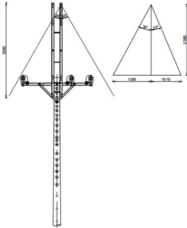
Mẫu đầu trụ CS-02
