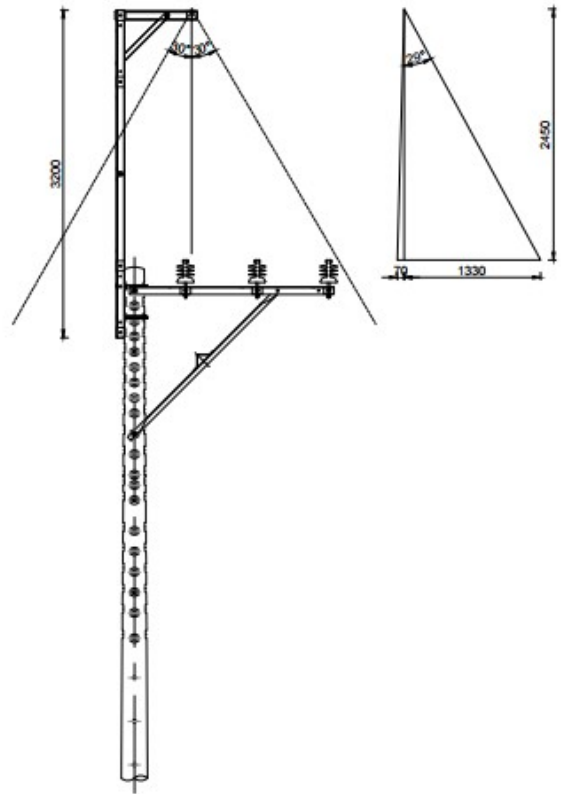
Mẫu đầu trụ CS-01A
