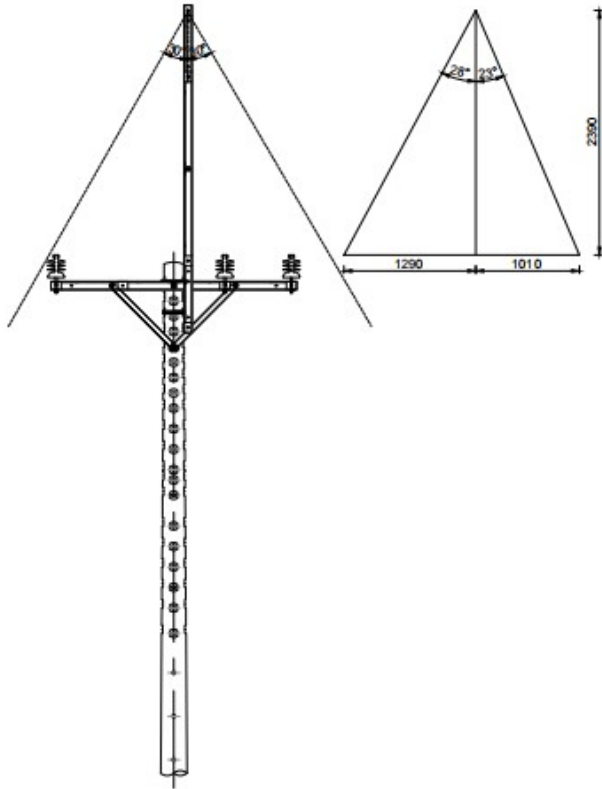
Mẫu đầu trụ CS-01
