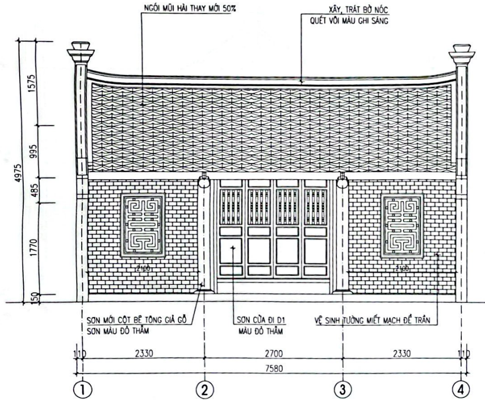
MẶT ĐỨNG TRỰC 1-4
