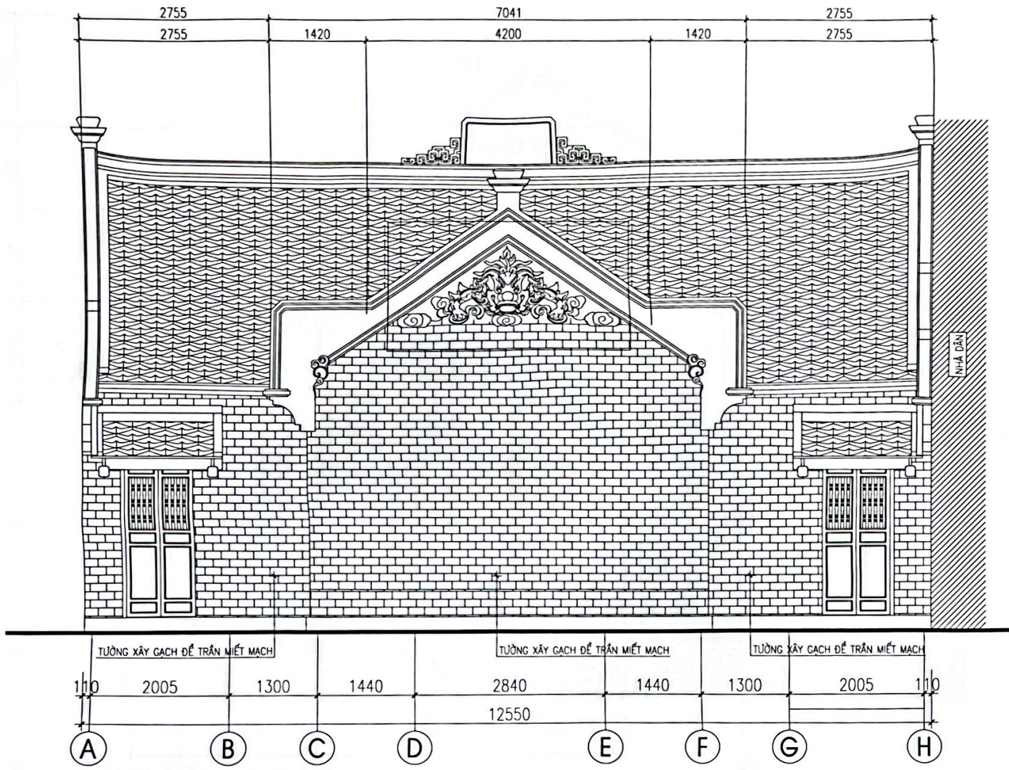
MẶT ĐỨNG TRỰC A-H ĐẾN CHÍNH
