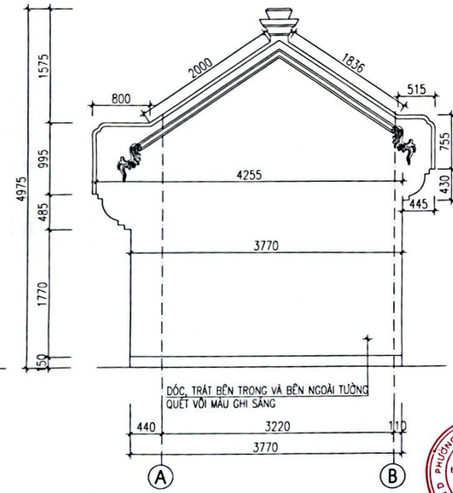
MẶT ĐỨNG TRỰC A-B
