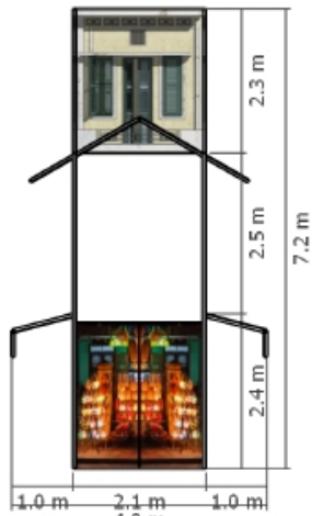
MẶT BÊN PHẢI TỔNG THỂ
