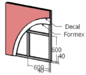
CẤU TẠO VÁCH KHUNG SẮT - FORMEX - DECAL
