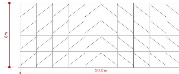
LAYER TRUSS LED CHÍNH - LỚP 2
