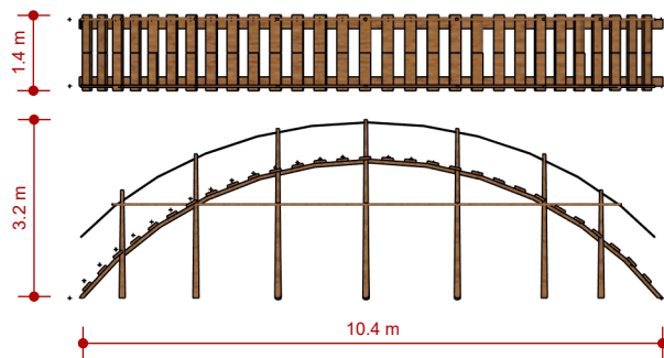
MÔ HÌNH CẦU GỖ
