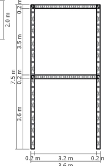
KHUNG GIÀN TRUSS
