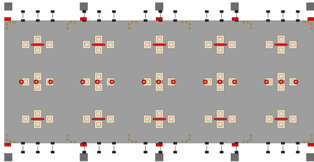
MẶT BẰNG BỤC, VÒM TRANG TRÍ, ĐÈN PHA
