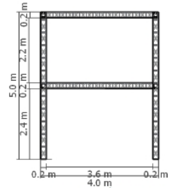
KHUNG GIÀN TRUSS
