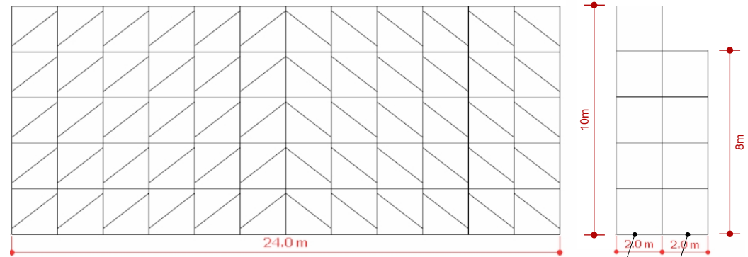
LAYER TRUSS LED CHÍNH - LỚP 1
