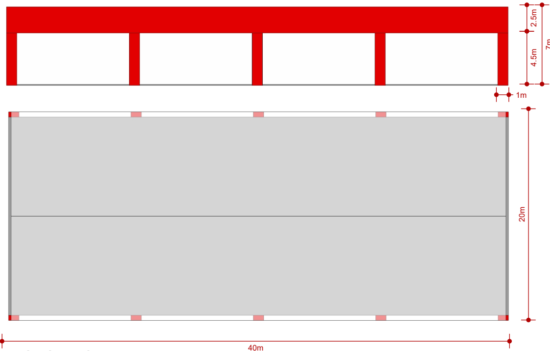
NHÀ TIỀN CHẾ
