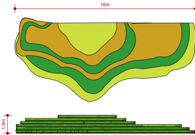
MÔ HÌNH SÀN RUỘNG BẠC THANG
