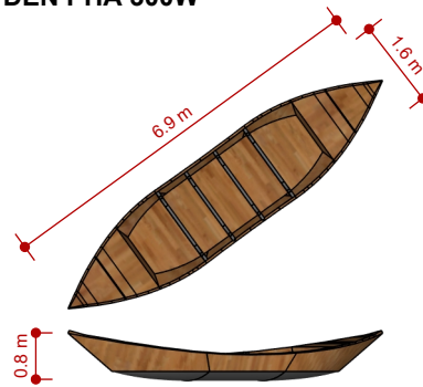
MÔ HÌNH THUYỀN
