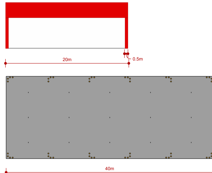
SÀN PALLET
