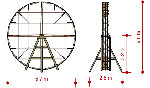
MÔ HÌNH CỌN NƯỚC
