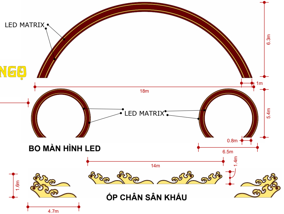
MÀN HÌNH LED
