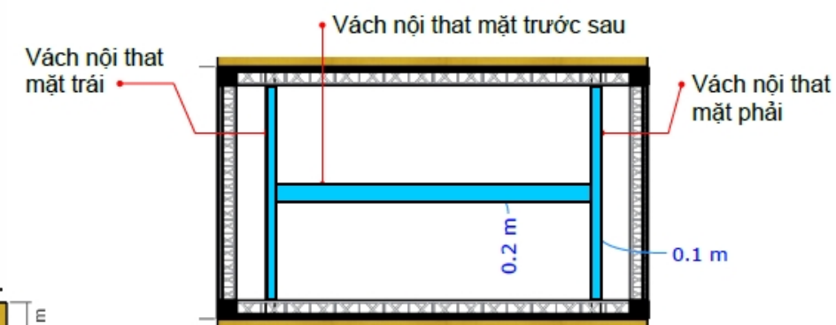
CHI TIẾT ĐỘ DÀY VÁCH NỘI THẤT
