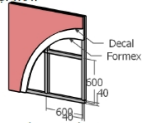
CẤU TẠO VÁCH KHUNG SẮT - FORMEX - DECAL
