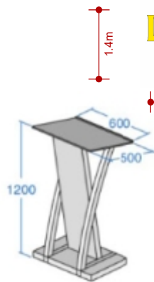
CHI TIẾT BỤC PHÁT BIỂU
