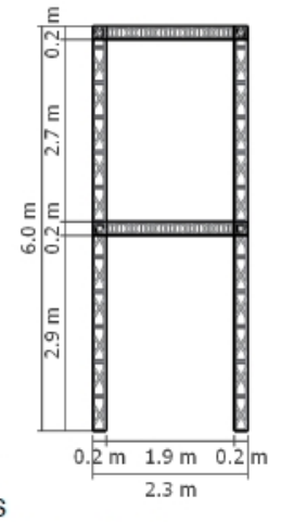
CẤU TẠO VÁCH KHUNG SẮT - FORMEX - DECAL
