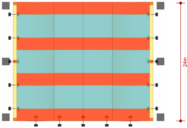
NHÀ TIỀN CHẾ
