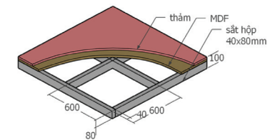
CHI TIẾT SÀN PALLET
