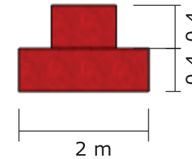
BỤC VUÔNG 2 CẤP
