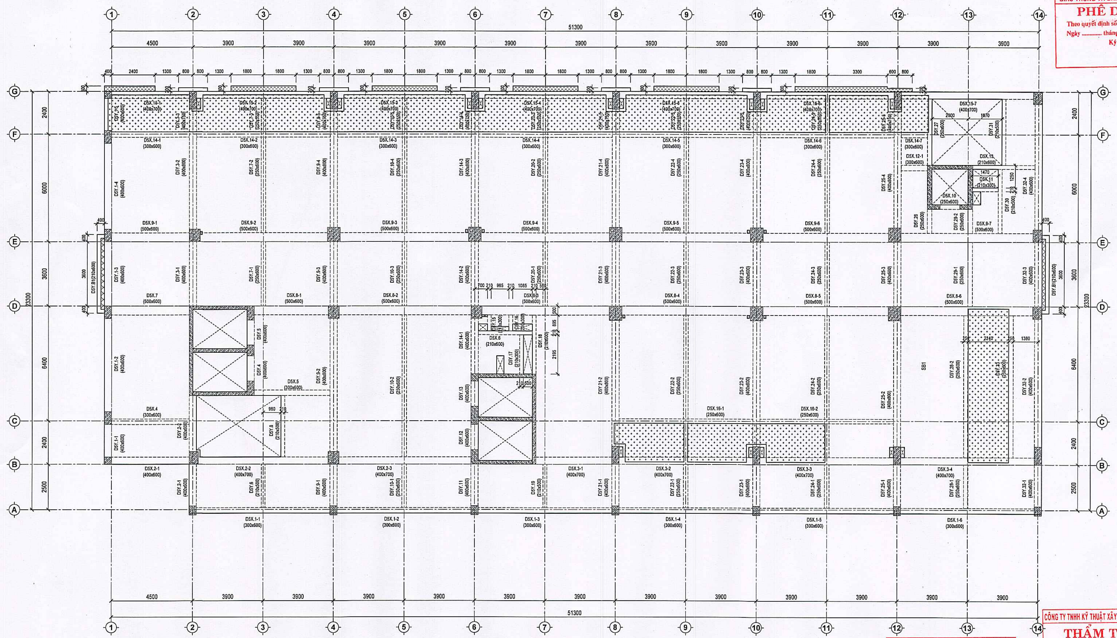
MẶT BẰNG KẾT CẤU SÀN TẦNG 5 TỶ LỆ: 1:100
