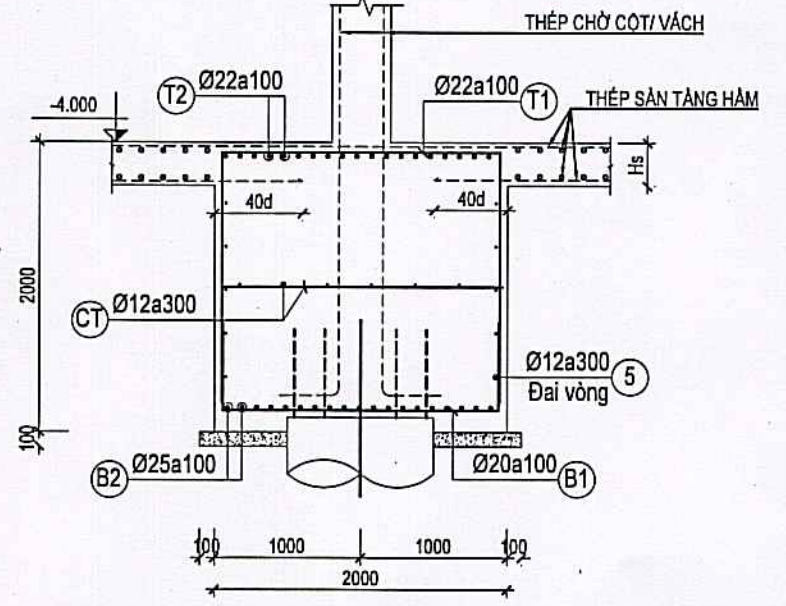
MẶT CẮT 4-4 TL: 1/50
