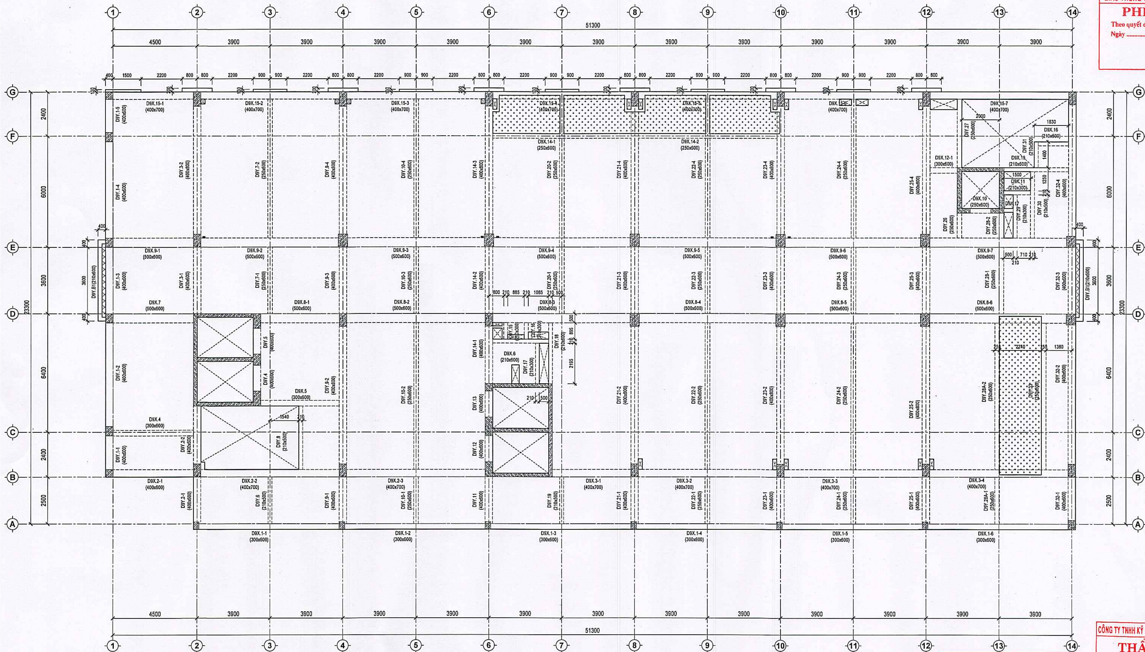
MẶT BẰNG KẾT CẤU SÀN TẦNG 9 TỶ LỆ: 1:100
