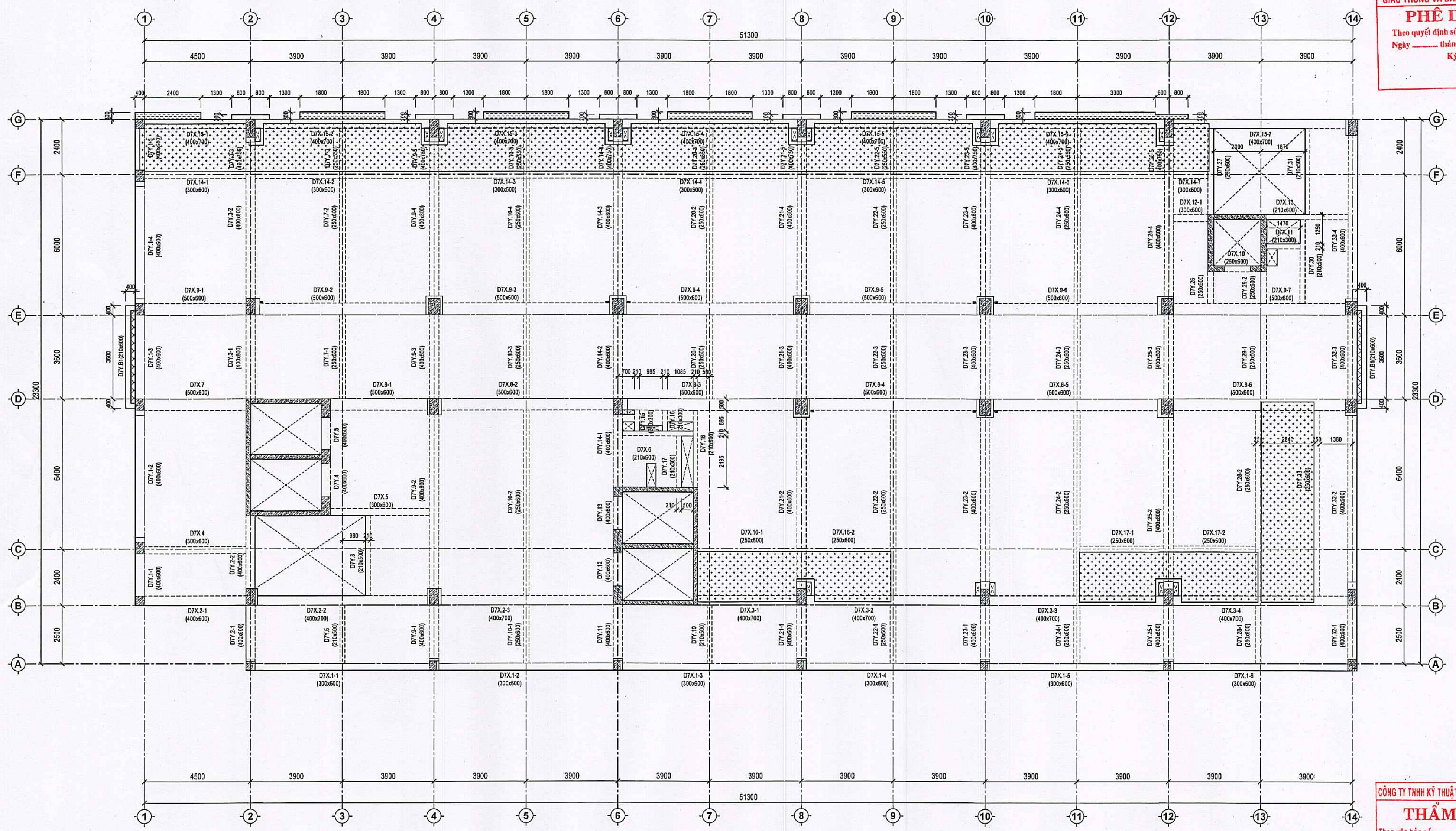
MẶT BẰNG KẾT CẤU SÀN TẦNG 7 TỶ LỆ: 1:100
