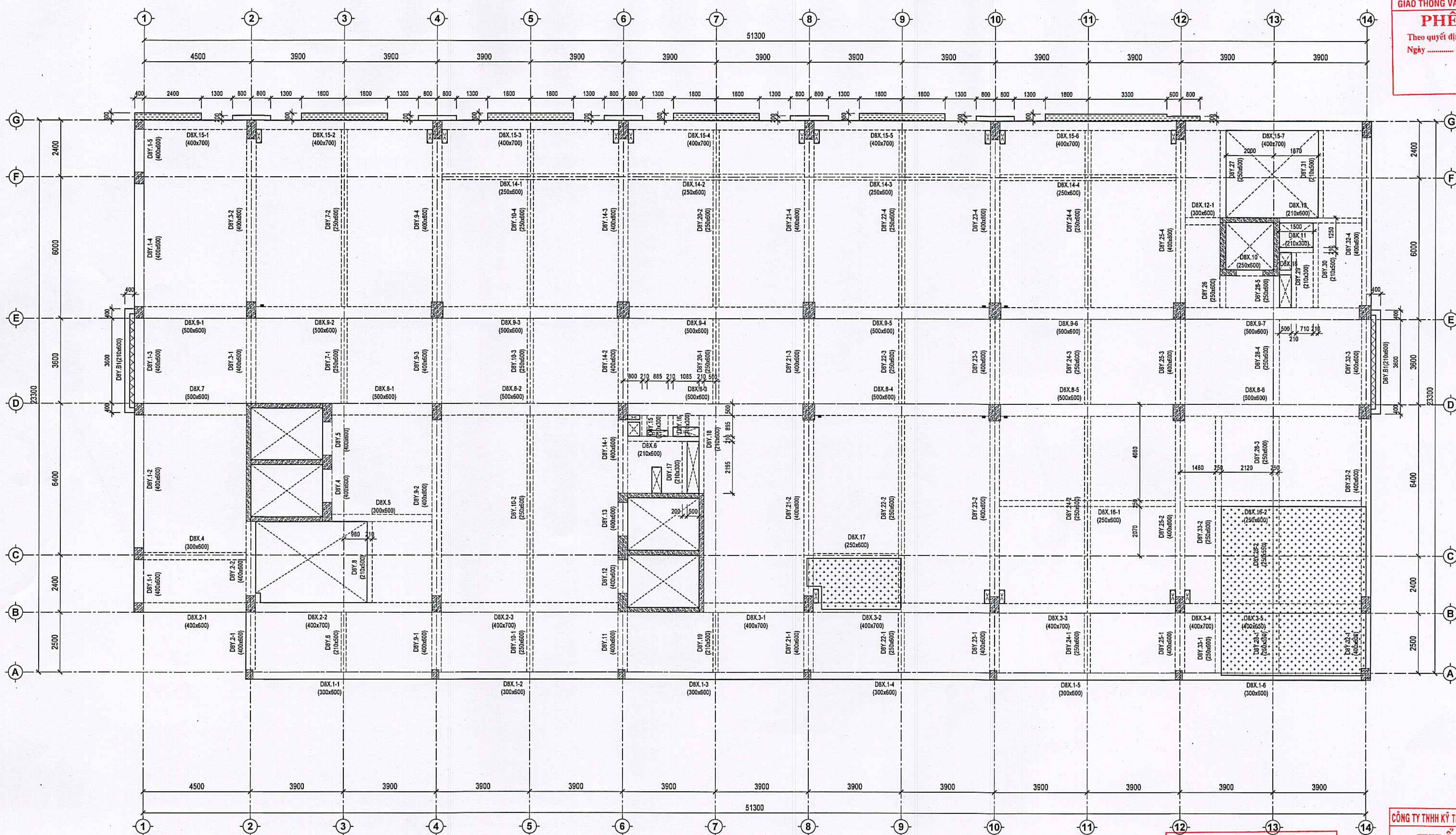
MẶT BẰNG KẾT CẤU SÀN TẦNG 8 TỶ LỆ: 1:100
