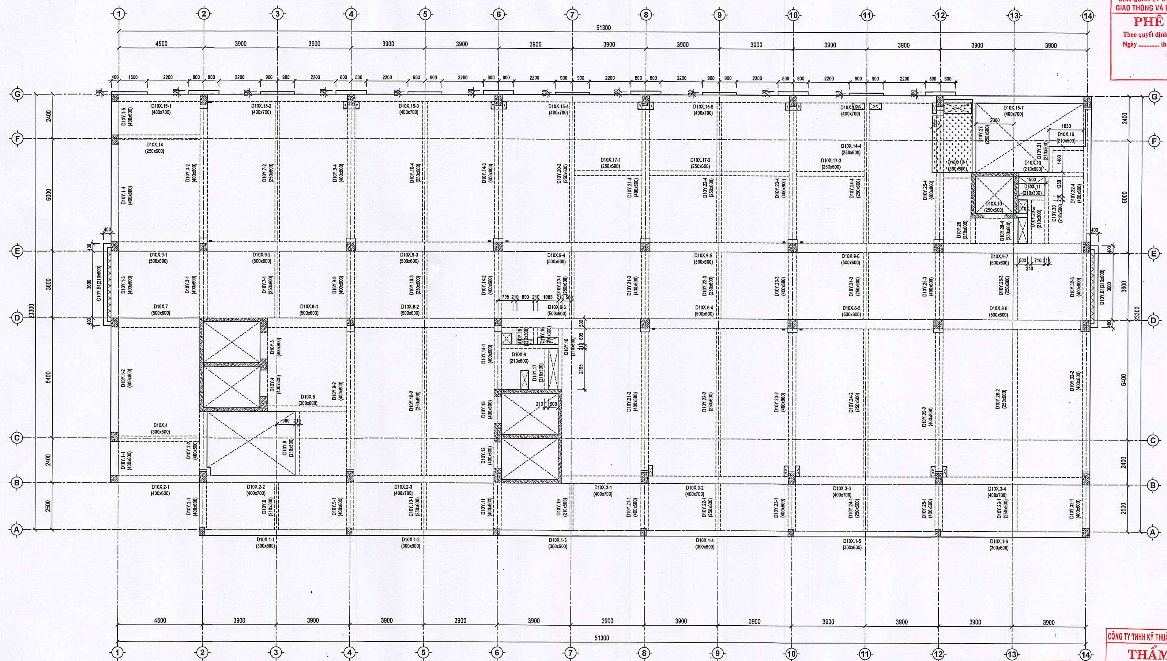
MẶT BẰNG KẾT CẤU SÀN TẦNG 10 TỶ LỆ: 1:100
