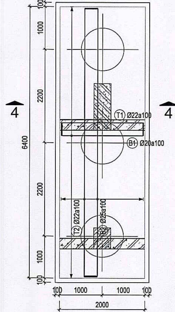
CHI TIẾT ĐÀI CỌC DC4 TL: 1/50
