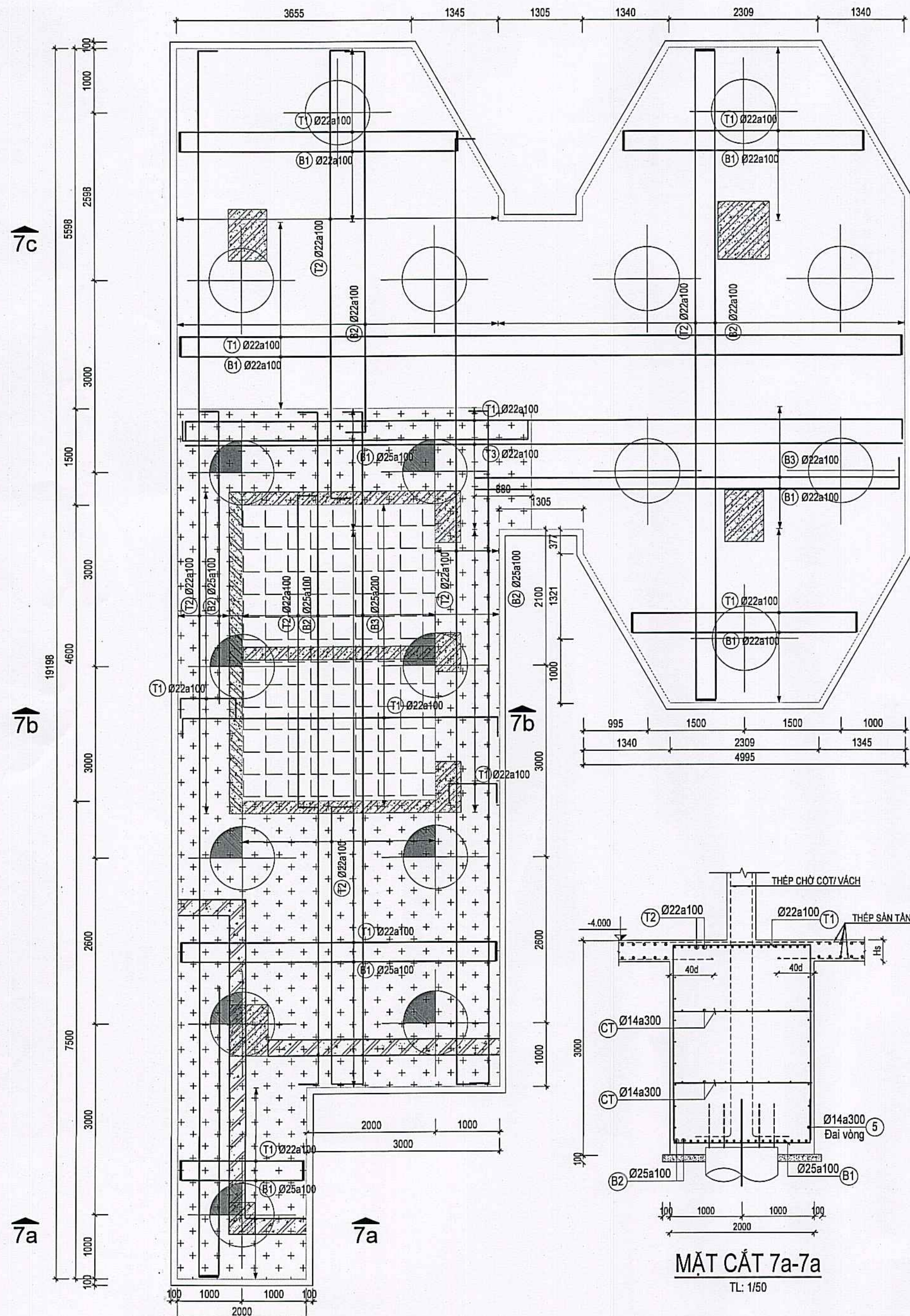
CHI TIẾT ĐÀI CỌC DC7 TL: 1/50
