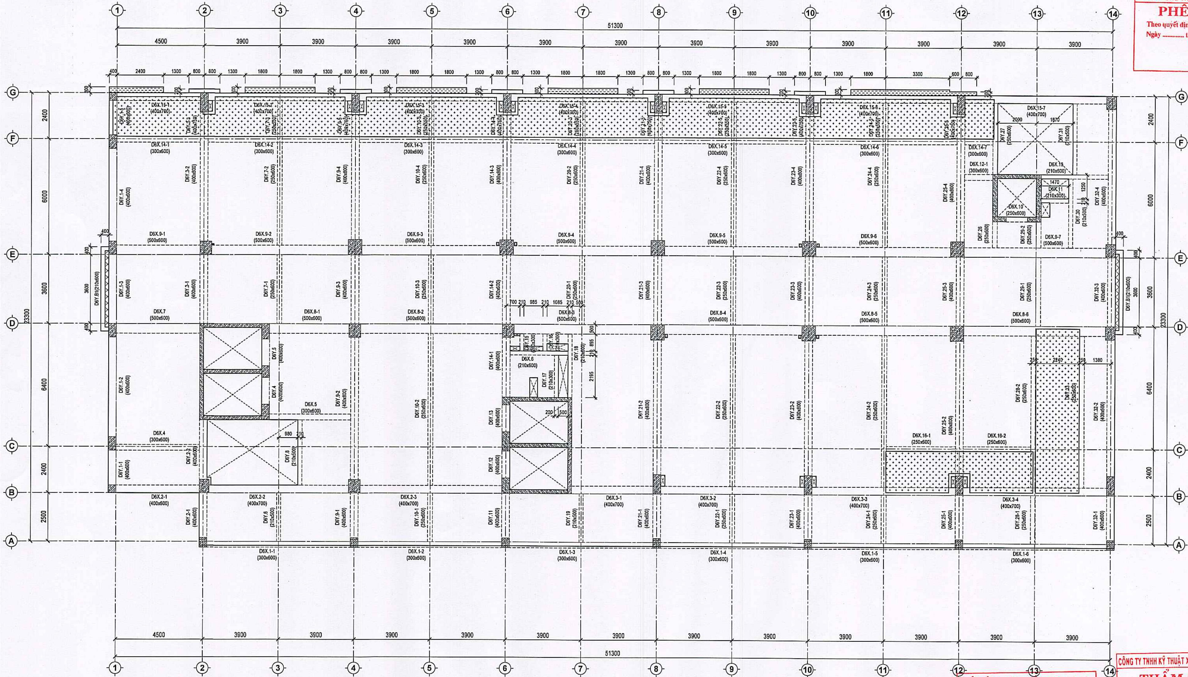
MẶT BẰNG KẾT CẤU SÀN TẦNG 6 TỶ LỆ: 1:100
