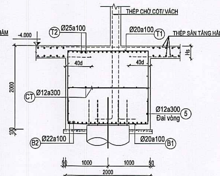
MẶT CẮT 6a-6a TL: 1/50
