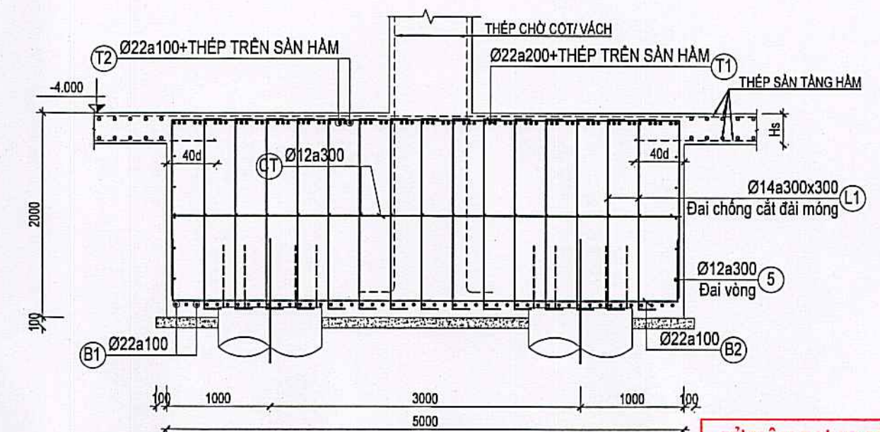
MẶT CẮT 9b-9b TL: 1/50
