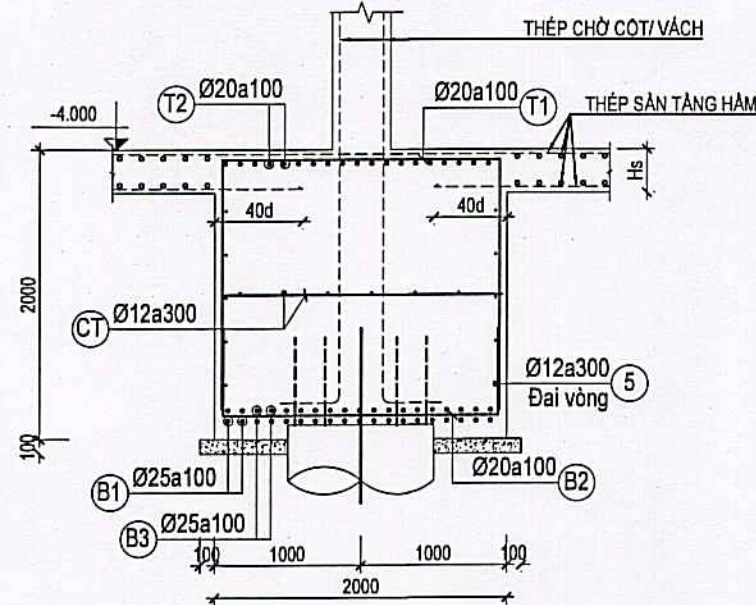
MẶT CẮT 1-1 TL: 1/50
