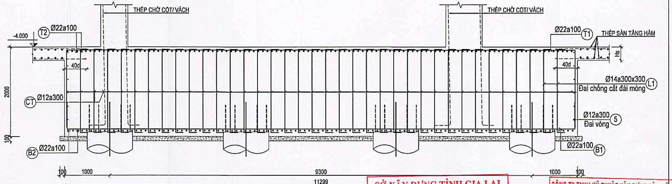
MẶT CẮT 7c-7c TL: 1/50
