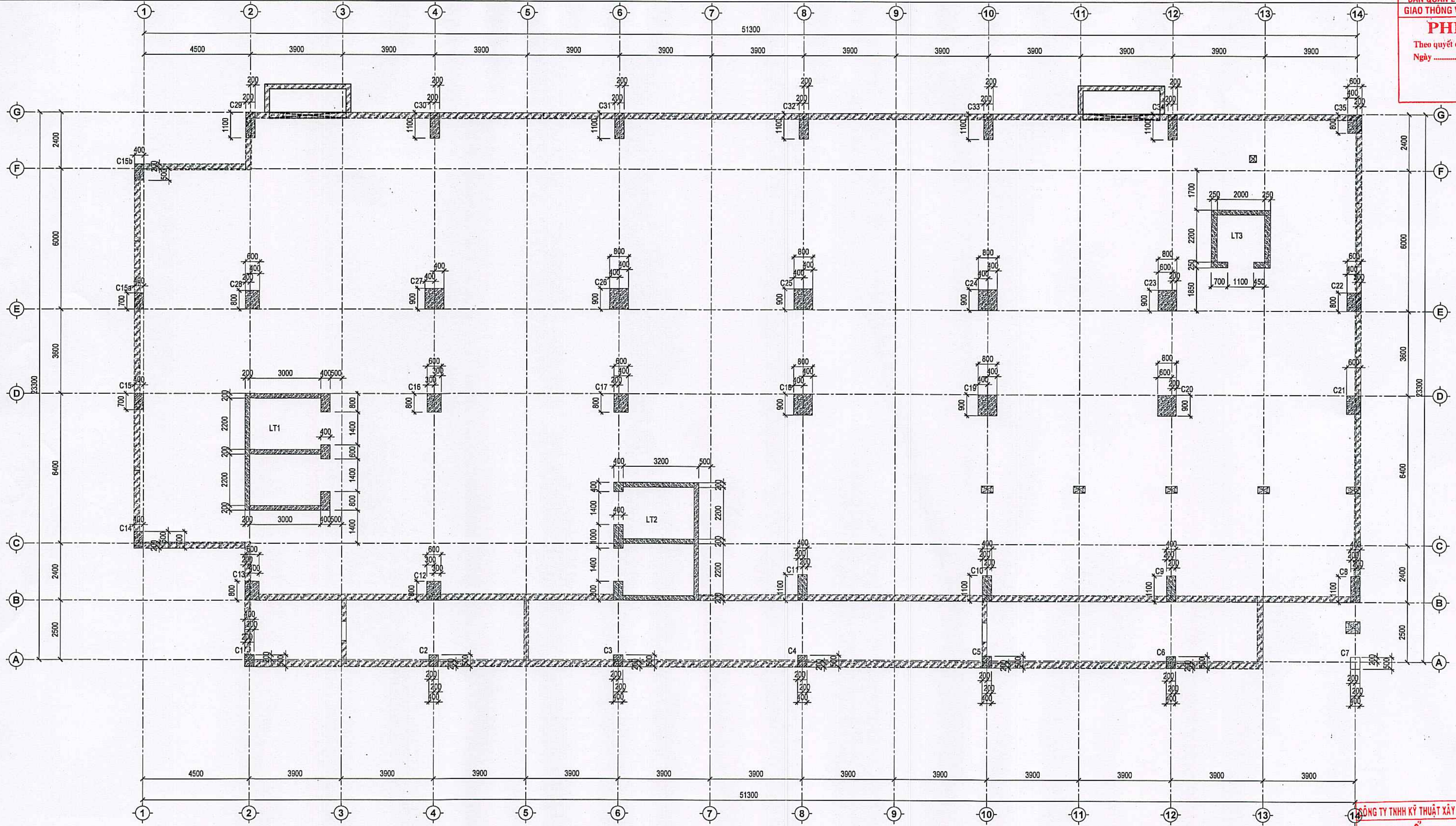
MẶT BẰNG CỘT VÁCH TẦNG 1 TỶ LỆ: 1:120
