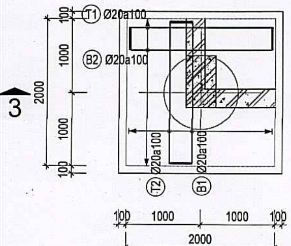
CHI TIẾT ĐÀI CỌC DC3 TL: 1/50
