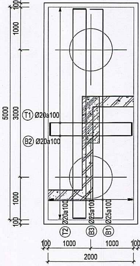
CHI TIẾT ĐÀI CỌC DC1a TL: 1/50
