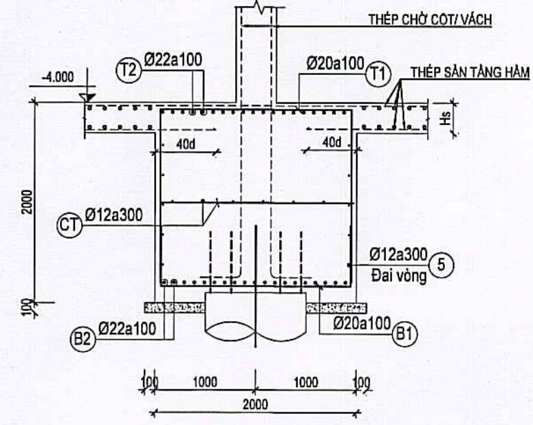
MẶT CẮT 2-2 TL: 1/50
