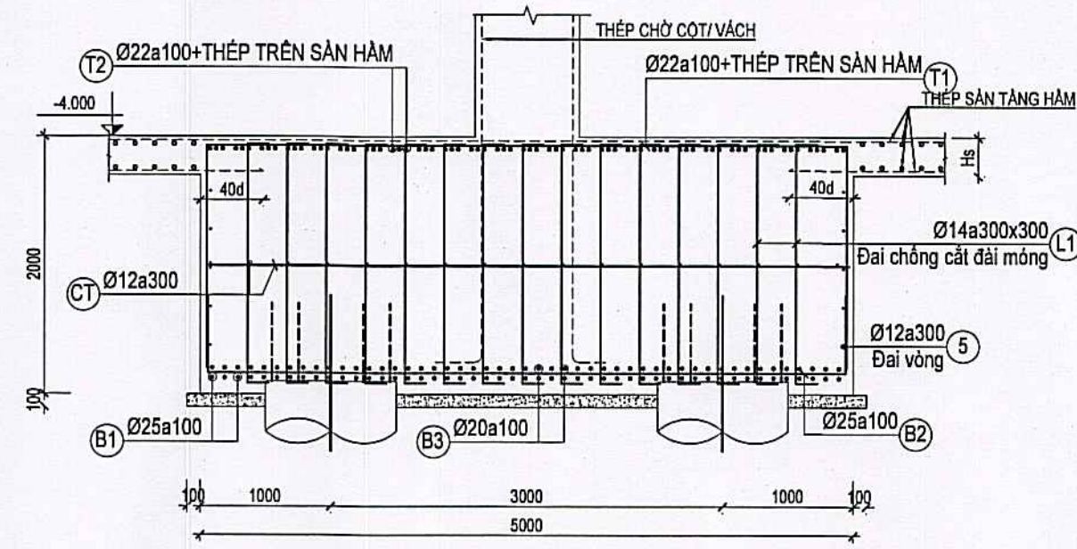
MẶT CẮT 8a-8a TL: 1/50
