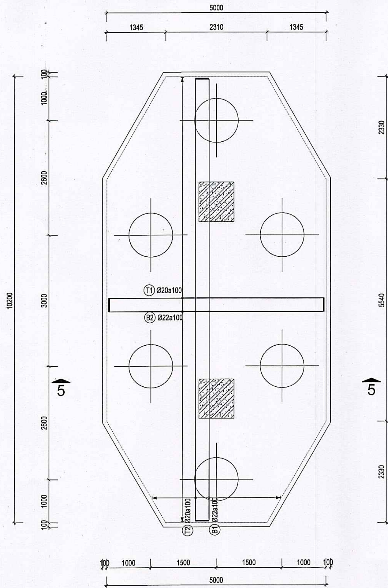
CHI TIẾT ĐÀI CỌC ĐC5 TL: 1/50
