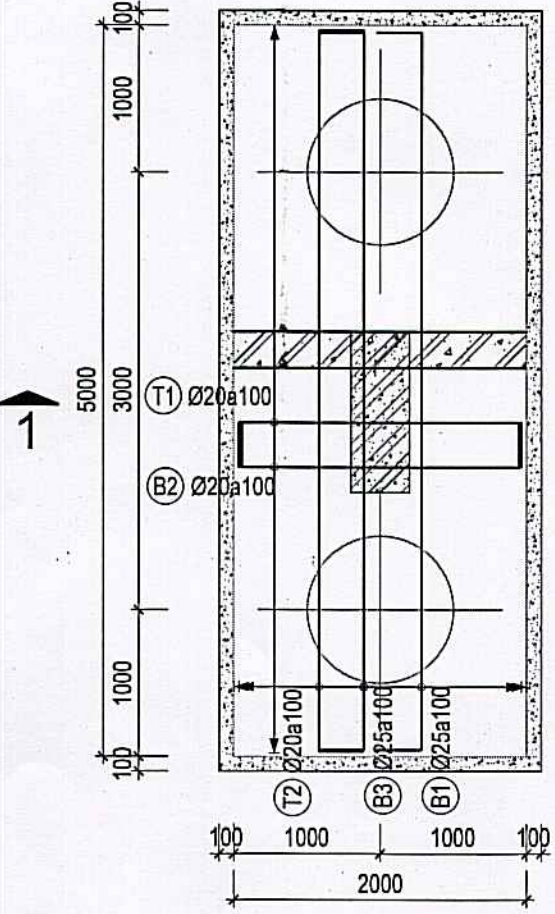
CHI TIẾT ĐÀI CỌC DC1 TL: 1/50
