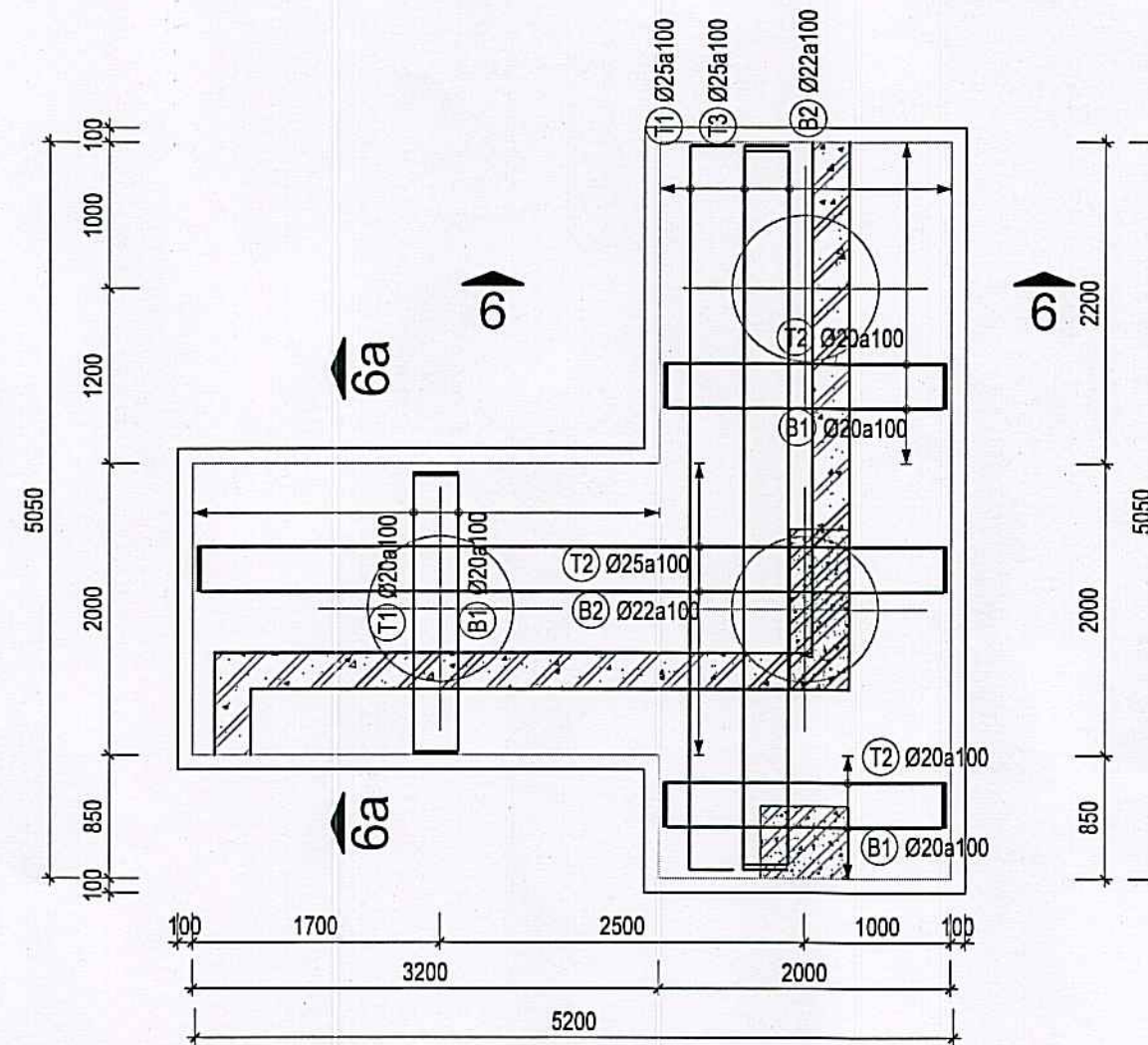
CHI TIẾT ĐÀI CỌC ĐC6 TL: 1/50
