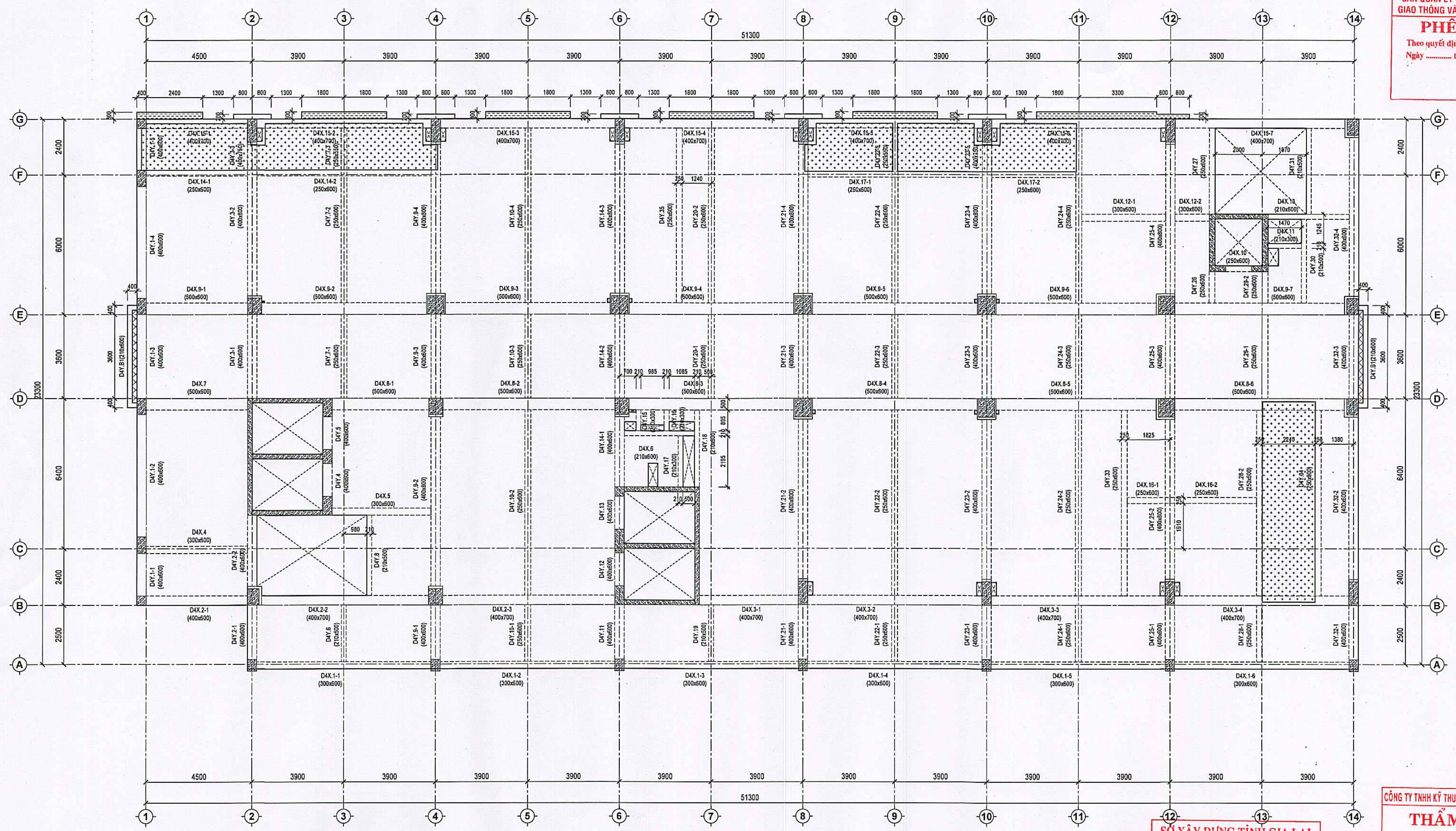
MẶT BẰNG KẾT CẤU SÀN TẦNG 4 TỶ LỆ: 1:100
