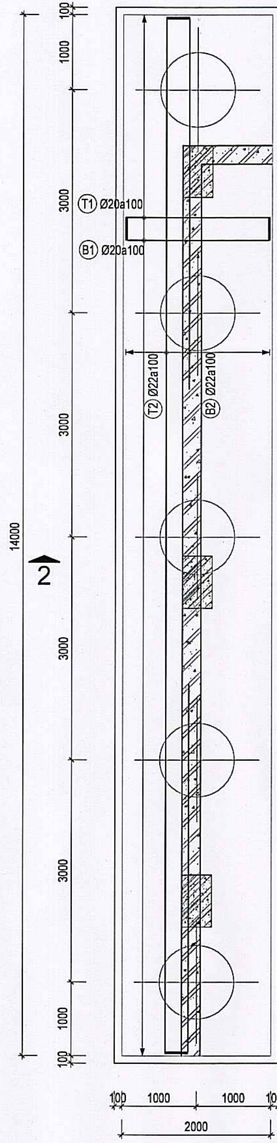
CHI TIẾT ĐÀI CỌC DC2 TL: 1/50
