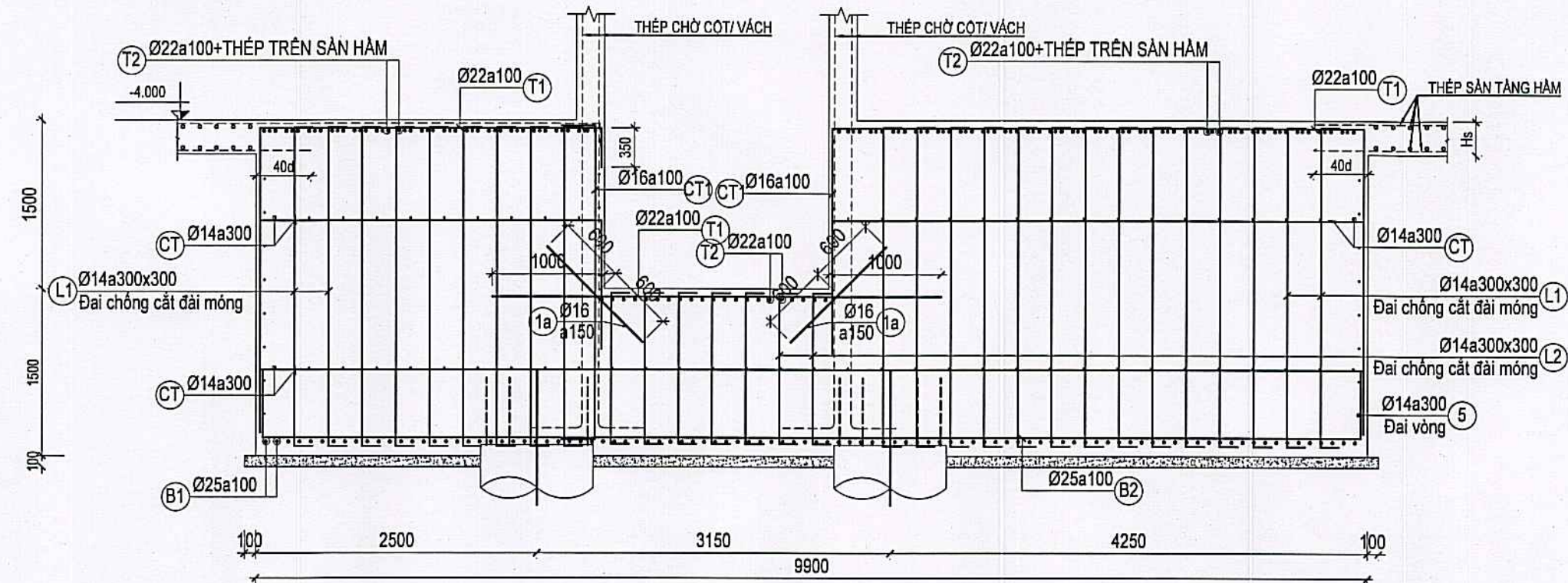
MẶT CẮT 9c-9c TL: 1/50
