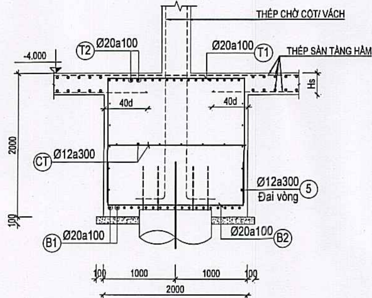
MẶT CẮT 3-3 TL: 1/50
