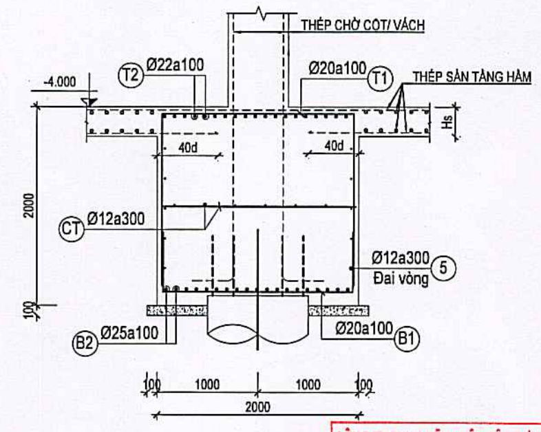
MẶT CẮT 4a-4a TL: 1/50
