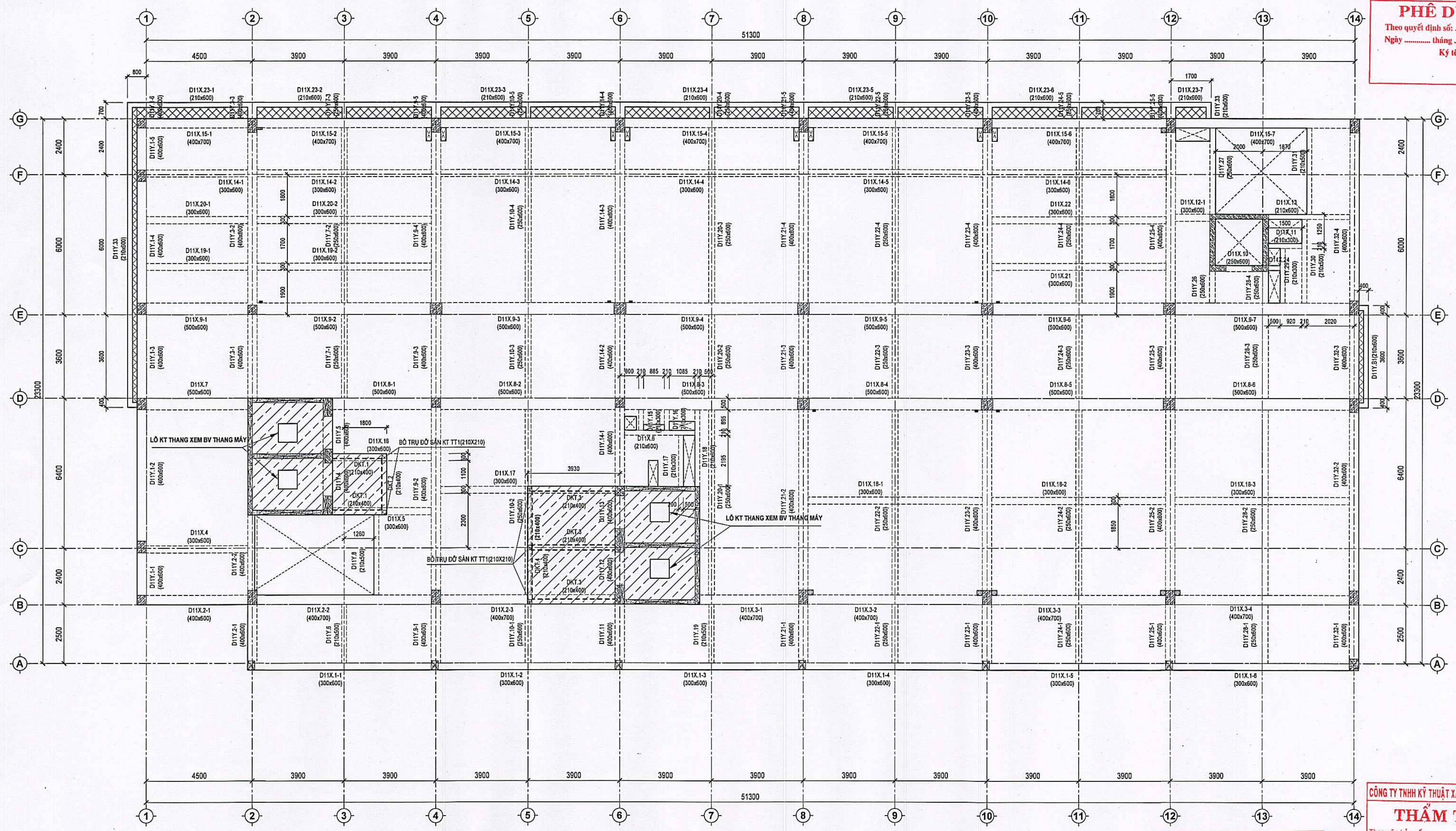
MẶT BẰNG KẾT CẤU SÀN TẦNG 11 TỶ LỆ: 1:100
