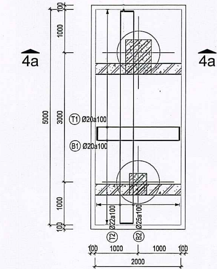
CHI TIẾT ĐÀI CỌC ĐC4a TL: 1/50
