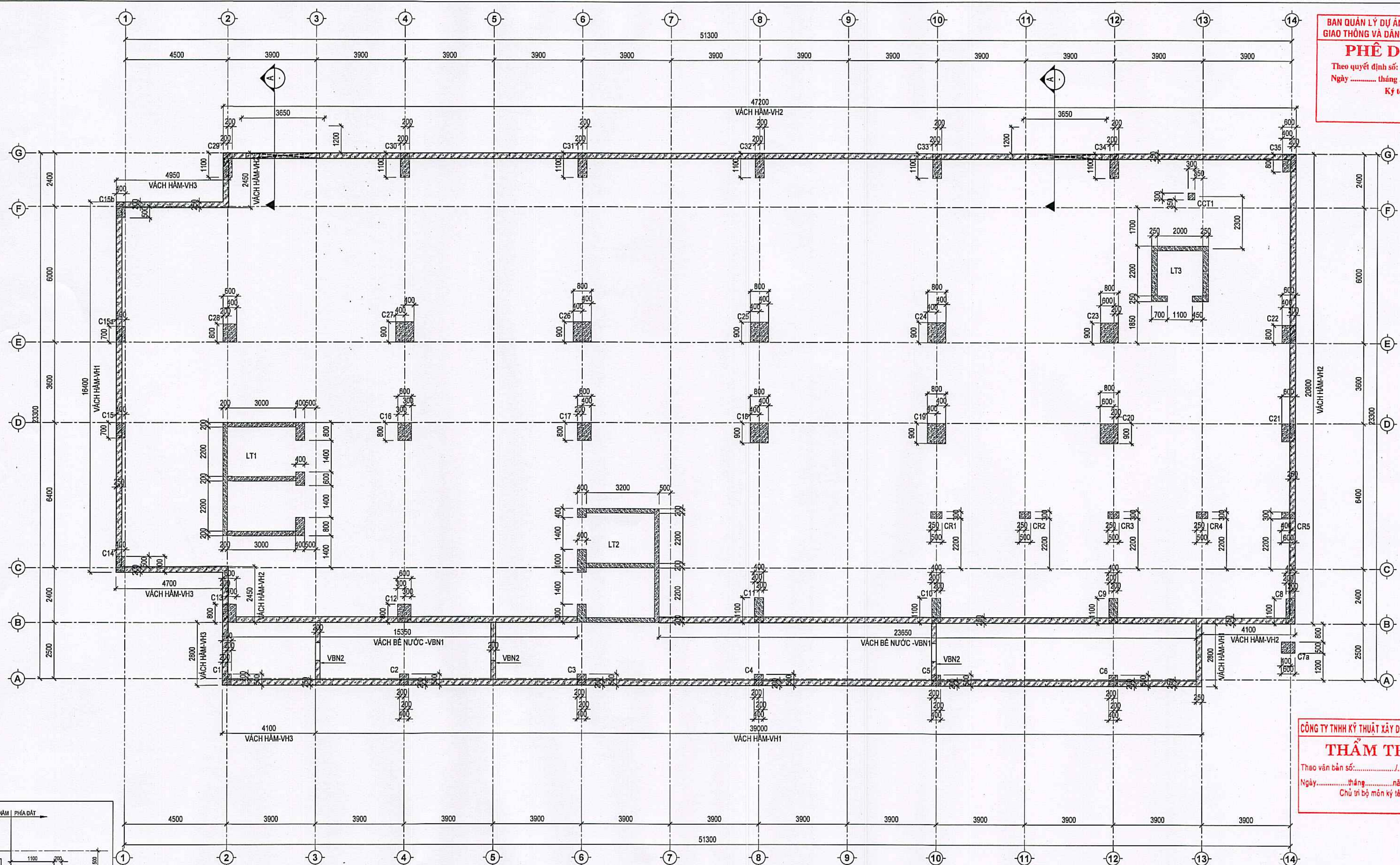
MẶT BẰNG CỘT VÁCH TẦNG HẠM TỶ LỆ: 1:120
