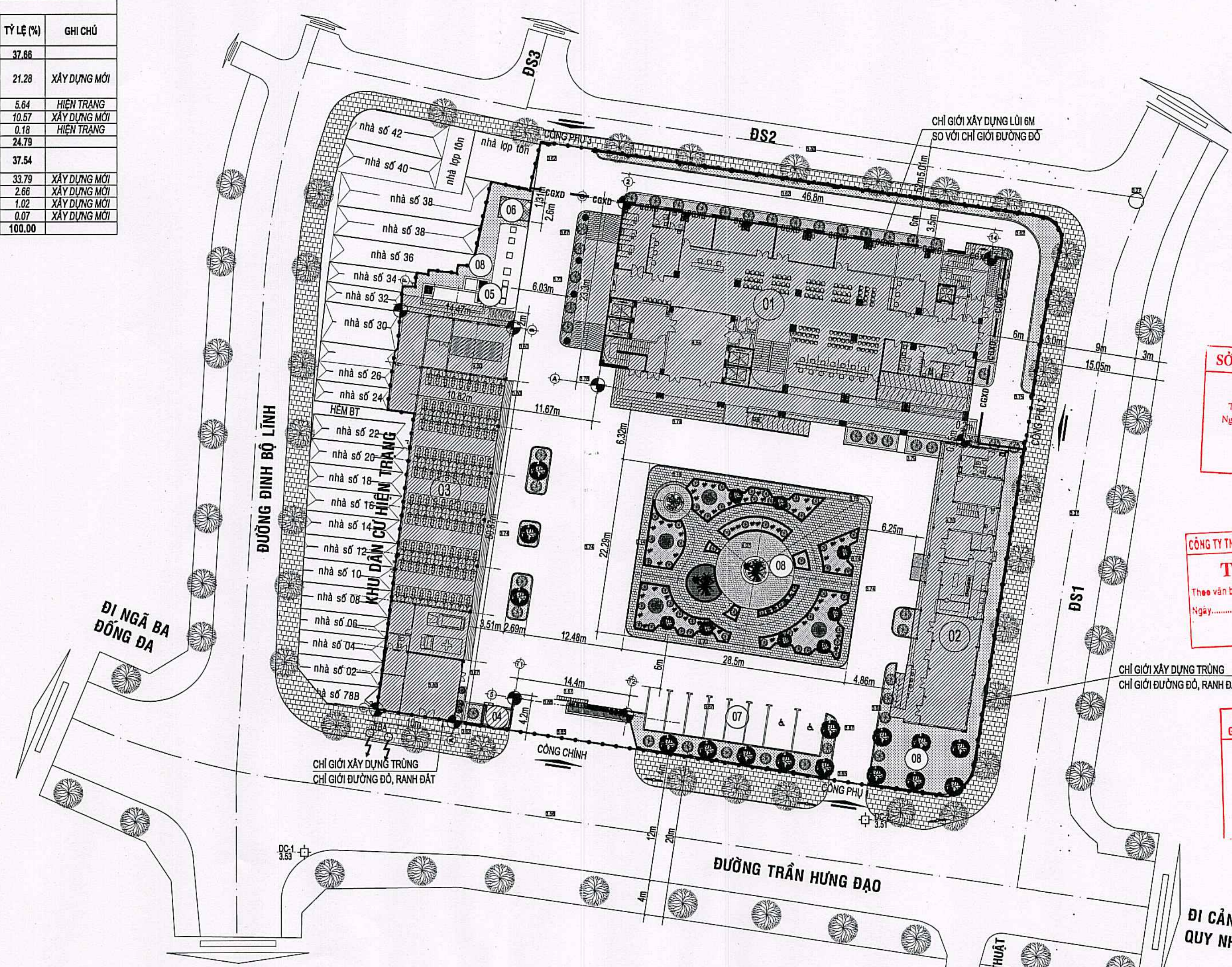
MẶT BẰNG TỔNG THỂ ĐỊNH VỊ CÁC HẠNG MỤC CÔNG TRÌNH
