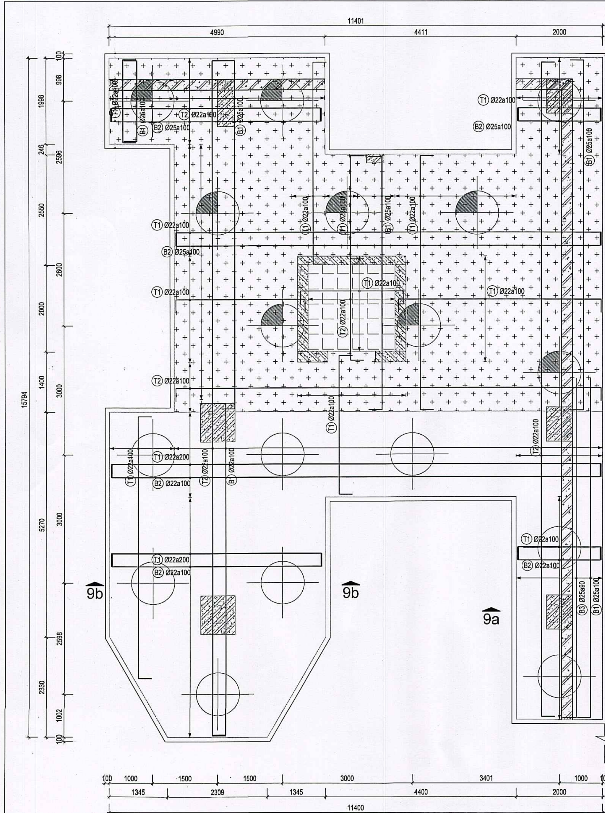
CHI TIẾT ĐÀI CỌC ĐC9 TL: 1/50
