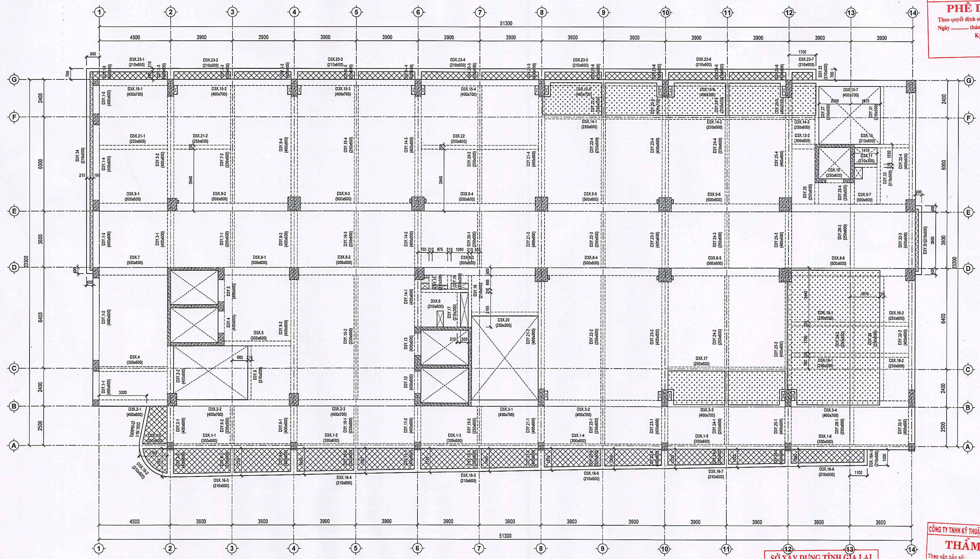
MẶT BẰNG KẾT CẤU SÀN TẦNG 3 TỶ LỆ: 1:100
