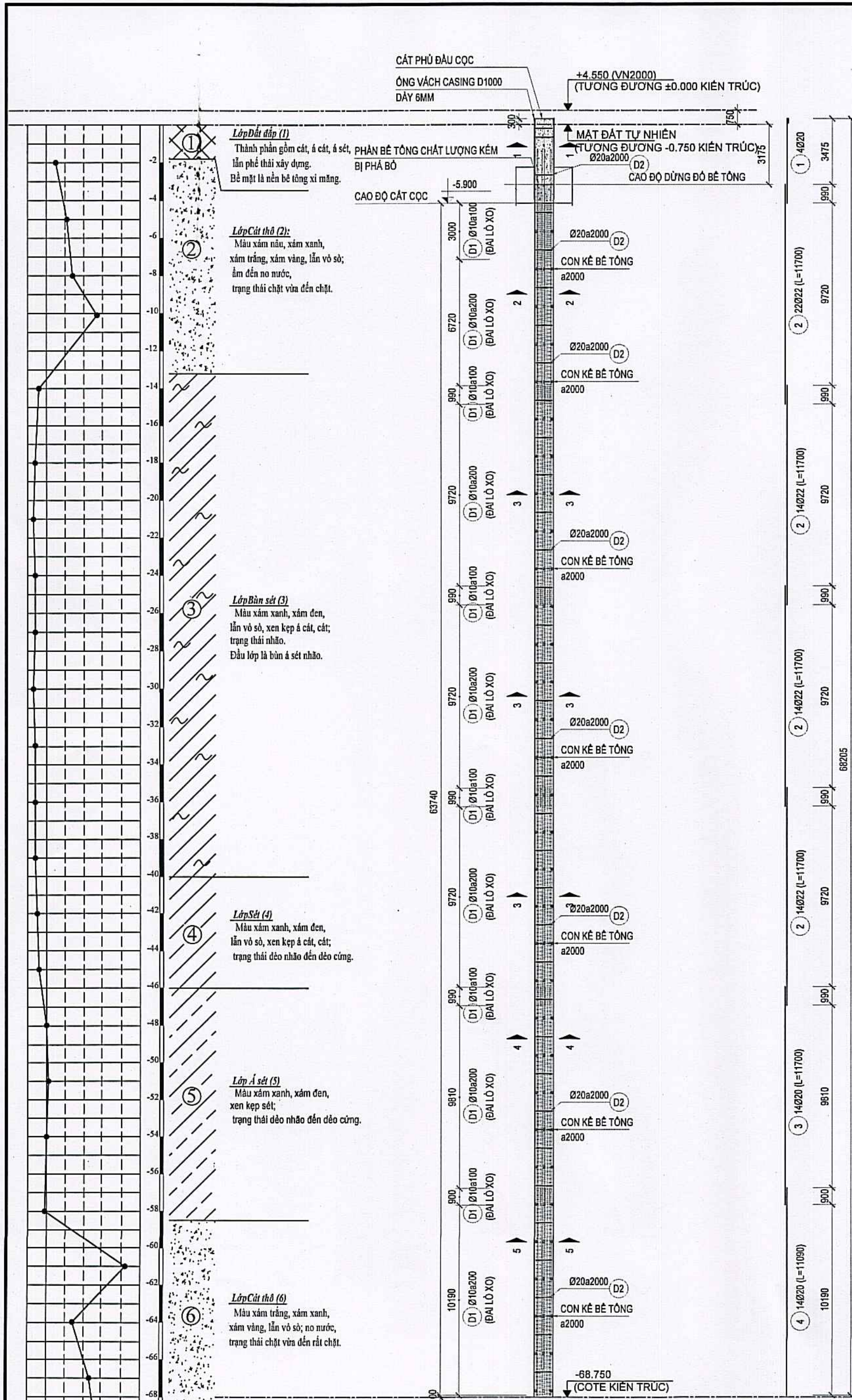
CỌC KHOAN NHỒI ĐẠ TRÀ - LOẠI CỌC C1
