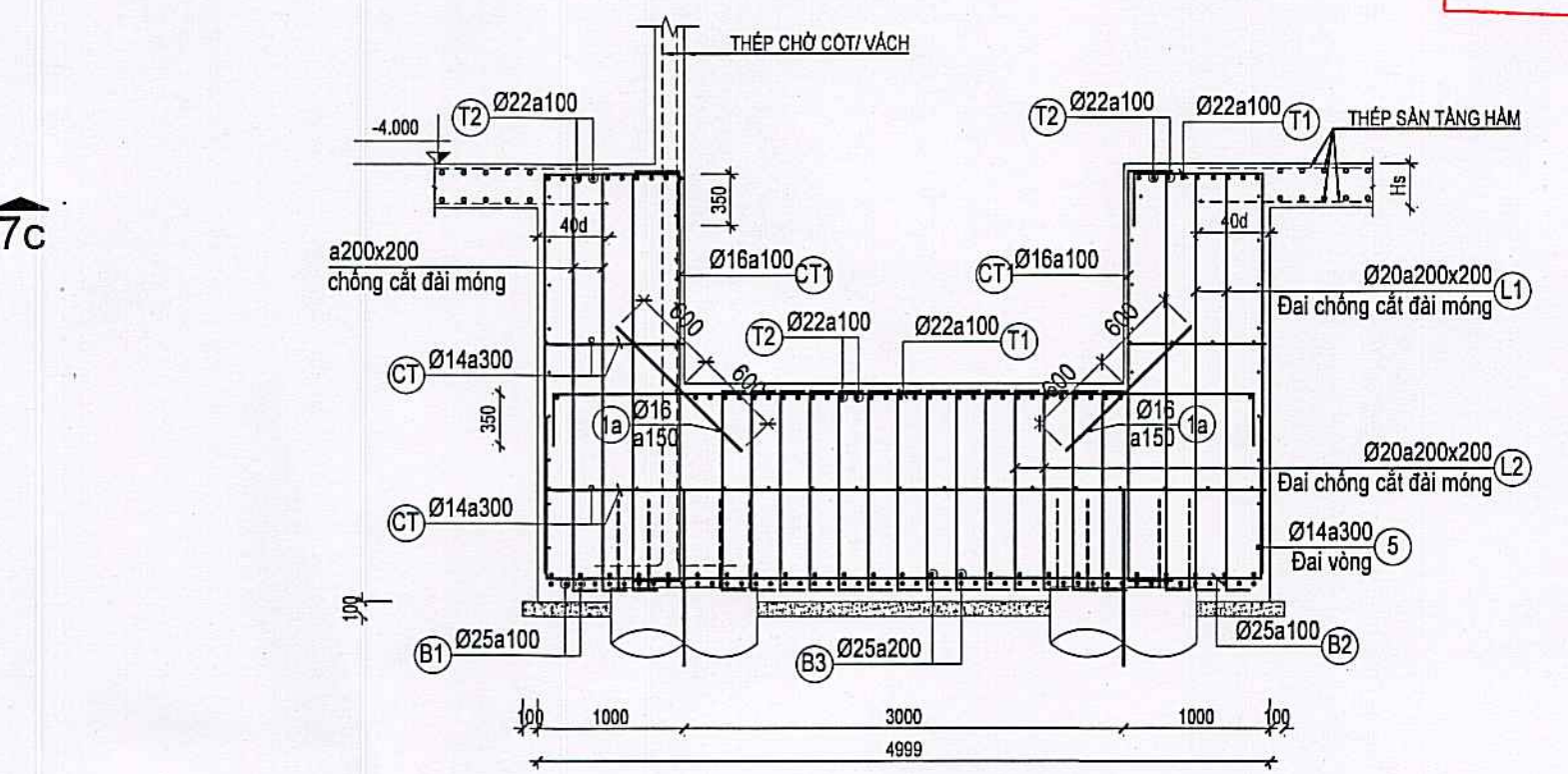
MẶT CẮT 7b-7b TL: 1/50
