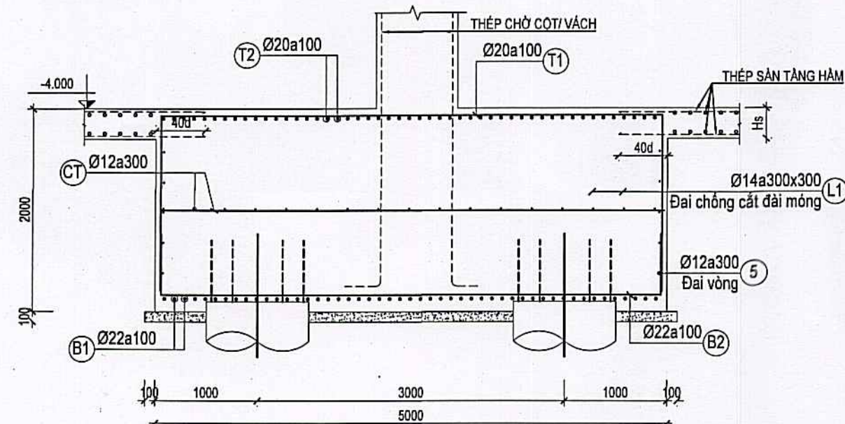
MẶT CẮT 5-5 TL: 1/50
