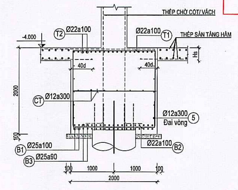
MẶT CẮT 9a-9a TL: 1/50
