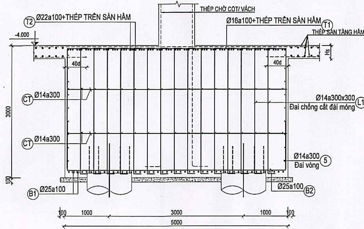
MẶT CẮT 8b-8b TL: 1/50
