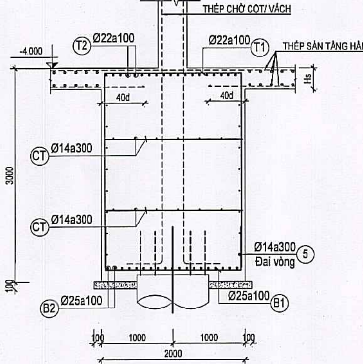
MẶT CẮT 7a-7a TL: 1/50
