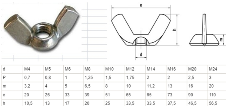
Hình 2.2: Đai ốc dạng tai hồng
