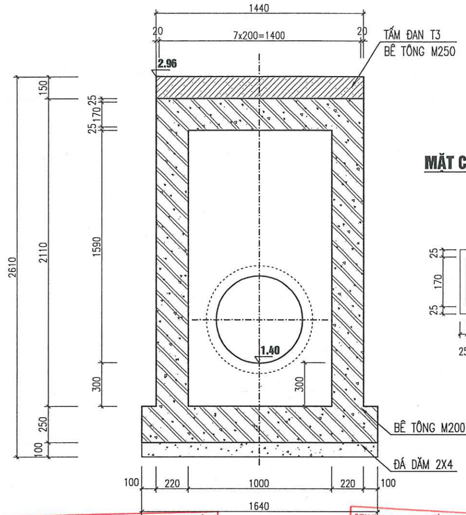
MẶT CẮT 2-2
