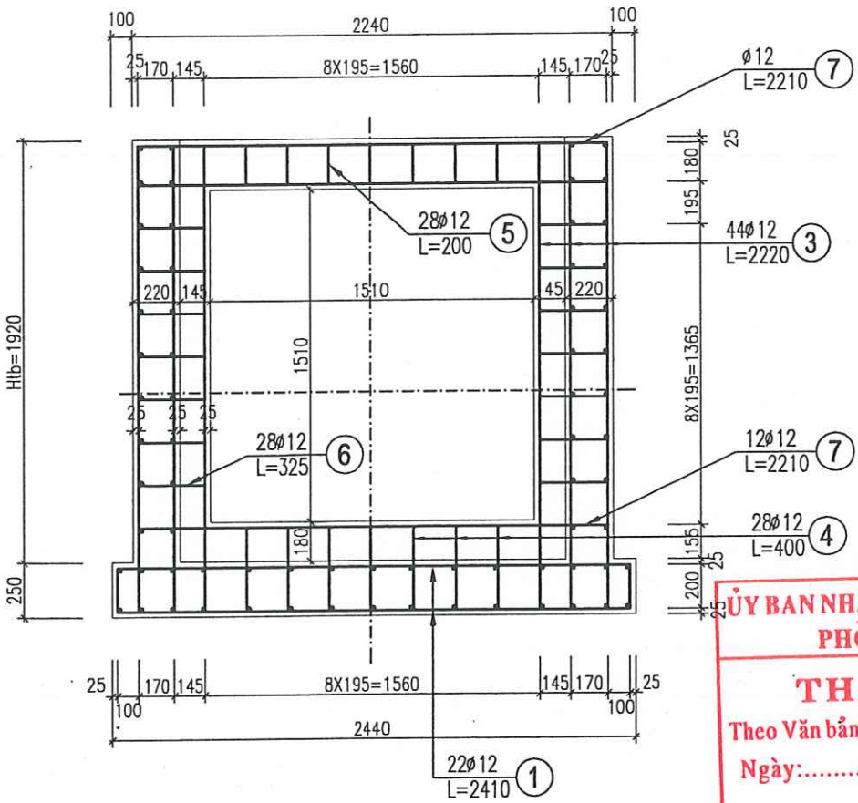
MẶT CẮT 2-2
