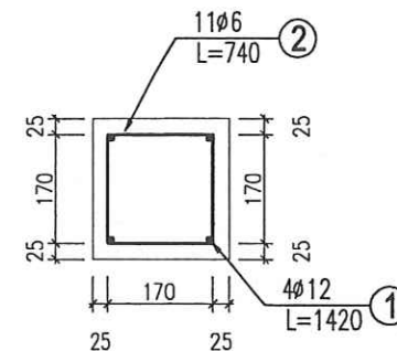
MẶT CẮT NGANG DẦM HỐ
