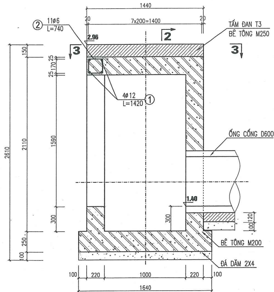
MẶT CẮT 1-1
