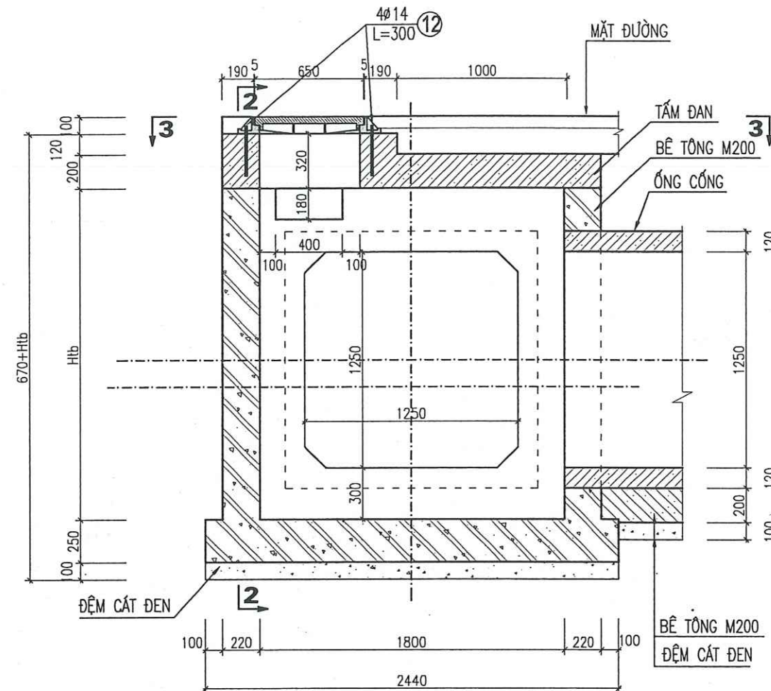
MẶT CẮT 1-1
