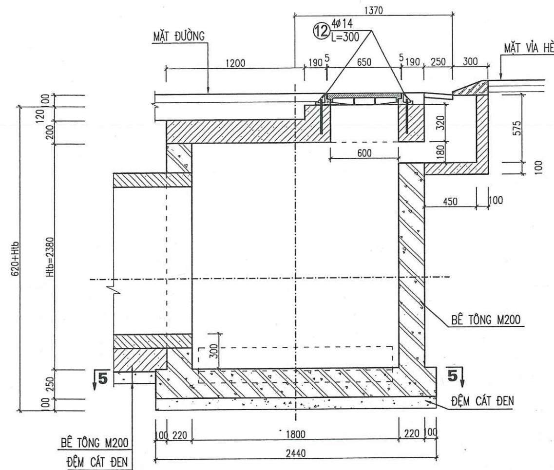
MẶT CẮT 2-2
