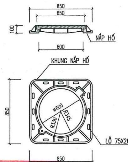
CẤU TẠO KHUNG, NẮP HỔ THU
