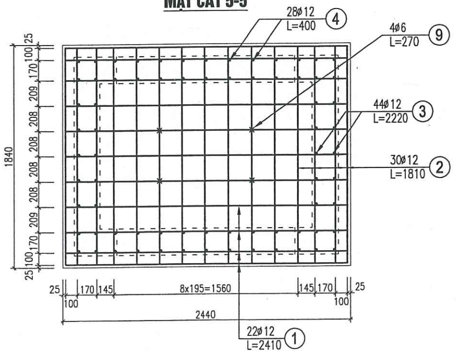
MẶT CẮT 5-5
