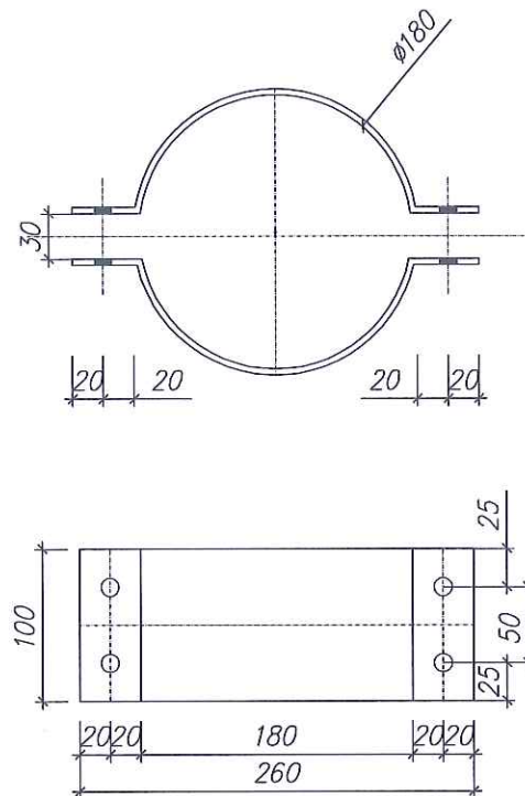
MỐI NỐI ỐNG THÉP FI 168,3 (Thép dẹt 100x4)
