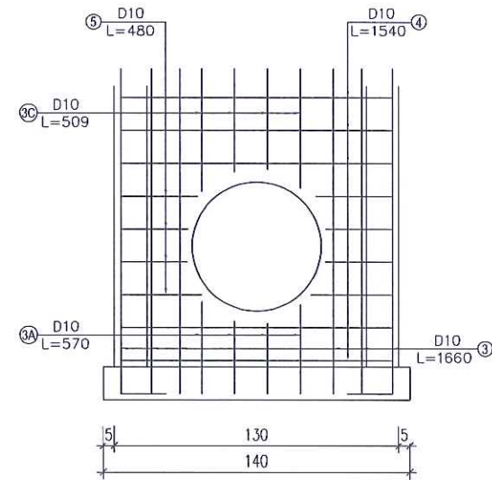
MẶT CẮT D-D
