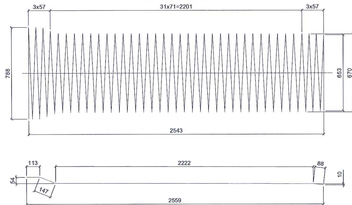
CỐT THÉP SỐ 2
