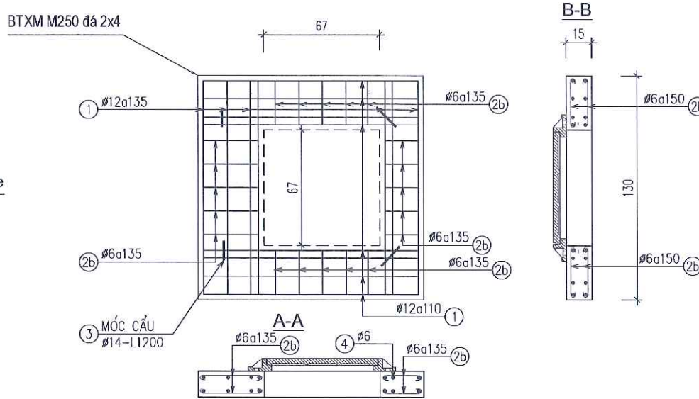
CHI TIẾT TẤM ĐAN KT:130X130X15CM
