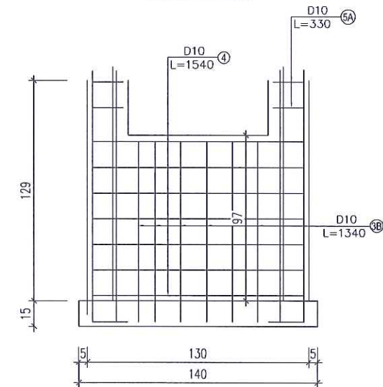
MẶT CẮT D-D
