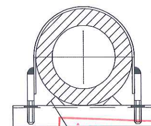
MẶT CẮT A -:- A
