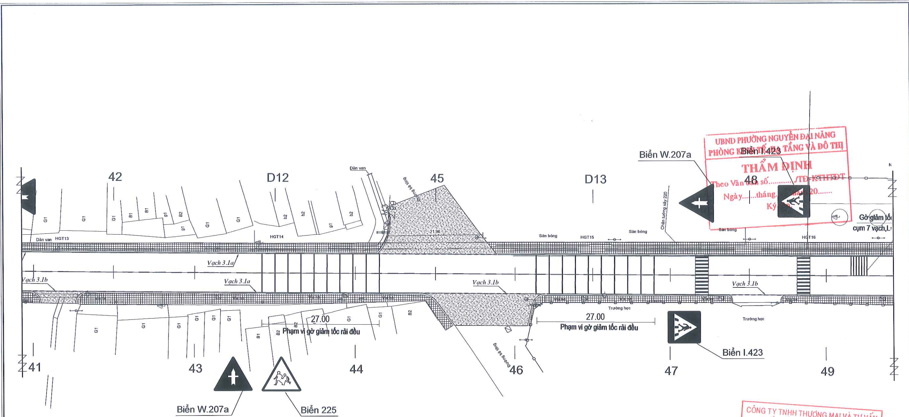
BẢNG KÝ HIỆU VẠCH SƠN BIỂN BÁO ATGT
