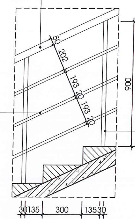
CHI TIẾT LAN CAN
