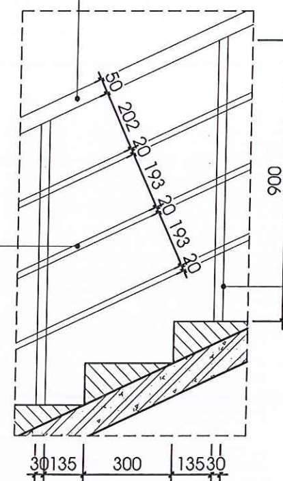
CHI TIẾT LAN CAN
