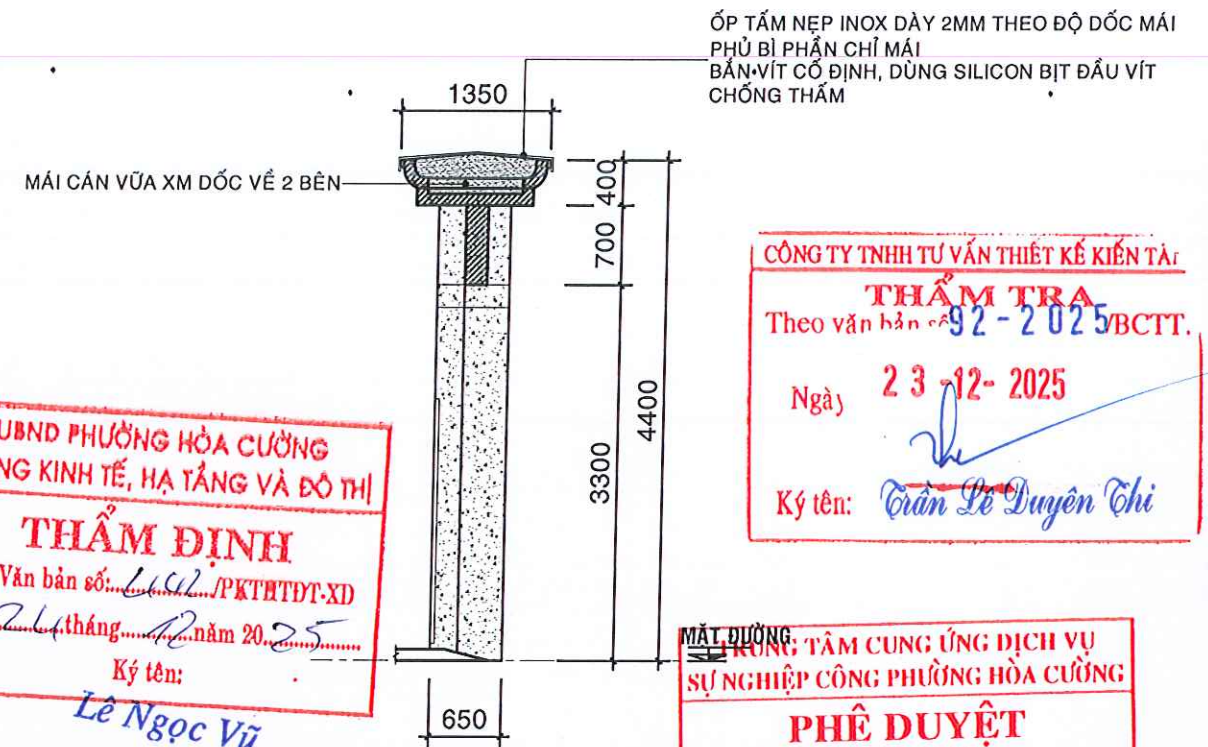
MẶT CẮT CẢI TẠO
