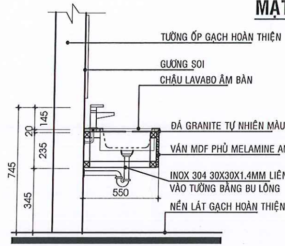
CHI TIẾT MẶT CẮT LAVABO
