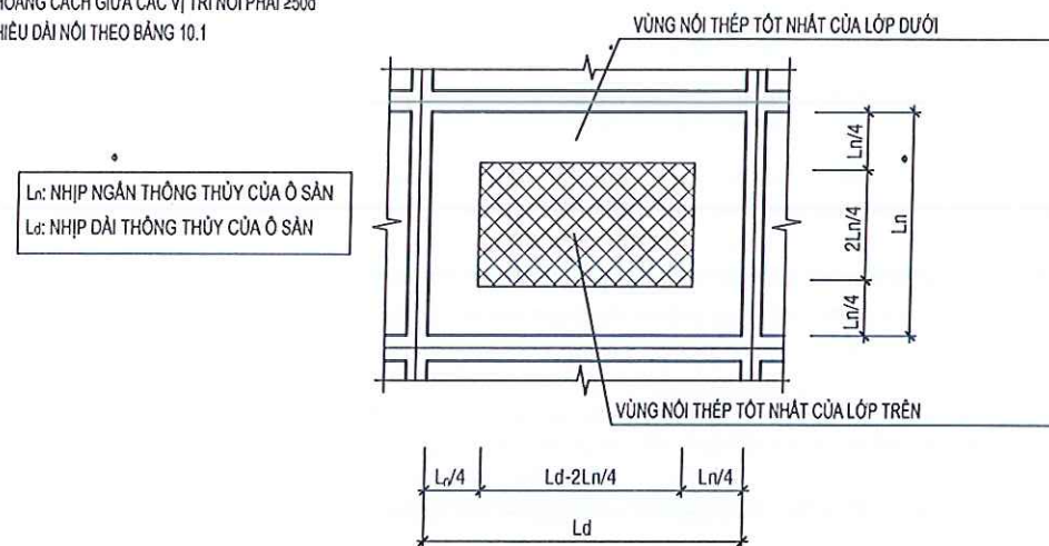
MINH HỌA VÙNG NỘI CỐT THÉP SÀN
