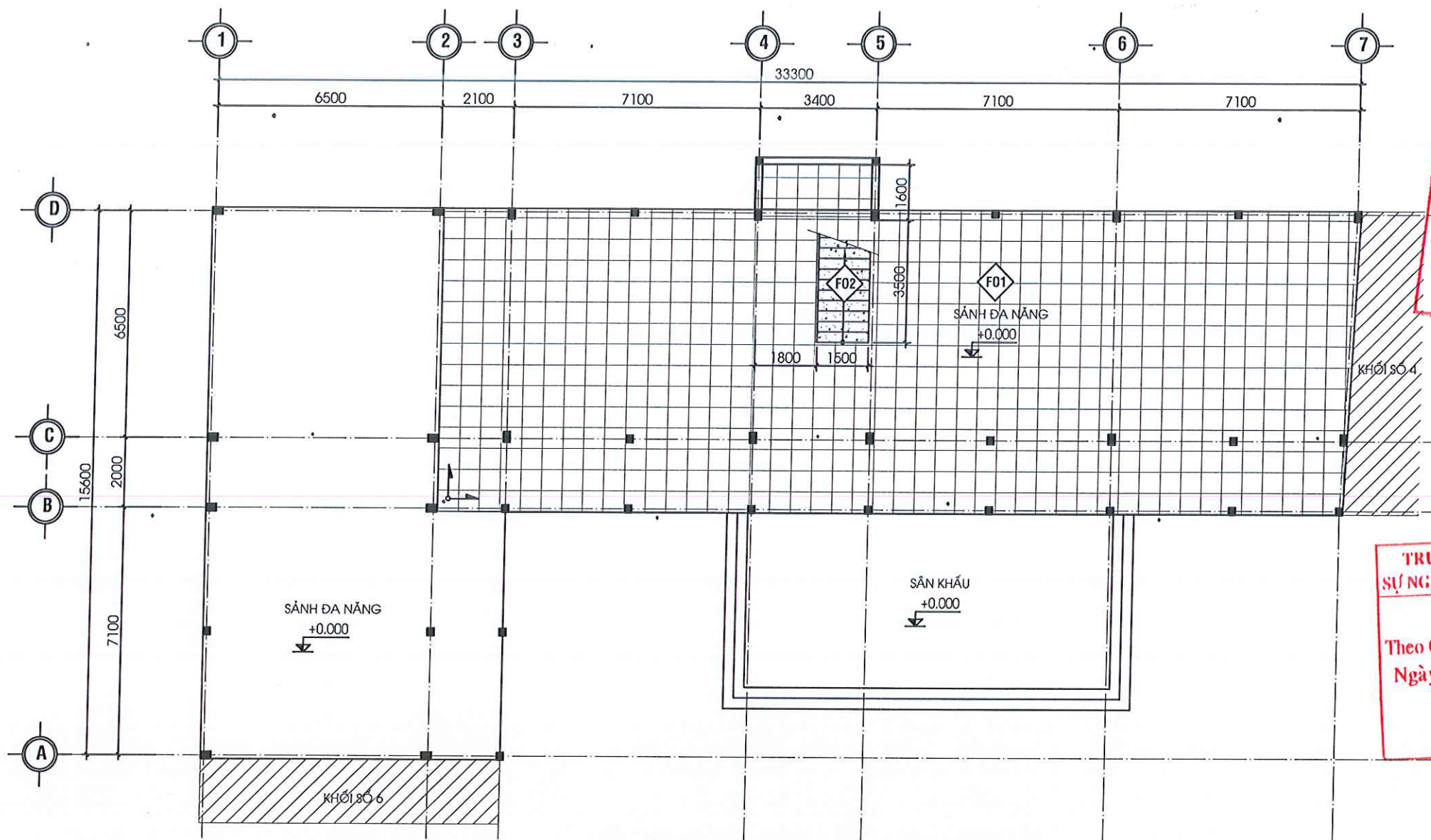
MẶT BẰNG LÁT GẠCH TẦNG 1 - KHỐI SỐ 5
