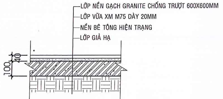
CẤU TẠO NỀN GẠCH (CẢI TẠO)
