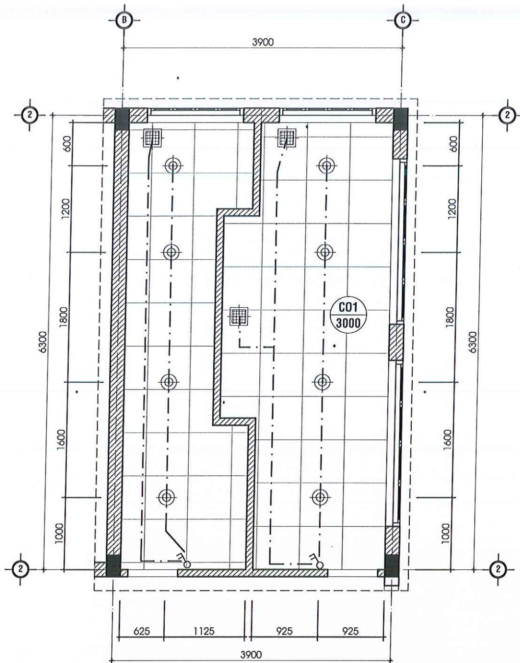
MẶT BẰNG TRẦN ĐÈN KHU VỆ SINH TẦNG 1
