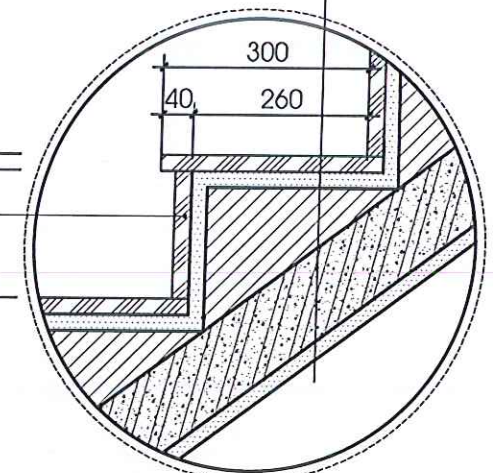
CHI TIẾT BẬC THANG
