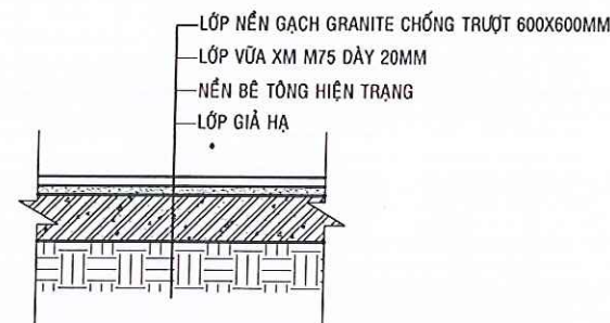
CẤU TẠO NỀN GẠCH
