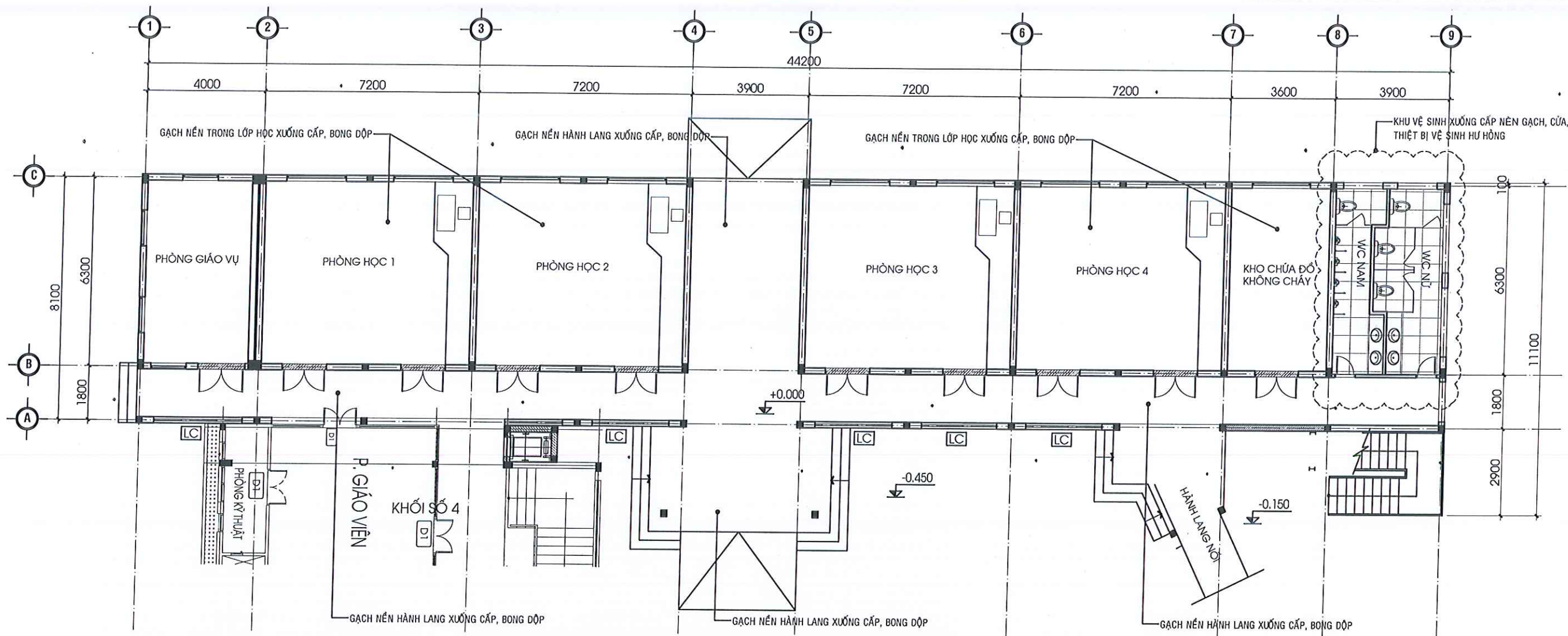
MẶT BẰNG HIỆN TRẠNG TẦNG 1 - KHỐI SỐ 2
