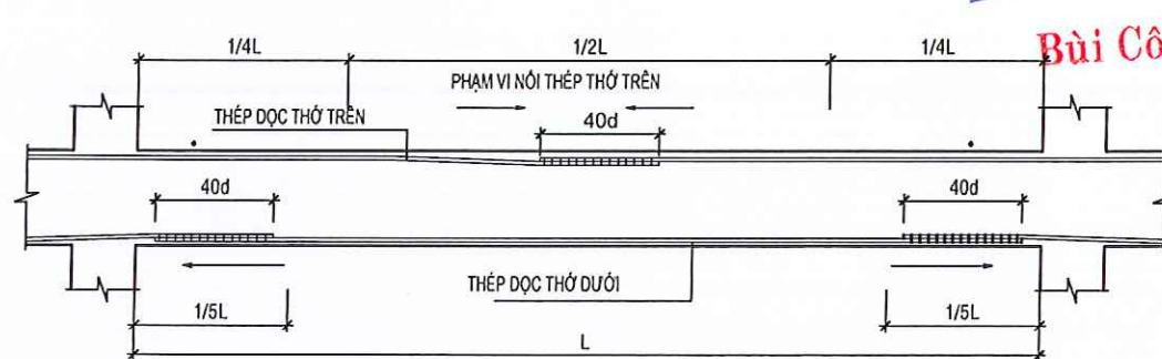
MINH HỌA NỐI THÉP DÀM ĐIỂN HÌNH
