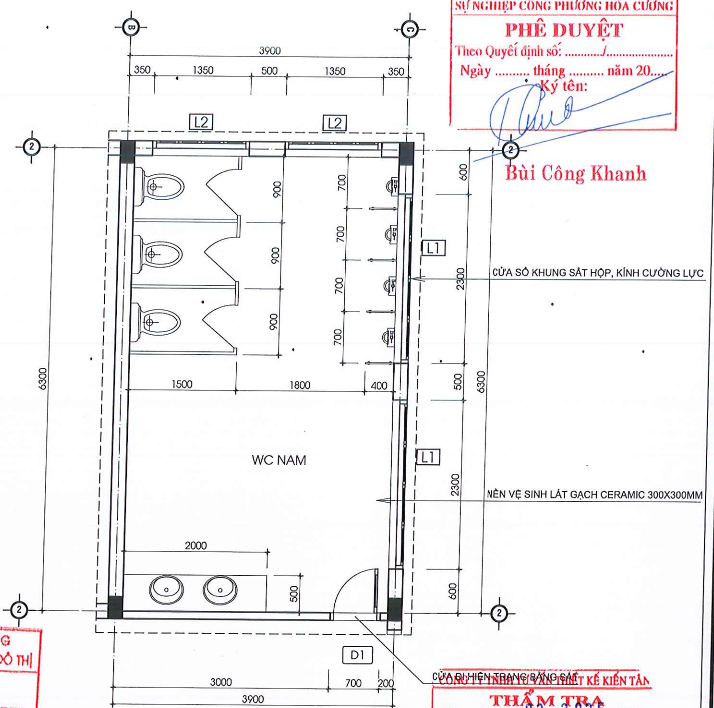
MẶT BẰNG KHU VỆ SINH TẦNG 2
