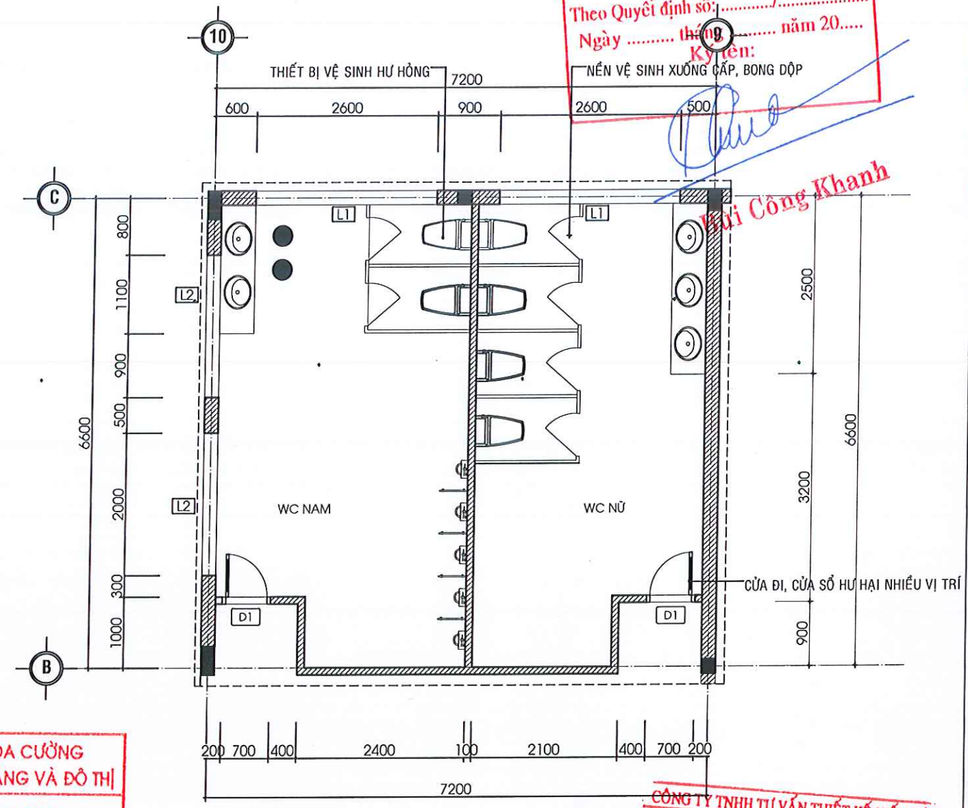
MẶT BẰNG HIỆN TRẠNG KHU VỆ SINH TẦNG 2
