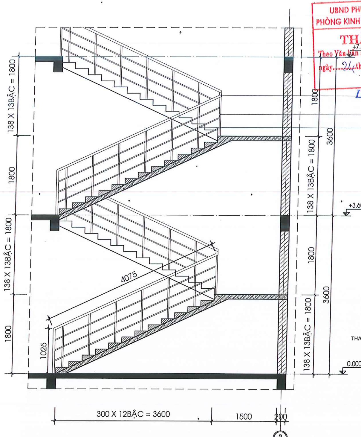
MẶT CẮT CẦU THANG HIỆN TRẠNG
