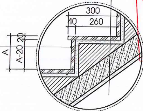
CHI TIẾT BẬC THANG
