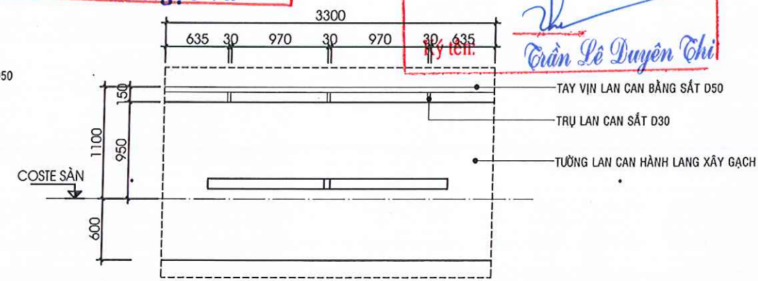
LAN CAN HÀNH LANG ĐIỂN HÌNH TẦNG 2, 3
