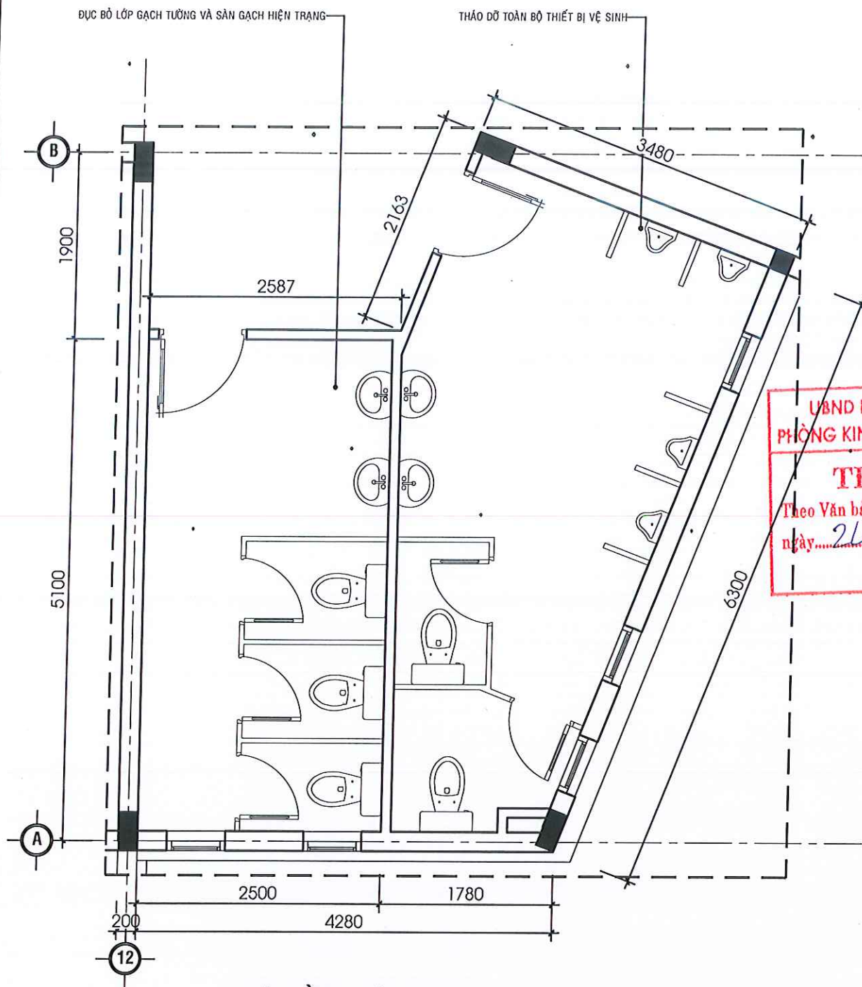
MẶT BẰNG HIỆN TRẠNG
