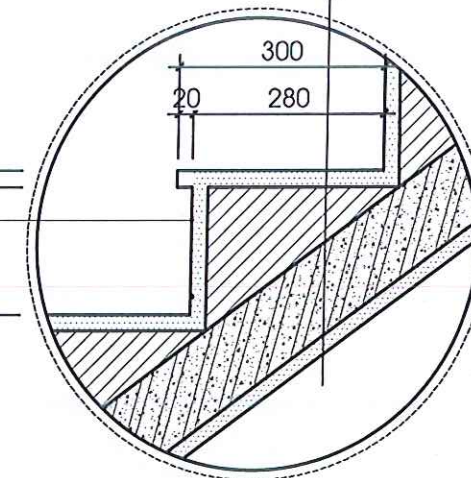
CHI TIẾT BẬC THANG
