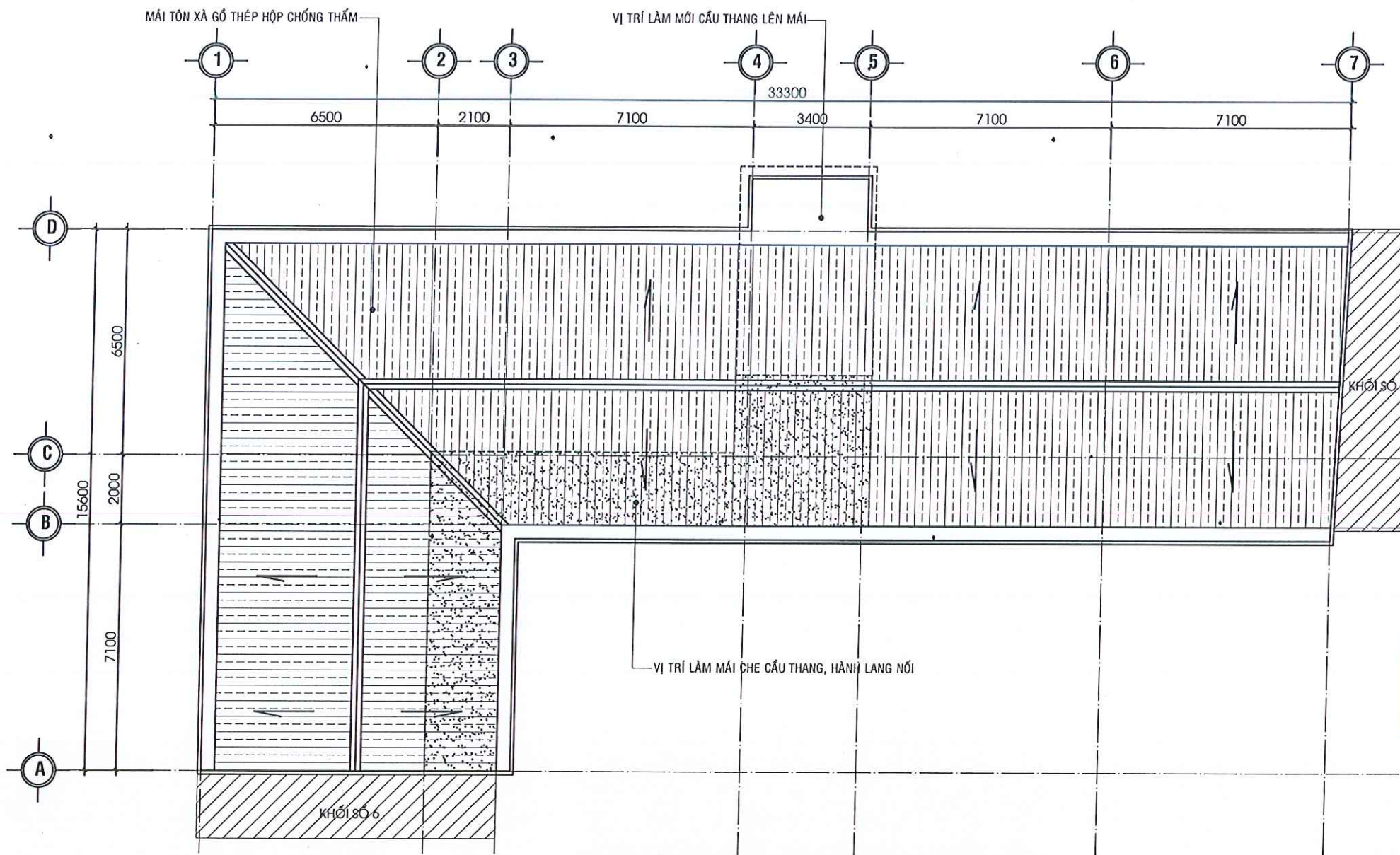
MẶT BẰNG HIỆN TRẠNG MÁI - KHỐI SỐ 5
