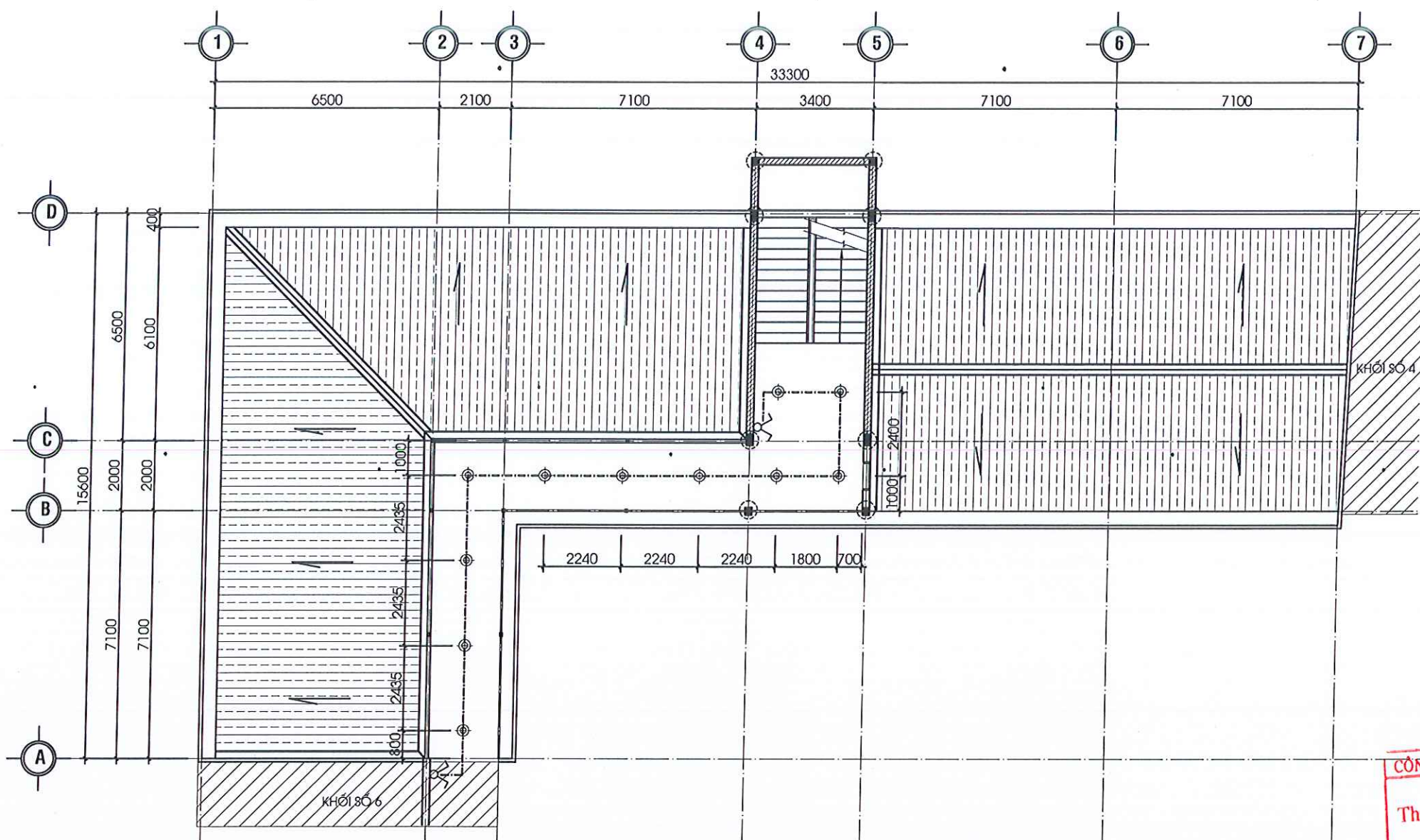
MẶT BẰNG CHIẾU SÁNG MÁI - KHỐI SỐ 5
