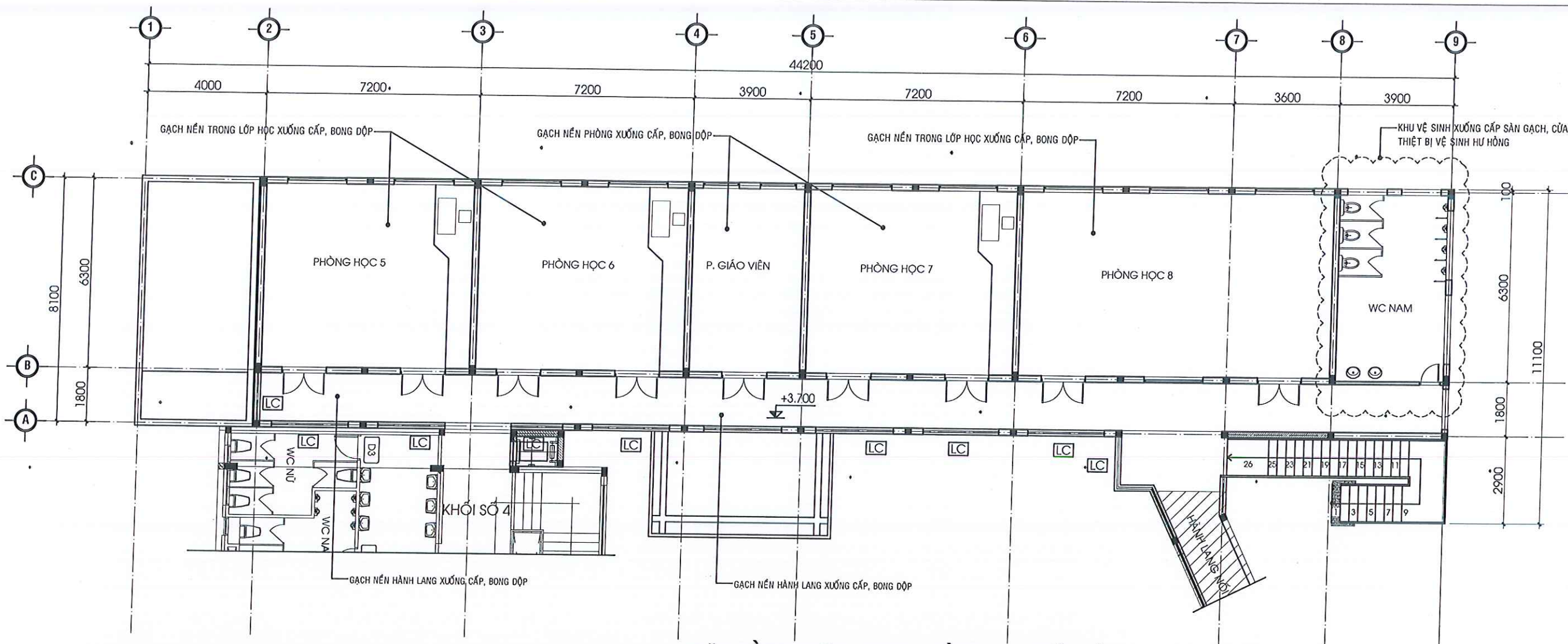
MẶT BẰNG HIỆN TRẠNG TẦNG 2 - KHỐI SỐ 2
