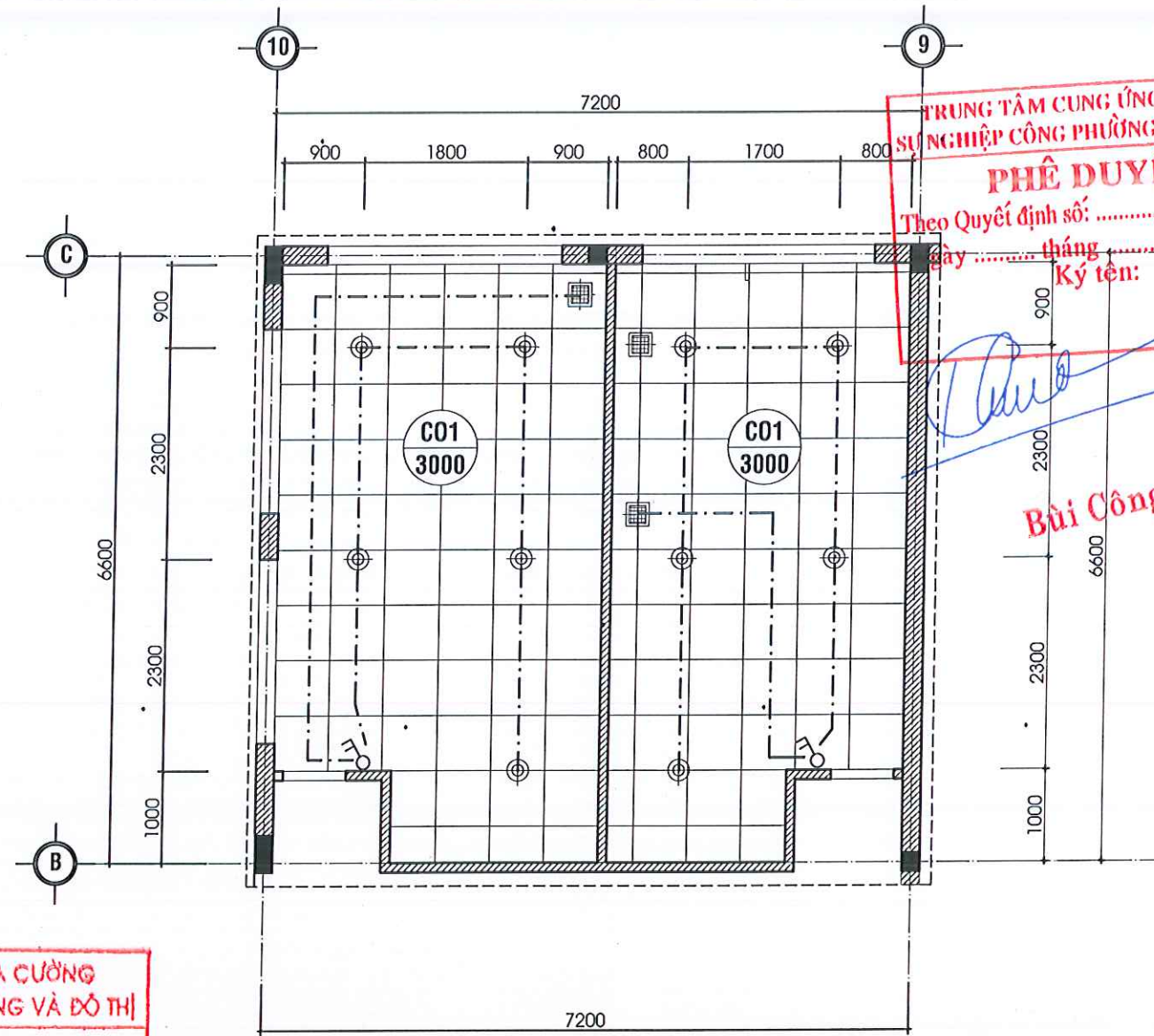
MẶT BẰNG TRẦN ĐÈN KHU VỆ SINH TẦNG 1
