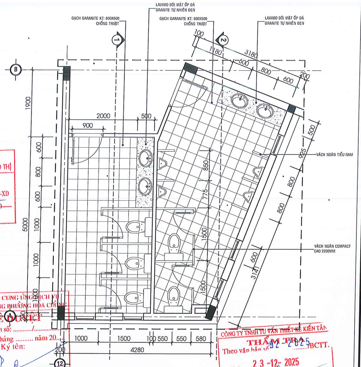
MẶT BẰNG CẢI TẠO
