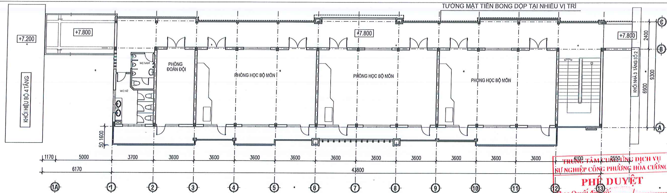
MẶT BẰNG HIỆN TRẠNG TẦNG 3
