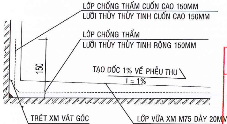
MẶT CẮT NGANG SÊ NÔ
