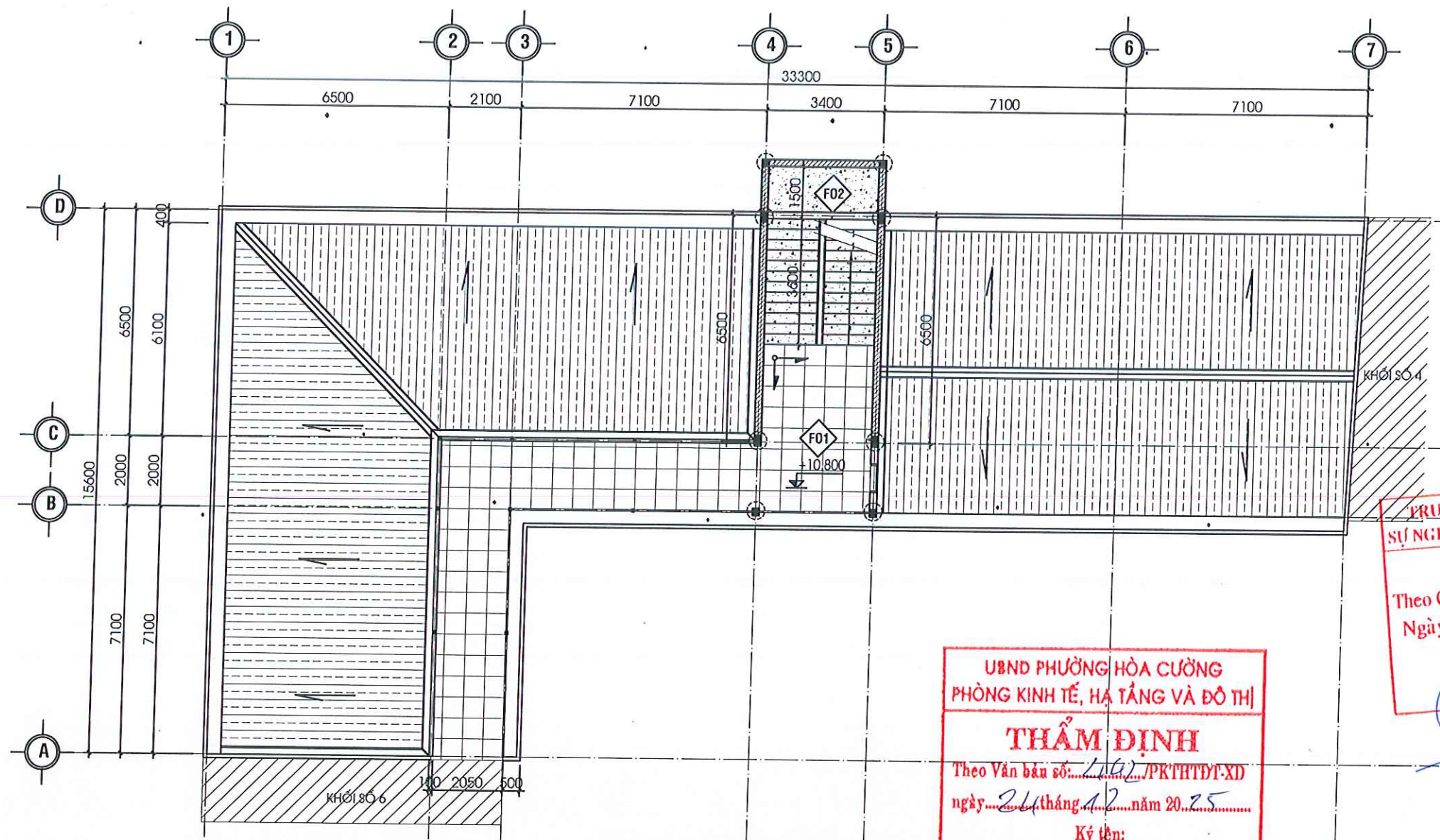
MẶT BẰNG LÁT GẠCH MÁI - KHỐI SỐ 5
