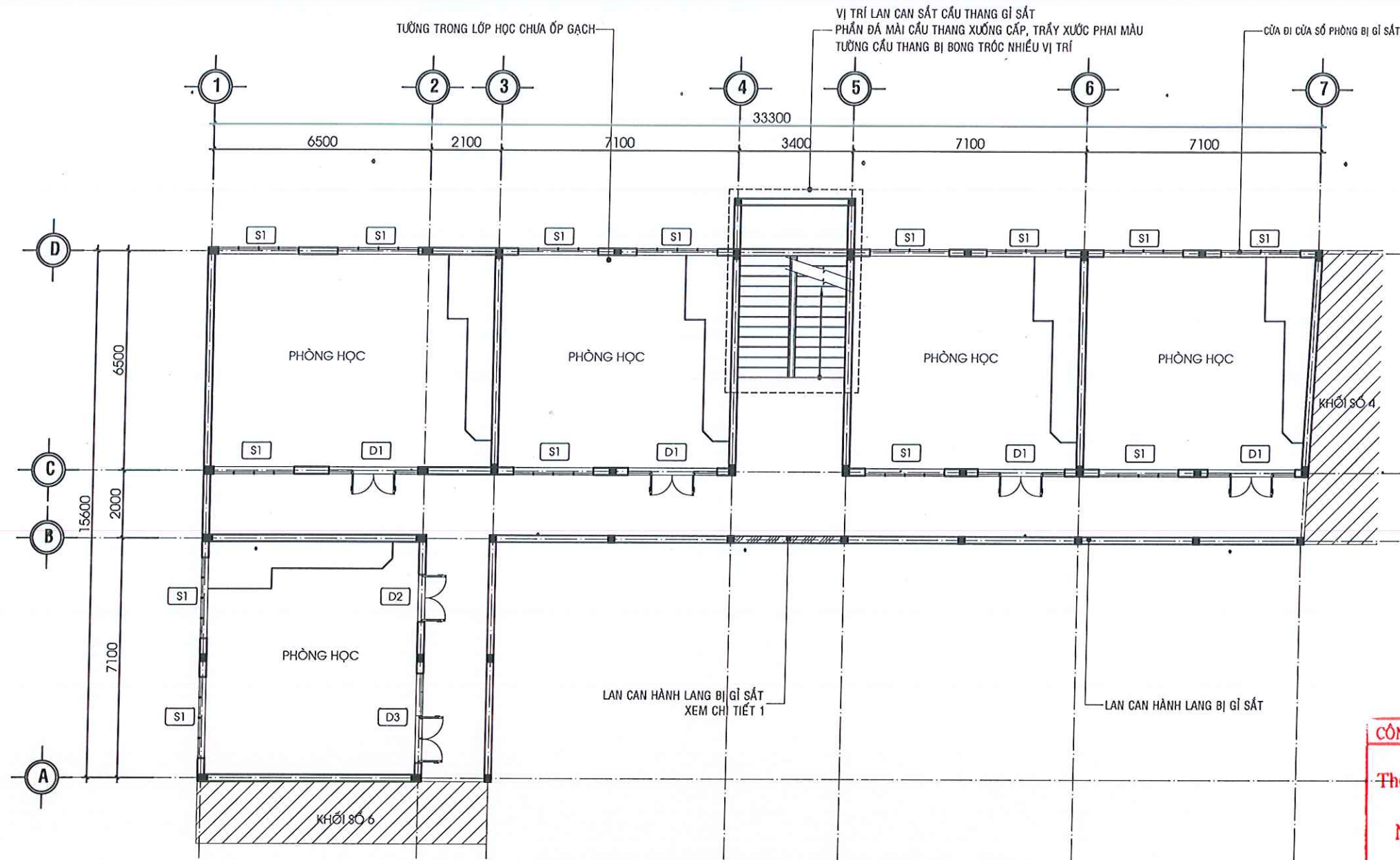
MẶT BẰNG HIỆN TRẠNG TẦNG 2 - KHỐI SỐ 5
