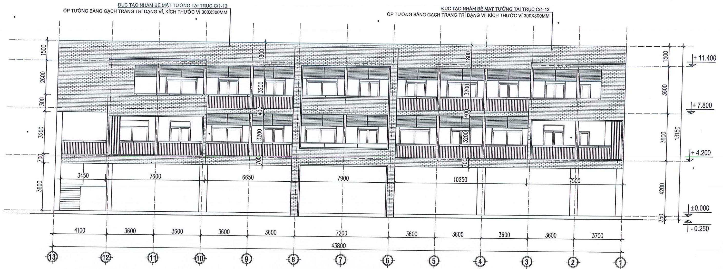
MẶT ĐỨNG CẢI TẠO TRỤC 13-1
