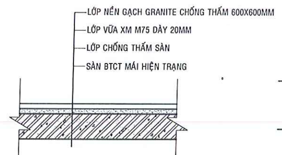
CẤU TẠO NỀN HÀNH LANG
