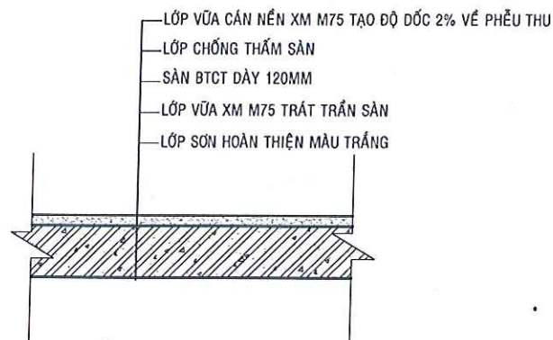
CẤU TẠO SÀN MÁI
