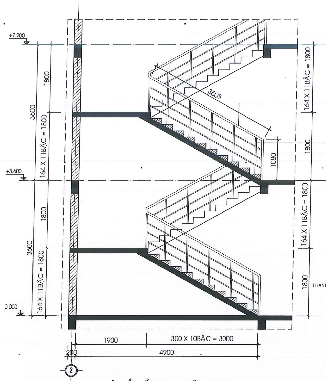
MẶT CẮT CẦU THANG HIỆN TRẠNG
