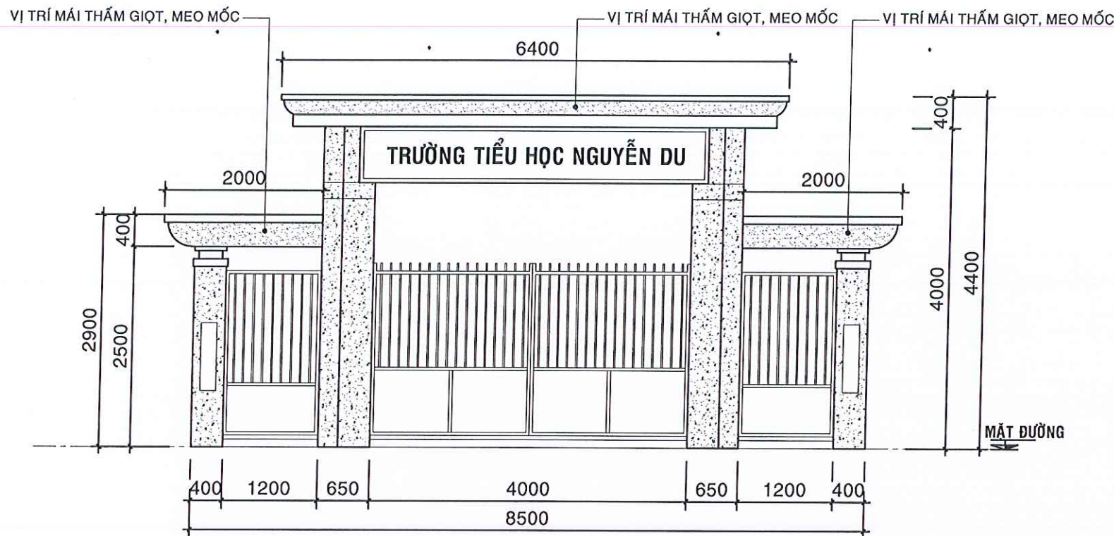
MẶT ĐỨNG HIỆN TRẠNG
