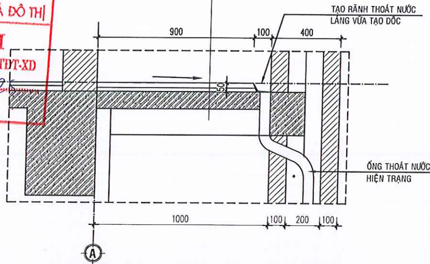
MẶT CẮT SÀN HÀNH LANG (CẢI TẠO)
