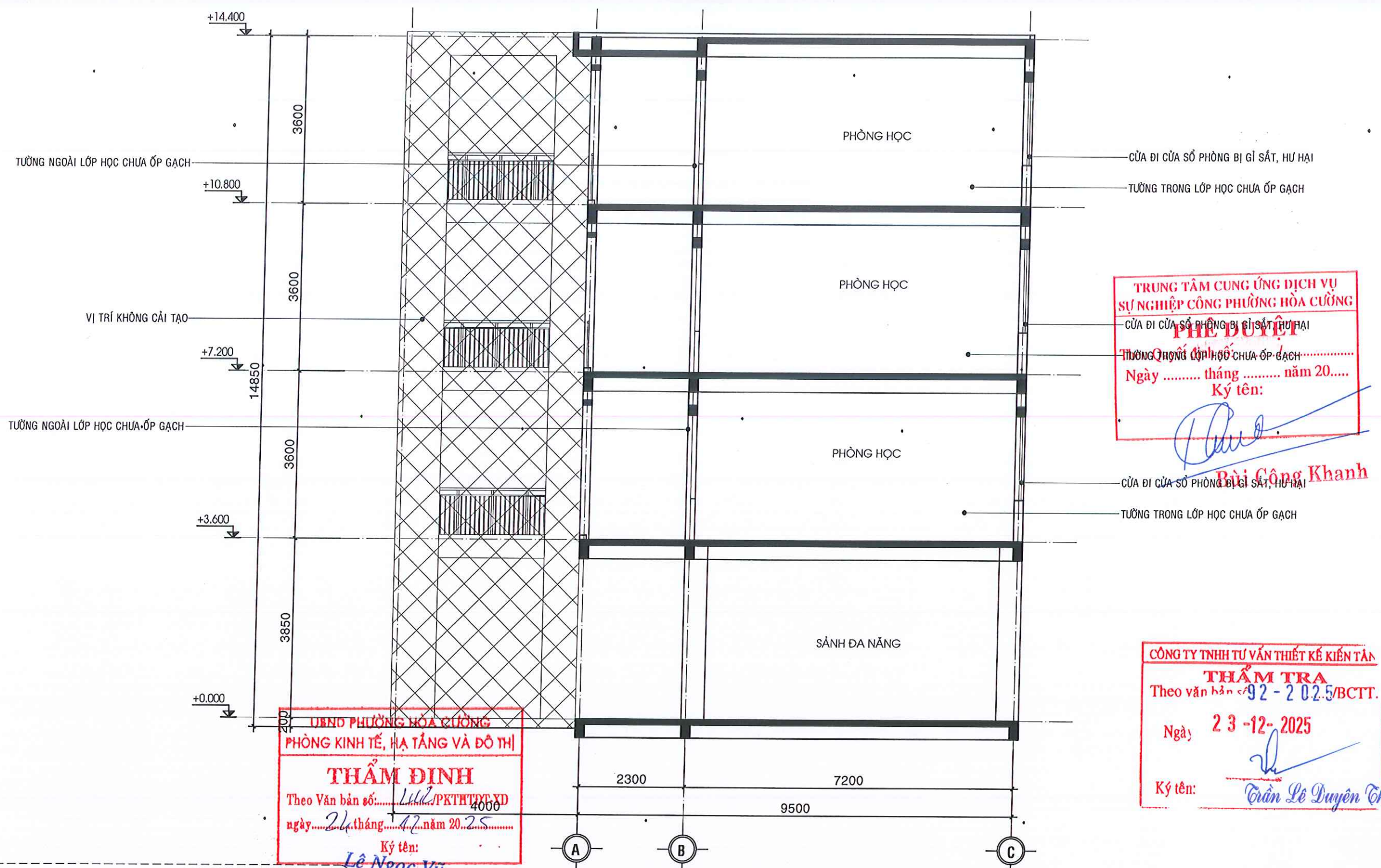
MẶT CẮT HIỆN TRẠNG - KHỐI SỐ 6
