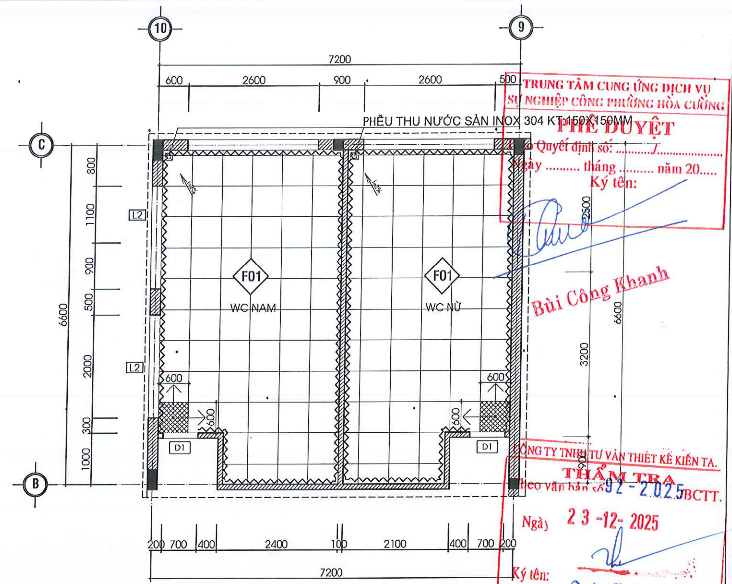
MẶT BẰNG LÁT GẠCH KHU VỆ SINH TẦNG 2
