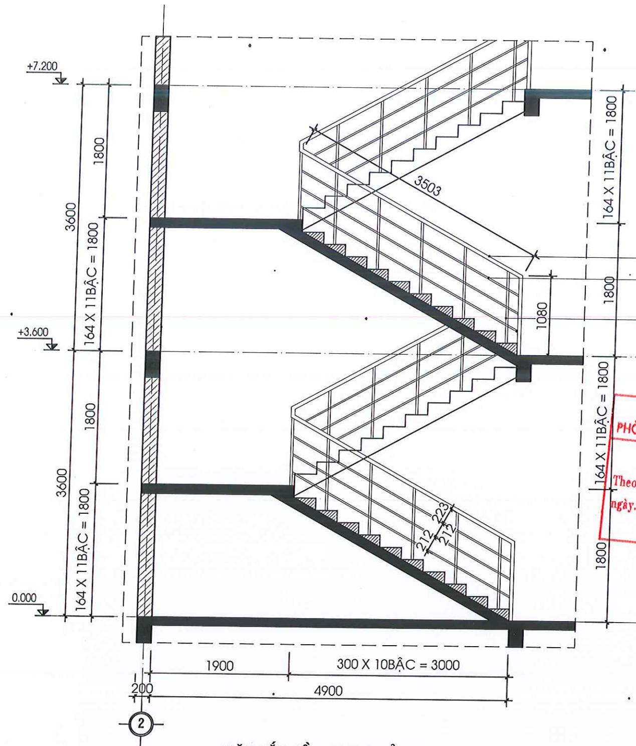
MẶT CẮT CẦU THANG CẢI TẠO
