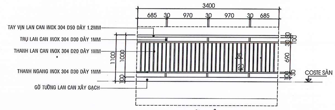
CHI TIẾT ĐIỂN HÌNH
