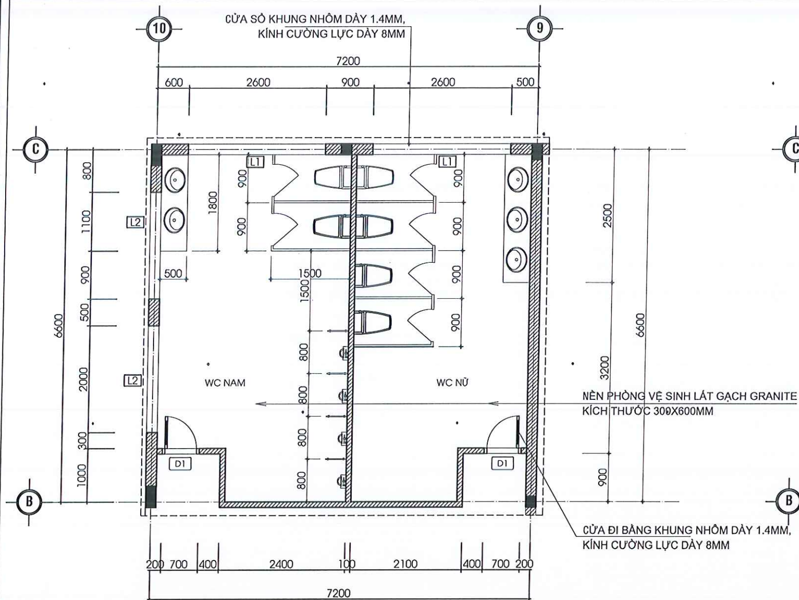
MẶT BẰNG CẢI TẠO KHU VỆ SINH TẦNG 1
