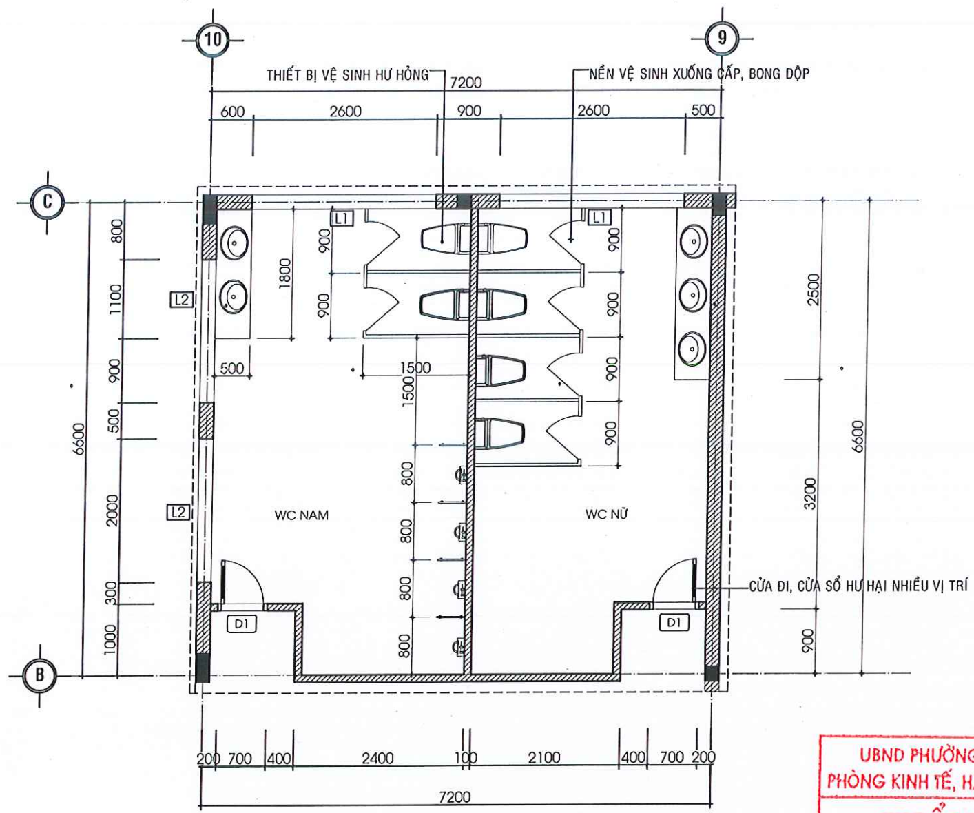
MẶT BẰNG HIỆN TRẠNG KHU VỆ SINH TẦNG 1
