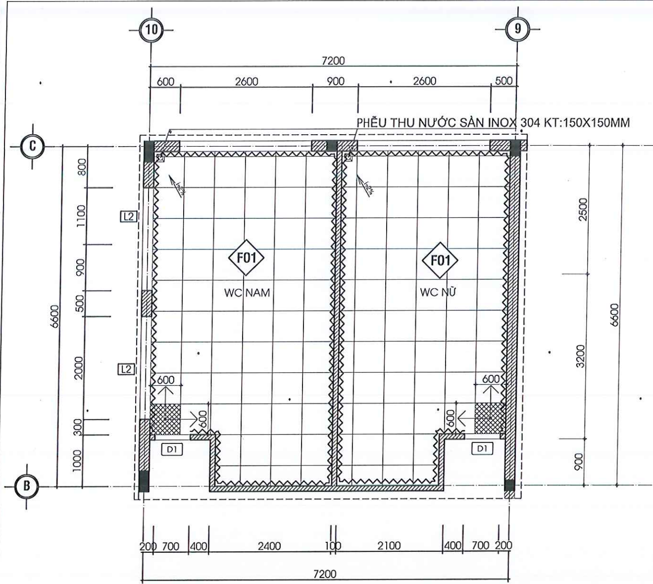
MẶT BẰNG LÁT GẠCH KHU VỆ SINH TẦNG 1
