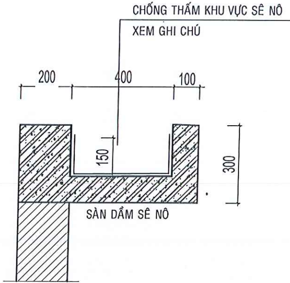
MẶT CẮT NGANG SÊ NÔ
