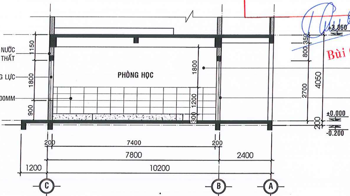
MẶT CẮT (CẢI TẠO)
