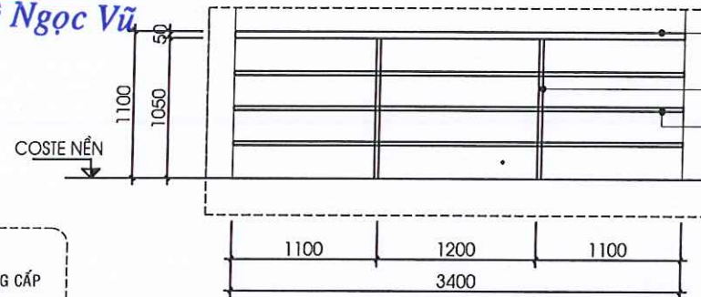
LAN CAN HÀNH LANG ĐIỂN HÌNH TẦNG 1
