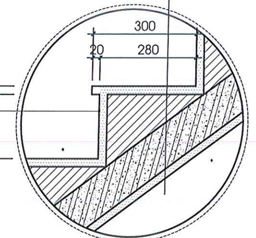
CHI TIẾT BẬC THANG
