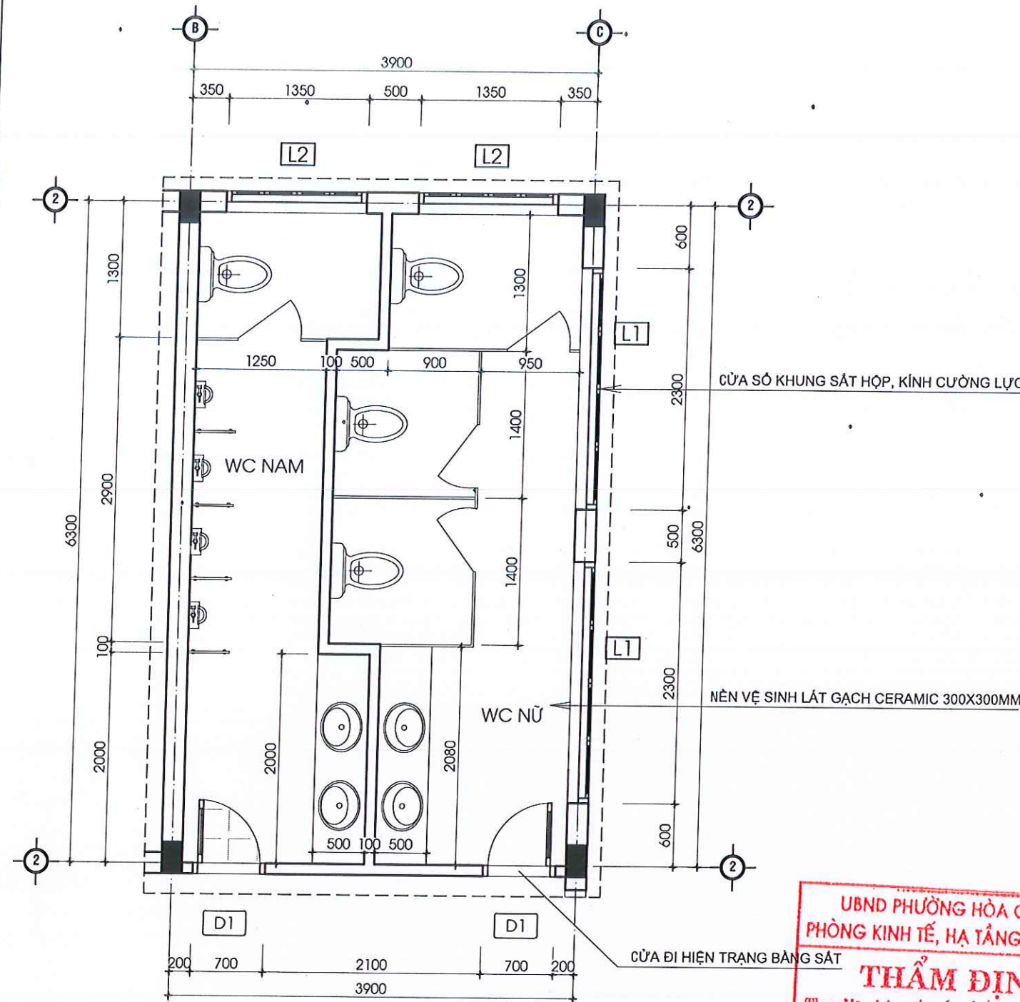
MẶT BẰNG KHU VỆ SINH TẦNG 1
