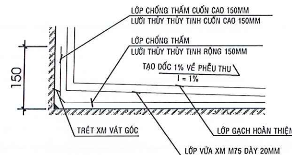
CẤU TẠO NỀN VỆ SINH
