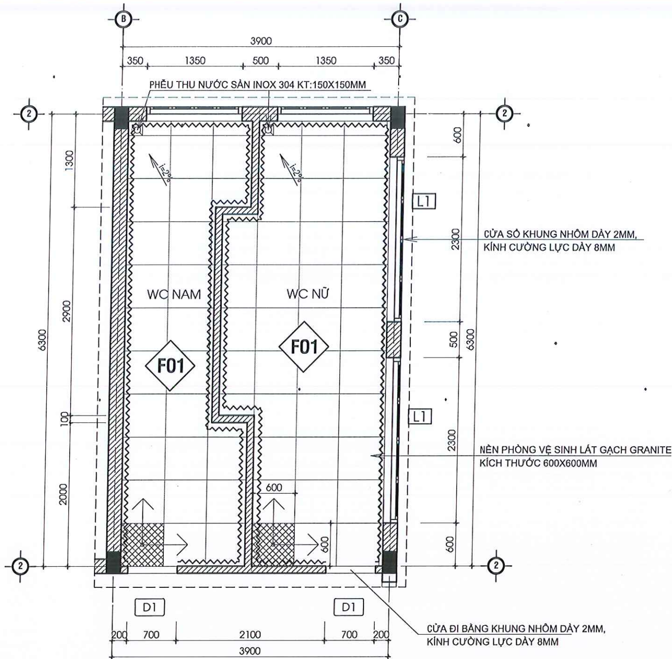
MẶT BẰNG LÁT GẠCH KHU VỆ SINH TẦNG 1
