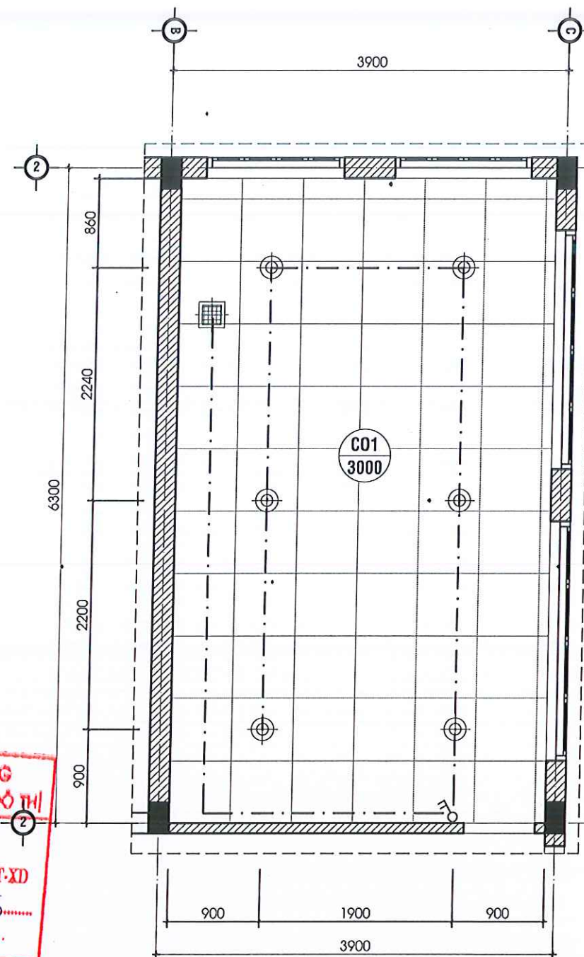
MẶT BẰNG TRẦN ĐÈN KHU VỆ SINH TẦNG 2
