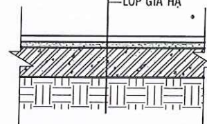
CẤU TẠO NỀN GẠCH
