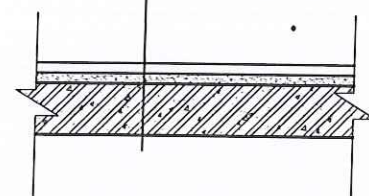
CẤU TẠO NỀN HÀNH LANG
