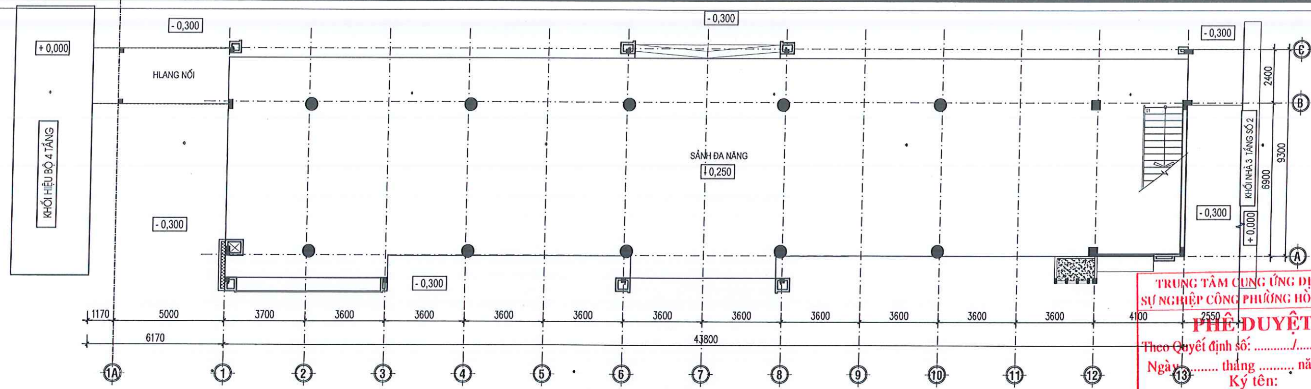
MẶT BẰNG HIỆN TRẠNG TẦNG 1
