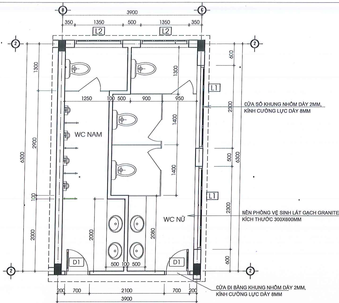
MẶT BẰNG CẢI TẠO KHU VỆ SINH TẦNG 1
