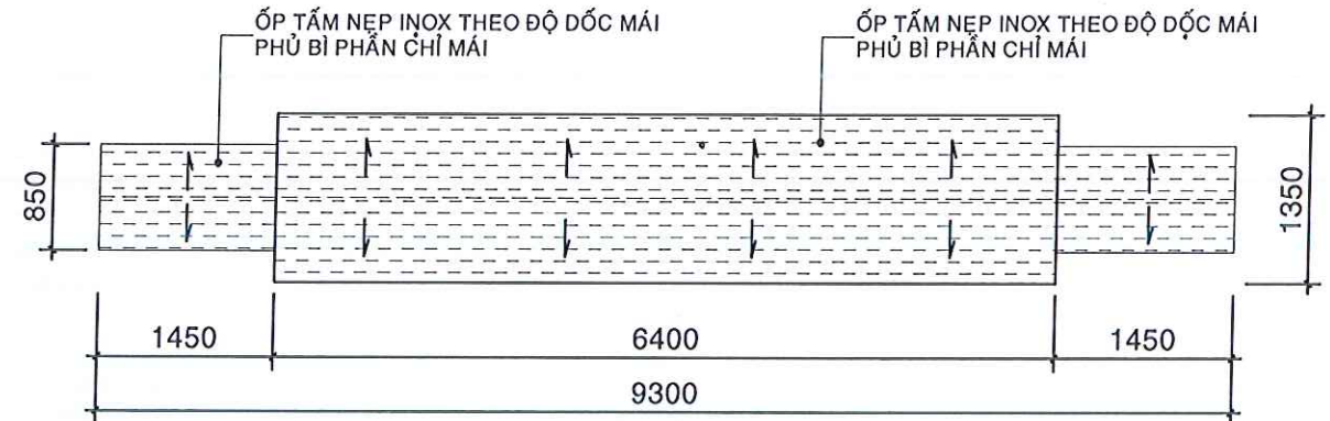
MẶT BẰNG MÁI CẢI TẠO
