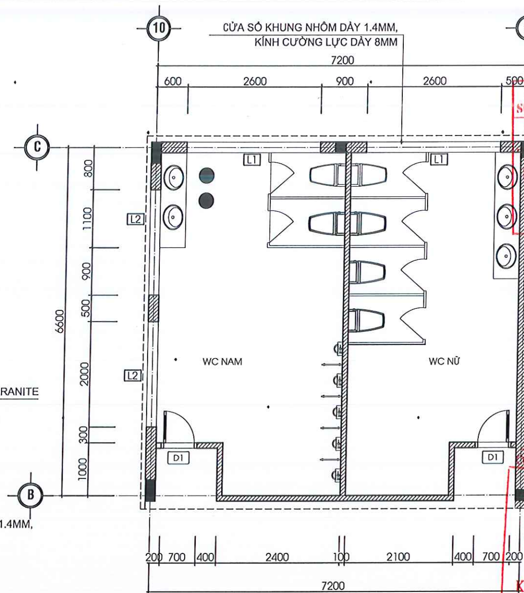
MẶT BẰNG CẢI TẠO KHU VỆ SINH TẦNG 2
