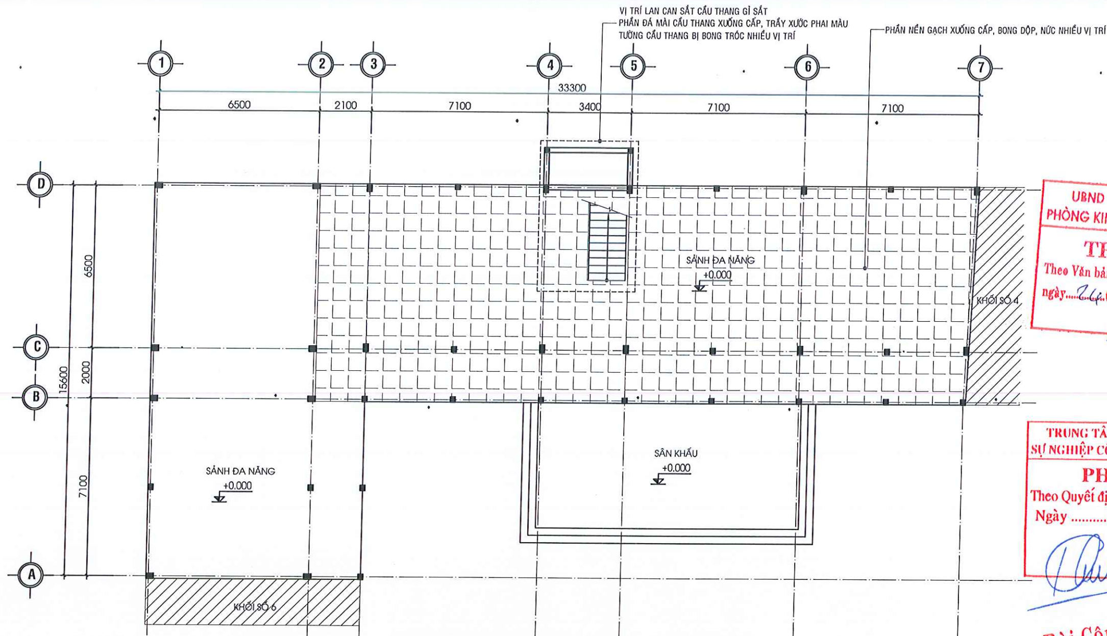
MẶT BẰNG HIỆN TRẠNG TẦNG 1 - KHỐI SỐ 5
