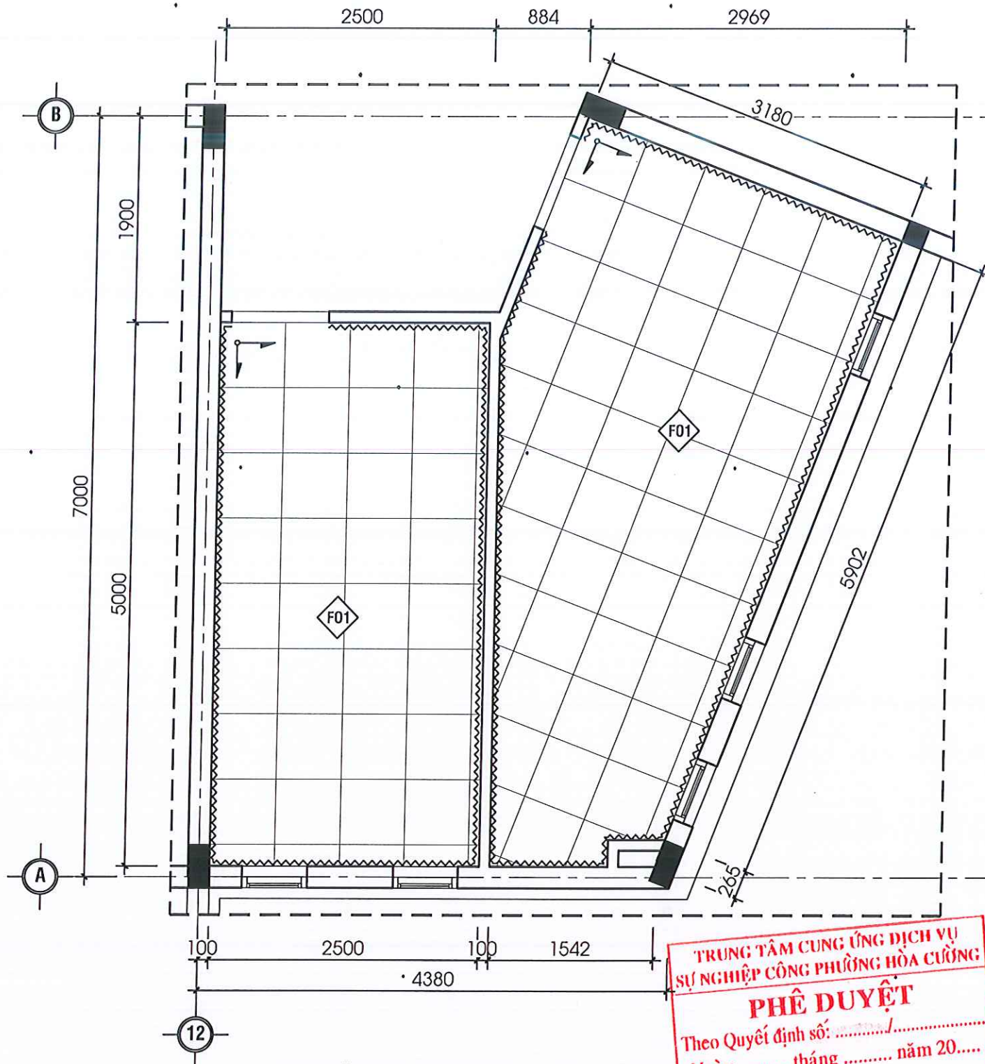
MẶT BẰNG LÁT GẠCH VỆ SINH TẦNG 2, 3
