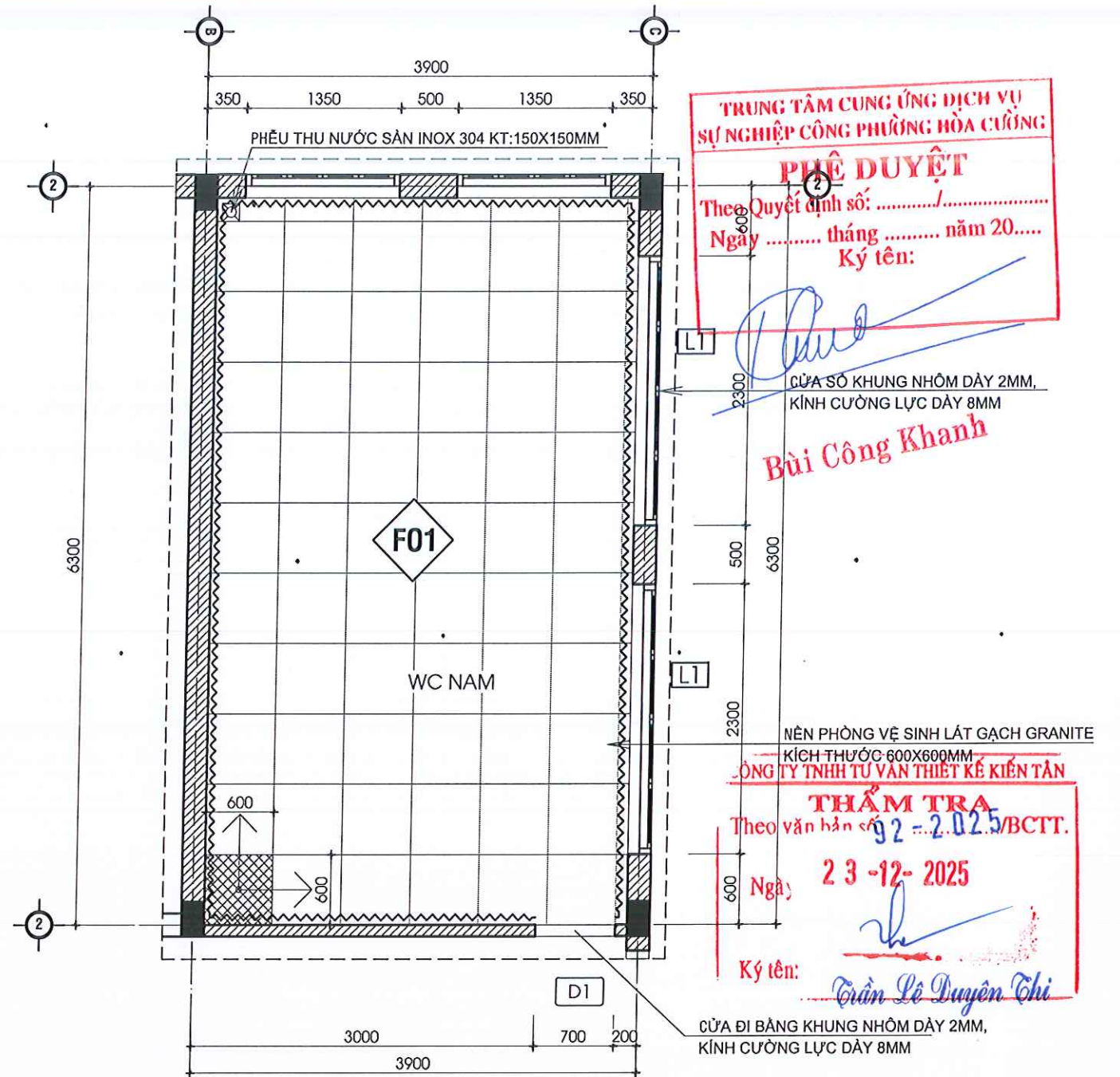
MẶT BẰNG LÁT GẠCH KHU VỆ SINH TẦNG 2
