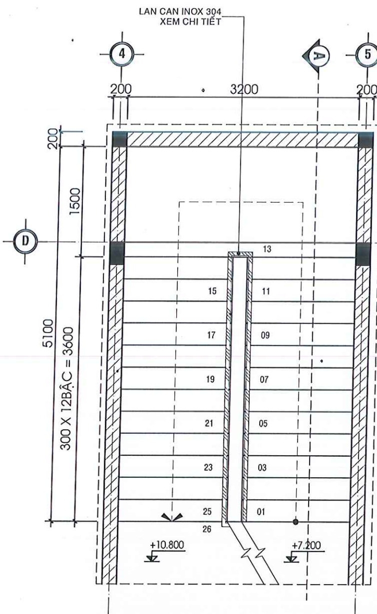
MB CẦU THANG TỪ COSTE +7.200 LÊN +10.800 (26 BẬC)
