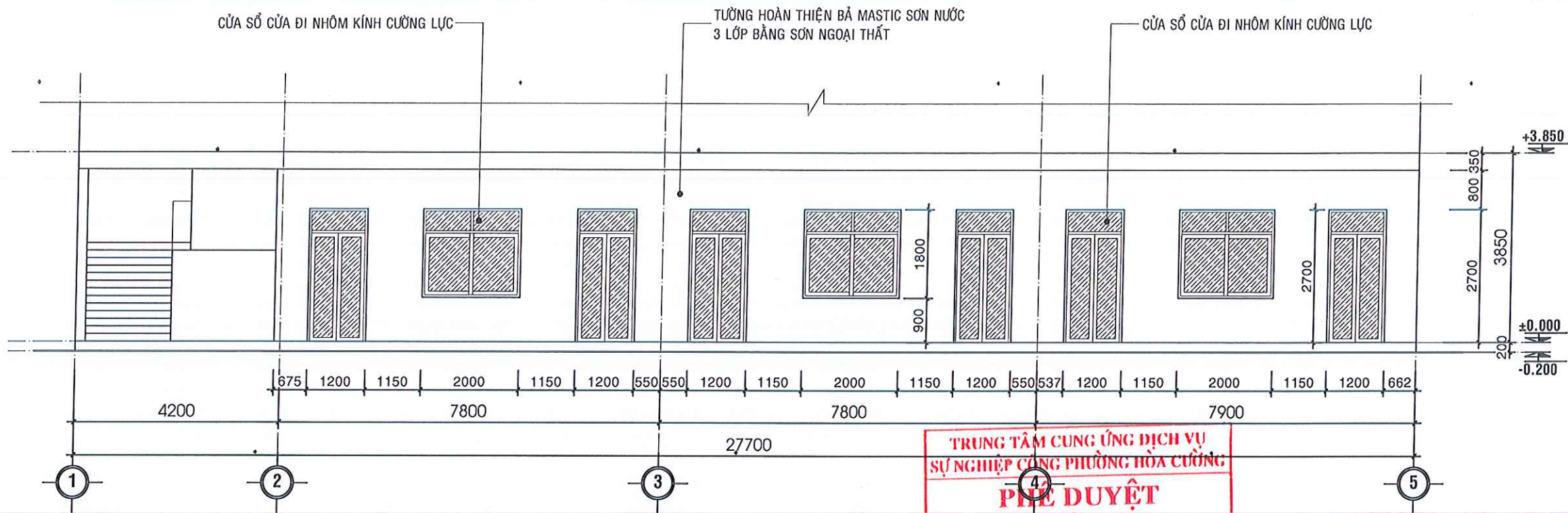
MẶT ĐỨNG 1-5 (CẢI TẠO)
