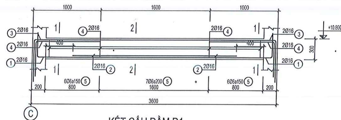
KẾT CẤU DÀM D1
