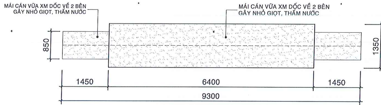
MẶT BẰNG MÁI HIỆN TRẠNG
