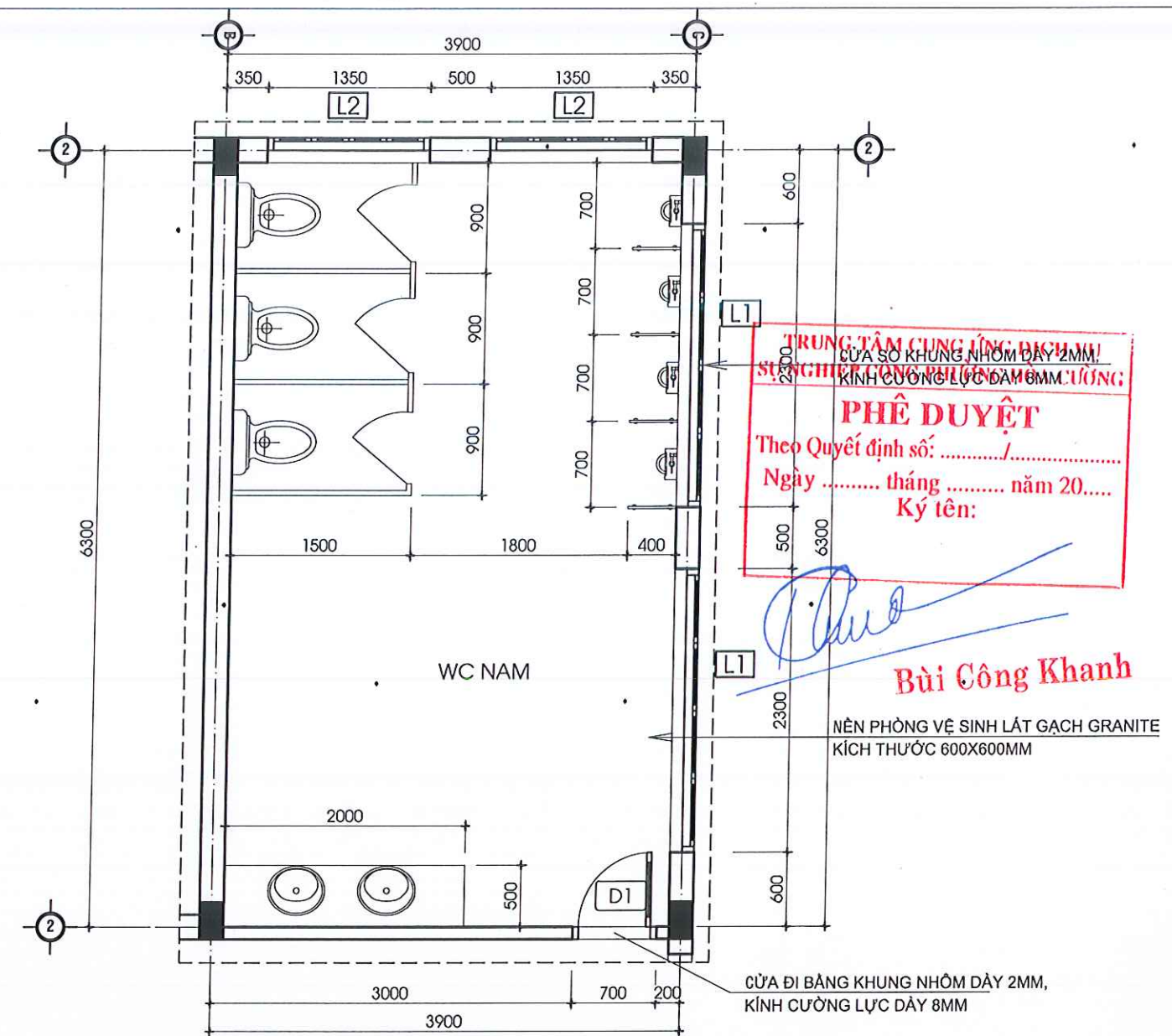
MẶT BẰNG CẢI TẠO KHU VỆ SINH TẦNG 2
