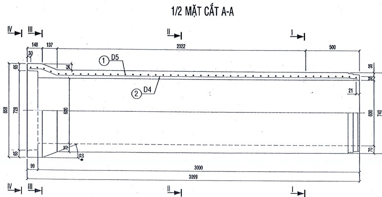
1/2 CHÍNH DIỆN
