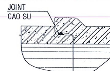
MỐI NỐI
