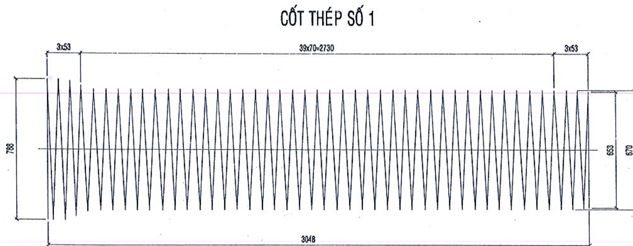
1/2 CHÍNH DIỆN
