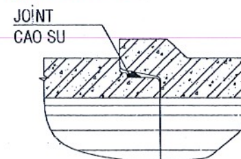
MỐI NỐI
