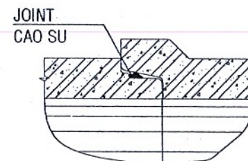
MỐI NỐI
