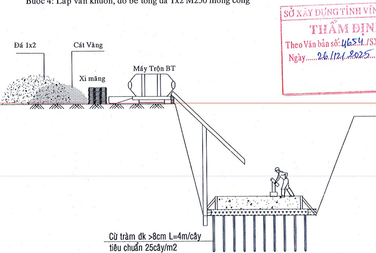
Bước 4: Lắp ván khuôn, đổ bê tông đá 1x2 M250 móng cống
