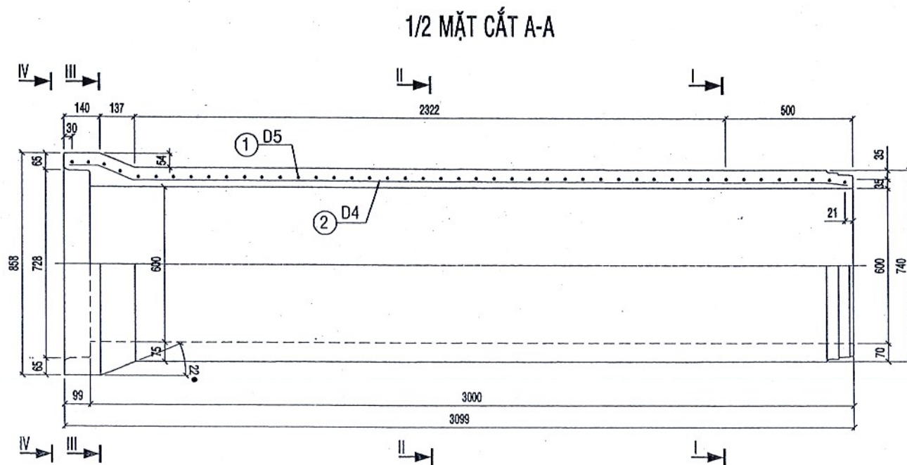
1/2 CHÍNH DIỆN
