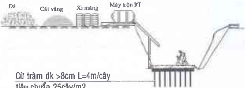
Bước 3: Đệm cát đầu cừ, lấp ván khuôn, đổ bê tông lót đá 1x2 M150
