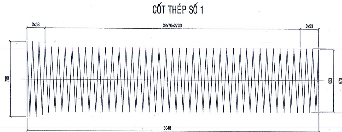
1/2 CHÍNH DIỆN
