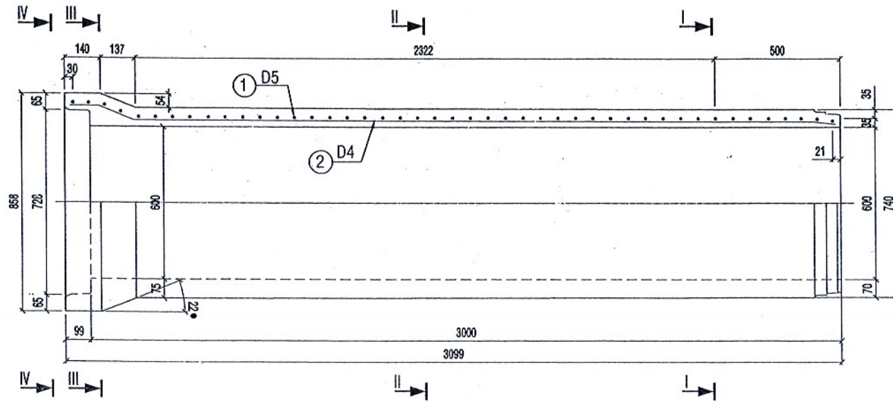
1/2 CHÍNH DIỆN
