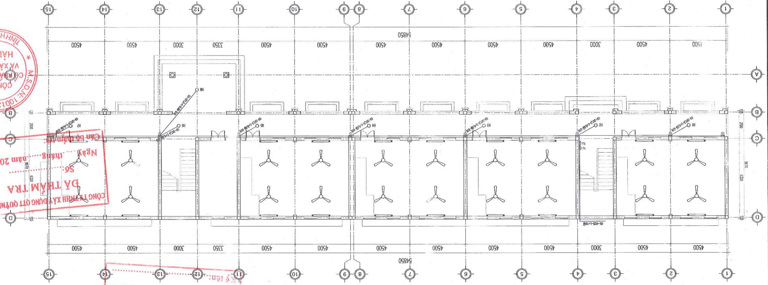
MẶT BẰNG CẤP ĐIỆN TẦNG 1
