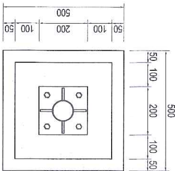
MẬT BẠNG MỘNG
