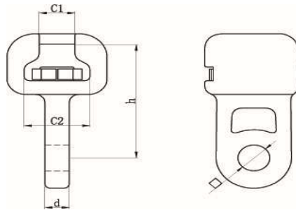
Mắt nối đơn (hình tượng trung)
