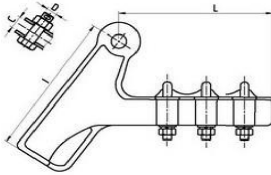
Khoá néo dây (hình tượng trung loại 3U)
