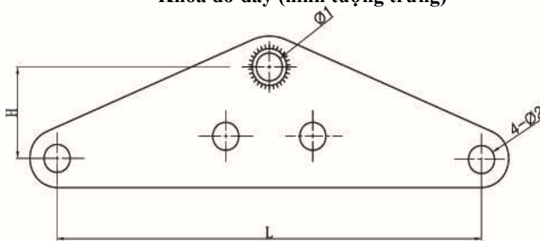
Khánh đơn (hình tượng trung)
