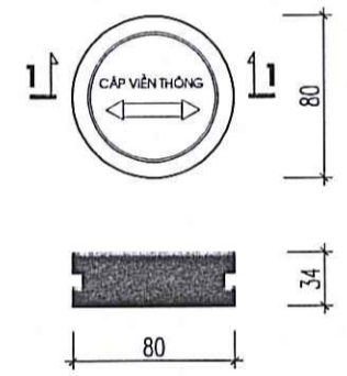
MẶT CẮT 1-1
