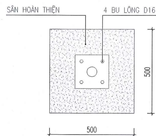
MẶT BẰNG CHÂN ĐỂ LẮP ĐẶT THIẾT BỊ (SL: 42 CÁI)
