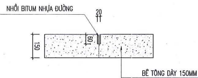
CẤU TẠO KHE CO (L=3.832M) (CỨ 5M BỐ TRÍ 1 KHE CO)
