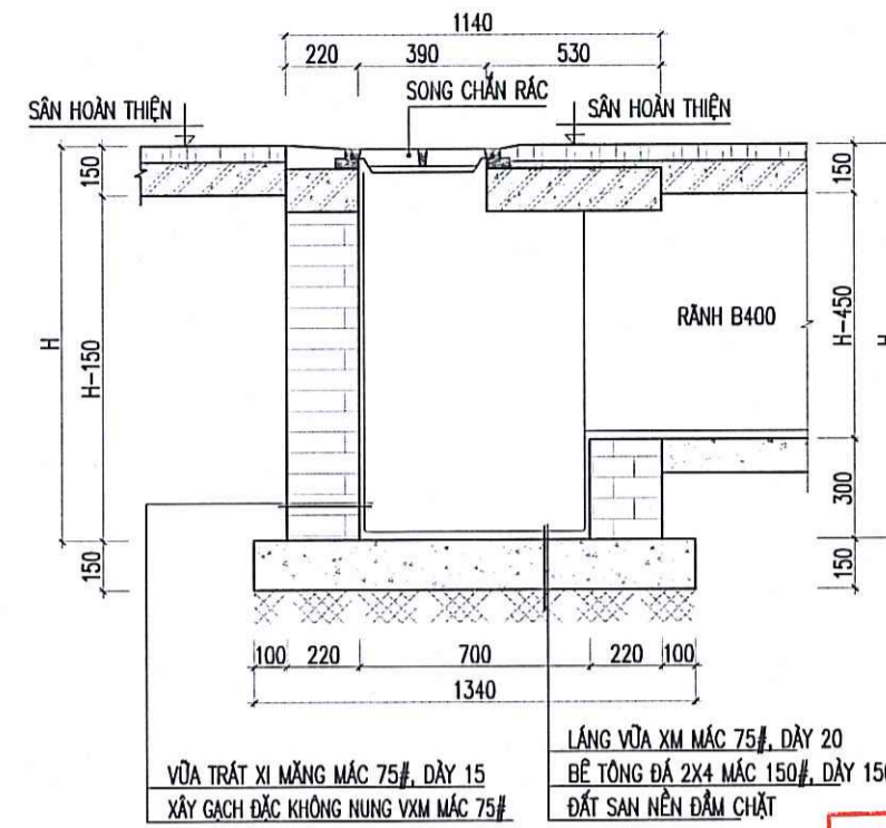
MẶT CẮT 2 - 2
