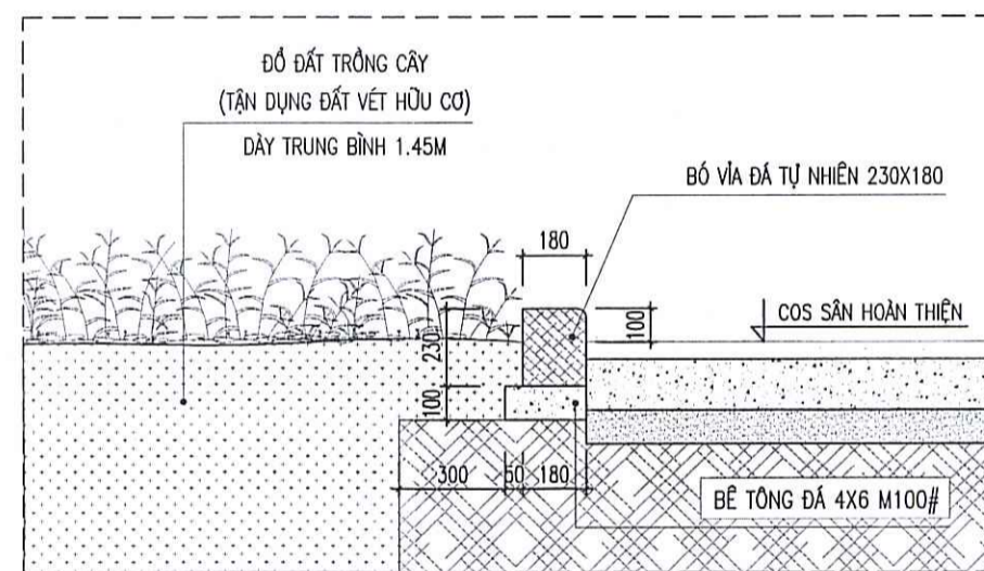
CHI TIẾT BÓ VÍA (L=1.926M)
