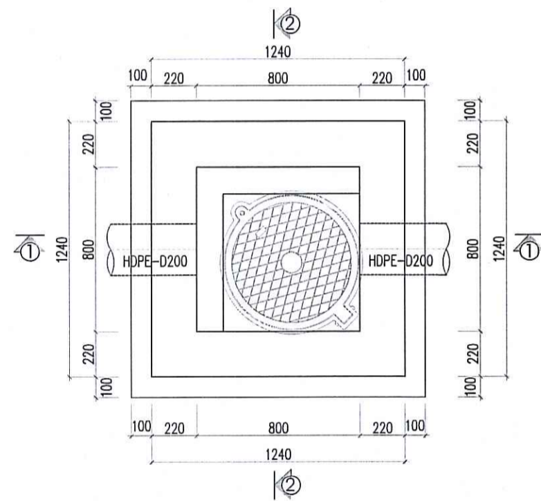
MẶT BẰNG HỒ GA THU NƯỚC THẢI LOẠI 2 (TL: 1/30) (ÁP DỤNG: T1.2, T1.3, T1.4, T1.6, T1.7, T1.8, T1.9, T1.10, T1.11, T1.12, T1.13, T2.2, T2.3, T3.2, T3.3, T3.4; SỐ LƯỢNG: 16 CÁI)
