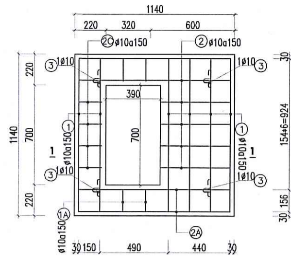
BỐ TRÍ THÉP NẮP GA (SỐ LƯỢNG: 63CÁI)
