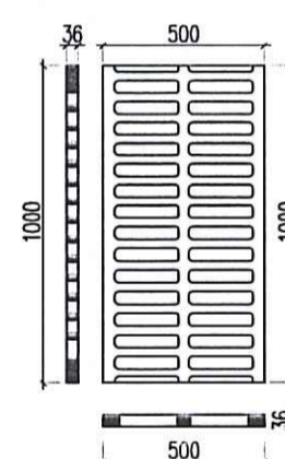
CHI TIẾT SONG CHẮN RÁC BẰNG COMPOSITE KT 1000X500 (SỐ LƯỢNG: 541 CÁI)
