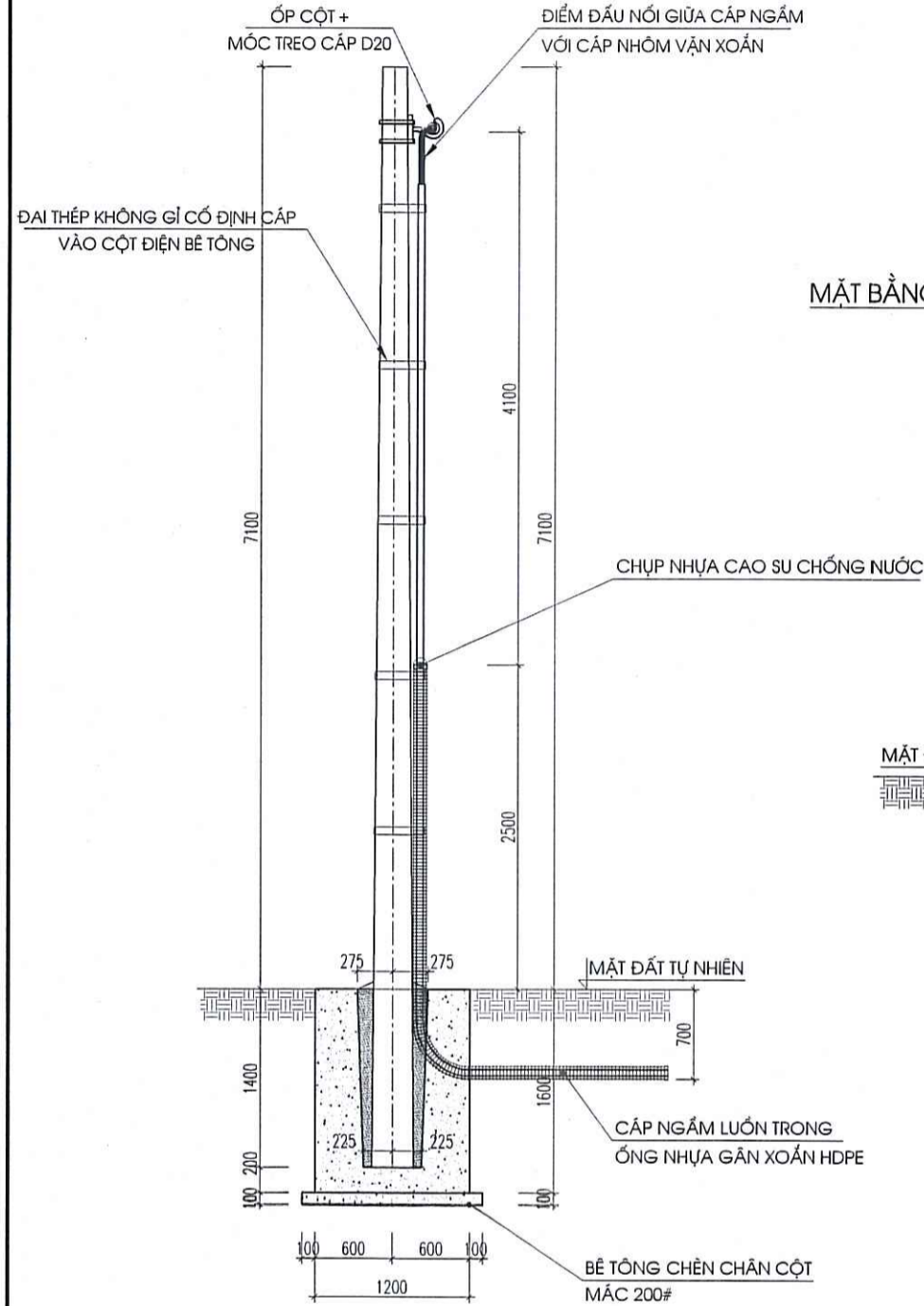
CHI TIẾT CỘT BÊ TÔNG LY TÂM 8.5M/190 (CỘT ĐƠN) TỶ LỆ: 1/40. CỘT KÝ HIỆU: CD1, CD2 (SỐ LƯỢNG: 02 CỘT ĐƠN)
