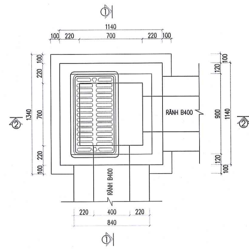
MẶT BẰNG HỔ GA LOẠI 2 (SỐ LƯỢNG: G2.3, G3.15, G4.2, G5.1, G6.2; SỐ LƯỢNG: 05 CÁI)
