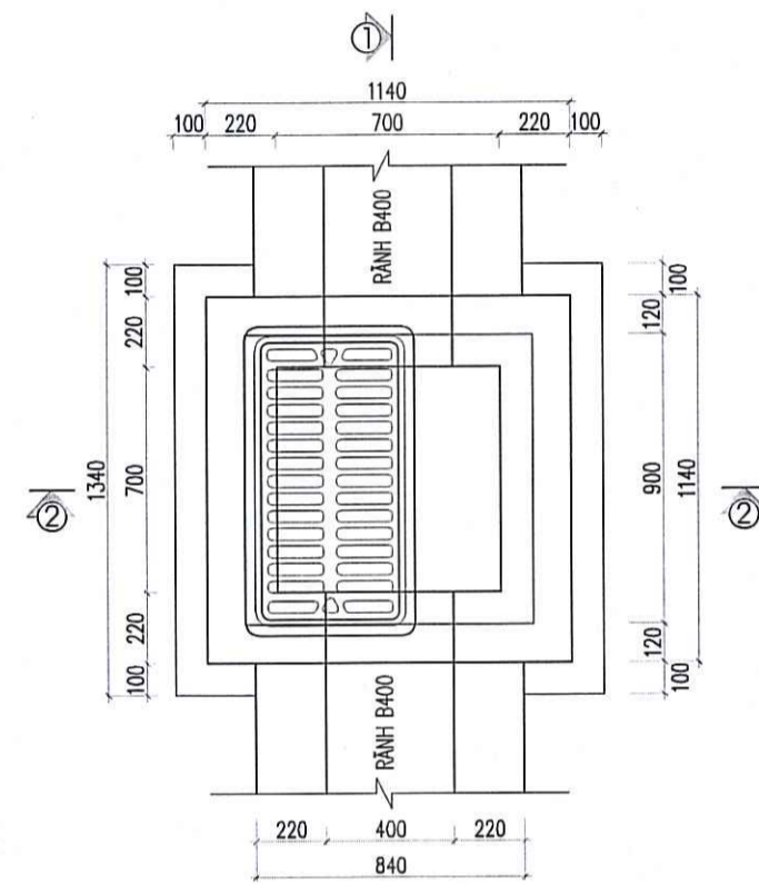
MẶT BẰNG HỔ GA LOẠI 1A (SỐ LƯỢNG: G2.1, G2A.1; SỐ LƯỢNG: 02 CÁI)
