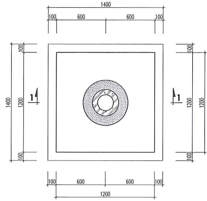
MẶT BẰNG MÓNG CỘT ĐIỆN BÊ TÔNG LY TÂM 8.5M-190 (CỘT ĐƠN) TỶ LỆ: 1/25. CỘT KÝ HIỆU: CD1, CD2 (SỐ LƯỢNG: 02 CỘT ĐƠN)
