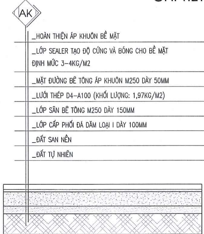
SÂN BÊ TÔNG ÁP KHUÔN (S=11.783M 2 )
