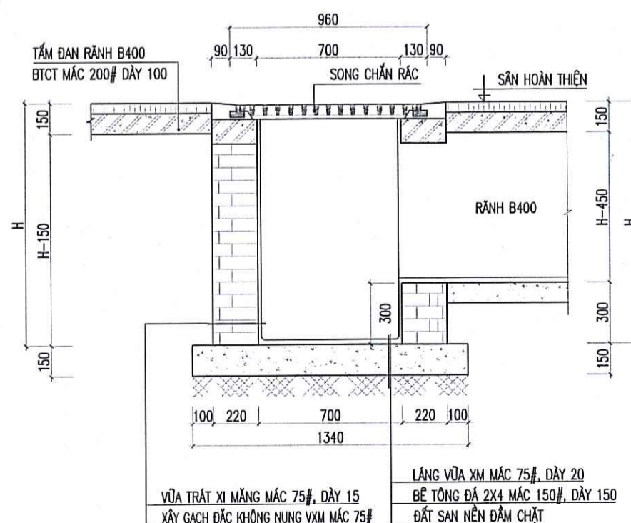
MẶT CẮT 1-1
