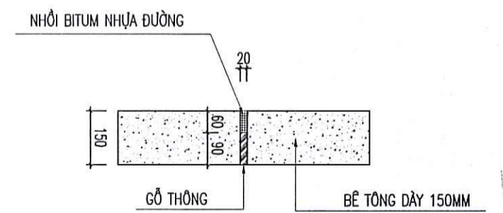
CẤU TẠO KHE GIÃN (L=676MD) (CỨ 25M BỐ TRÍ 1 KHE DẪN)
