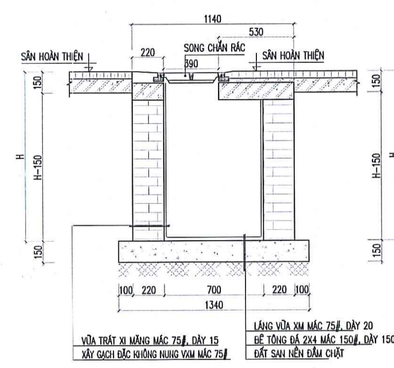
MẶT CẮT 2-2
