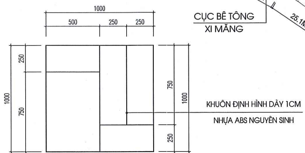
CHI TIẾT KHUÔN ĐỊNH HÌNH
