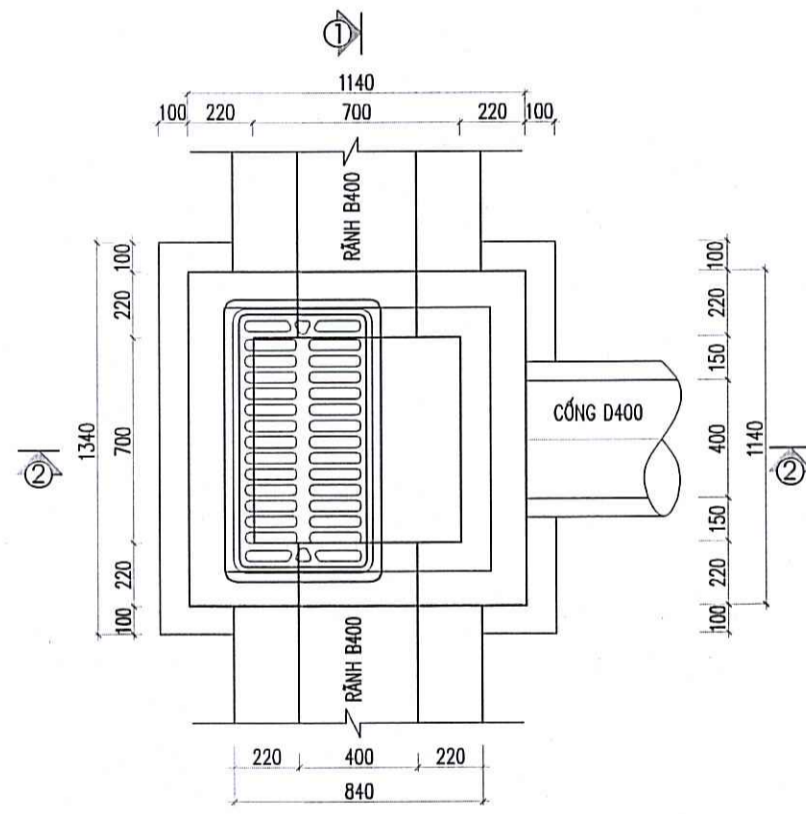
MẶT BẰNG HỐ GA LOẠI 4
