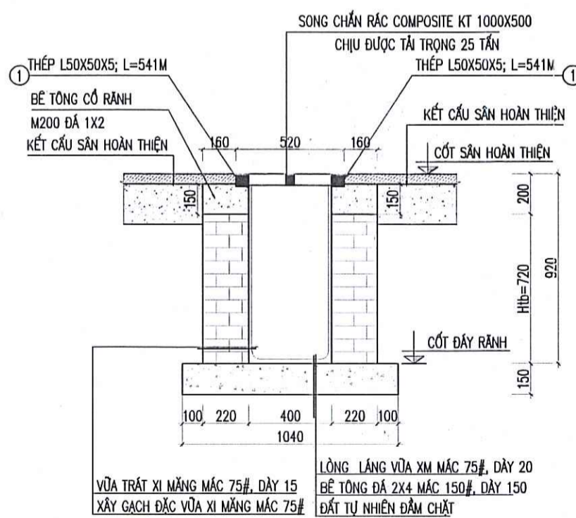
MẶT CẮT RÀNH B400 ĐIỂN HÌNH CÓ SONG CHẮN RÁC COMPOSITE QUÁ SÀN LÀM MỚI
