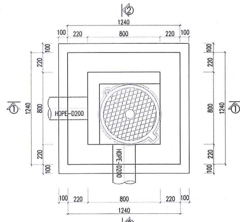
MẶT BẰNG HỒ GA THU NƯỚC THẢI LOẠI 3 (TL: 1/30) (ÁP DỤNG: T1.14, T3.5; SỐ LƯỢNG: 02 CÁI)
