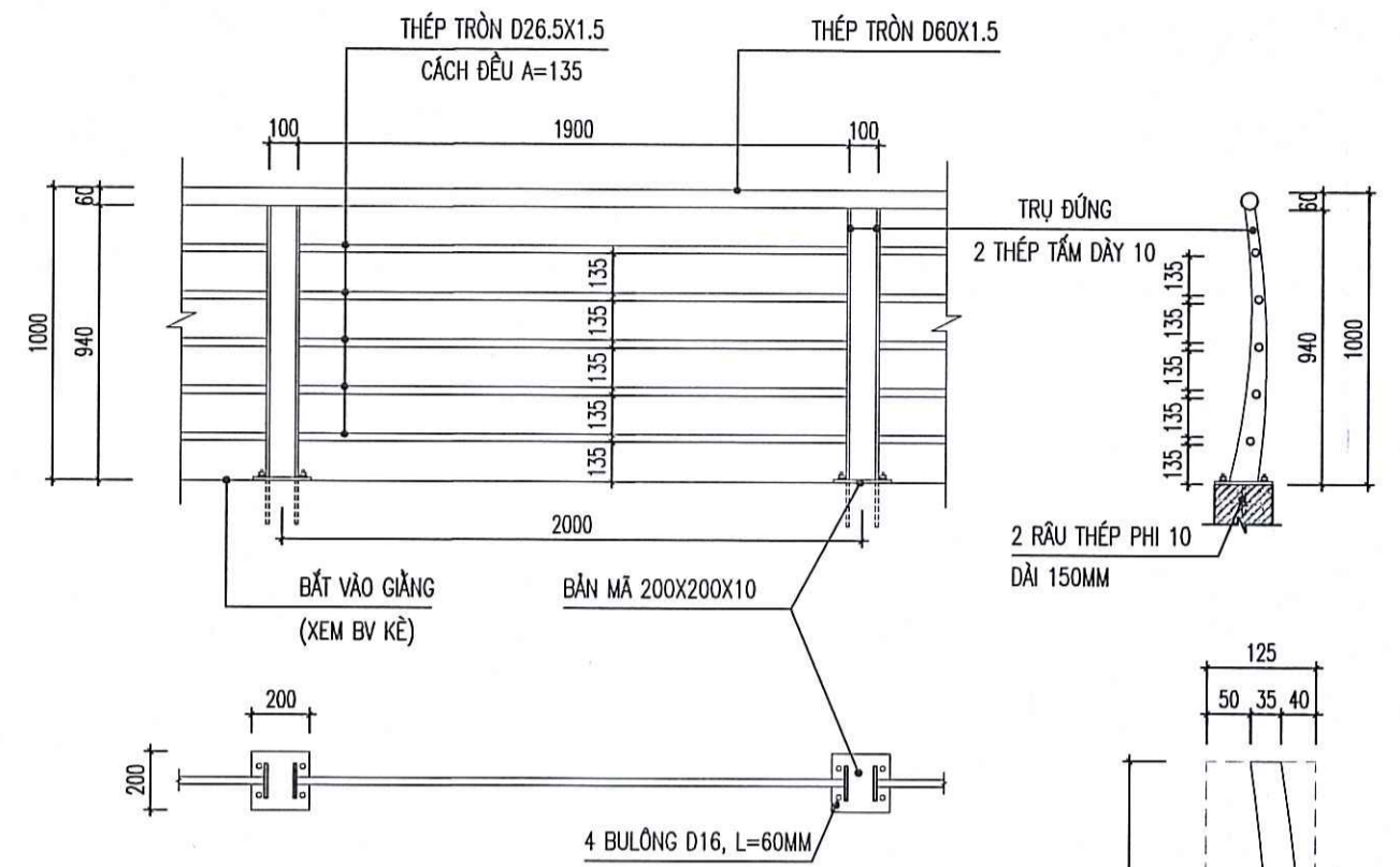
CHI TIẾT LAN CAN QUANH HỒ (L=426M) (TOÀN BỘ THÉP SƠN TÍNH ĐIỆN MÀU GHI)
