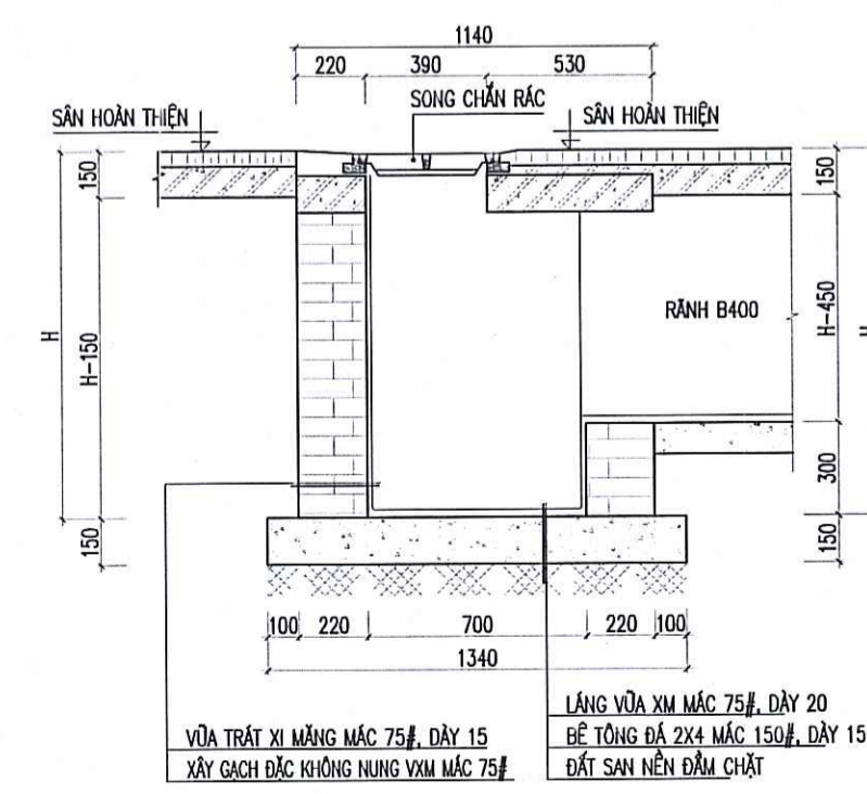
MẶT CẮT 2-2
