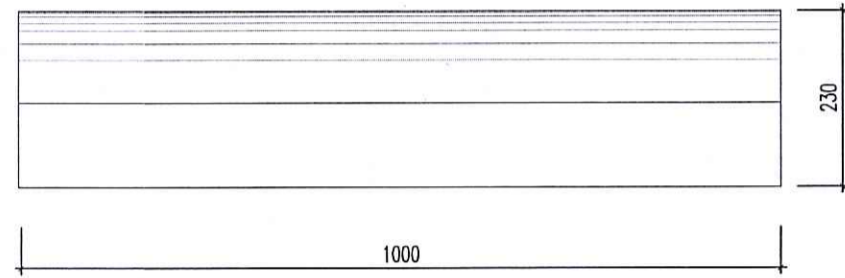
CHI TIẾT CỤC BÊ TÔNG XI MĂNG (SỐ LƯỢNG: 138 CỤC)
