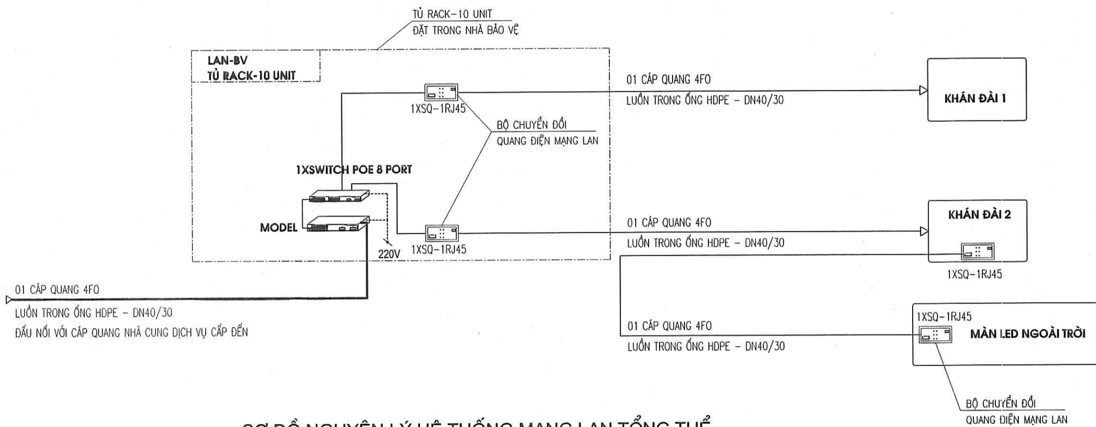
SƠ ĐỒ NGUYÊN LÝ HỆ THỐNG MẠNG LAN TỔNG THỂ
