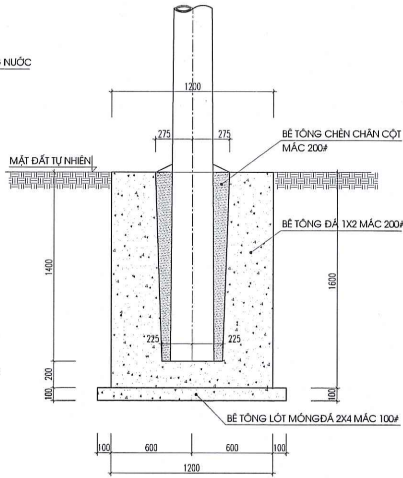
MẶT CẮT 1-1 (TỶ LỆ: 1/25)
