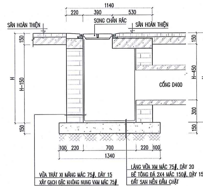
MẶT CẮT 2 - 2
