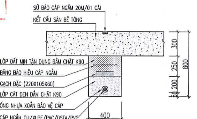
MẶT CẮT RĀNH ĐẶT CÁP CHIẾU SÁNG ĐI QUA SÂN BÊ TÔNG (TL:1/25) (BẢNG KẾ KHAI VẬT LIỆU TÍNH CHO 1M DÀI) BĂNG BẢO HIỆU CÁP RỘNG 0.3M : 1.0M KHỐI LƯỢNG ĐẤT ĐÁO : 0.20M3 CÁT ĐEN ĐÁM CHẶT K90 : 0.10M3 GẠCH ĐẶC KHÔNG NUNG : 9 VIÊN TỔNG CHIỀU DÀI TUYẾN RĀNH : 591.0M
