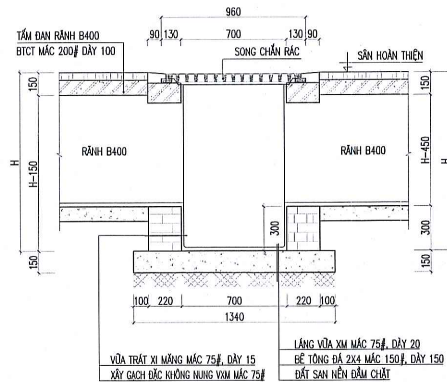
MẶT CẮT 1 - 1
