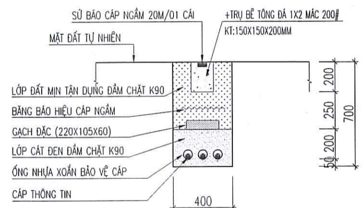
MẶT CẮT RÃNH CÁP THÔNG TIN ĐI QUA BỒN HOA (TL:1/25) (BẢNG KÊ KHAI VẬT LIỆU TÍNH CHO 1M DÀI) BẢNG BẢO HIỆU CÁP RỘNG 0.3M : 1,0M KHỐI LƯỢNG ĐẤT ĐÀO : 0.28M 3 CÁT ĐEN ĐẦM CHẶT K90 : 0.10M 3 GẠCH ĐẶC KHÔNG NUNG : 9 VIÊN TỔNG CHIỀU DÀI TUYẾN RÃNH : 77.0M
