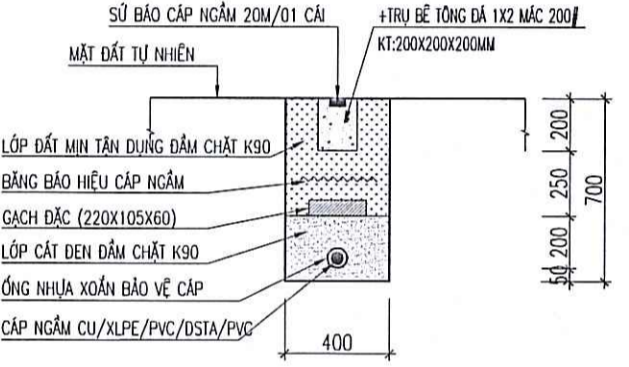
MẶT CẮT RĀNH ĐẶT CÁP CHIẾU SÁNG ĐI QUA BỐN HOA (TL:1/25) (BẢNG KẾ KHAI VẬT LIỆU TÍNH CHO 1M DÀI) BĂNG BẢO HIỆU CÁP RỘNG 0.3M : 1.0M KHỐI LƯỢNG ĐẤT ĐÁO : 0.28M3 CÁT ĐEN ĐÁM CHẶT K90 : 0.10M3 GẠCH ĐẶC KHÔNG NUNG : 9 VIÊN TỔNG CHIỀU DÀI TUYẾN RĀNH : 1157.0M
