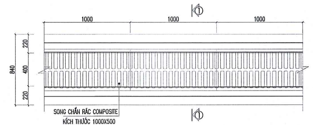
MẶT BẰNG RÀNH THOÁT NƯỚC B400 CÓ SONG CHẮN RÁC BẰNG COMPOSITE (KHỐI LƯỢNG: 541 M)
