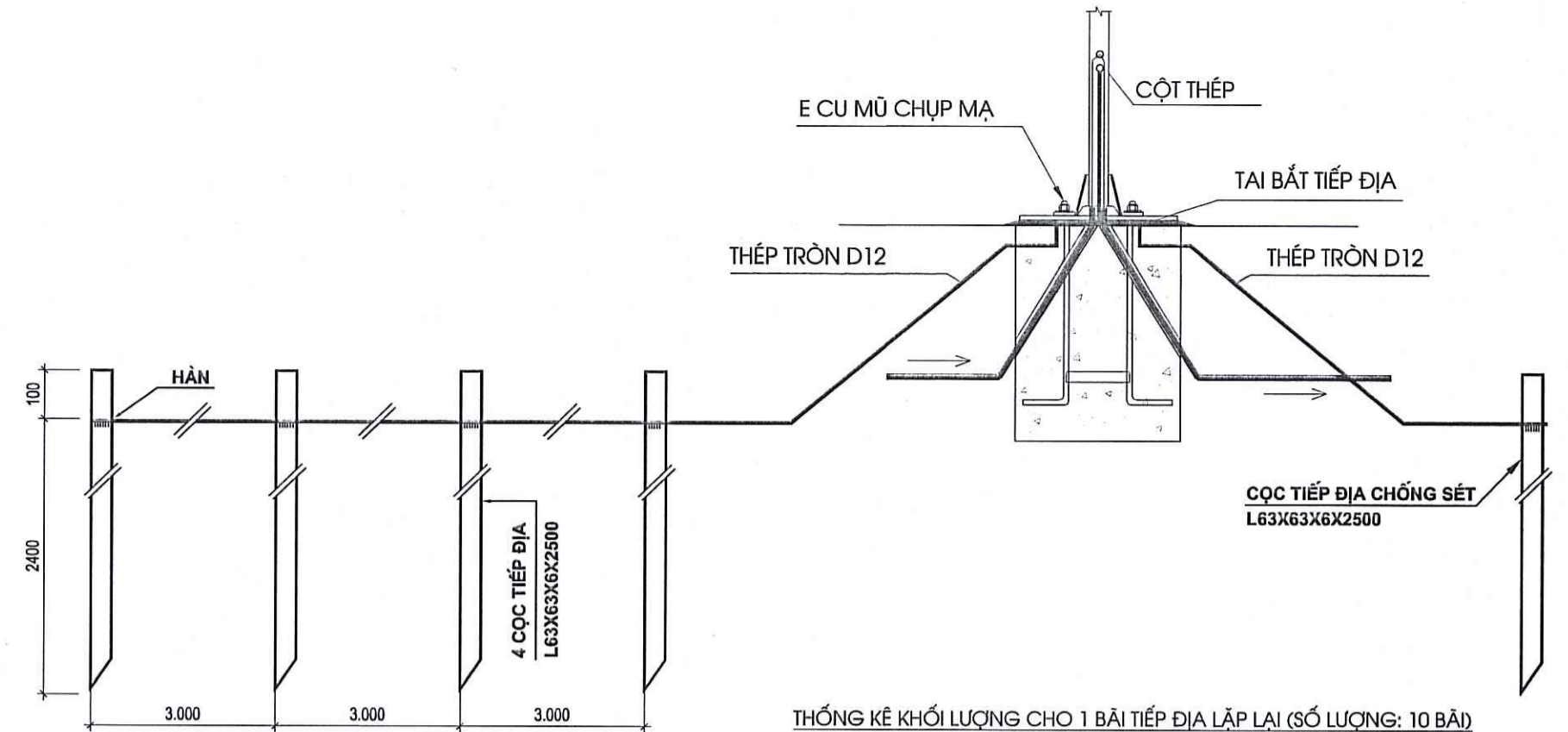
THỐNG KÊ KHỐI LƯỢNG CHO 1 BÀI TIẾP ĐẤT LẬP LẠI (SỐ LƯỢNG: 10 BÀI)
