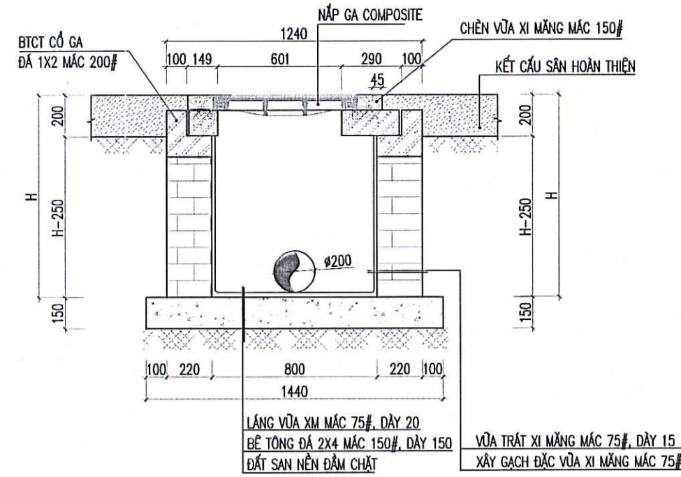
MẶT CẮT 2 - 2 (TL: 1/30)
