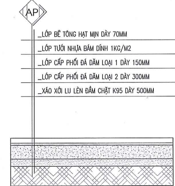
MC ĐƯỜNG BÊ TÔNG NHỰA ASPHALT KHU VỰC CỔNG (S=1.272M 2 )
