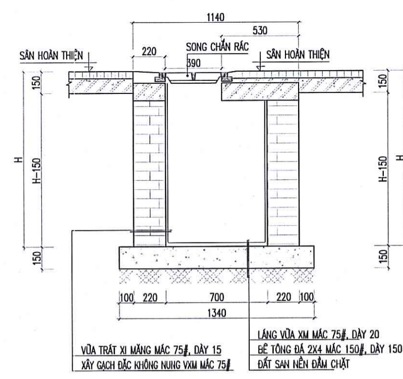
MẶT CẮT 2-2
