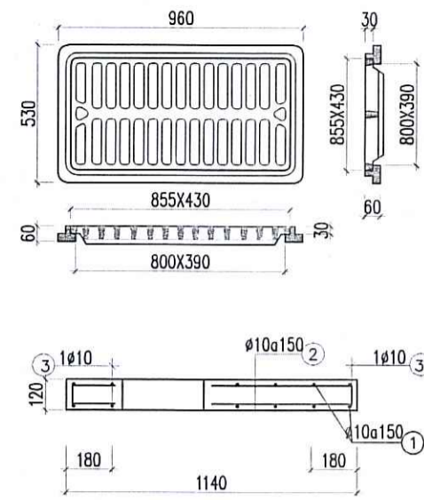
MẶT CẮT 1-1
