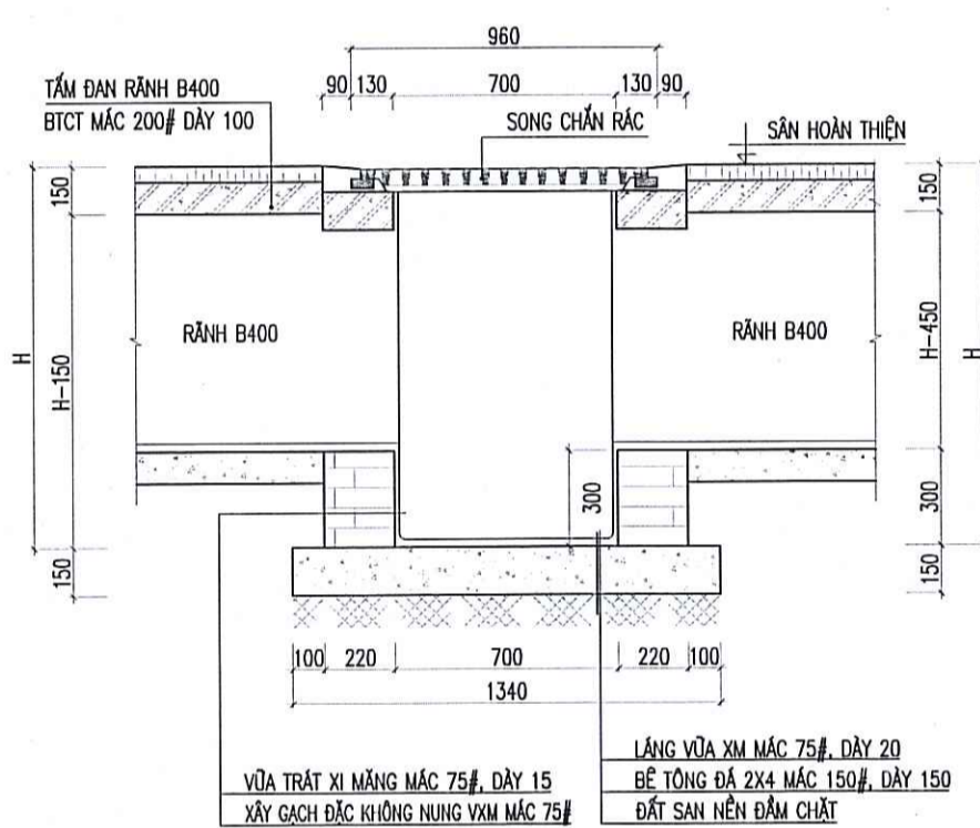
MẶT CẮT 1-1
