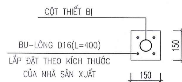
CHI TIẾT BẢN MÃ
