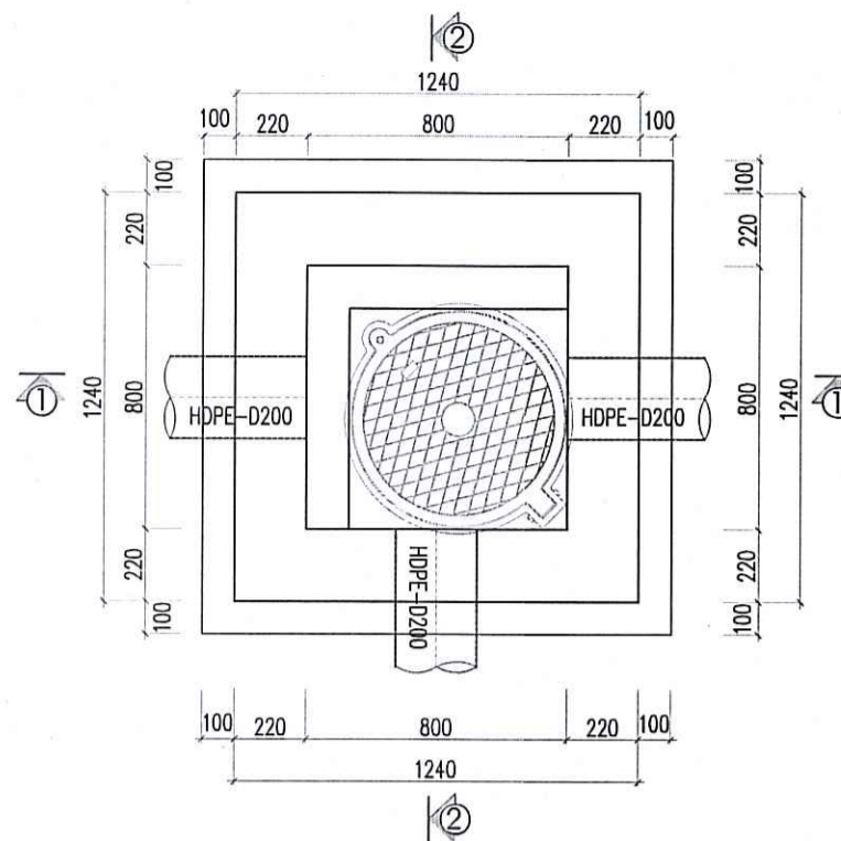
MẶT BẰNG HỒ GA THU NƯỚC THẢI LOẠI 4 (TL: 1/30) (ÁP DỤNG: T1.5; SỐ LƯỢNG: 01 CÁ)
