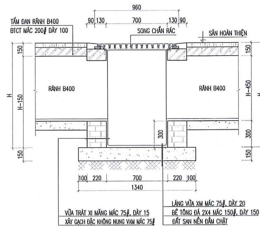
MẶT CẮT 1 - 1
