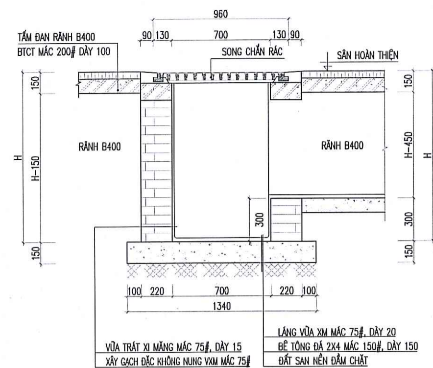
MẶT CẮT 1-1
