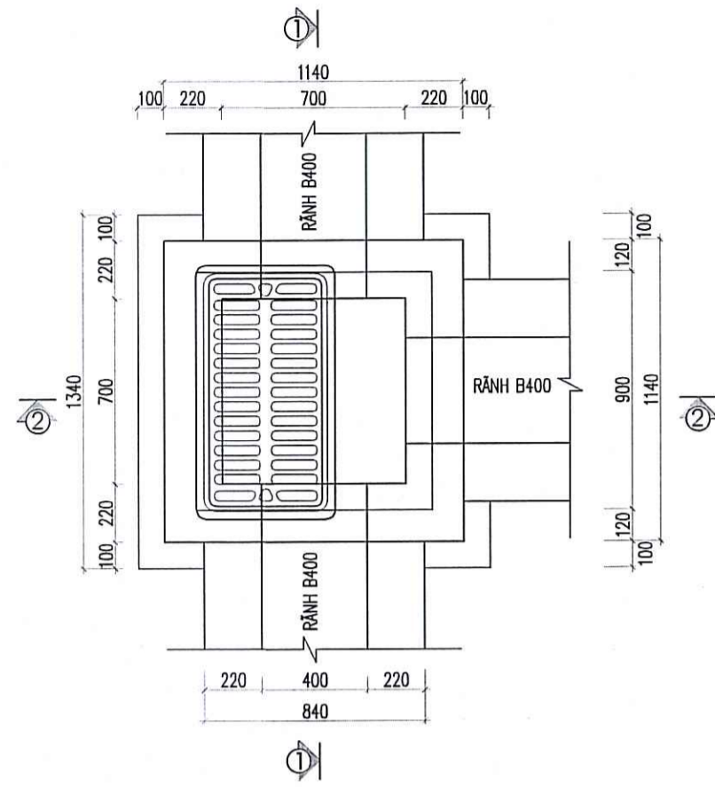
MẶT BẰNG HỐ GA LOẠI 3
