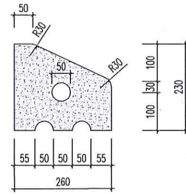
MẶT CẮT
