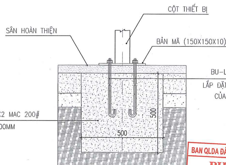
MẶT CẮT
