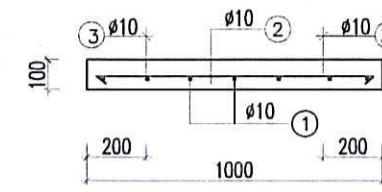
THỐNG KÊ THÉP NẤP ĐẠN CHO 1M DÀI RÀNH B400
