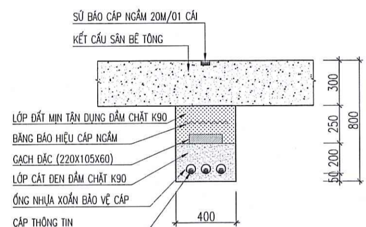
MẶT CẮT RÃNH CÁP THÔNG TIN ĐI QUA SÂN BÊ TÔNG (TL:1/25) (BẢNG KÊ KHAI VẬT LIỆU TÍNH CHO 1M DÀI) BẢNG BẢO HIỆU CÁP RỘNG 0.3M : 1,0M KHỐI LƯỢNG ĐẤT ĐÀO : 0.20M 3 CÁT ĐEN ĐẦM CHẶT K90 : 0.10M 3 GẠCH ĐẶC KHÔNG NUNG : 9 VIÊN TỔNG CHIỀU DÀI TUYẾN RÃNH : 308.0M
