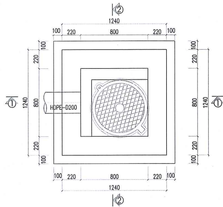
MẶT BẰNG HỒ GA THU NƯỚC THẢI LOẠI 1 (TL: 1/30) (ÁP DỤNG: T1.1, T2.1, T3.1; ; SỐ LƯỢNG: 03 CÁI)
