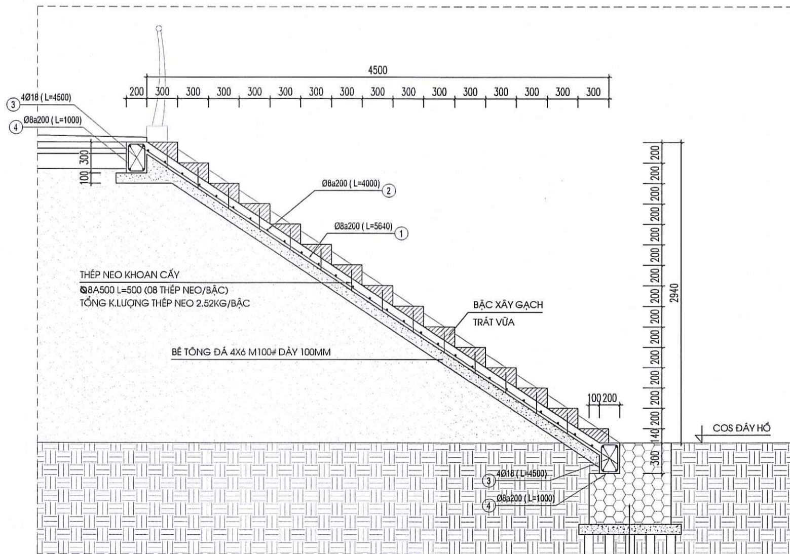
MẶT CẮT VỊ TRÍ LỐI LÊN XUỐNG (KHỐI LƯỢNG THÉP Ø8 = 246.1KG; THÉP Ø18= 70.6KG)
