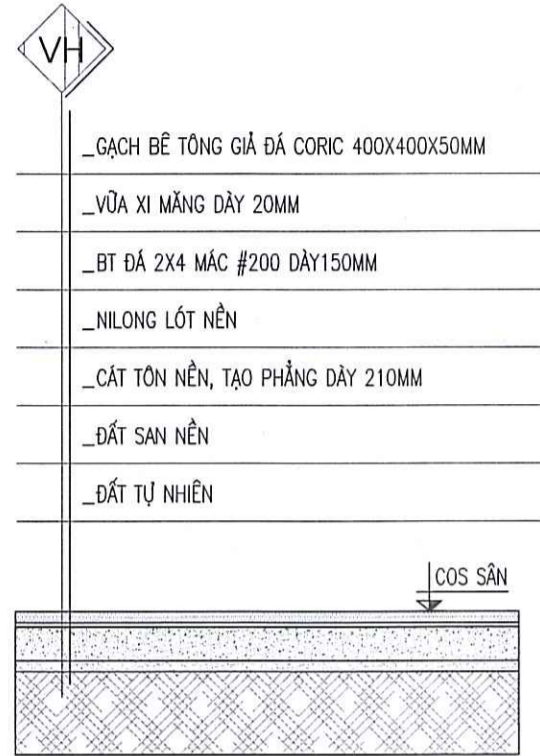
MẶT CẮT VÍA HÈ (S=1.850M 2 )
