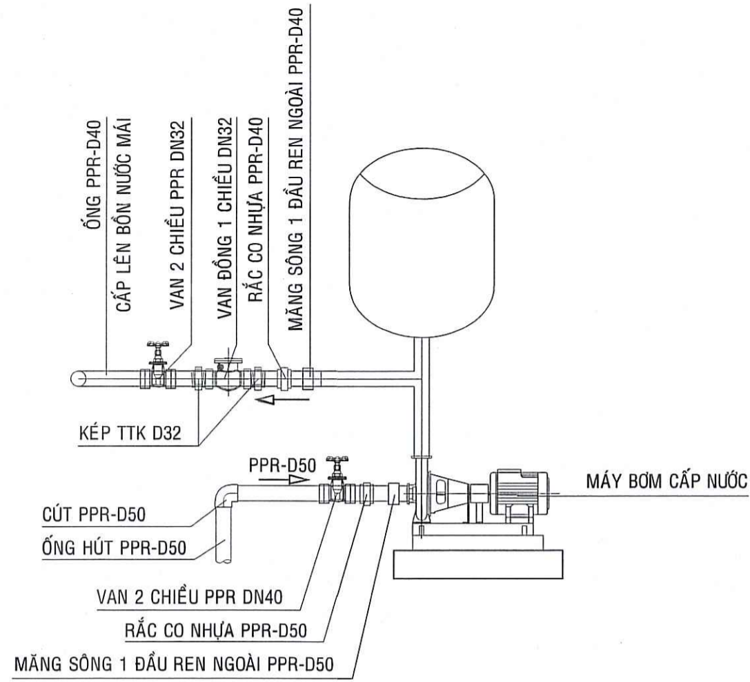
CHI TIẾT LẮP ĐẶT MÁY BƠM NƯỚC SINH HOẠT
