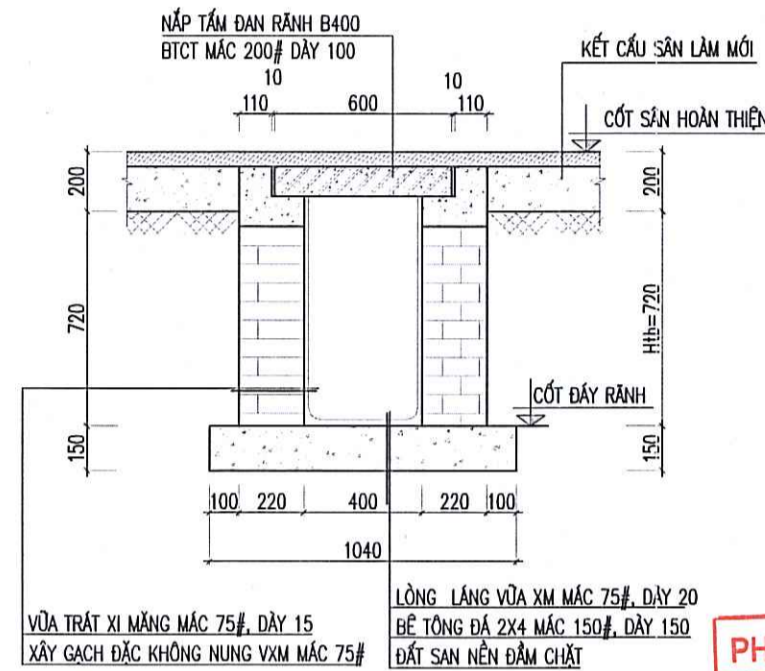
MẶT CẮT 1-1 MẶT CẮT RÀNH B400 LÀM MỚI
