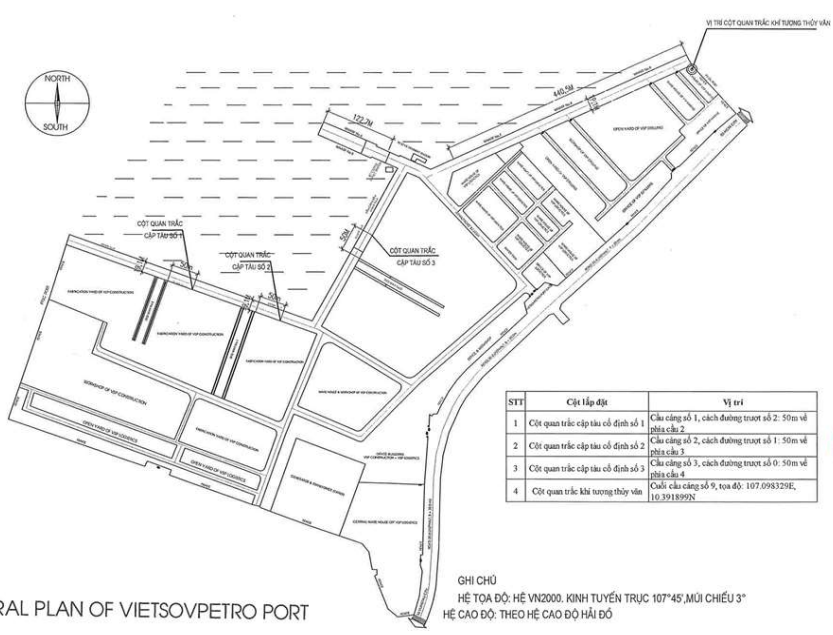
SƠ ĐỒ VỊ TRÍ LẮP ĐẶT THIẾT BỊ QUAN TRẮC
