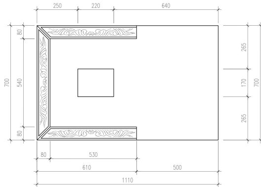
MẶT BỀ MẶT NẮP MỘ
