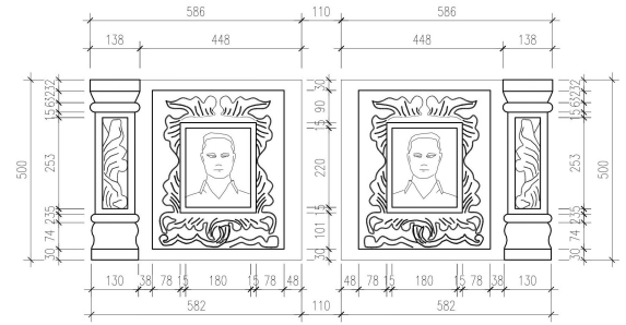
CHI TIẾT LƯNG TRƯỚC MỘ ĐÔI
