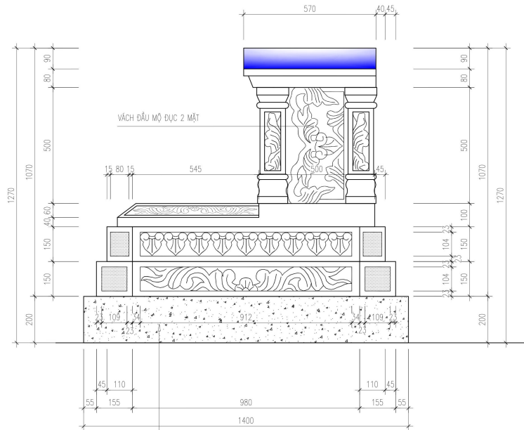
MẶT ĐÚNG HÔNG
