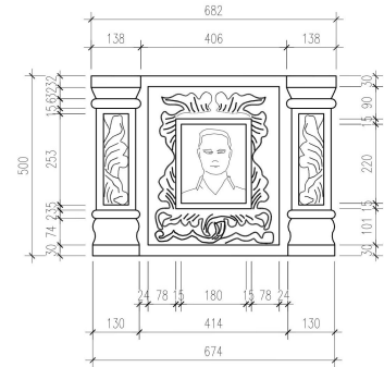
CHI TIẾT LƯNG TRƯỚC MỘ ĐƠN
