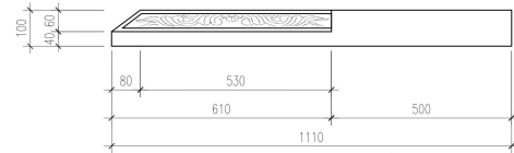
MẶT ĐỨNG BÊN NẮP MỘ
