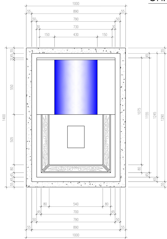
MẶT BẰNG
