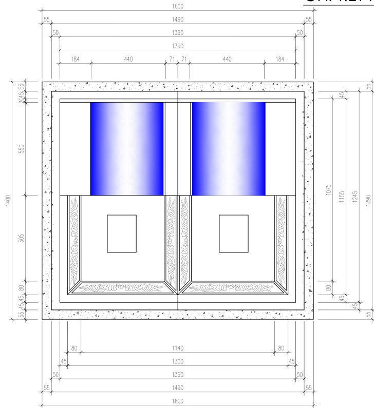
MẶT BẰNG
