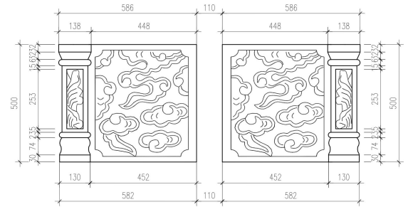
CHI TIẾT LƯNG SAU MỘ ĐÔI
