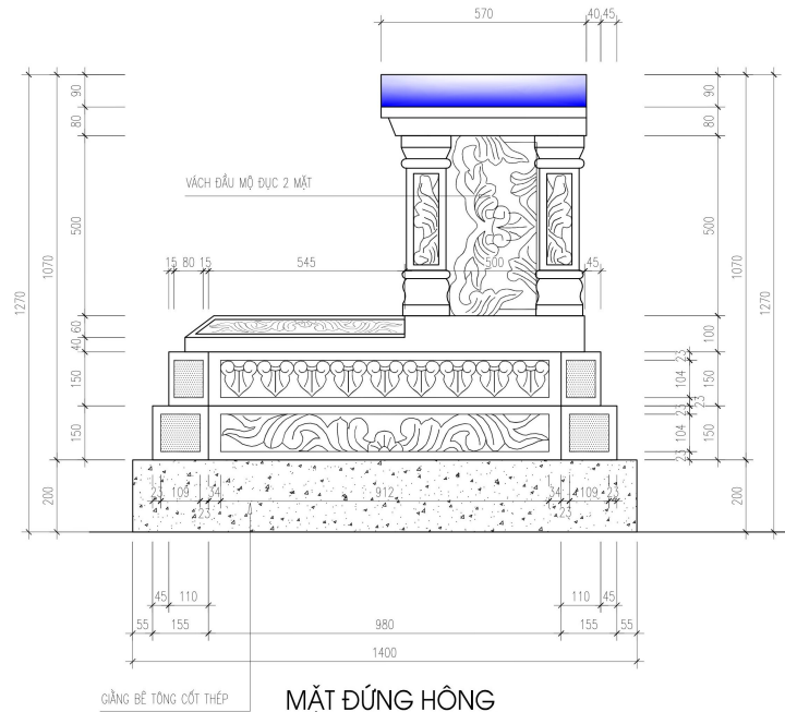
MẶT ĐÚNG HÔNG
