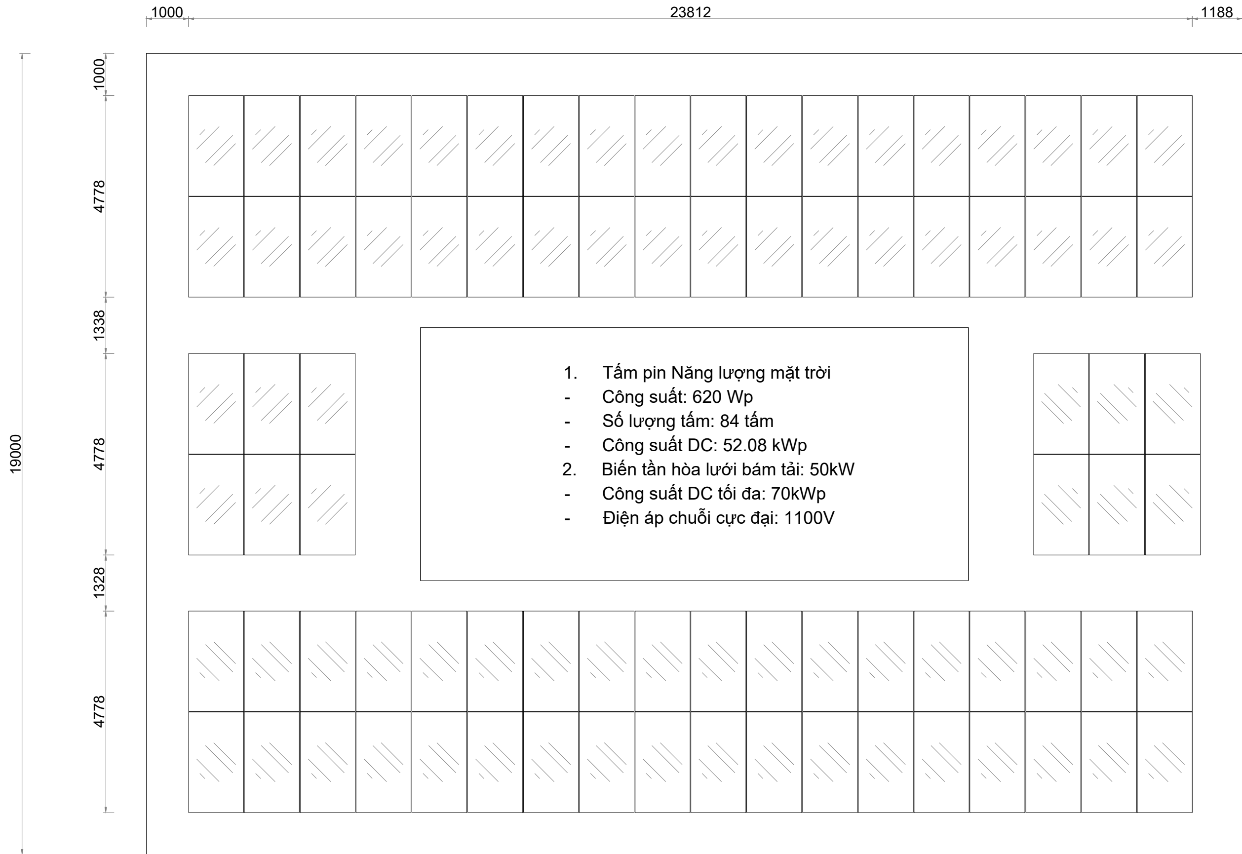
MẶT BẰNG LẮP PIN NHÀ KHO
