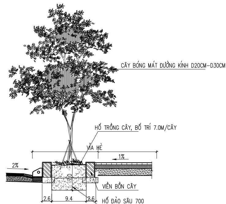
MẶT CẮT ĐIỂN HÌNH TRỒNG CÂY XANH BÓNG MÁT TRÊN VỈA HÈ (SỐ LƯỢNG: 100 CÂY) (LOẠI CÂY: 25 CÂY SẦU CÂY SẦU, XOÀI, BÀNG ĐÀI LOAN , CÂY HOA BAN...)
