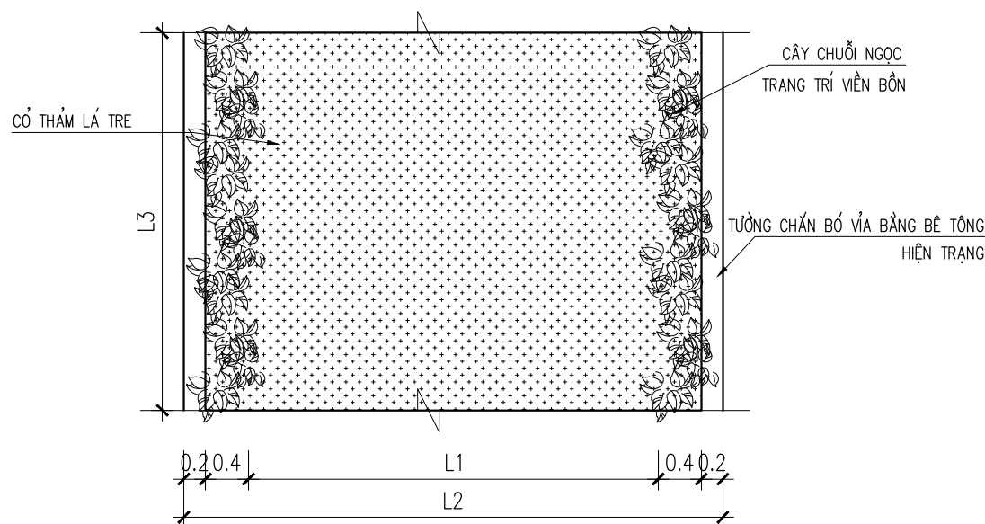
MẶT BẰNG ĐIỂN HÌNH KHU VỰC TRỒNG CỎ LÁ TRE (DIỆN TÍCH: S=2.980 M2)
