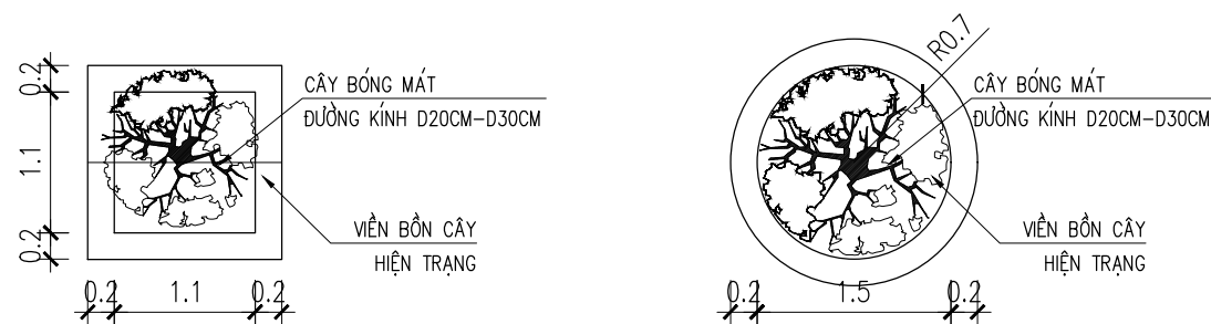
MẶT BẰNG ĐIỂN HÌNH TRỒNG CÂY XANH BÓNG MÁT TRÊN VỈA HÈ (SỐ LƯỢNG: 100 CÂY) (LOẠI CÂY: 25 CÂY SẦU CÂY SẦU, XOÀI, BÀNG ĐÀI LOAN , CÂY HOA BAN...)
