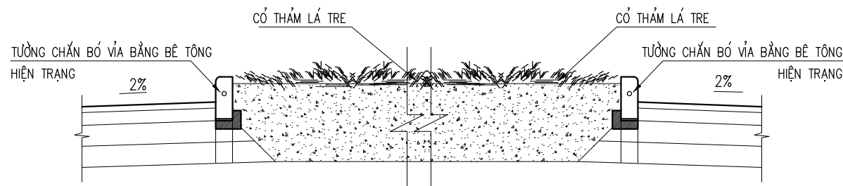
MẶT CẮT ĐIỂN HÌNH KHU VỰC TRỒNG CỎ LÁ TRE (DIỆN TÍCH: S=2.980 M2)
