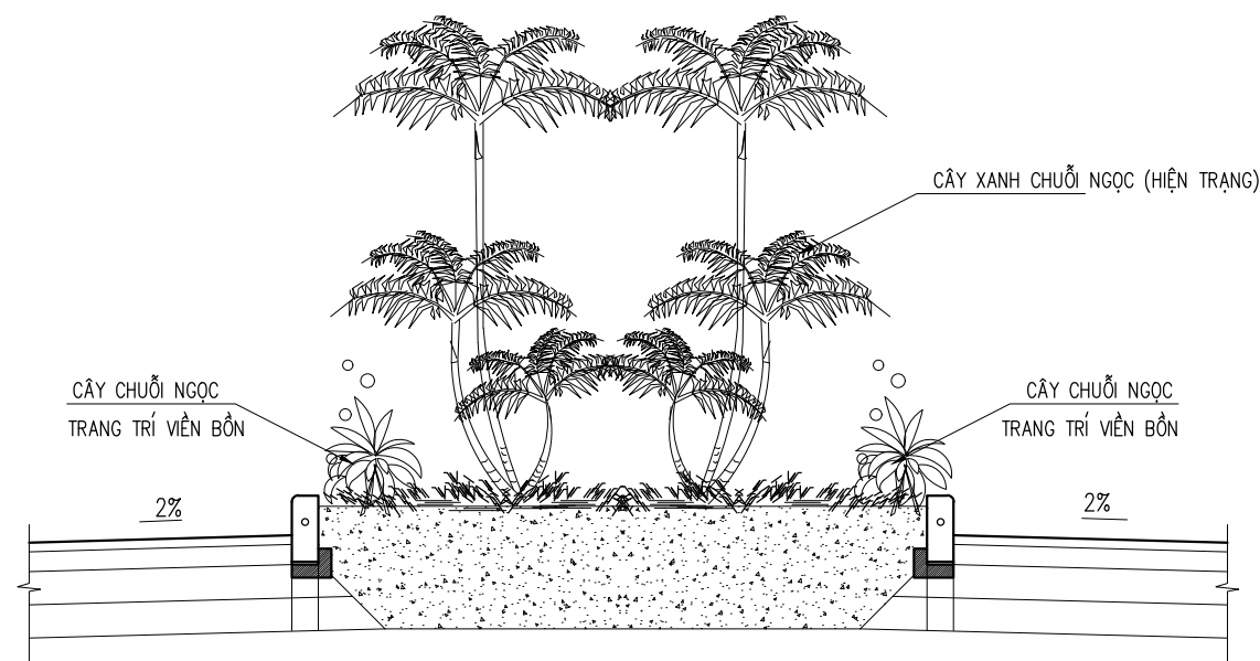
MẶT CẮT ĐIỂN HÌNH KHU VỰC TRỒNG CÂY CÂY CHUỐI NGỌC TRANG TRÍ VIÊN BỒN (SỐ LƯỢNG : 695 M2 )
