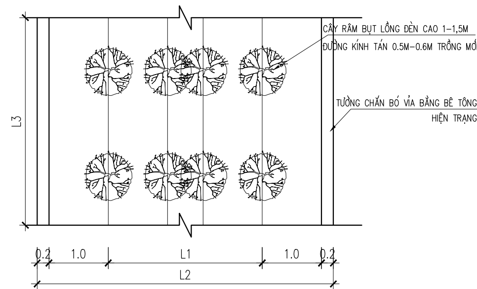
MẶT BẰNG ĐIỂN HÌNH KHU VỰC TRỒNG CÂY RÂM BỤT (SỐ LƯỢNG : 500 CÂY)
