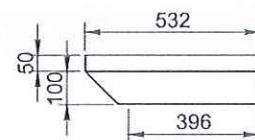
mặt cạnh
