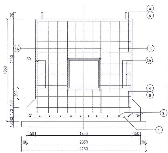
MẶT ĐÚNG MÓNG
