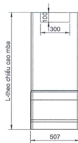
mặt đứng
