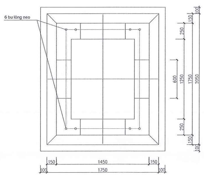
MẶT BẰNG MÓNG
