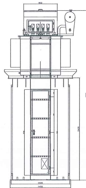
MẶT BÊN PHÍA THANG CẤP HẠ THỂ
