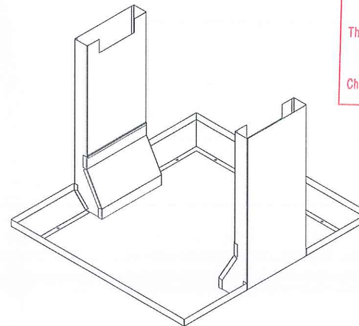
máng cáp trung-hạ áp-máng thu dầu
