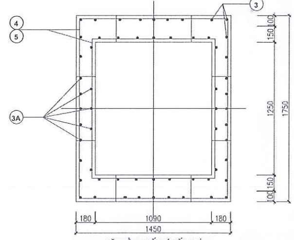
MẶT BẰNG BỐ TRÍ CỐT THÉP
