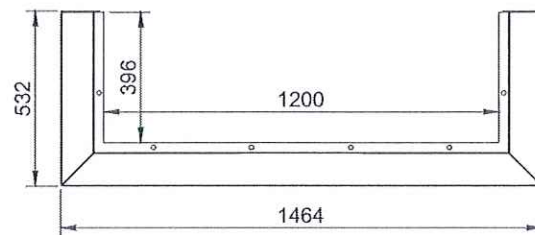
mặt bằng
