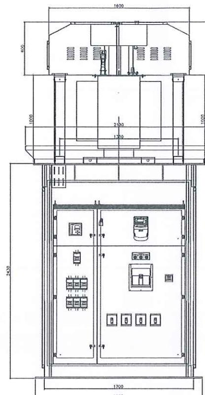
MẶT CÁN TRONG PHÍA TỦ HẠ THỂ
