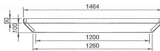
mặt đứng
