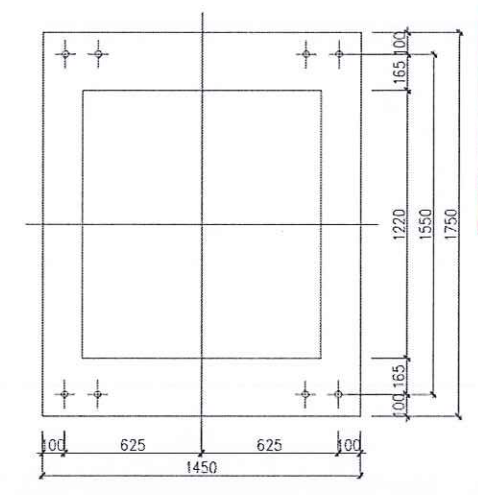
BỐ TRÍ BU LÔNG
