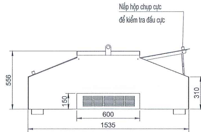
mặt đứng
