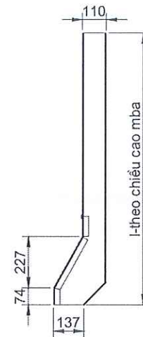
mặt cạnh
