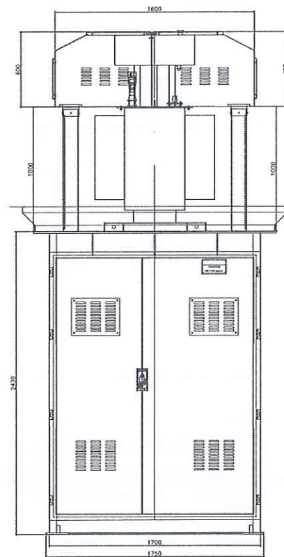
MẶT PHÍA TỦ TRUNG THỂ
