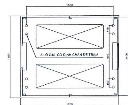
MẶT PHÍA TỦ TRUNG THỂ
