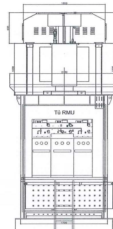
MẶT PHÍA TỦ TRUNG THỂ
