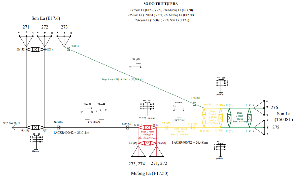
Hình ảnh: Sơ đồ thứ tự pha Đường dây 220kV 500kV Sơn La – Sơn La
