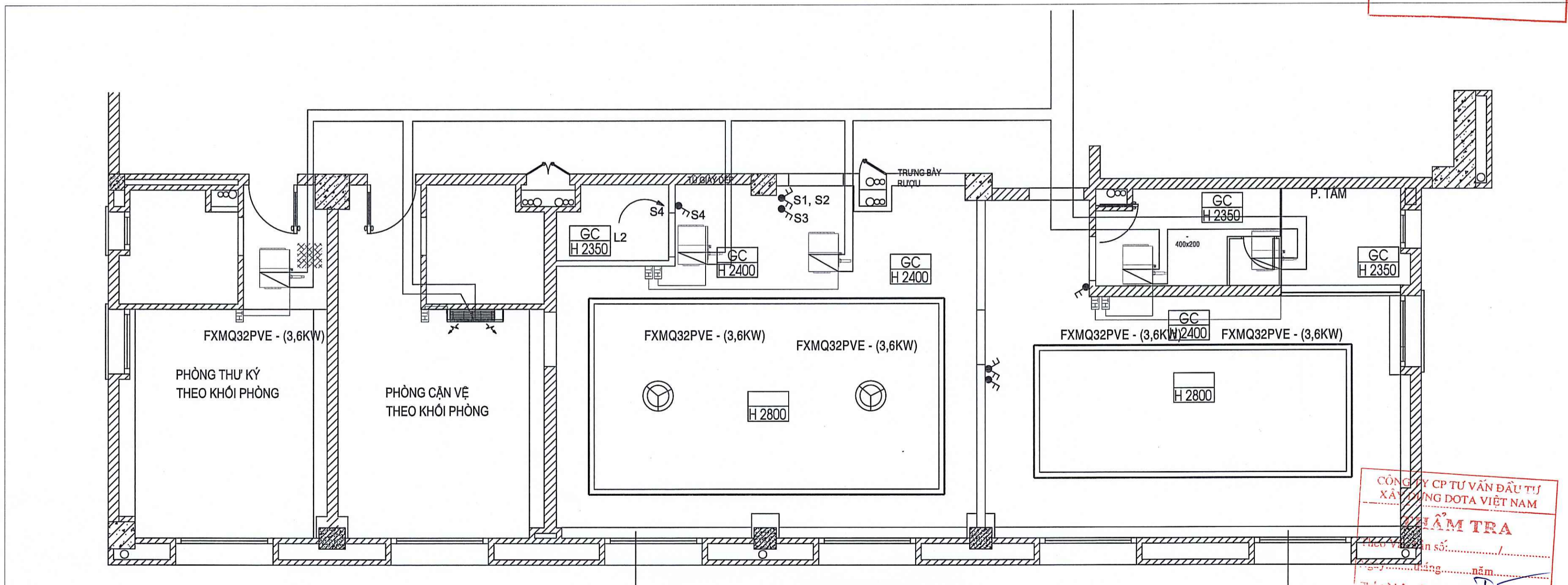
MẶT BẰNG BỐ TRÍ ỚNG GIÓ PHÒNG PRESIDENT
