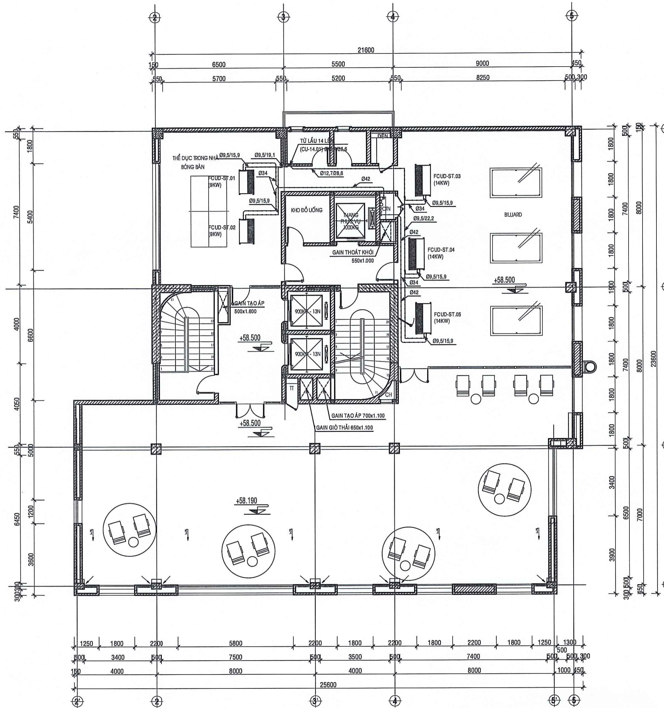
MẶT BẰNG CẢI TẠO ĐHKK SÂN THƯỢNG
