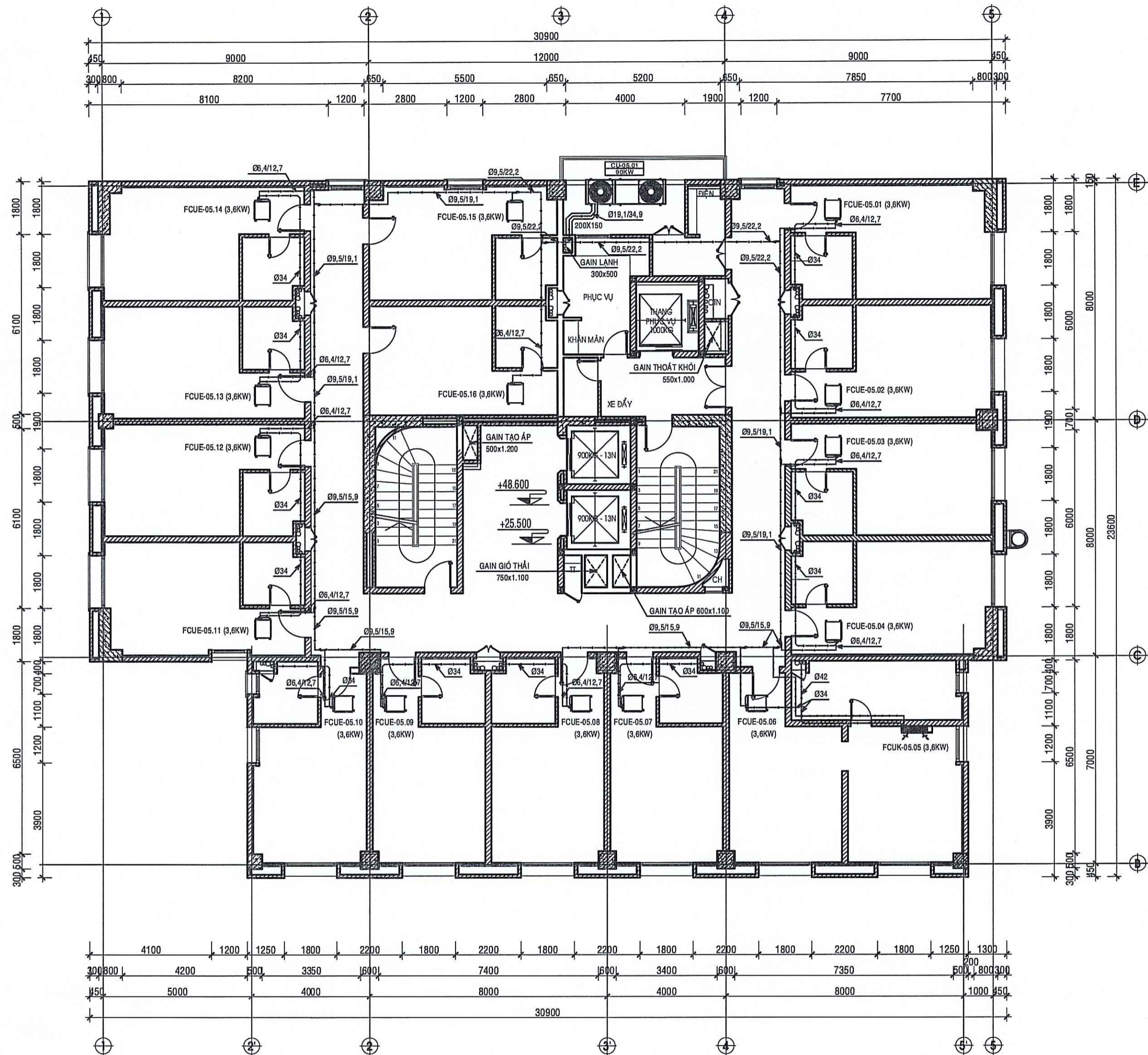
MẶT BẰNG CẢI TẠO ĐHKH LẦU 5-7-9-11
