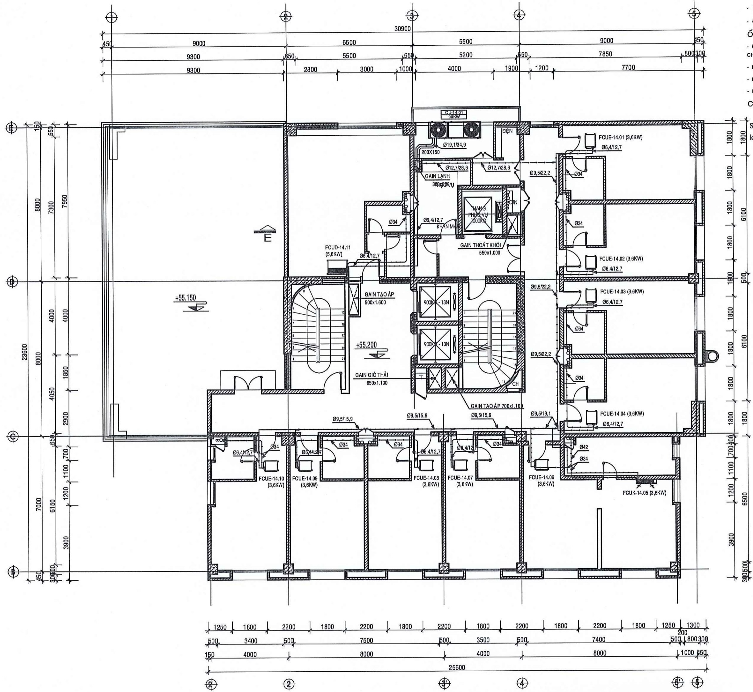
MẶT BẰNG CẢI TẠO ĐHKHK LẦU 14
