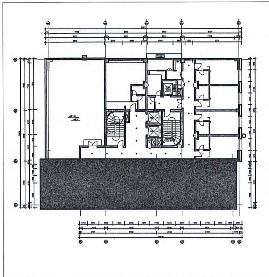
MẶT BẰNG ĐỊNH VỊ PHÒNG PRESIDENT LẦU 14
