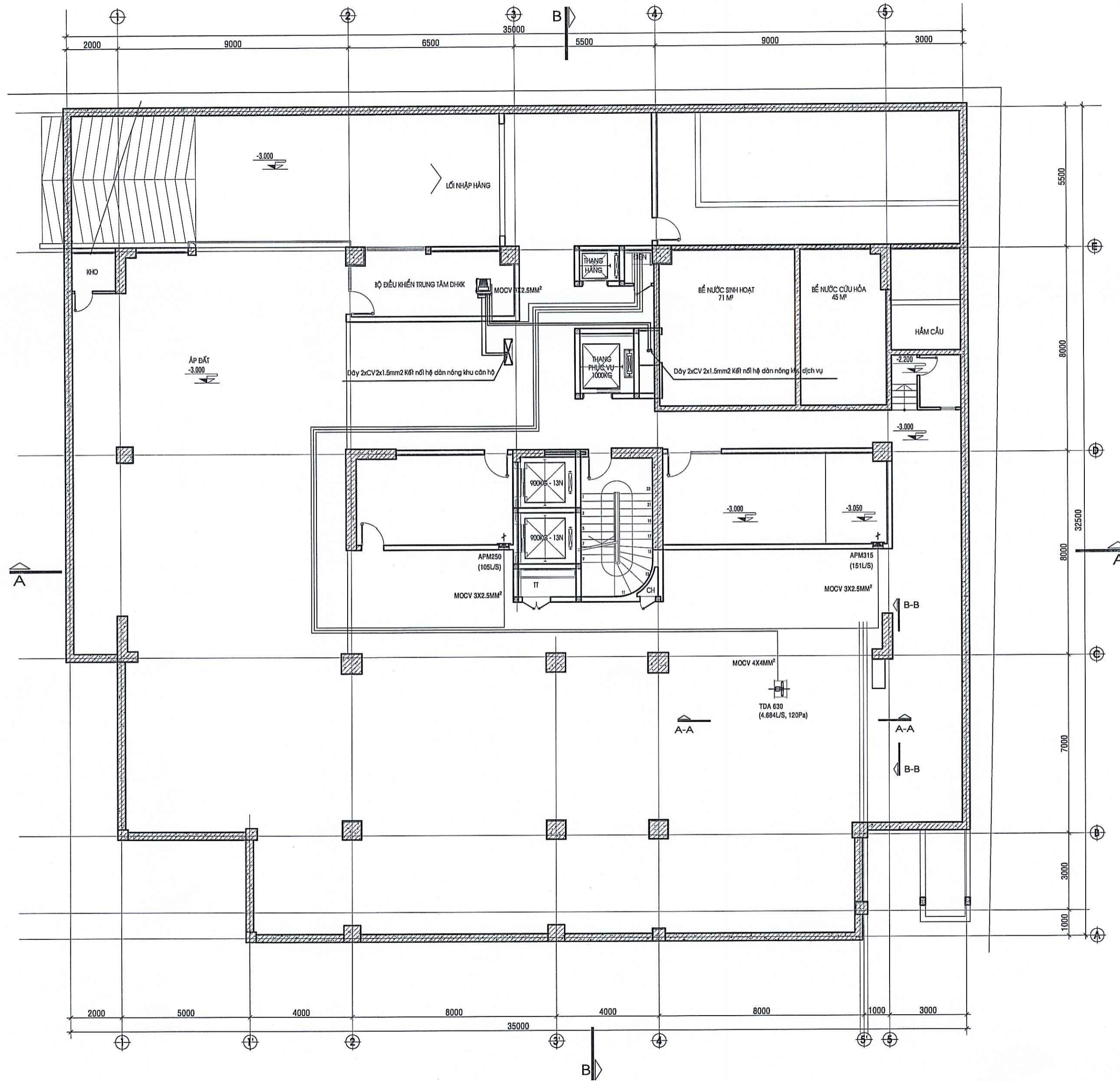
MẶT BẰNG TẦNG ÁP ĐẤT
