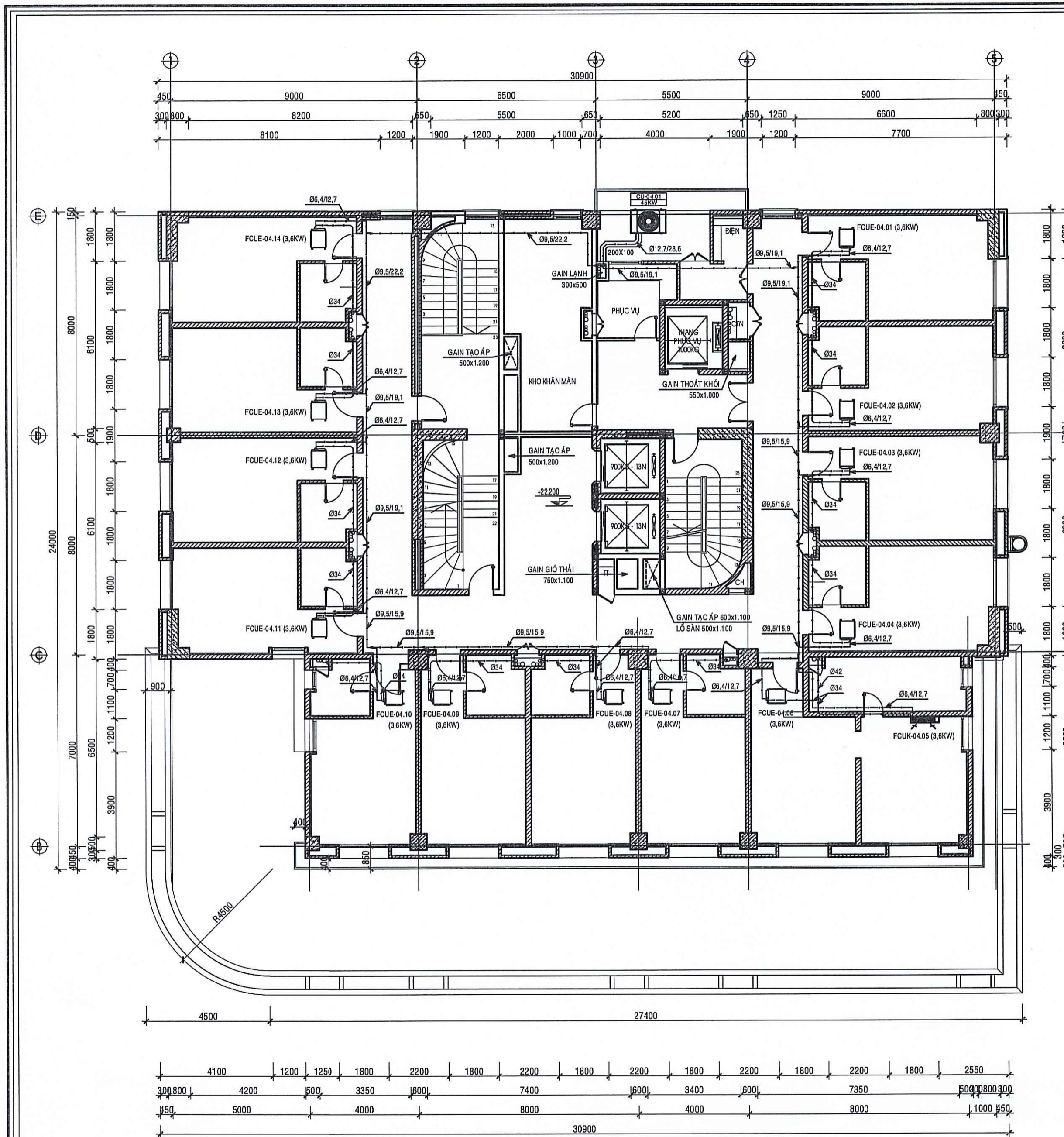
MẶT BẰNG CẢI TẠO ĐHKH LẦU 4
