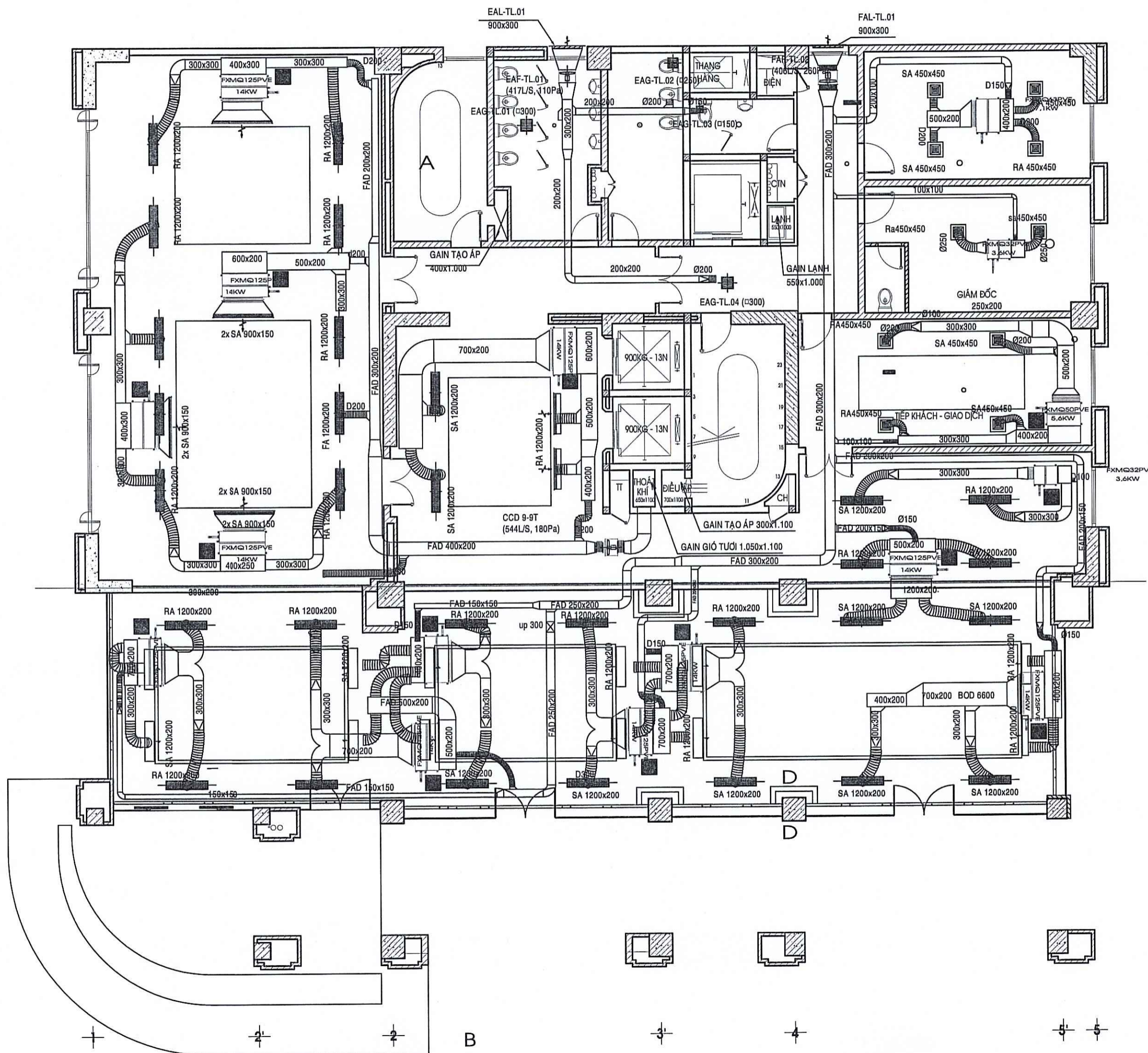
MẶT BẰNG TRẦN LỬNG
