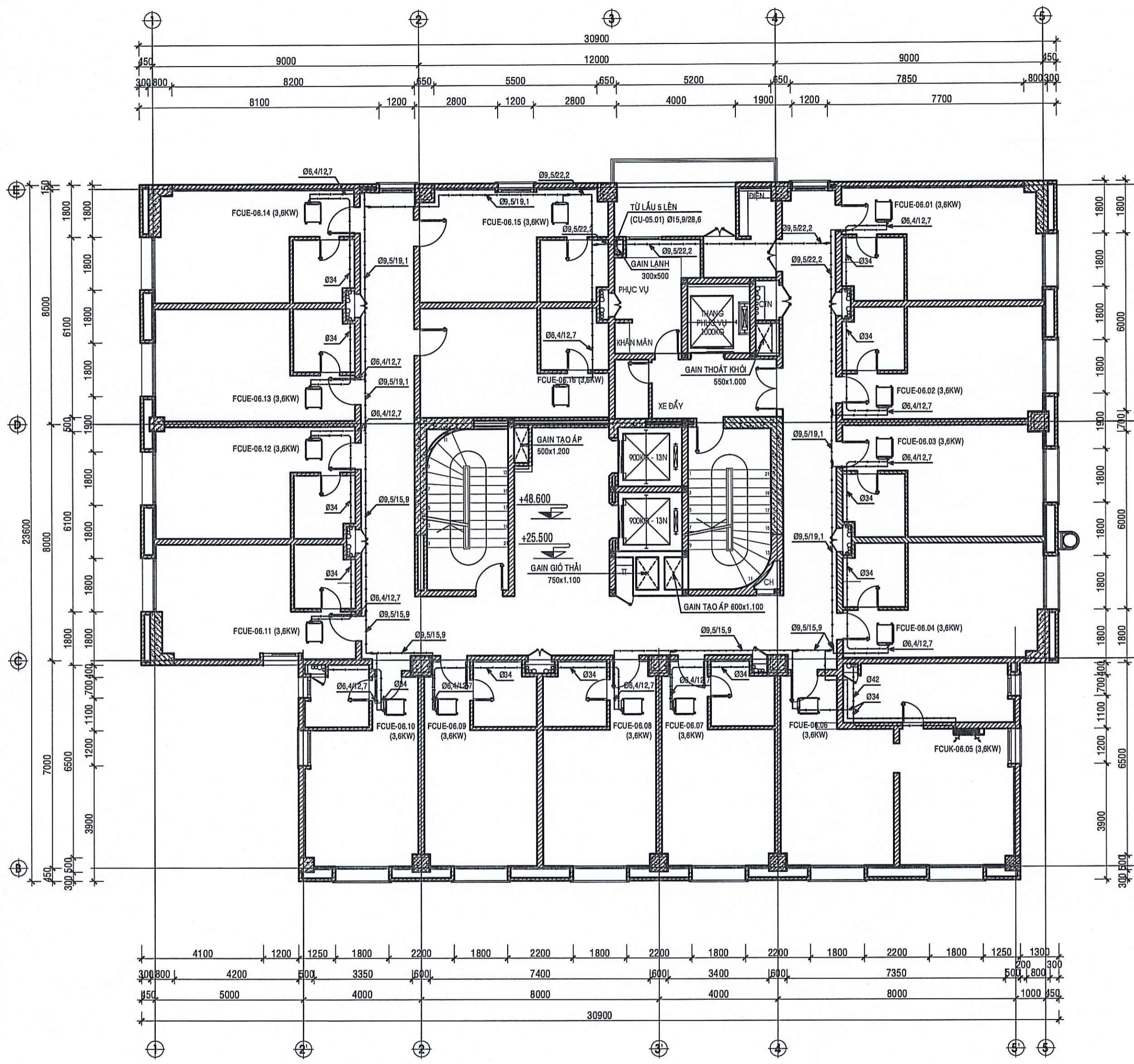
MẶT BẰNG CẢI TẠO ĐHKH LẦU 6-8-10-12
