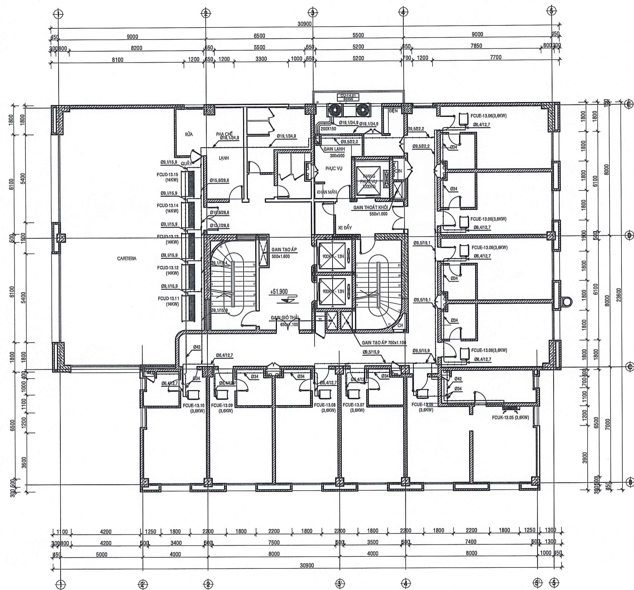
MẶT BẰNG CẢI TẠO ĐHKH LẦU 13
