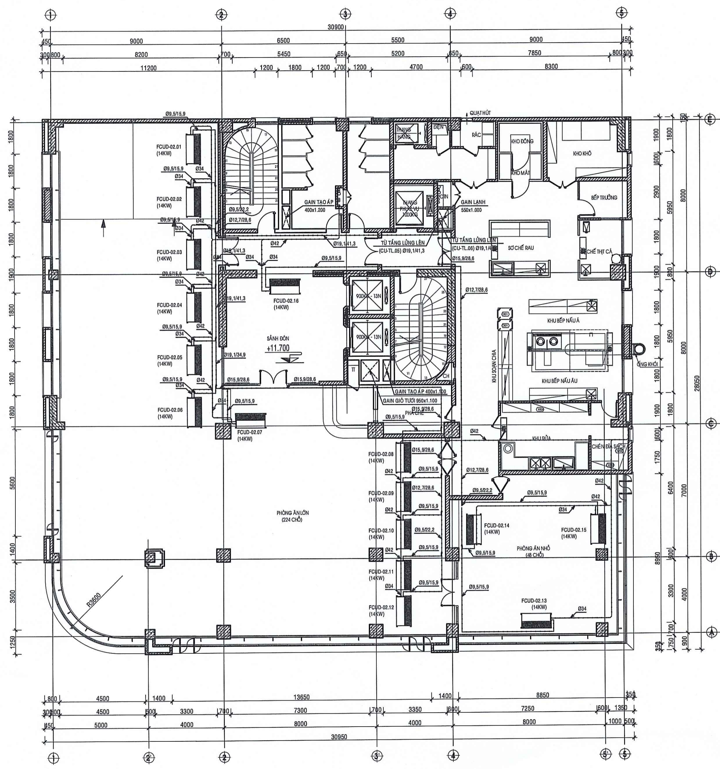
MẶT BẰNG CẢI TẠO ĐHKH LẦU 2
