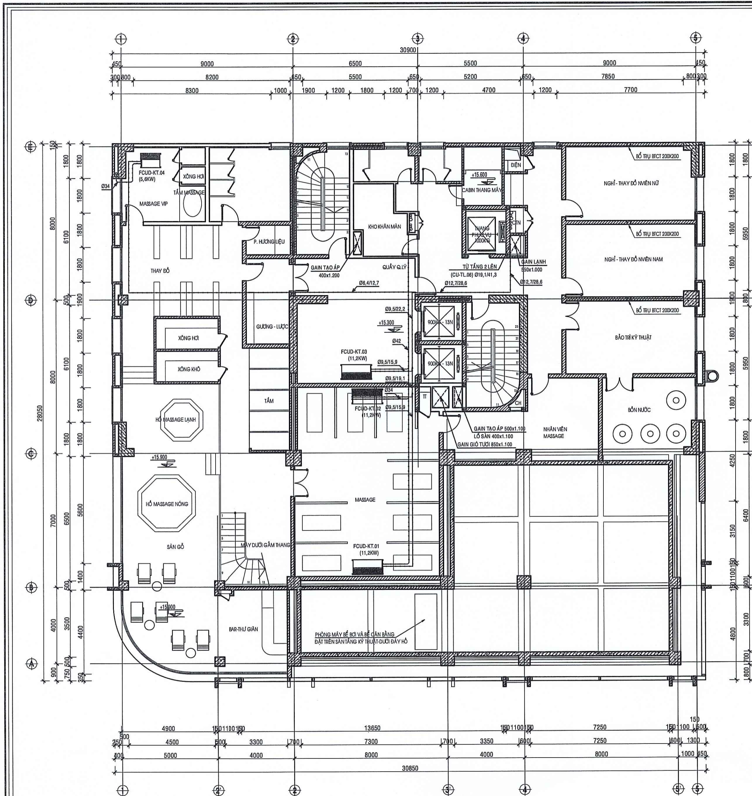
MB CẢI TẠO ĐHKK TẦNG KỸ THUẬT
