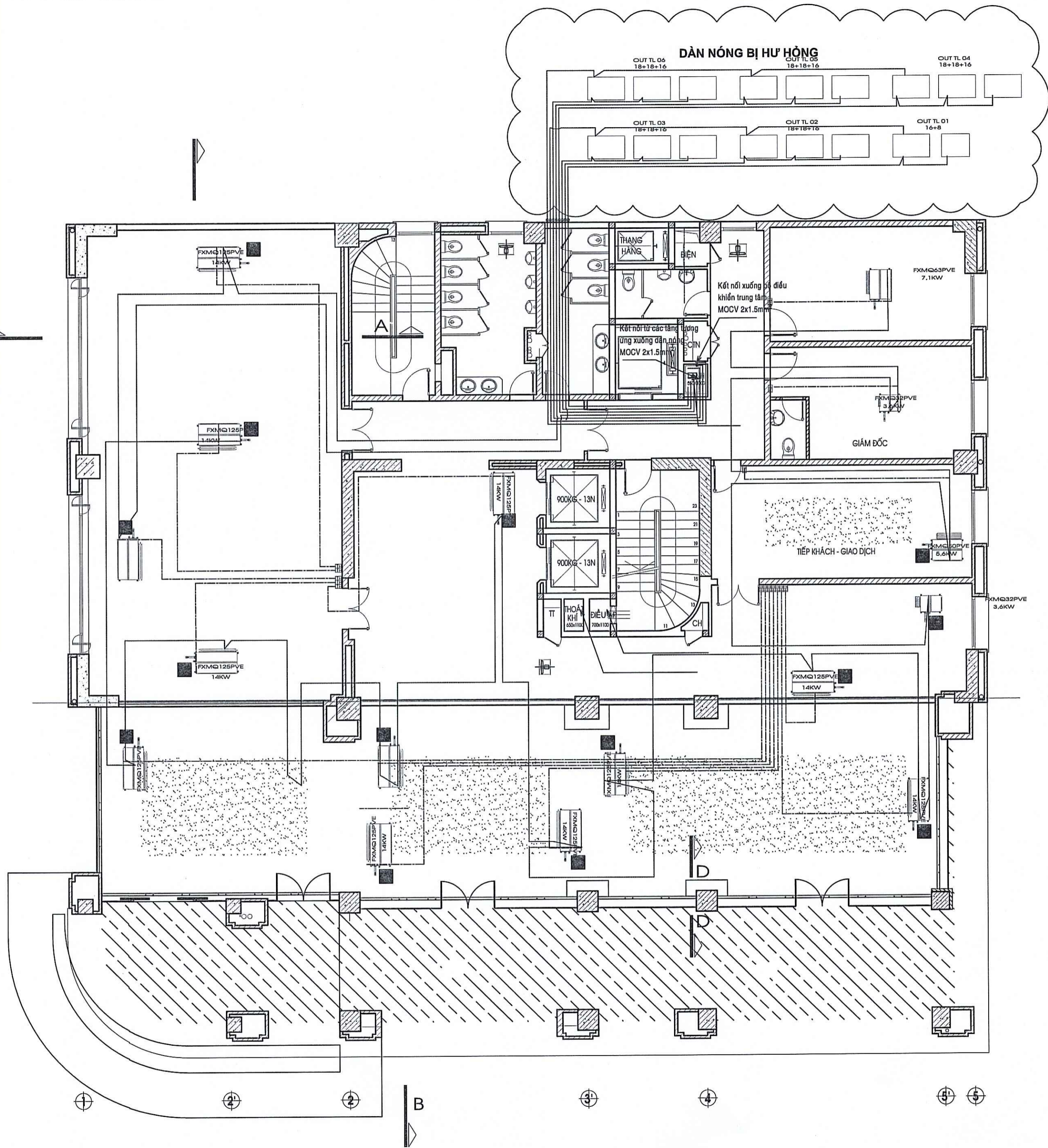
MẶT BẰNG TRẦN LỬNG
