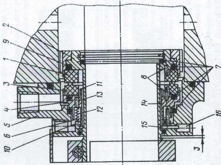
Рис. 1. Торцовое уплотнение БО:
