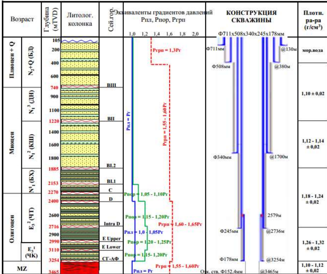
СОВМЕЩЕННЫЙ ГРАФИК ДАВЛЕНИЙ СКВАЖИНЫ № KTN-P3. (По вертикали от роторного стола)
