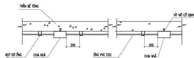
CHI TIẾT LẮP ĐẶT ĐÈN CHỈ DẪN THOÁT HIỂM
