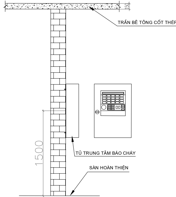
CHI TIẾT LẮP ĐẶT TỦ TRUNG TÂM BÁO CHÁY
