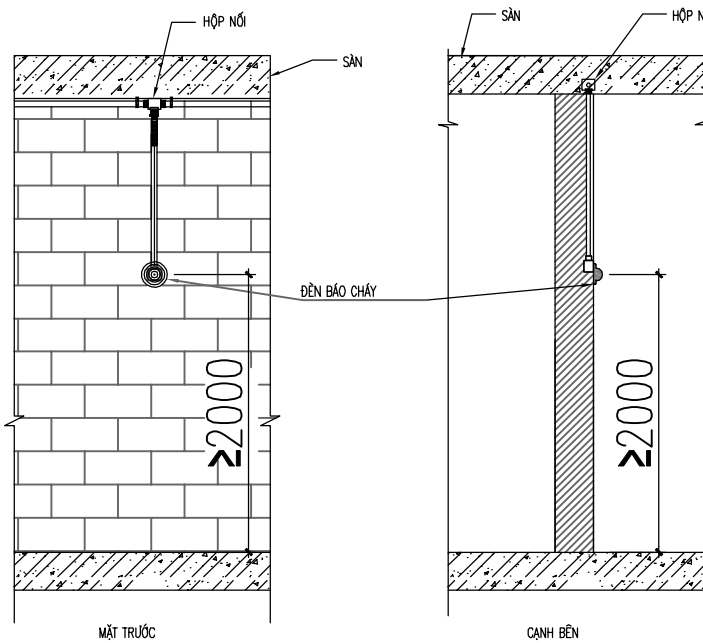
CHI TIẾT LẮP ĐẶT TỔ HỢP CHUÔNG , ĐÈN, NÚT NHẤN BÁO CHÁY
