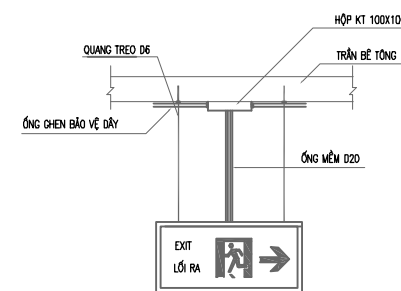
ĐÈN XÍT LOẠI HAI MẶT LOẠI CÓ MŨI TÊN CHỈ PHẢI
