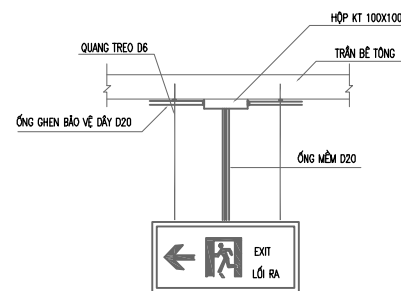
ĐÈN XÍT LOẠI HAI MẶT LOẠI CÓ MŨI TÊN CHỈ TRÁI
