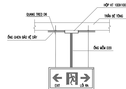
ĐÈN XÍT LOẠI HAI MẶT LOẠI CÓ MŨI TÊN CHỈ 2 BÊN
