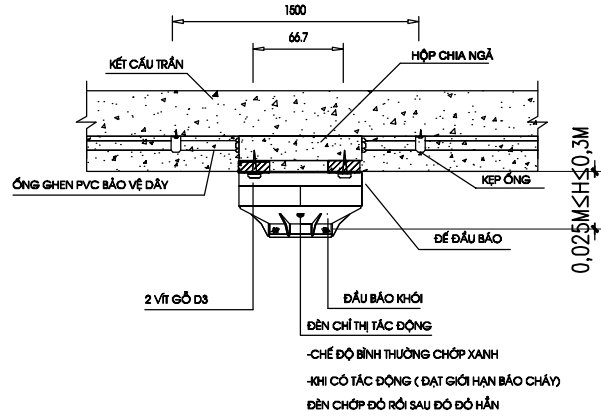
LẮP ĐẶT ĐẦU BÁO KHÓI DƯỚI TRẦN BTCT
