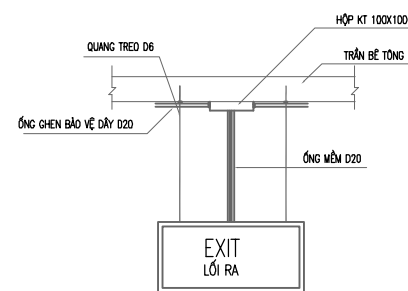
ĐÈN XÍT LOẠI HAI MẶT
