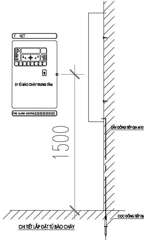
CHI TIẾT LẮP ĐẶT THIẾT BỊ BÁO CHÁY
