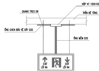
ĐÈN XÍT LOẠI HAI MẶT LOẠI CÓ MŨI TÊN CHỈ 2 CHIỀU
