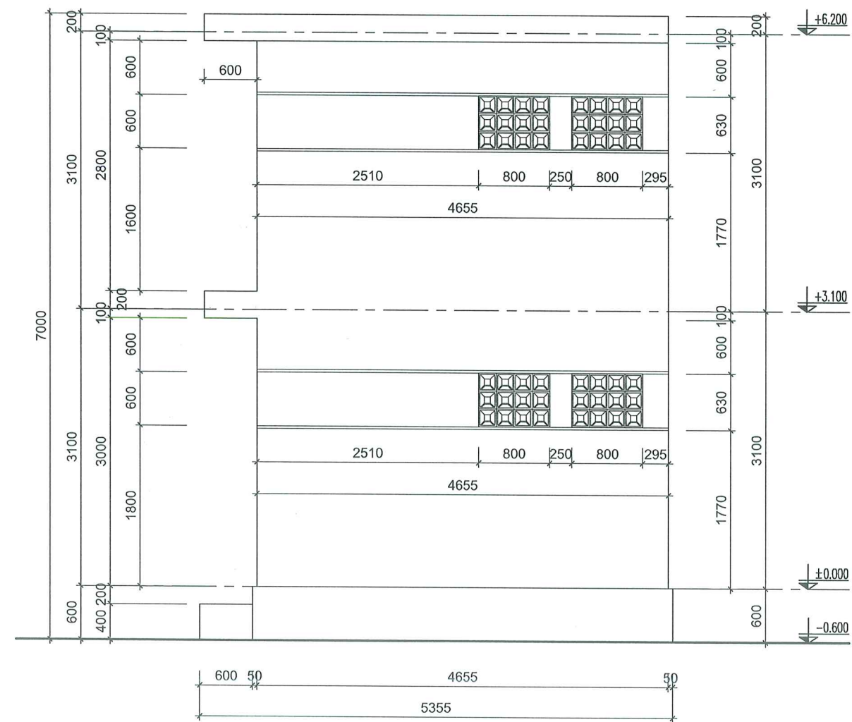
MẶT ĐỪNG BÊN CẢI TẠO TL 1/100
