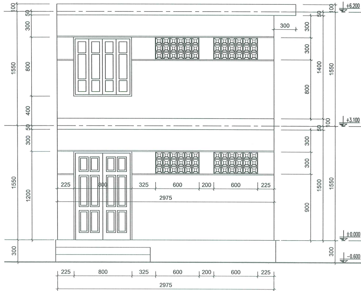
ĐỨNG CHÍNH HIỆN TRẠNG TL 1/100
