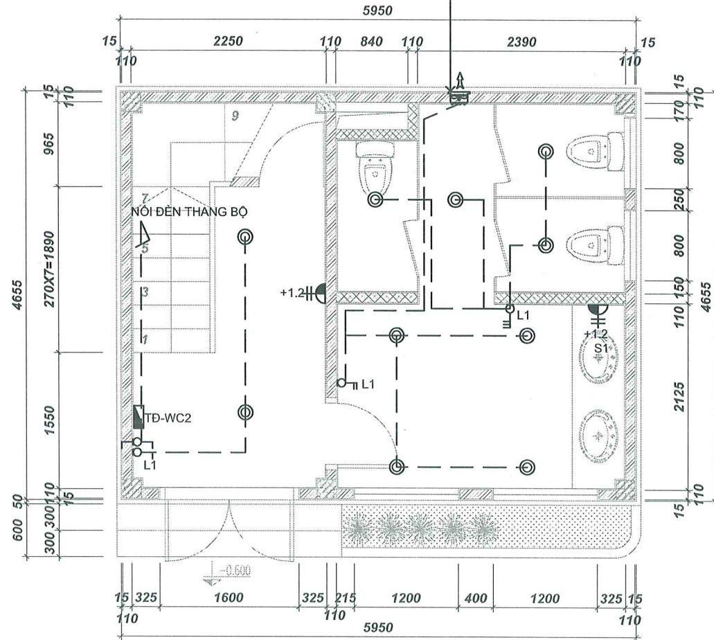
MẶT BẰNG ĐIỆN TẦNG 1 WC CÔNG CỘNG 32 TRẦN QUỐC TOẢN
