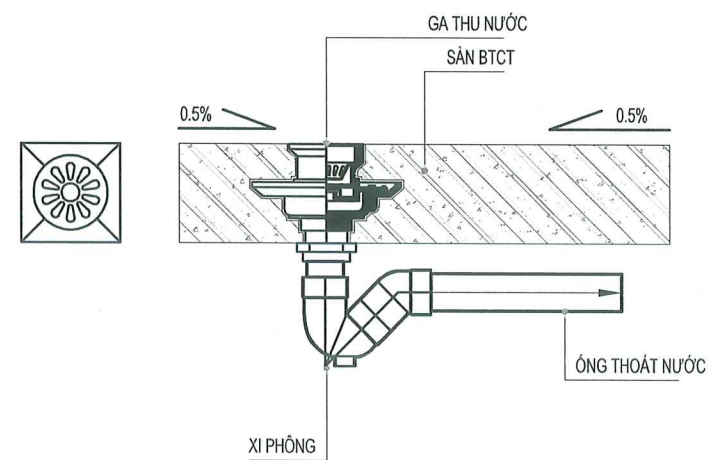
CHI TIẾT LẮP ĐẶT GA THU NƯỚC SÀN
