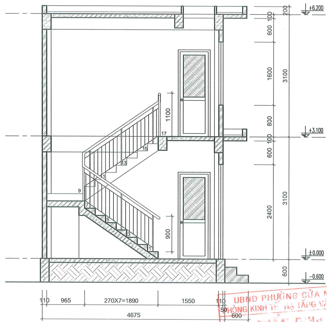
MẶT CẮT B-B TL 1/100
