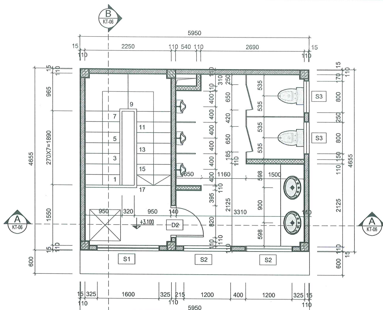
MẶT BẰNG CẢI TẠO TẦNG 2 TL 1/100
