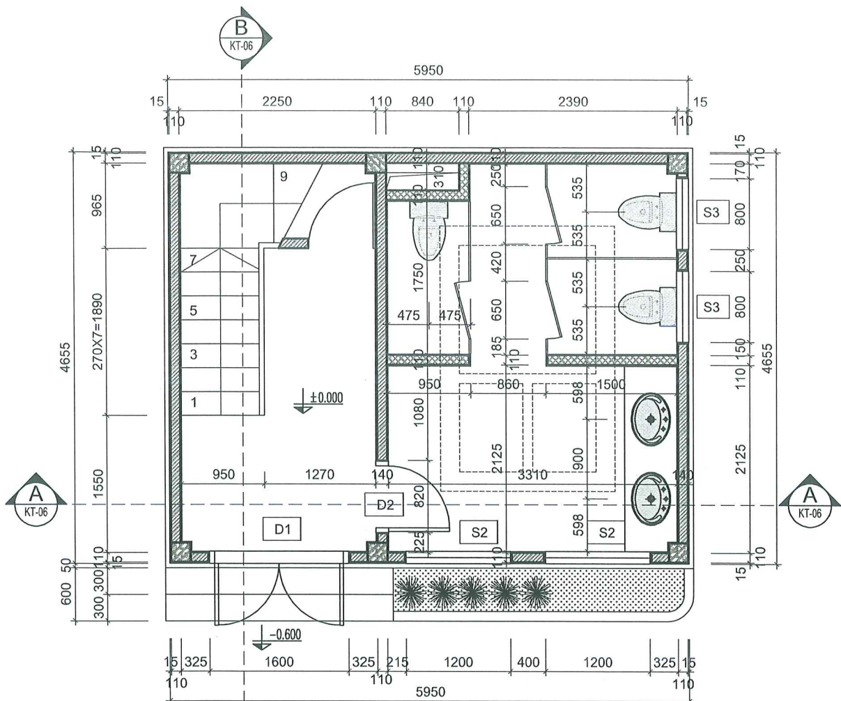
MẶT BẰNG CẢI TẠO TẦNG 1 TL 1/100
