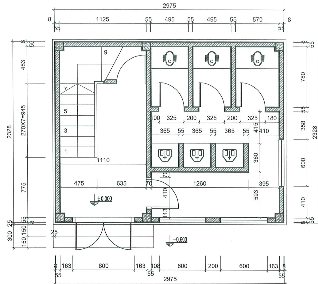
MẶT BẰNG HIỆN TRẠNG TẦNG 1 TL 1/100
