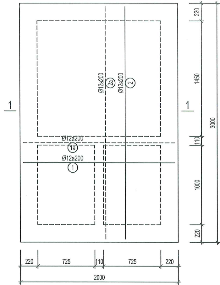
MẶT BẰNG ĐÁY BỀ PHỐT
