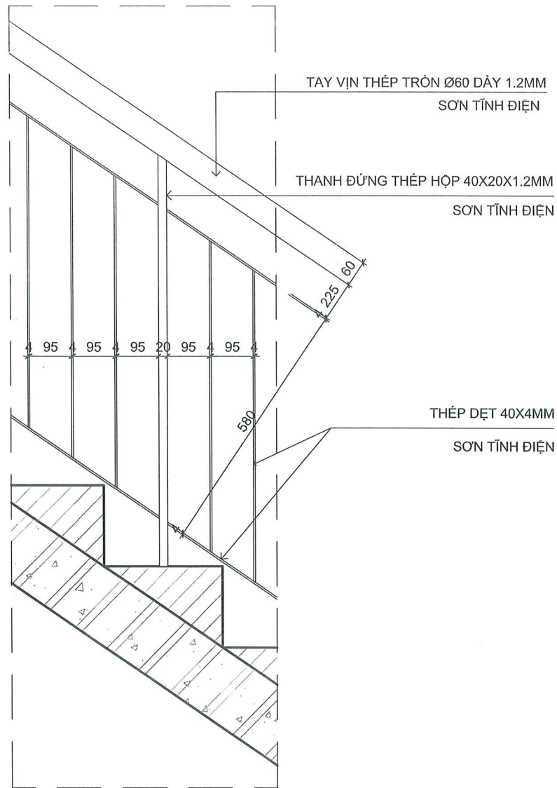
CHI TIẾT LAN CAN CẦU THANG TL 1/10
