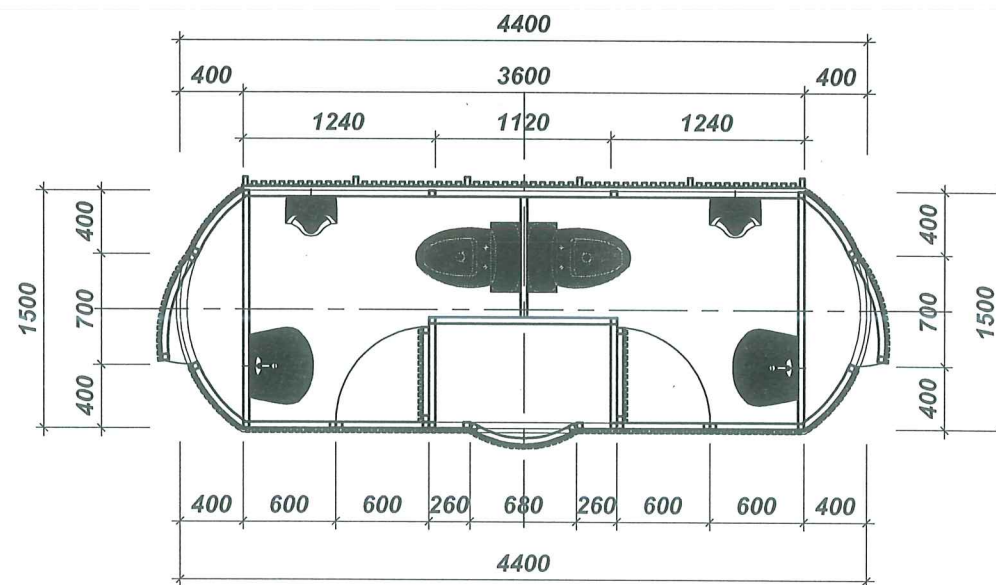
MẶT BẰNG CẢI TẠO
