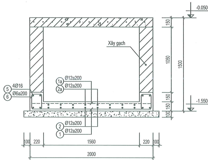
MẶT CẮT 1-1
