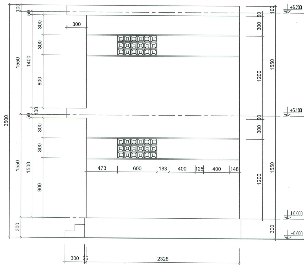
MẶT ĐỨNG BÊN HIỆN TRẠNG TL 1/100
