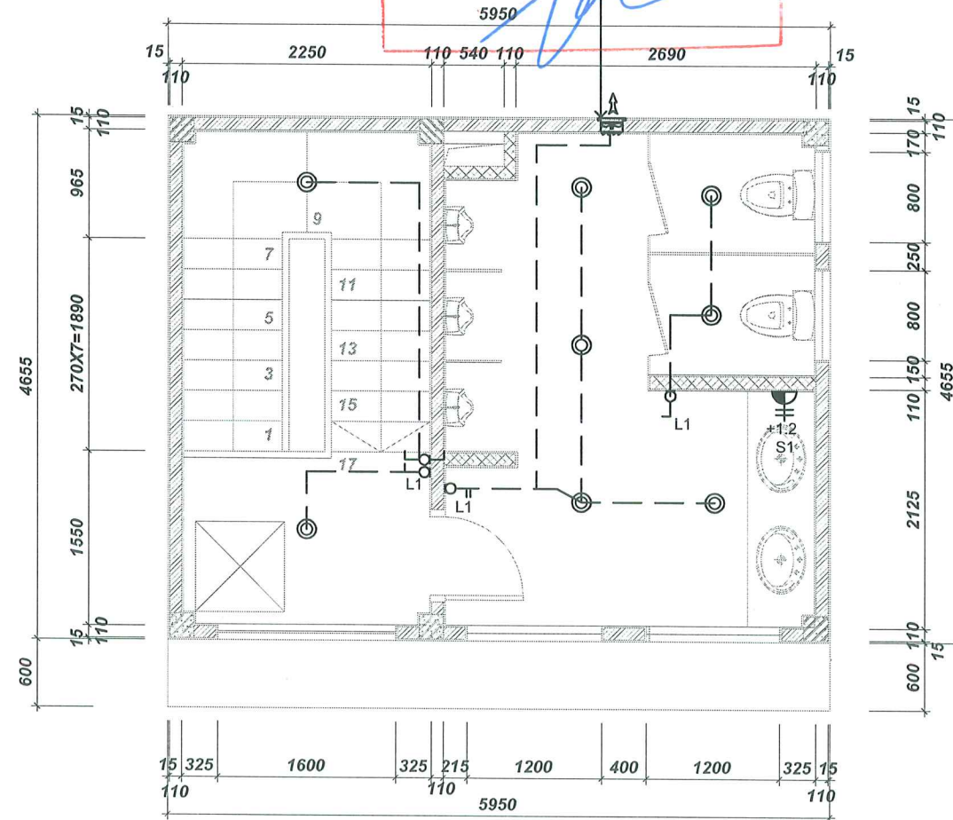
MẶT BẰNG ĐIỆN TẦNG 2 WC CÔNG CỘNG 32 TRẦN QUỐC TOẢN
