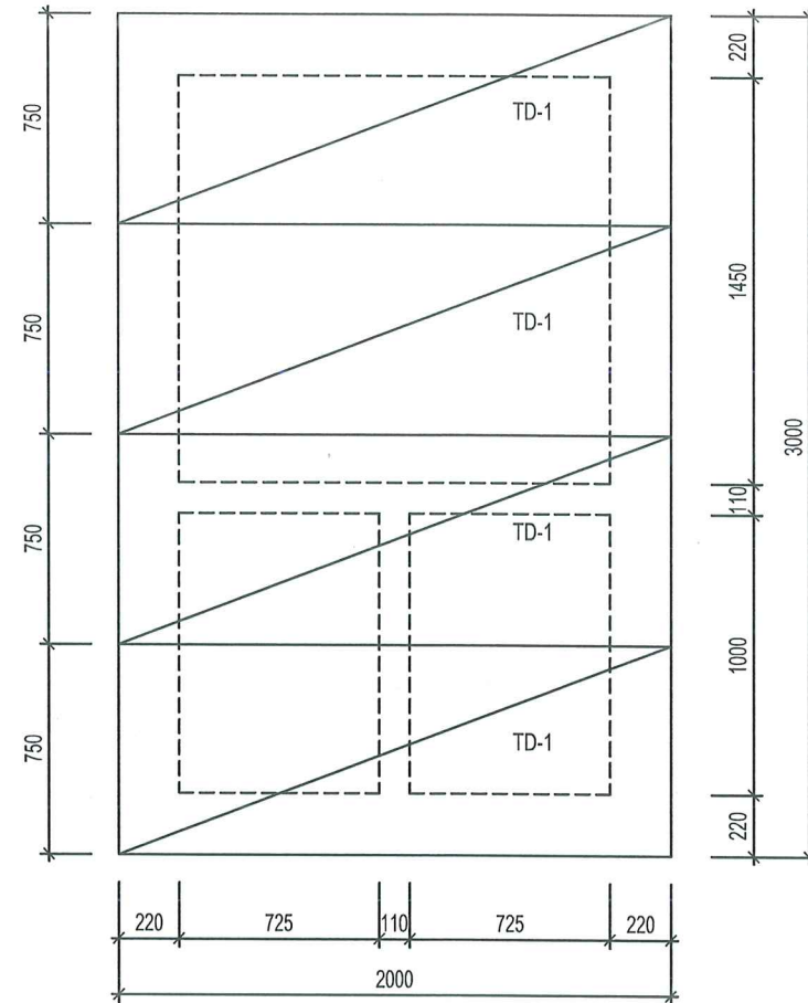
MẶT BẰNG NẤP BỀ PHỐT
