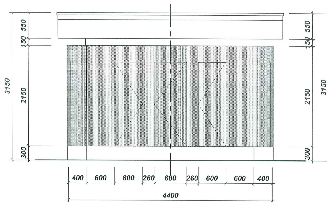
MẶT BẰNG ĐỨNG HIỆN TRẠNG
