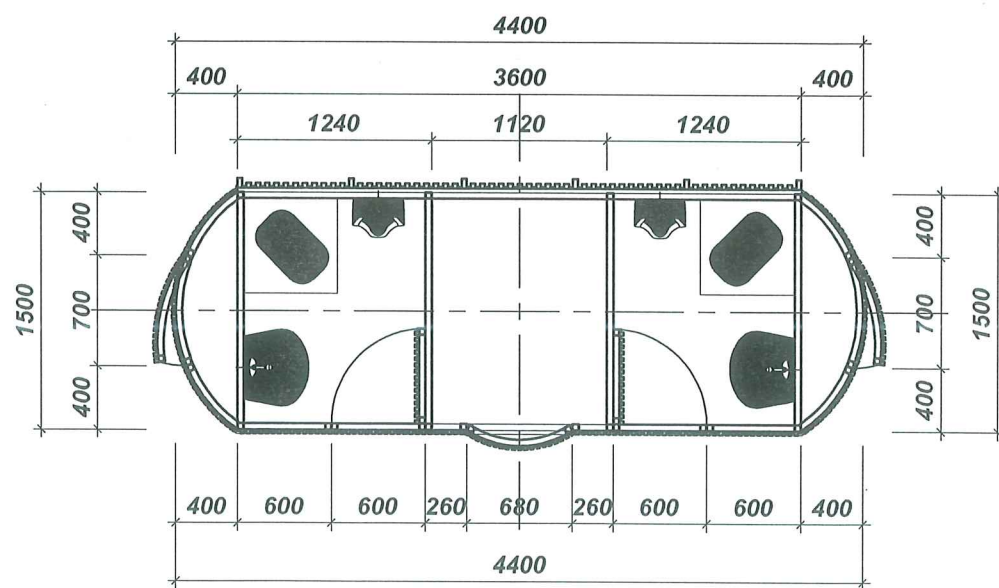
MẶT BẰNG HIỆN TRẠNG
