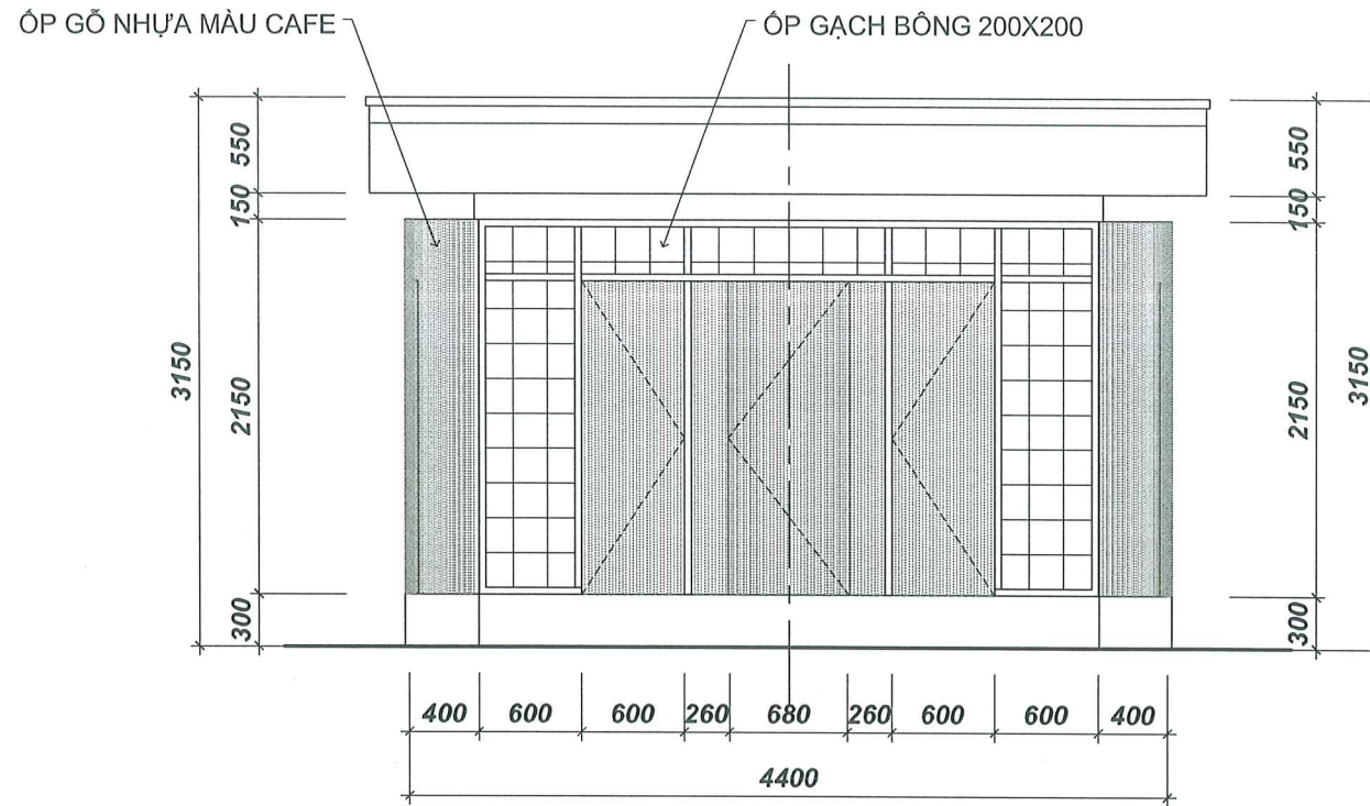
MẶT ĐỨNG CẢI TẠO
