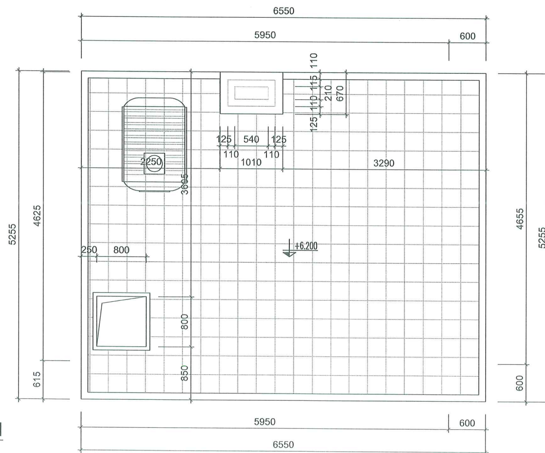
MẶT BẰNG CẢI TẠO TẦNG 2 TL 1/100
