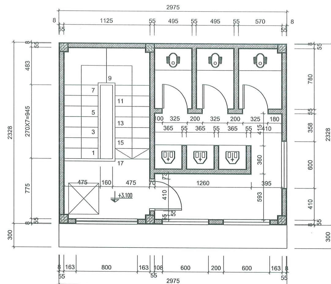
MẶT BẰNG HIỆN TRẠNG TẦNG 2 TL 1/100
