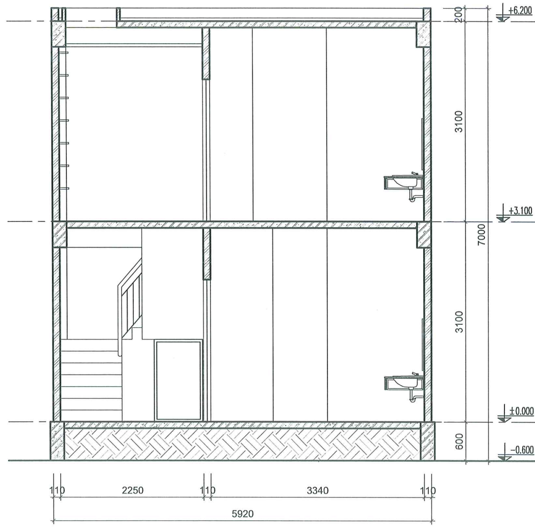
MẶT CẮT A-A TL 1/100
