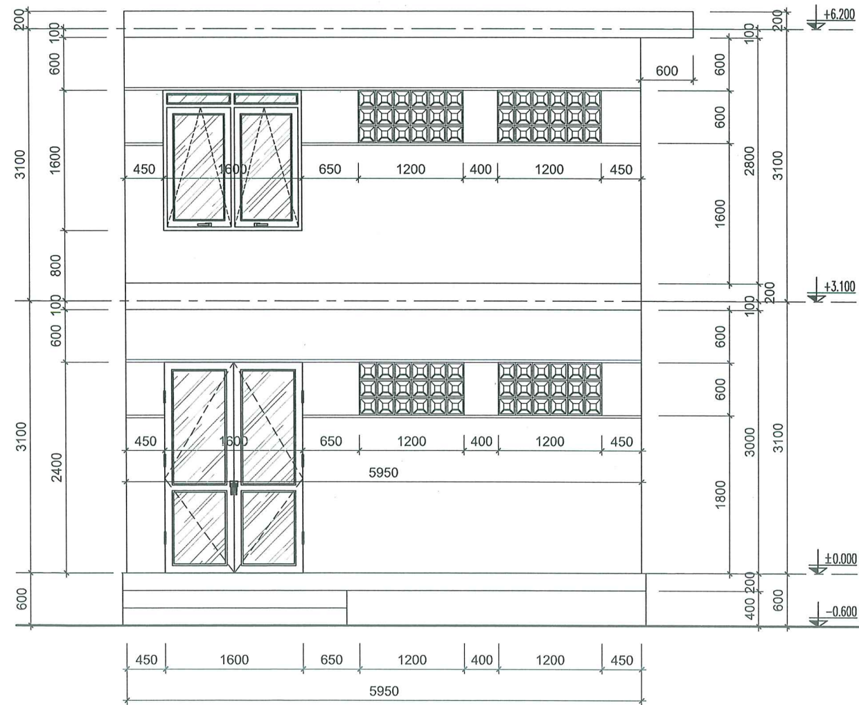
ĐỪNG CHÍNH CẢI TẠO TL 1/100
